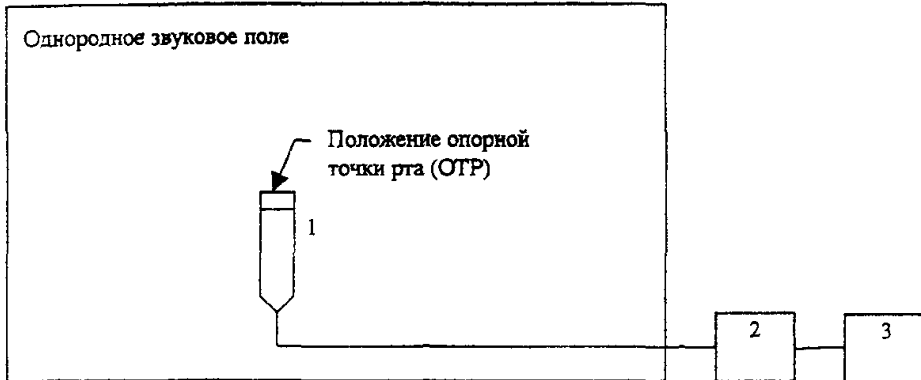
Измерение однородного звукового поля в ОТР
