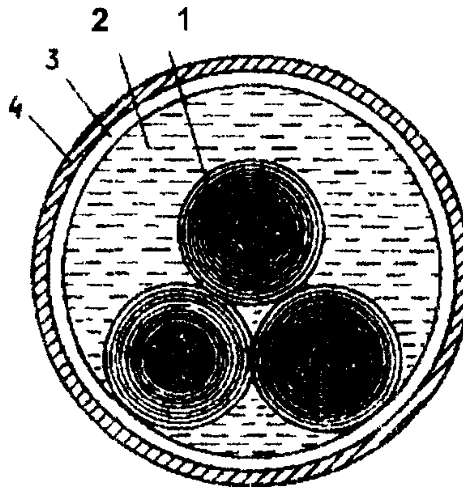
Рис 3 Схема маслонаполненного кабеля высокого давления
