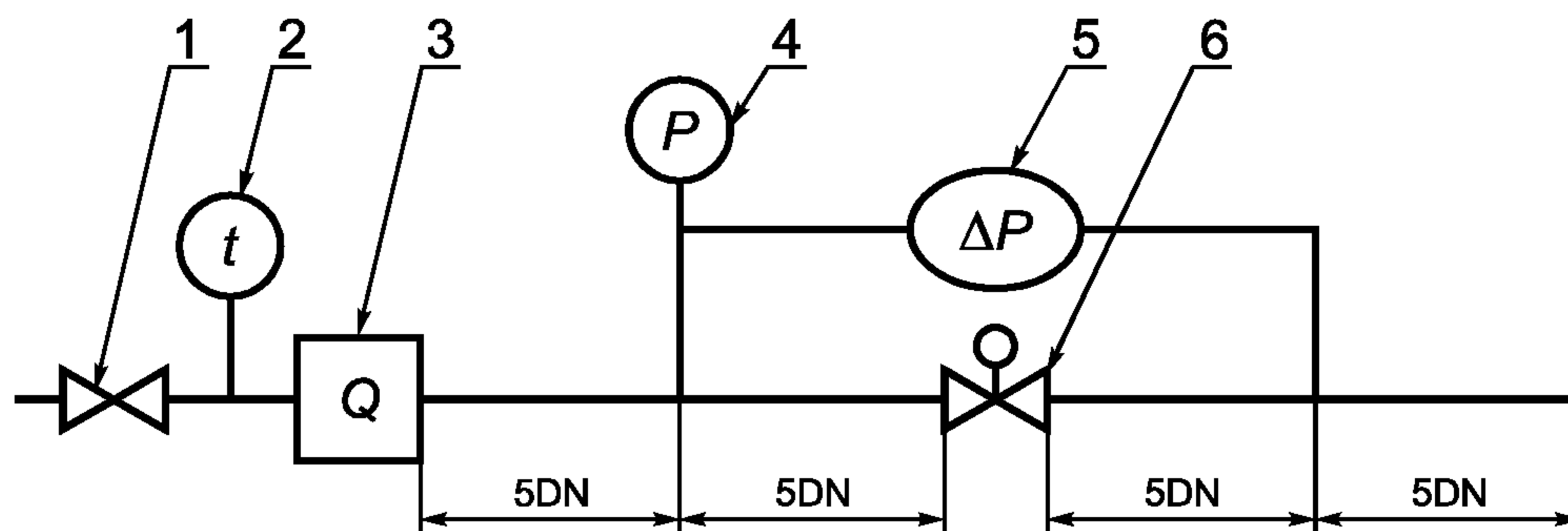
1 — регулятор расхода; 2 — термометр; 3 — расходомер или счетчик расхода газа; 4 — манометр; 5 — дифманометр; 6 — испытываемый КТЗ
