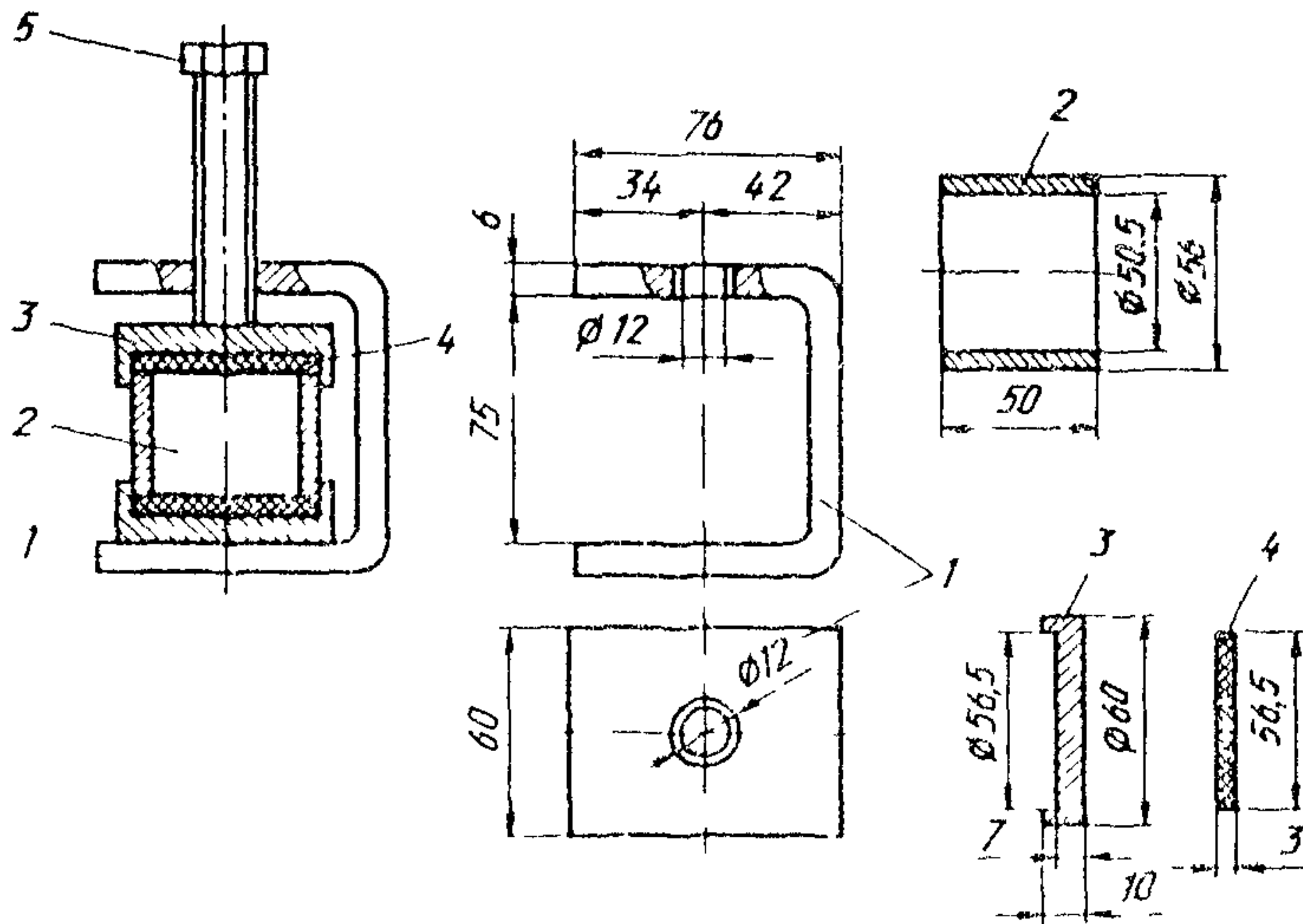
Рис. 13. Обойма для прогрева цементогрунтовых образцов: 1 - струбцина; 2 - кольцо; 3 - крышка; 4 - резиновая прокладка; 5 - болт
