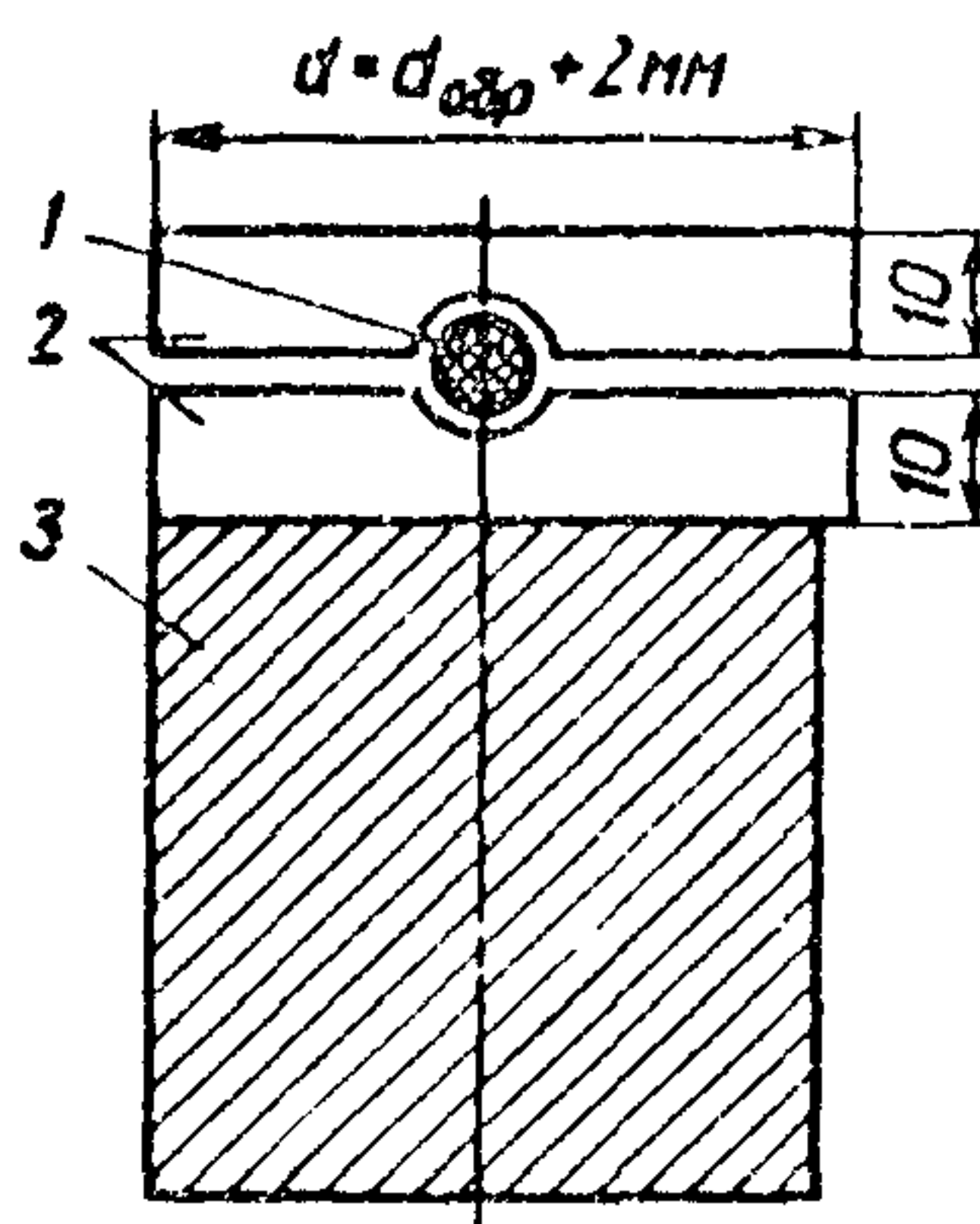
Рис.9. Схема шарнирного устройства: 1 - шарик стальной диаметром 6-8 мм; 2 - металлические пластинки диаметром d ; 3 - образец укрепленного грунта диаметром d_{обр}
