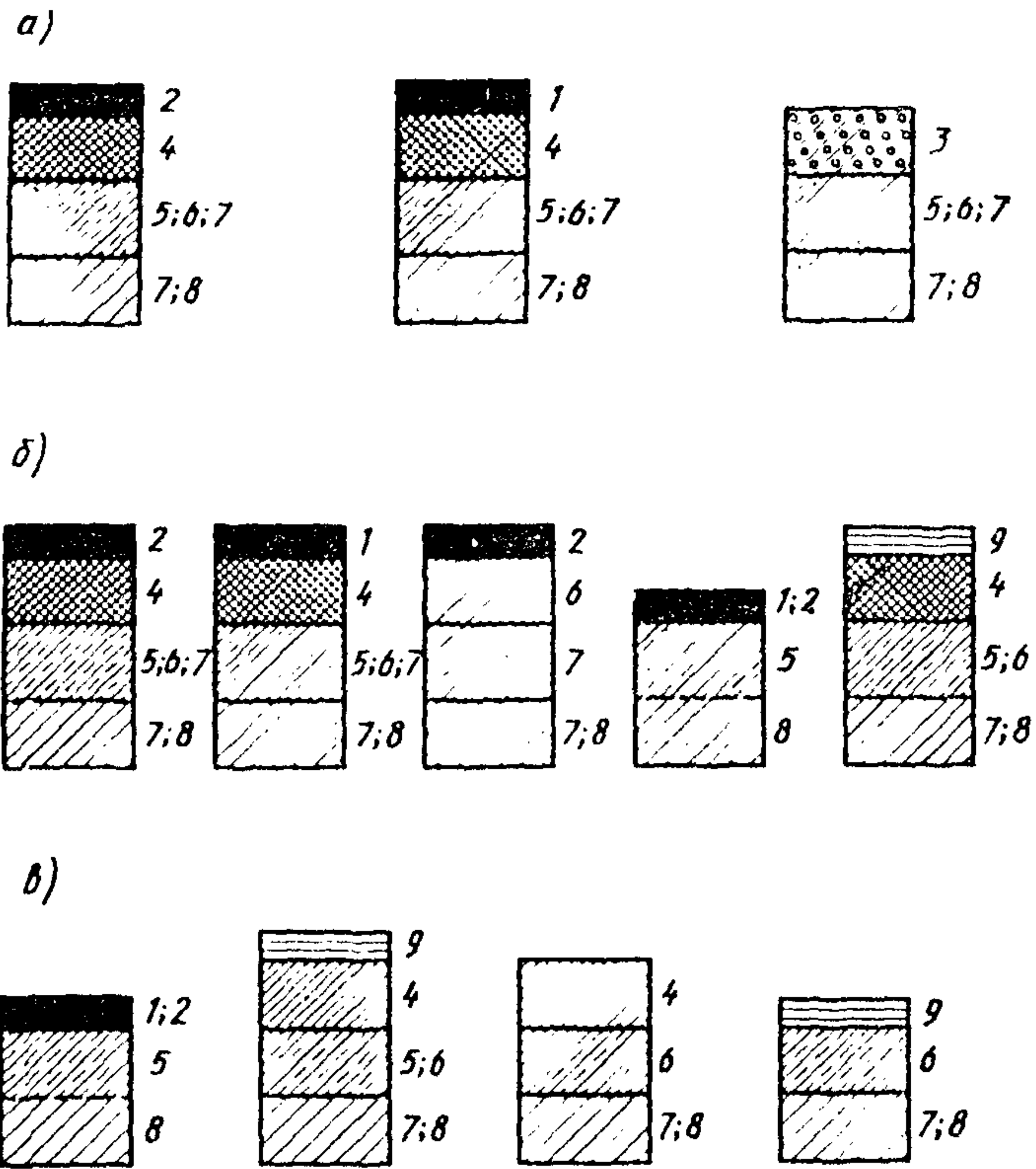
Рис. 12. Рекомендуемые конструкции дорожных одежд со слоями из укрепленных грунтов для дорог I и II (а); III (б); IV и V (в) категорий: 1 и 2 - одно- и двухслойное асфальтобетонное покрытие; 3 - цементобетонное покрытие; 4 - черный щебень; 5 - основание из цементогрунта I класса прочности; 6 - основание из грунта, укрепленного карбамидоформальдегидной смолой или комплексными методами, I класса прочности и повышенной деформативности; 7 - основание из грунтов, укрепленных цементом, карбамидоформальдегидной смолой и комплексными методами, II класса прочности; 8 - морозозащитный слой из укрепленного грунта II-III классов прочности; 9 - двойная поверхностная обработка
