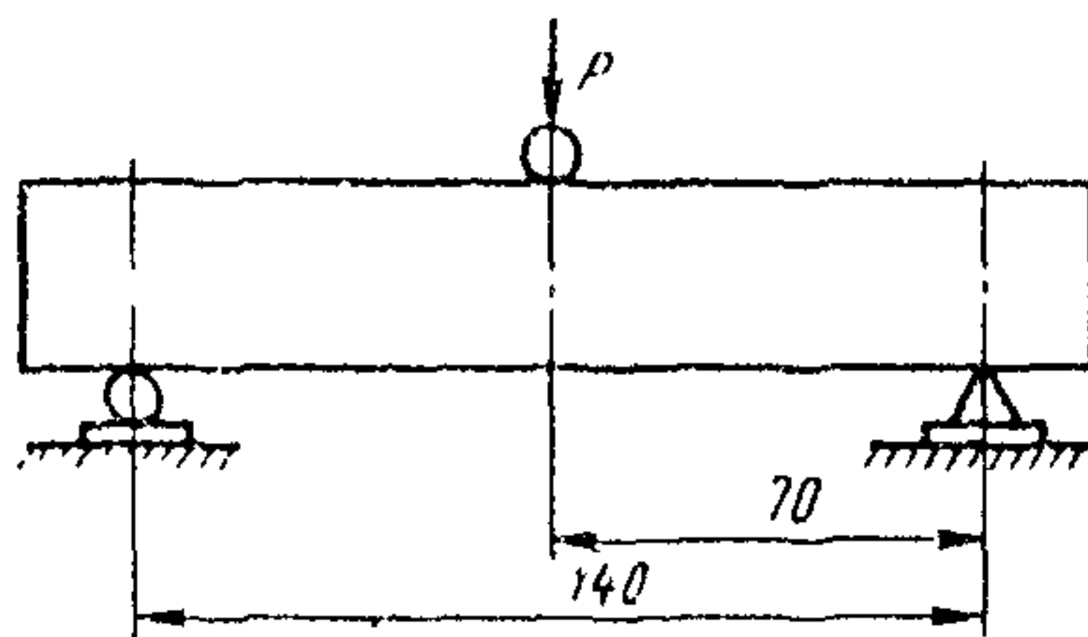
Рис.10. Схема испытания образцов-балочек на изгиб
