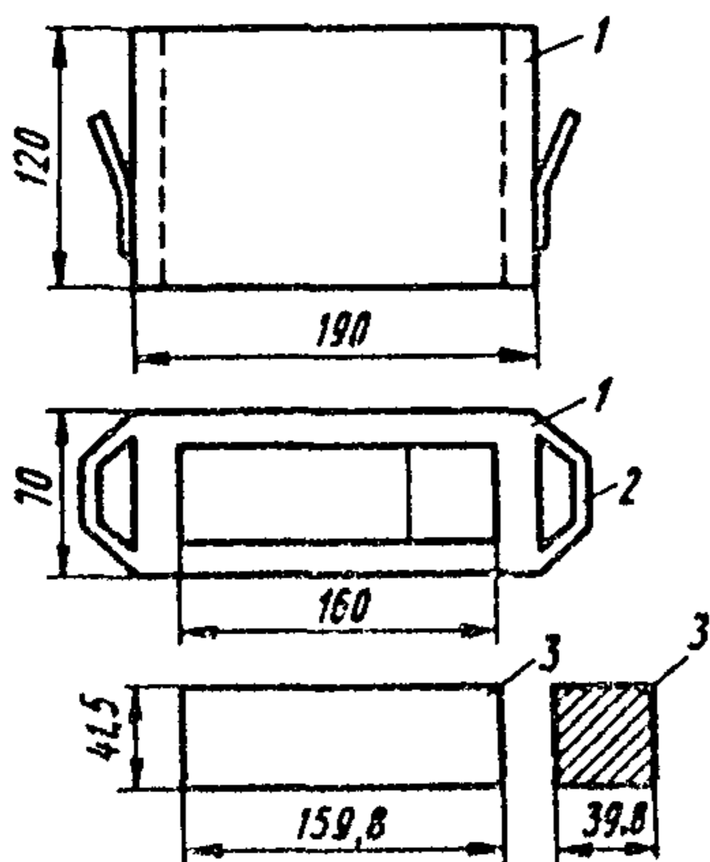
Рис. 5. Форма для изготовления образцов-балочек: 1 - корпус; 2 - ручка; 3 - вкладыш
