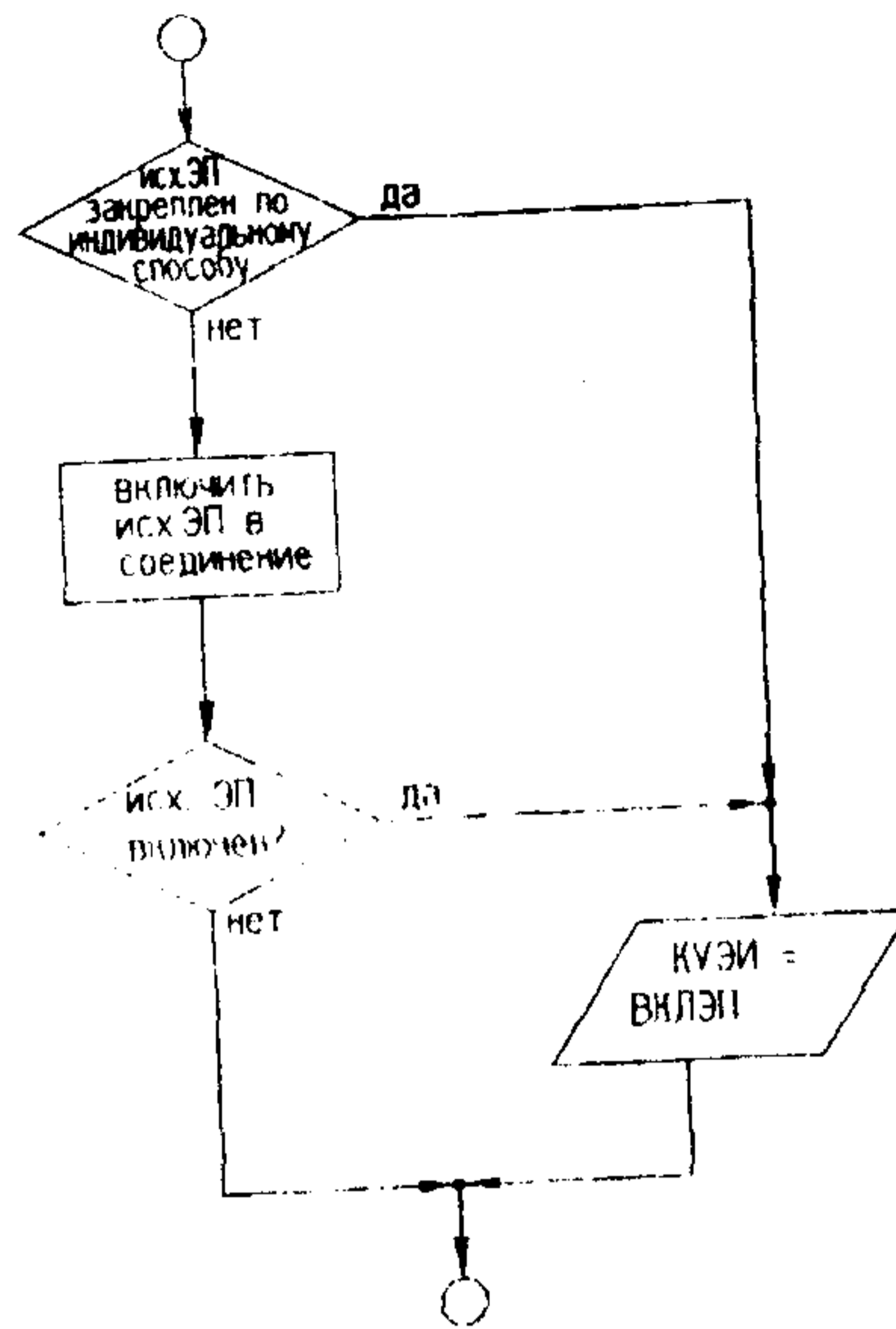
Рис.18. Блок схема алгоритма процедуры "Включить исходящее ЭП".
