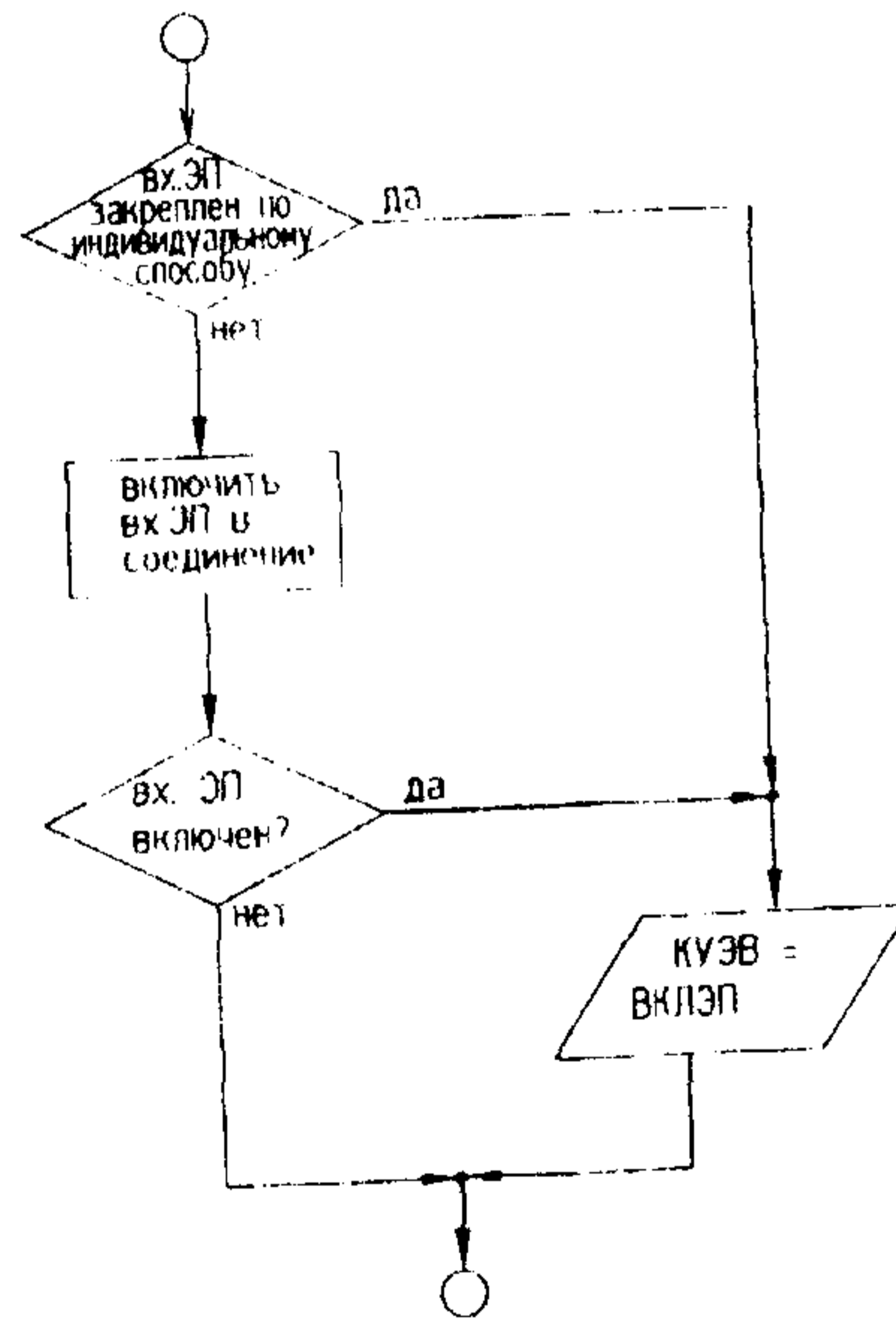
Рис.19. Блок схема алгоритма процедуры "Включить входящее ЭП".
