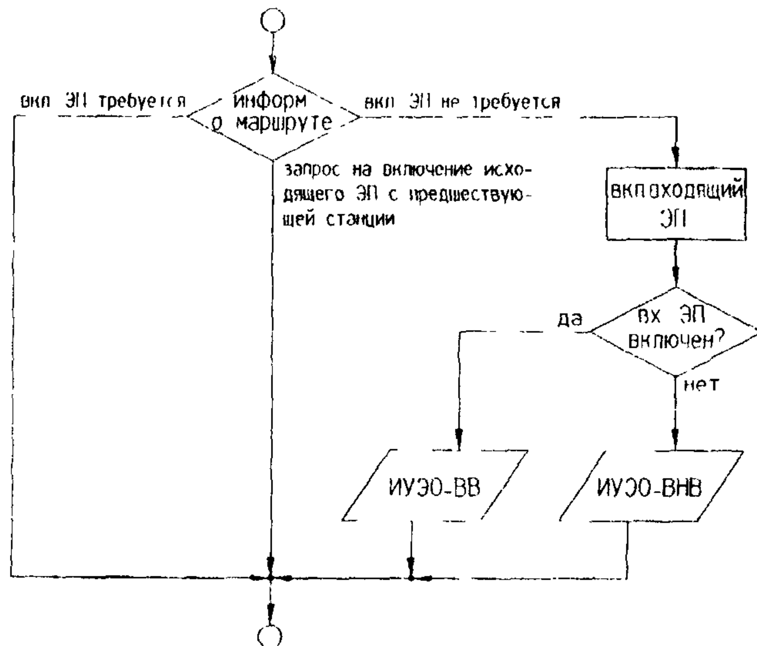
Рис.10 Блок схема алгоритма процедуры ПИЭПВК
