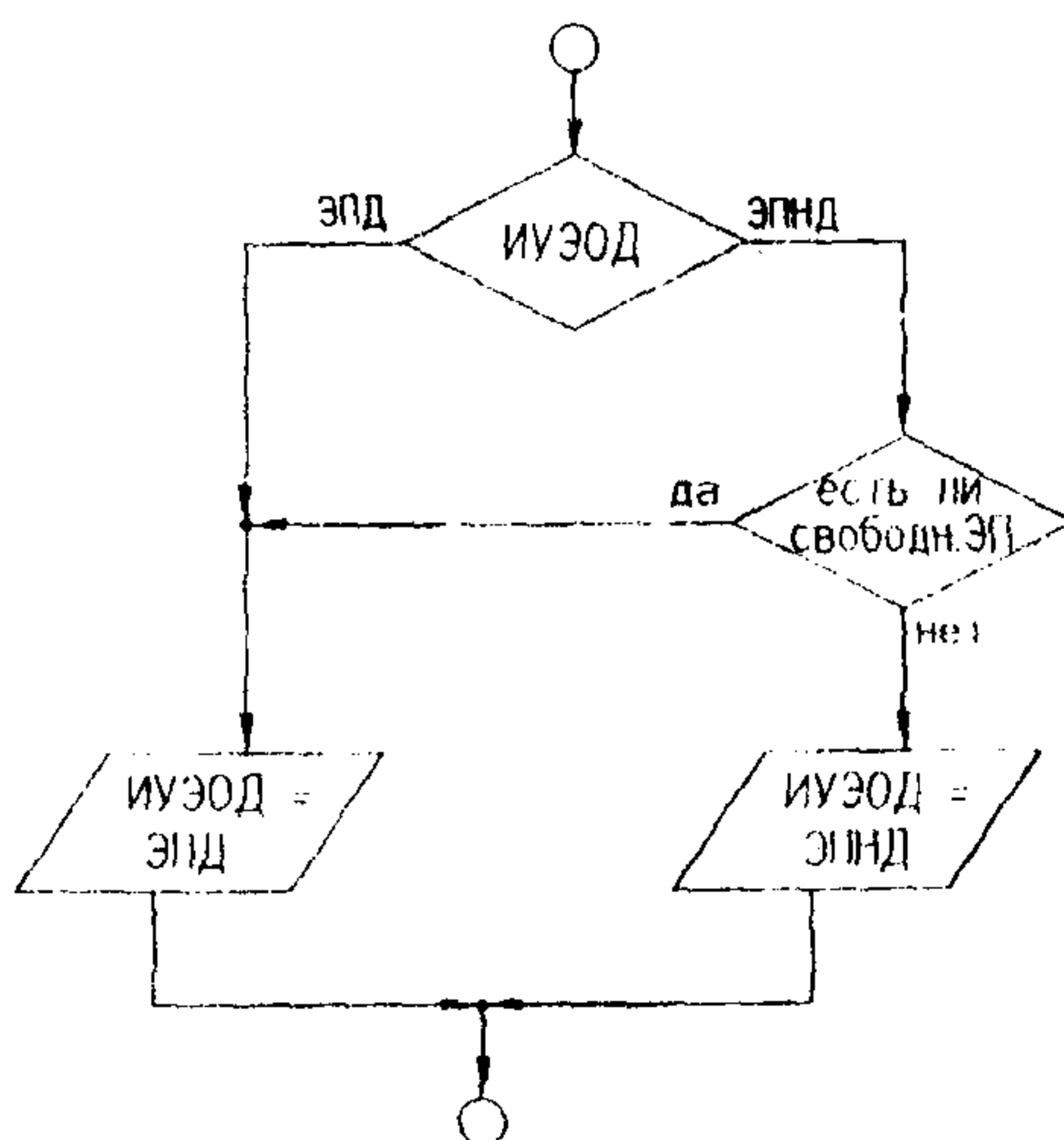
Рис.15. Блок схема алгоритма процедуры ПИУЭОД.
