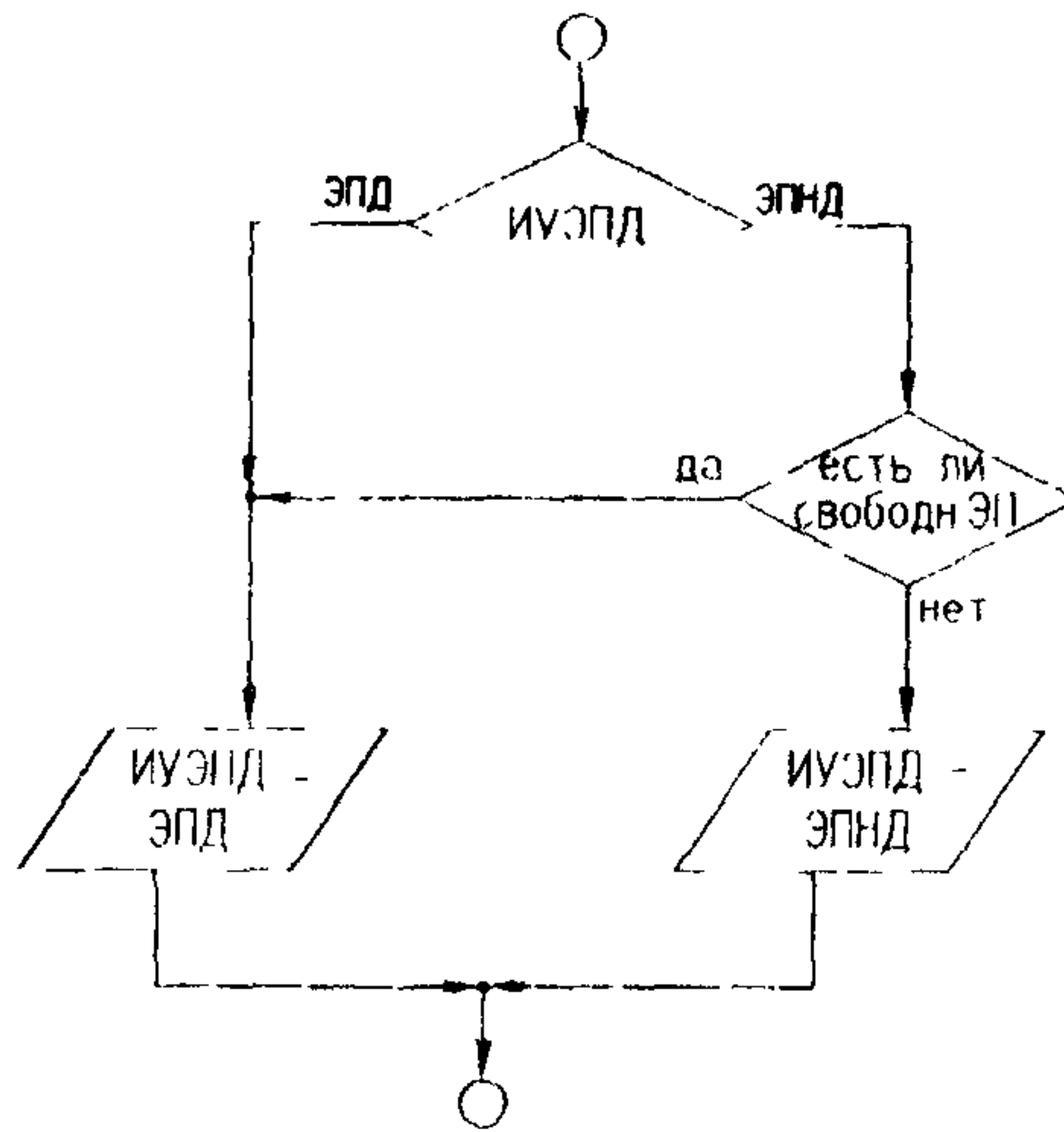
Рис.9 Блок схема алгоритма процедуры ПИУЭПД.
