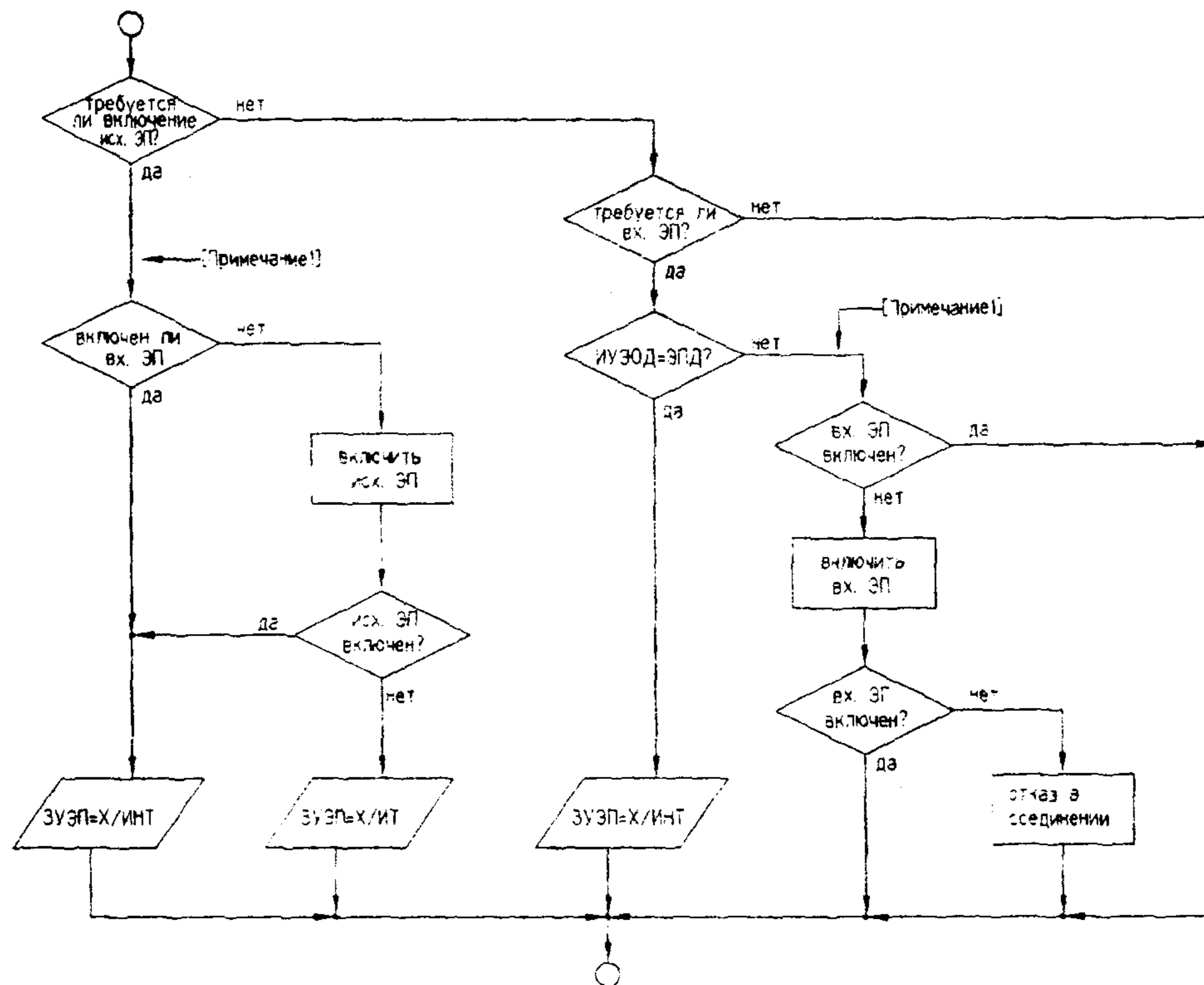
Рис.13. Блок-схема алгоритма процедуры пЗУЭП.
