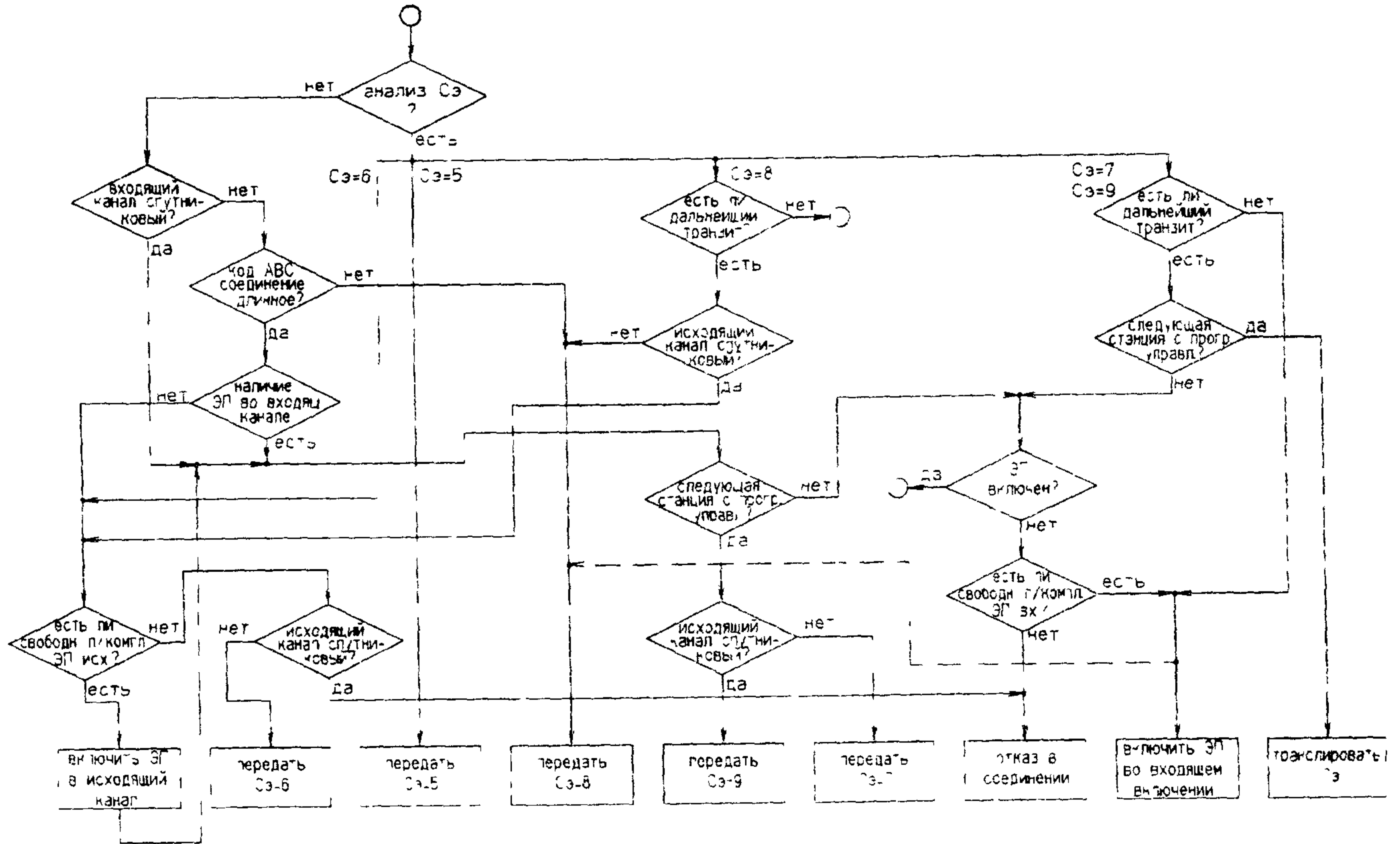
Рис 5 Алгоритм управления ЭП и формирования сигналов Sz на коммутационных станциях электронного и электровакуумного типа
