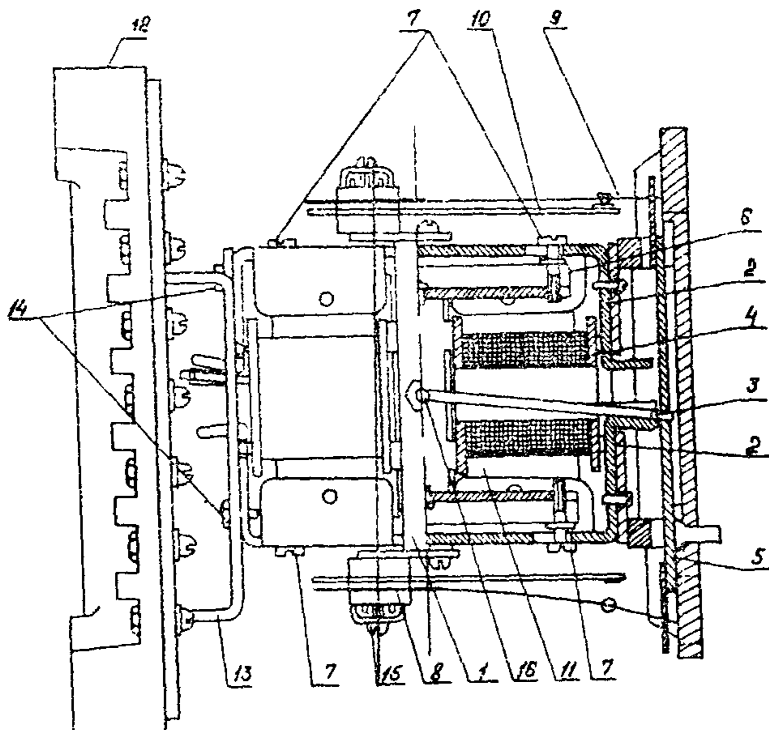
Рис.10. Общий вид реле РП-11, РП-12:
