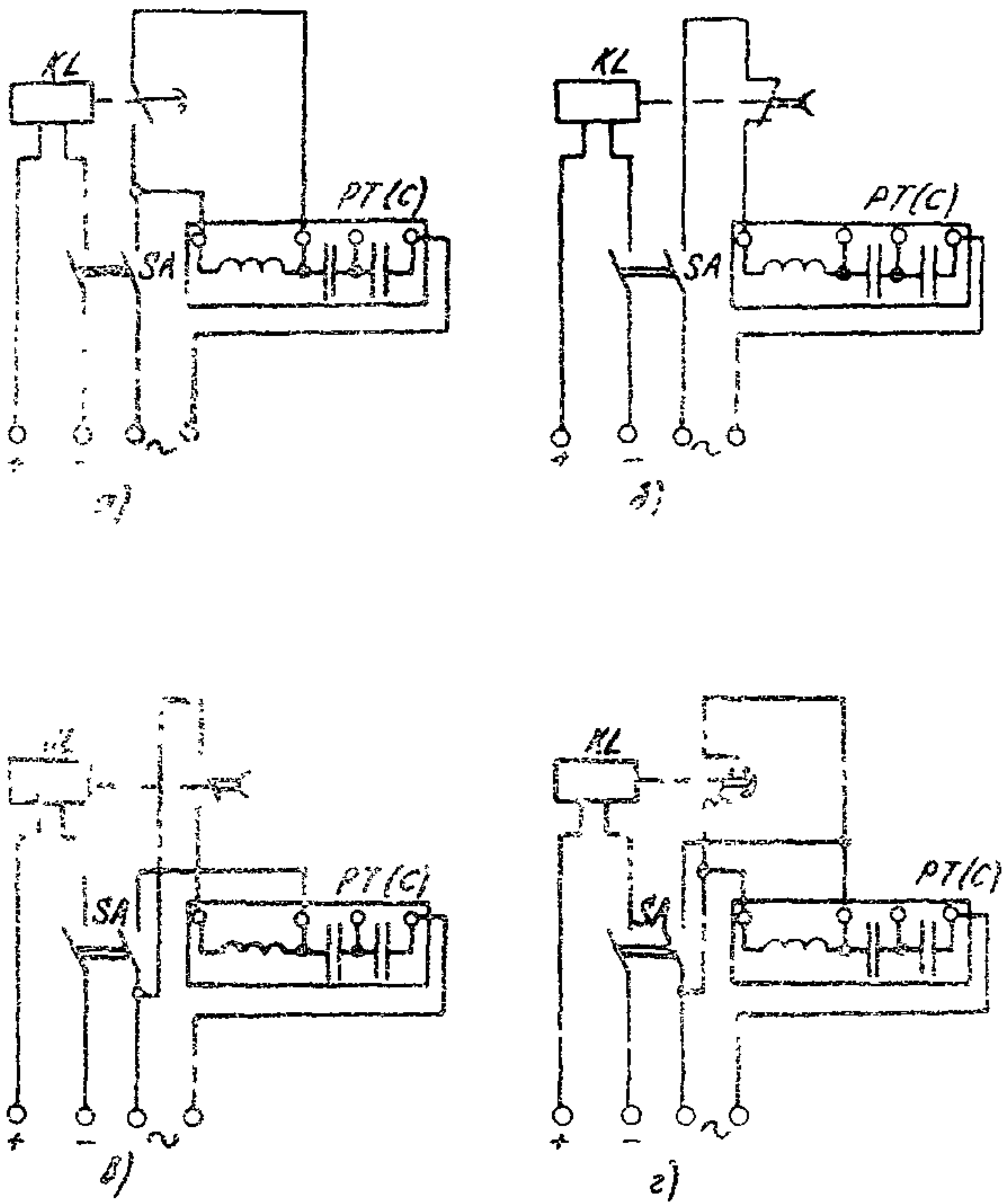
Рис. 19. Схемы измерения:
