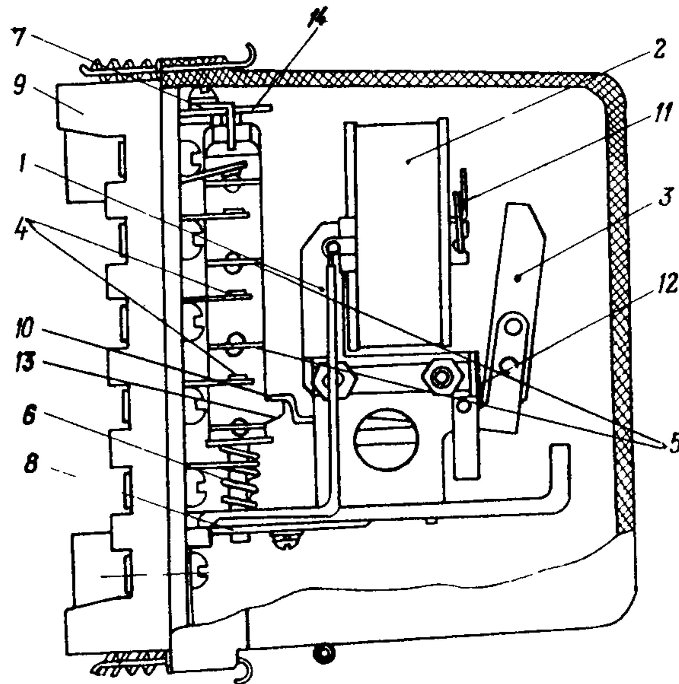
Рис. 3. Общий вид реле РП-25:
