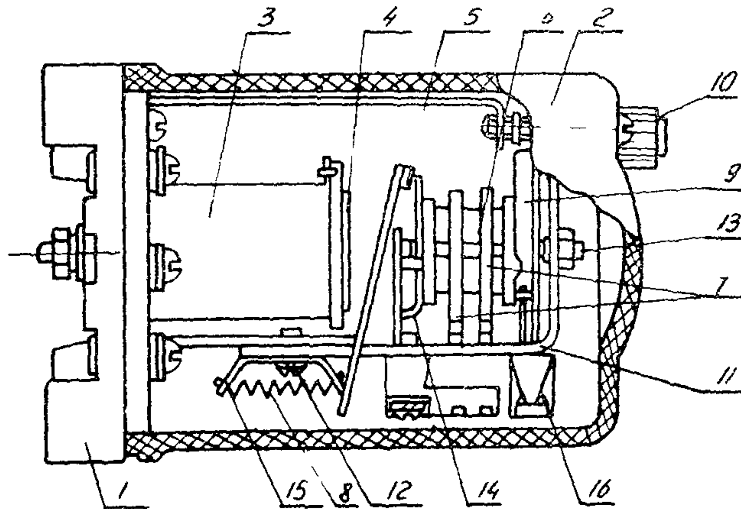
Рис. 12. Общий вид реле РУ-21:
