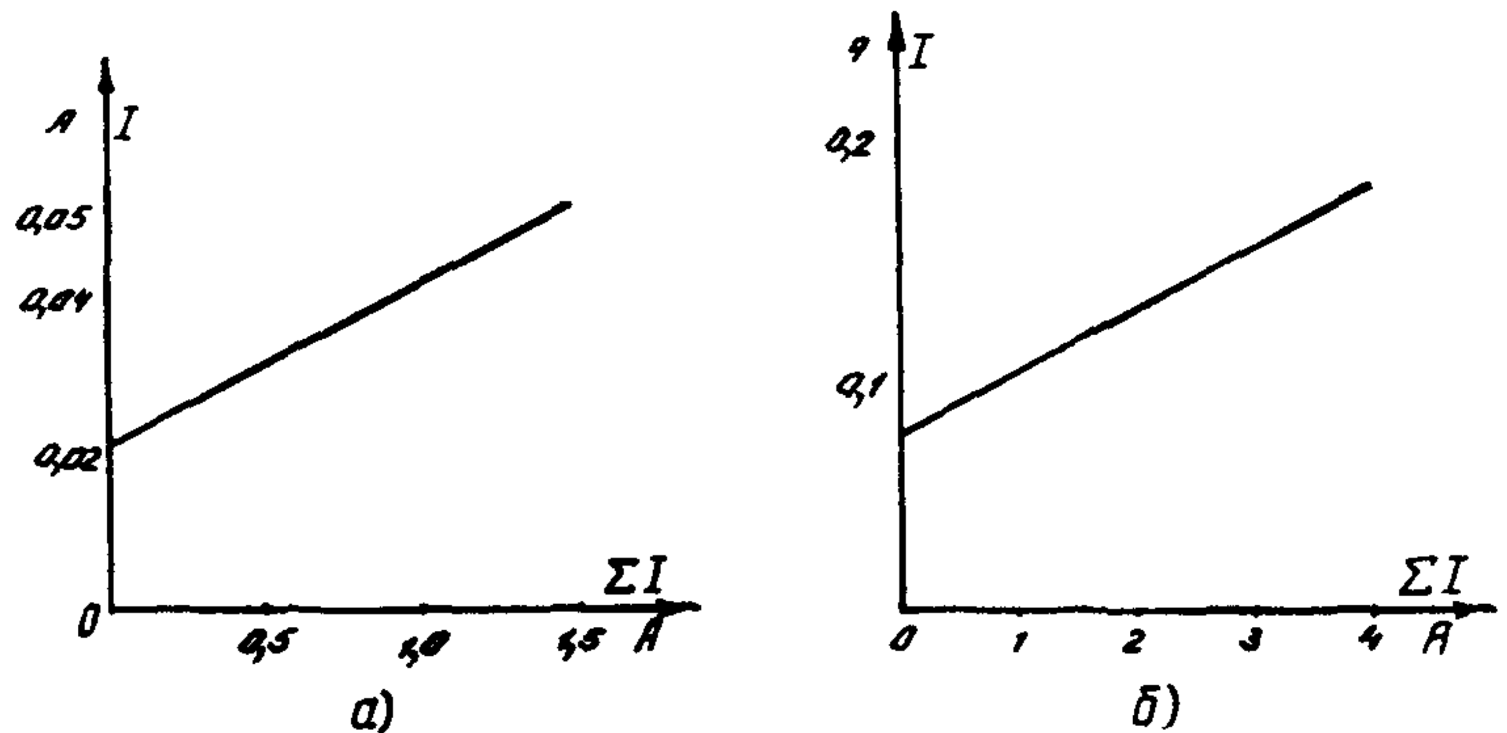
Рис.22. Зависимость значений импульса тока срабатывания: а - для реле РИС-ЭЗМ; б - для реле РИС-ЭЗМ-0,2
