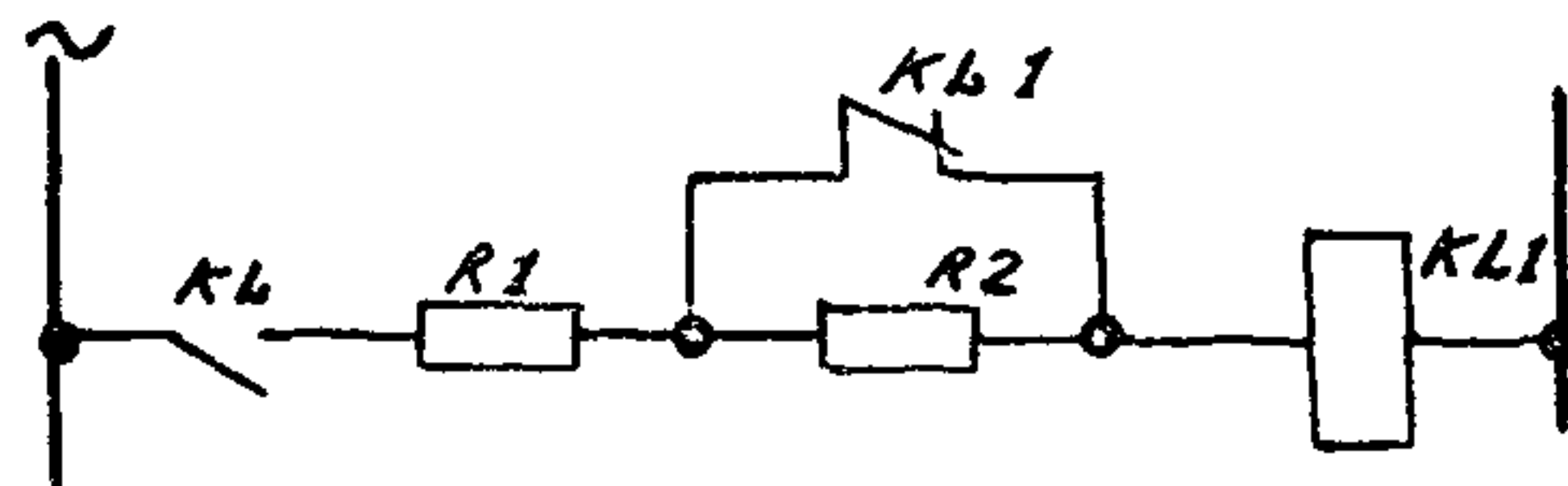
Рис. П.3. Схема включения промежуточного реле переменного тока с добавочными резисторами
