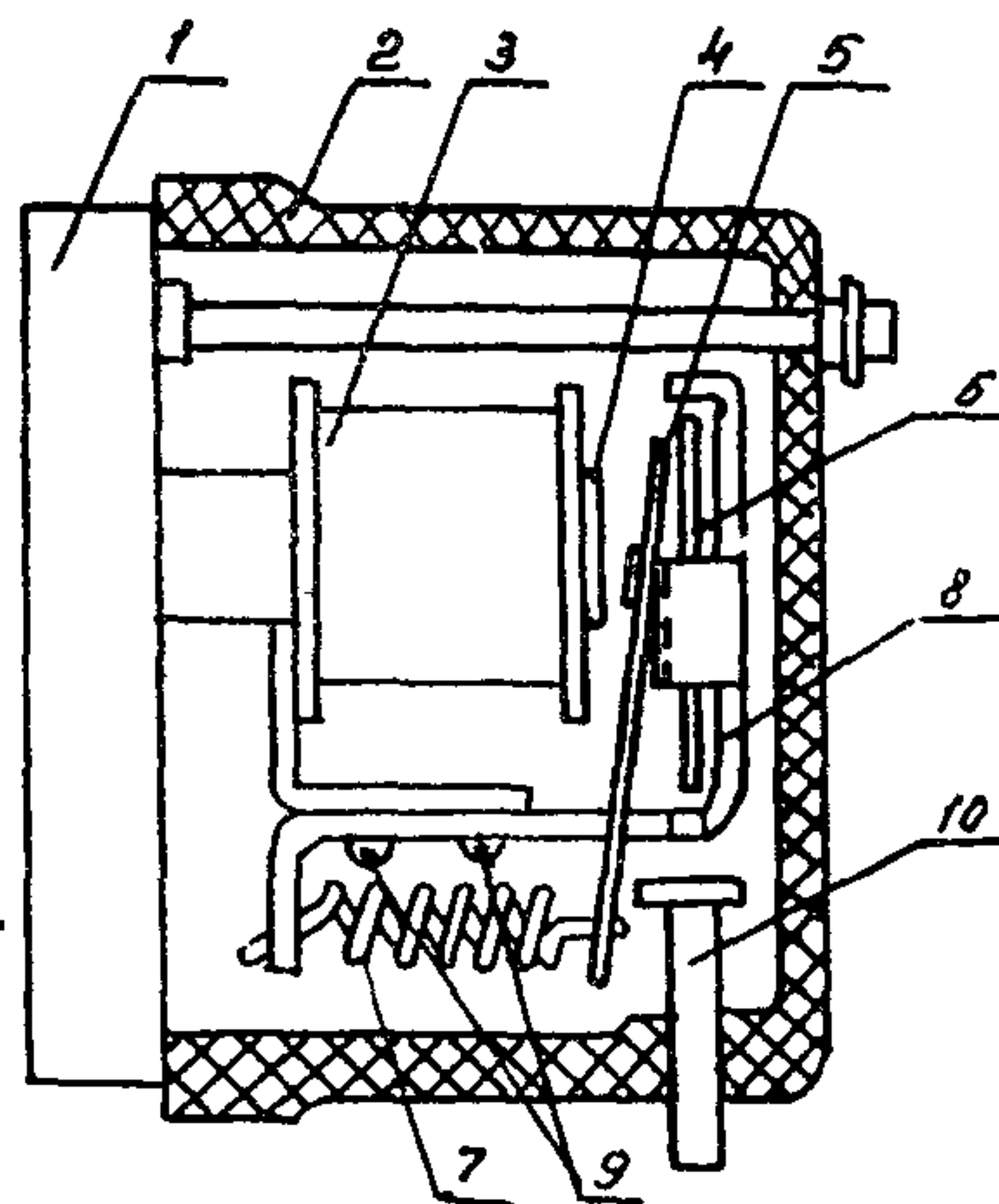
Рис. 13. Общий вид реле ЭС-41:
