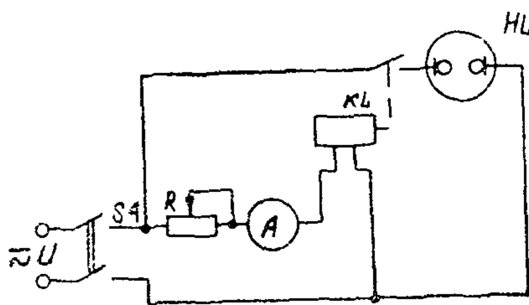
Рис. 17. Схема проверки тока срабатывания и возврата реле
