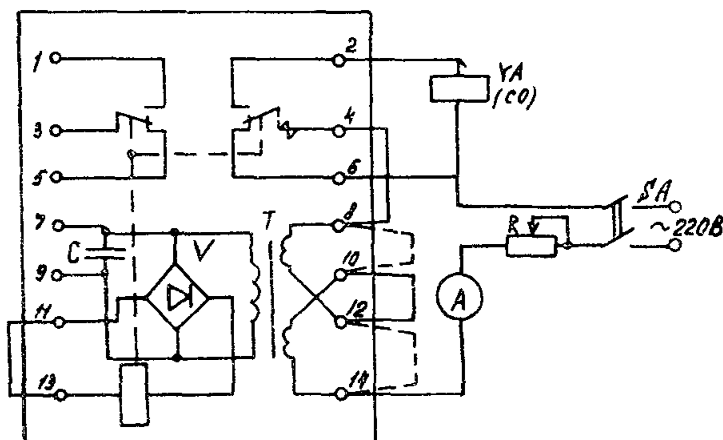
Рис.21. Схема проверки надежности работы контактной системы реле РП-341
