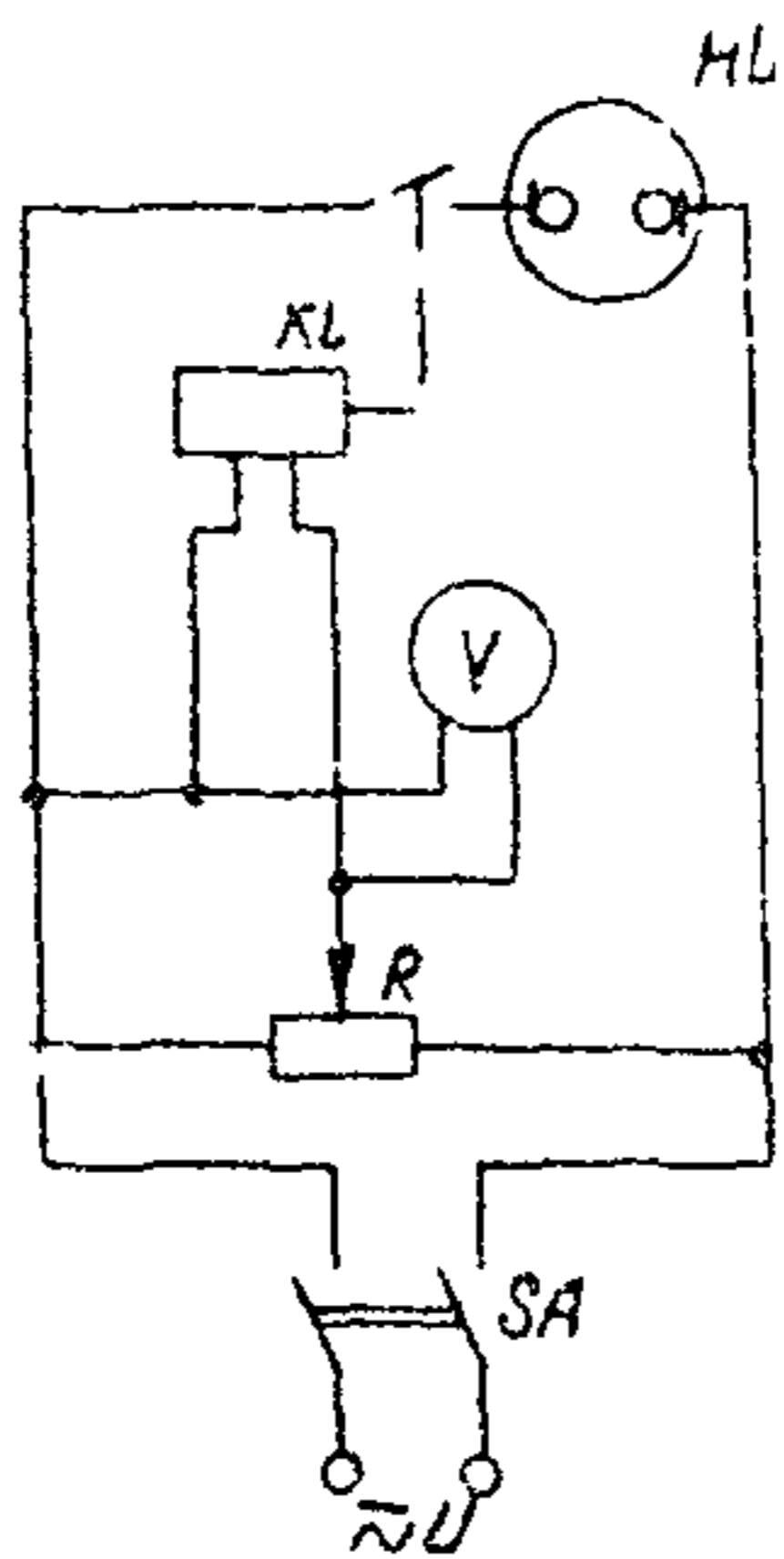
Рис. 16. Схема проверки напряжения срабатывания и возврата реле
