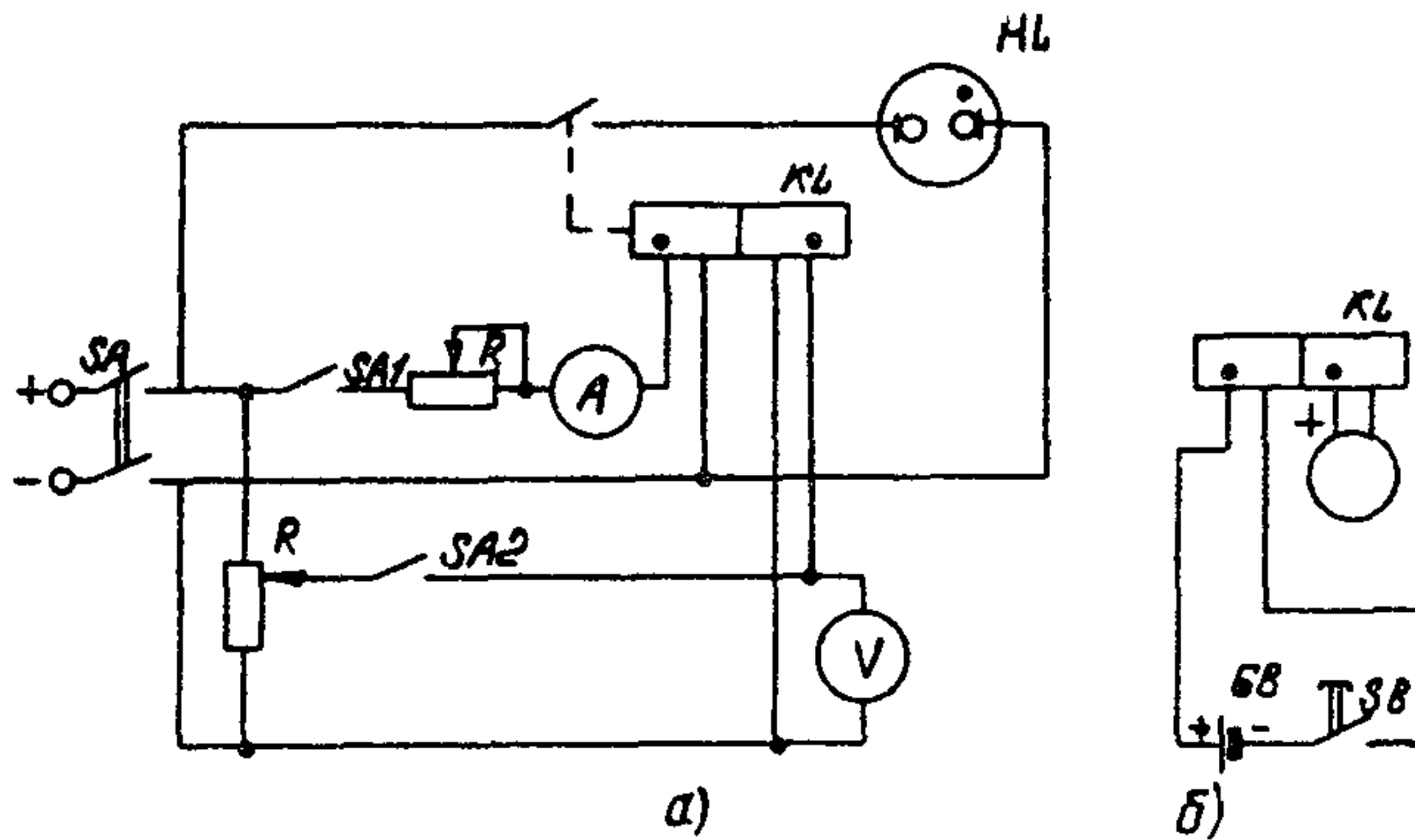
Рис. 18. Схемы проверки однополярных выводов реле: а - I-й вариант; б - 2-й вариант
