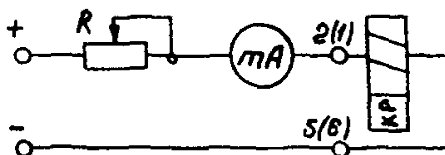
Рис. 25. Схема проверки поляризованного реле ТРМ-Т
