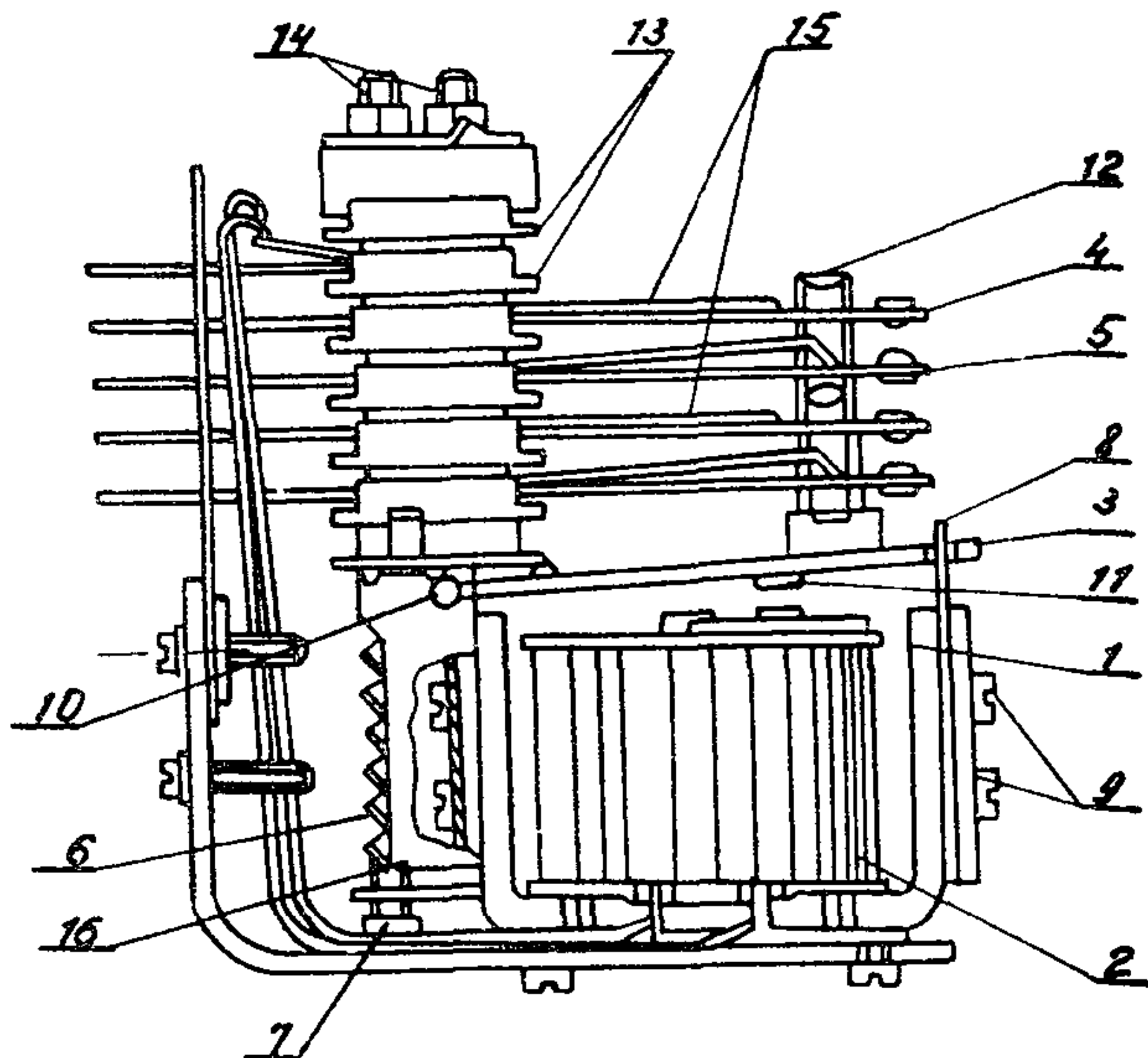
Рис. 7. Общий вид реле МКУ-48:
