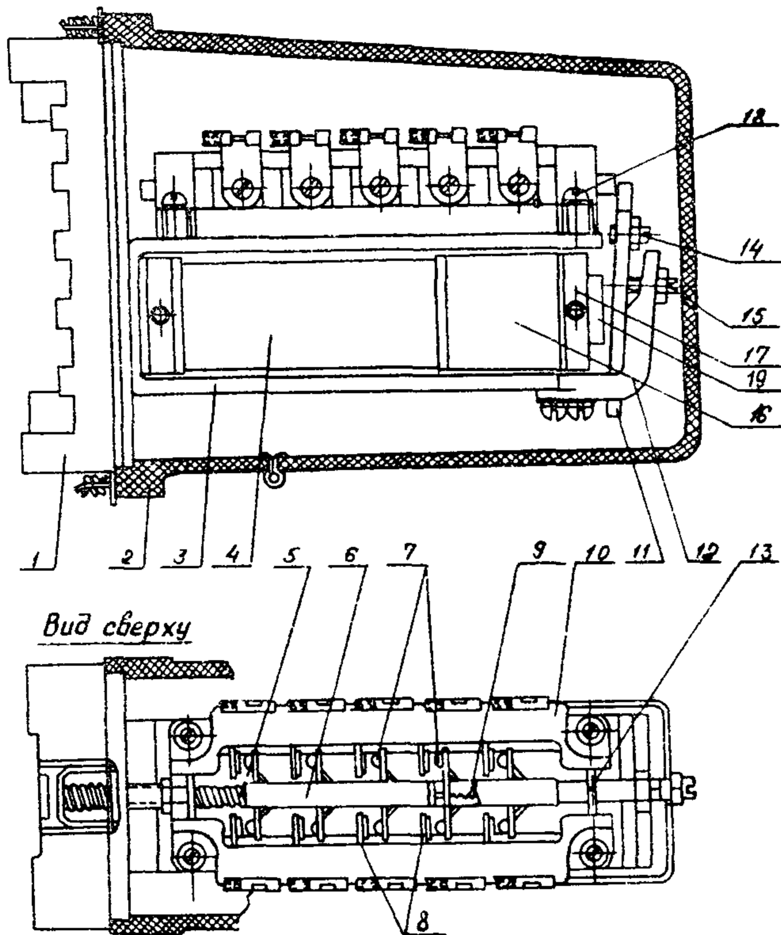
Рис. 4. Общий вид реле РП-25I:
