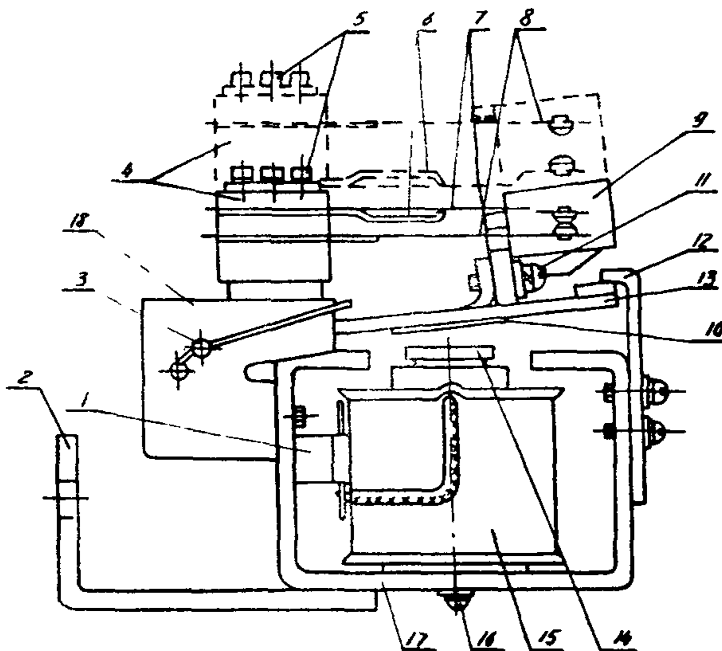
Рис. 6. Общий вид реле РПУ-1-010:
