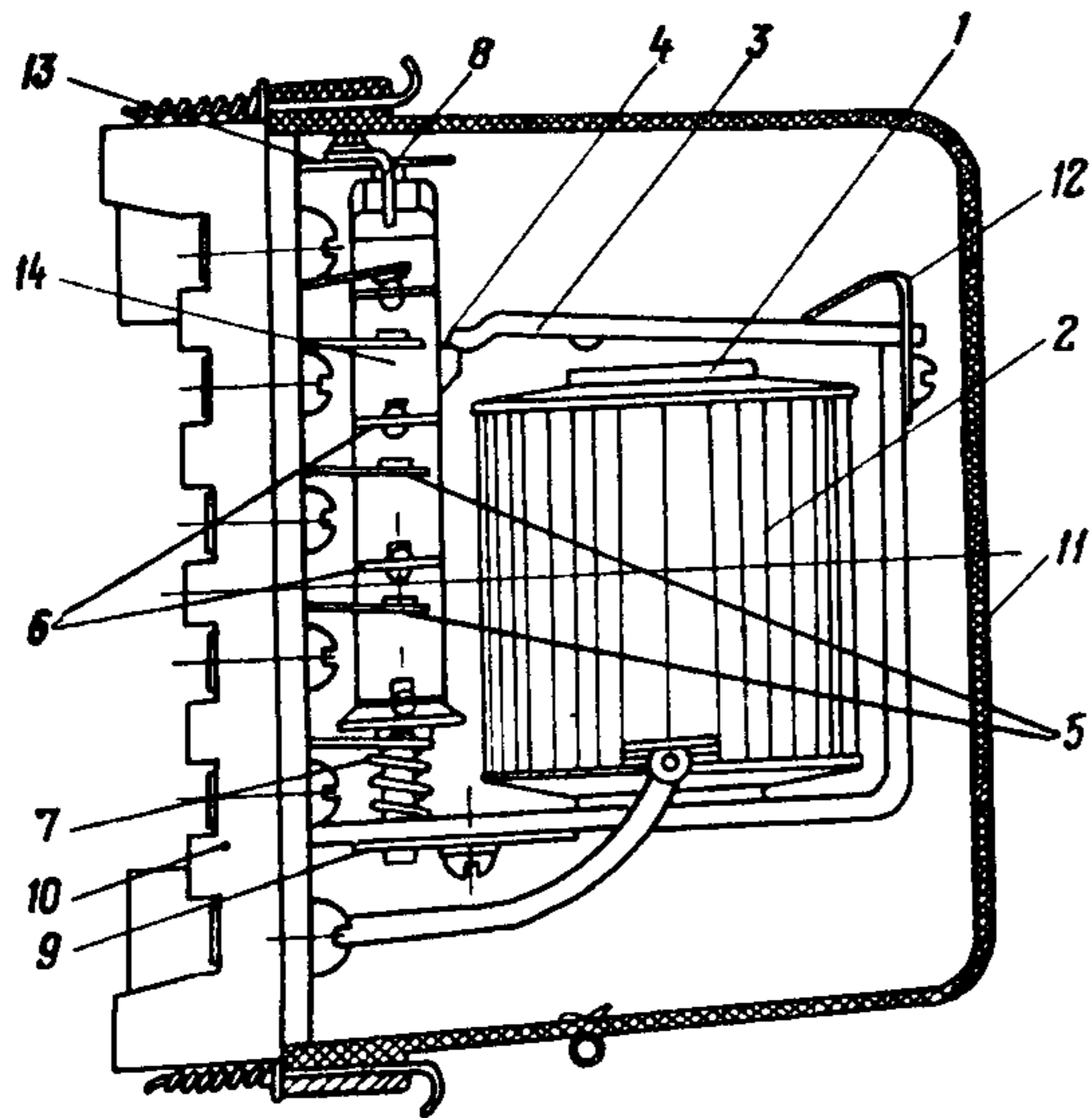
Рис. 2. Общий вид реле РП-23, РП-232, РП-233:
