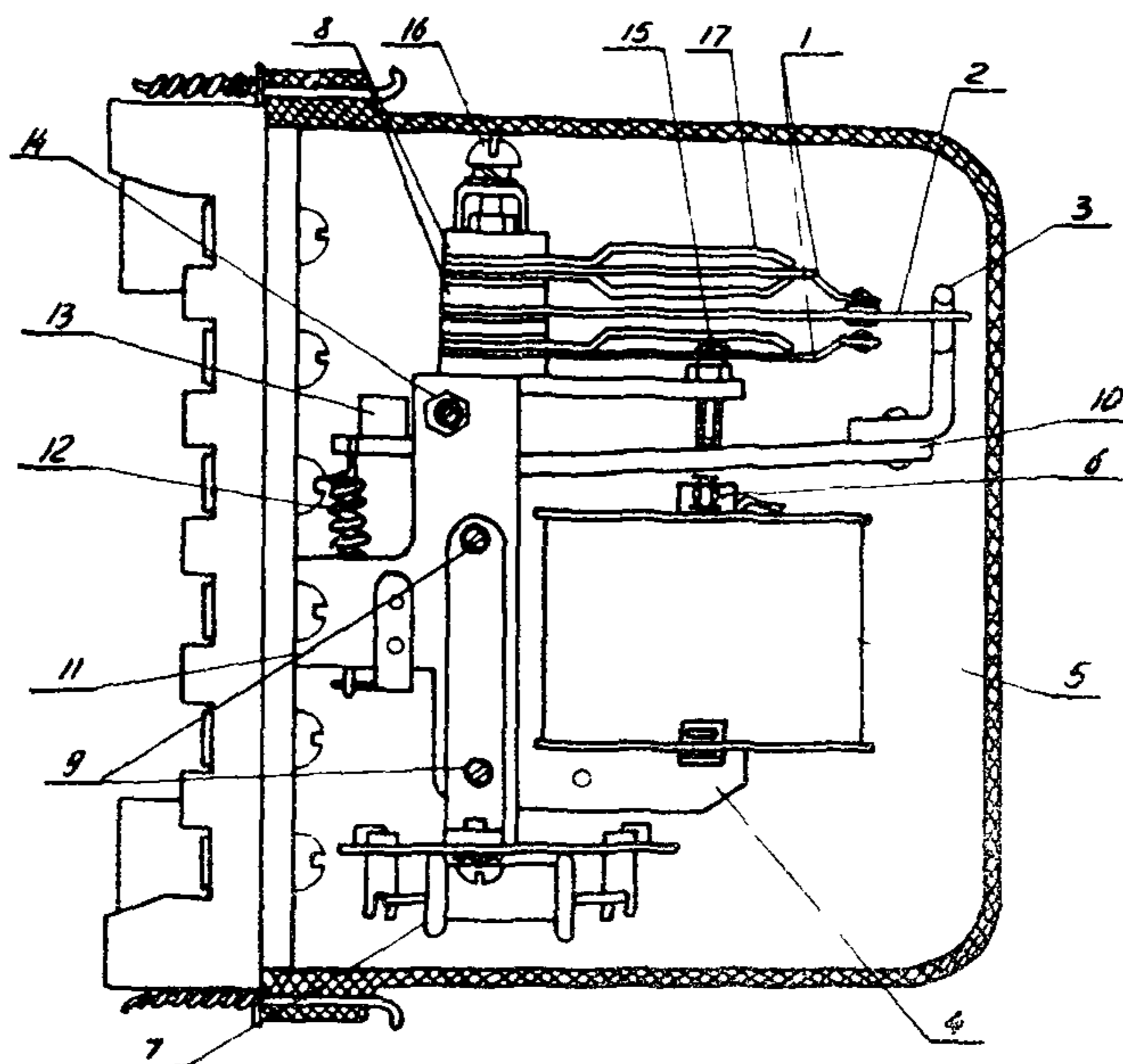
Рис. 5. Общий вид реле РП-220:
