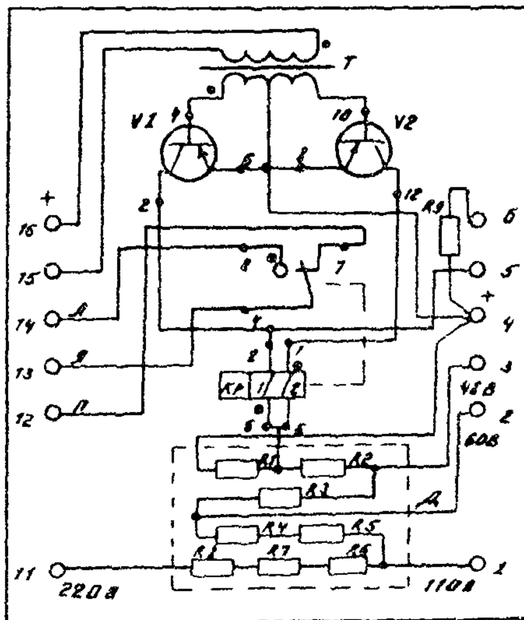
Рис. 14. Принципиальная схема реле РИС-32М
