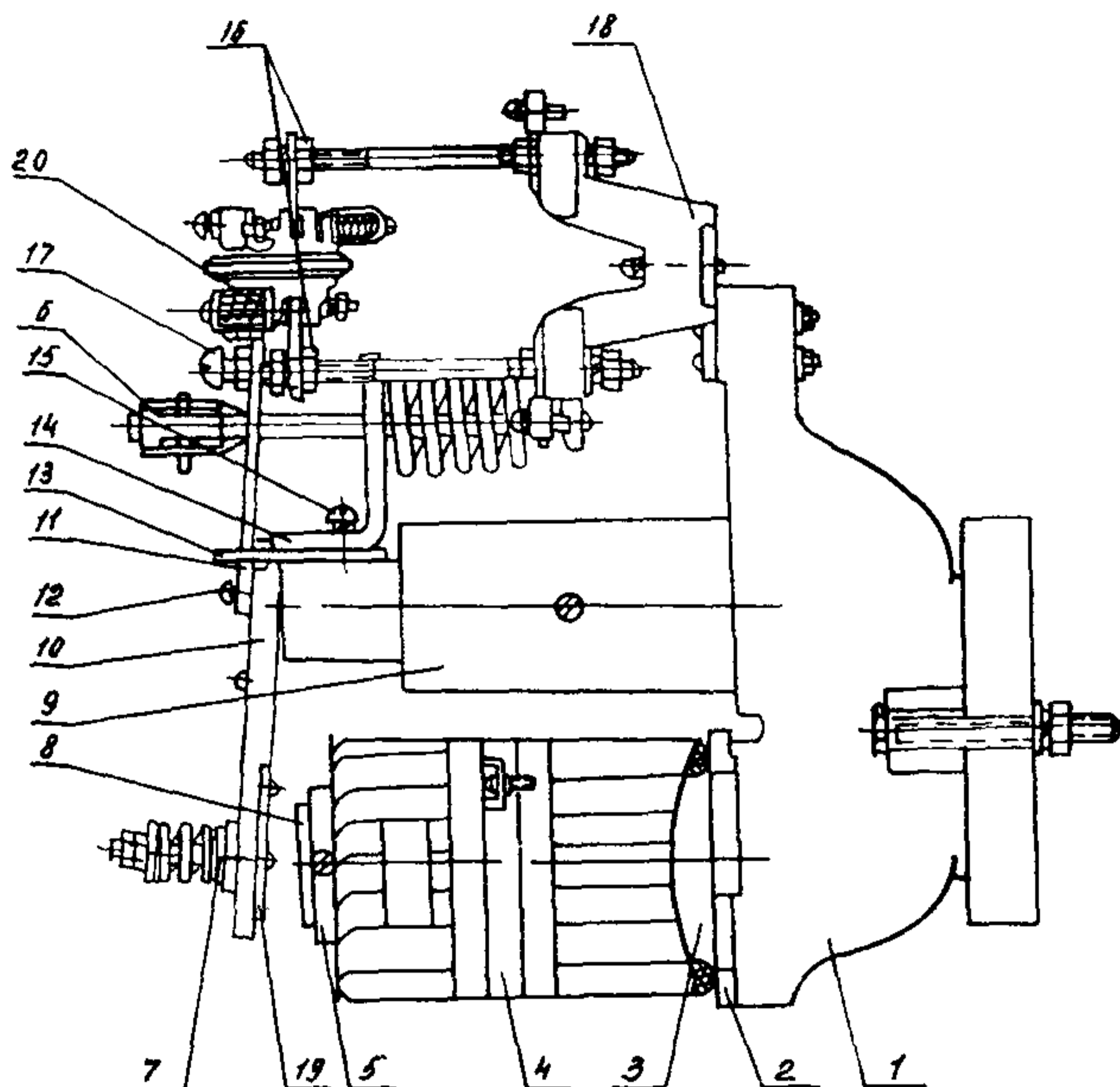
Рис. II. Общий вид реле РЭВ-883, РЭВ-884:
