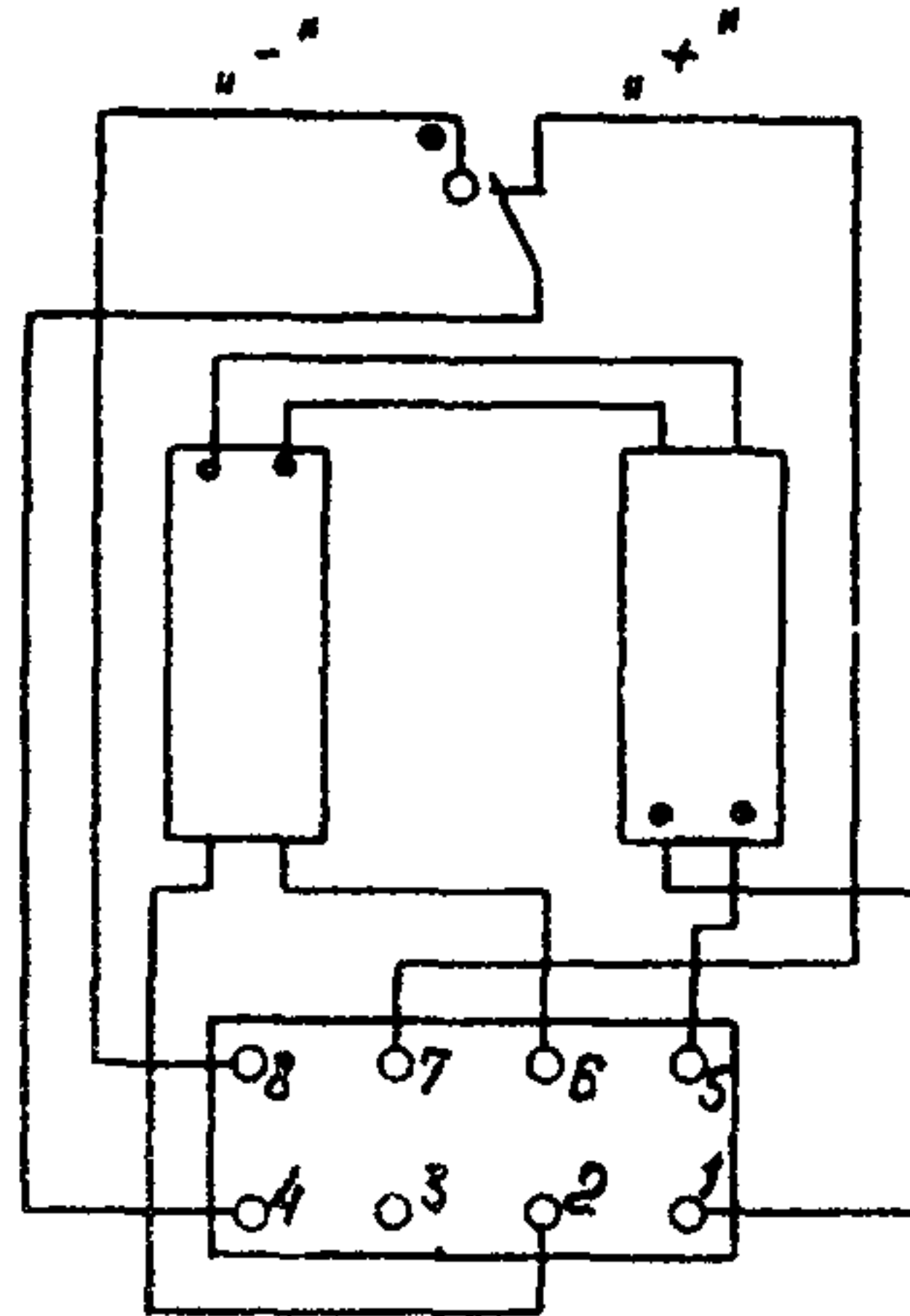
Рис. 26. Схема внутренних соединений поляризованного реле ТРМ-Т
