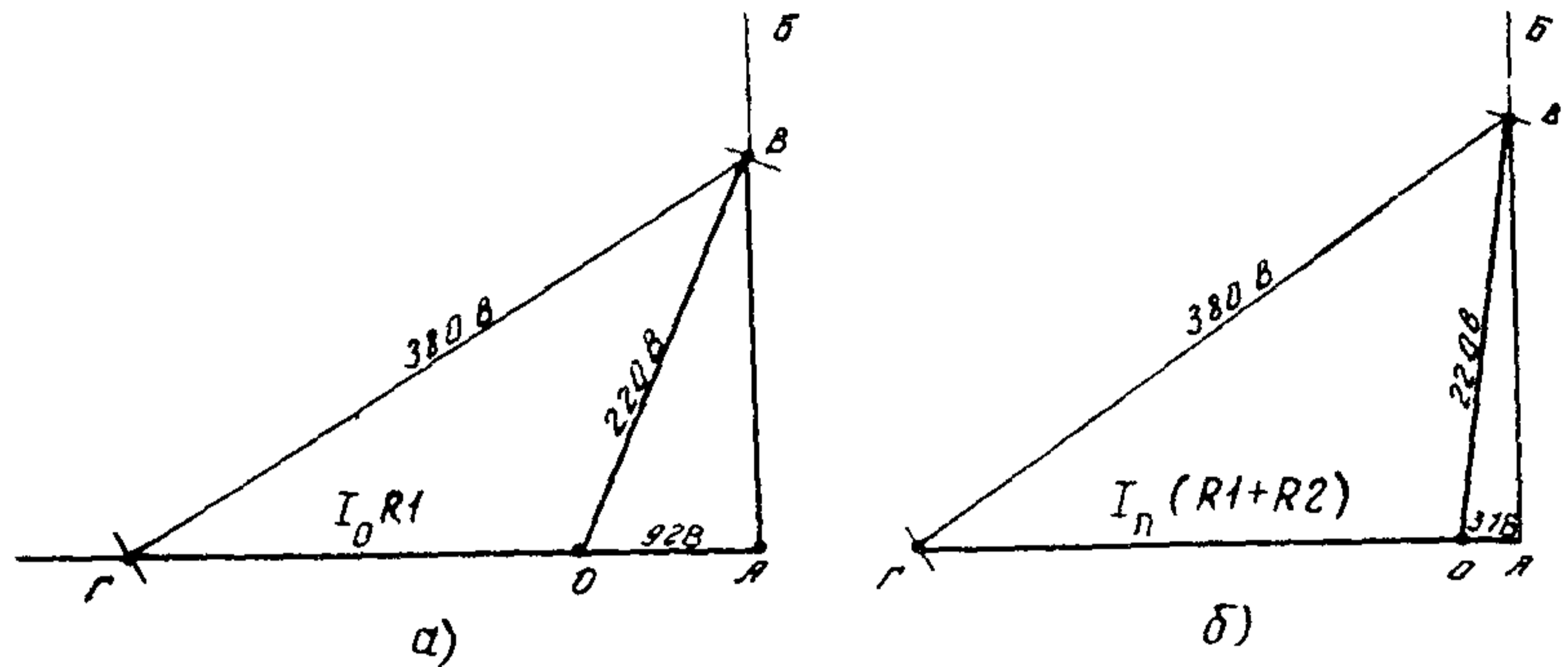
Рис. ПІ.4. Графическое определение сопротивления:
