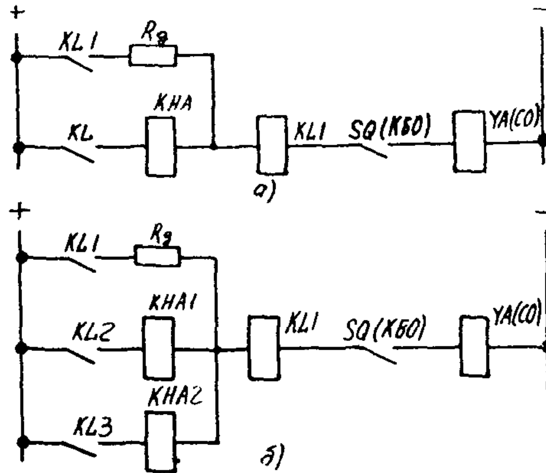
Рис. П.2. Схема выходных цепей защиты: а - при включении одного указательного реле; б - при включении двух указательных реле
