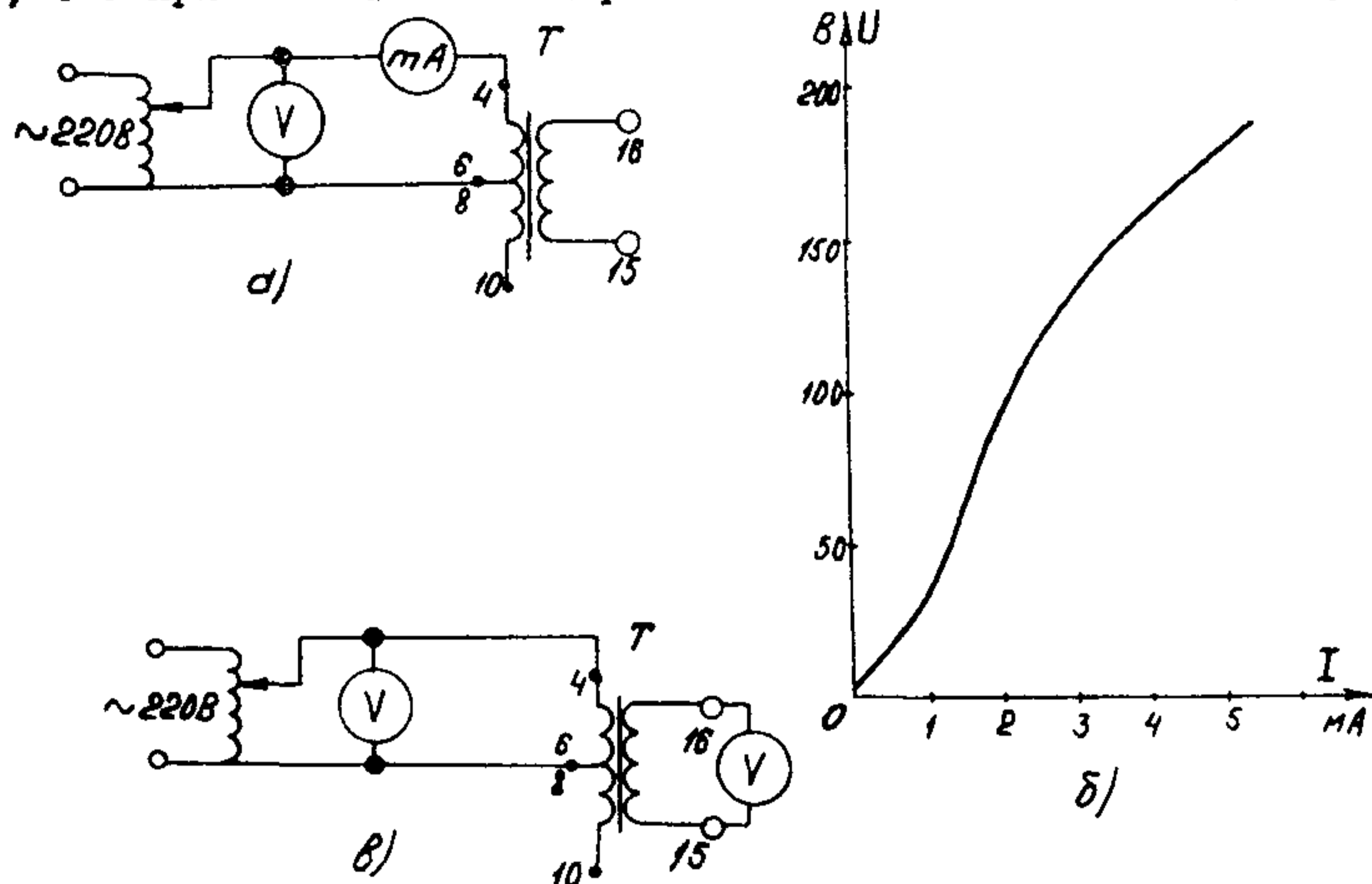
Рис. 27. Схемы проверки трансформатора реле РИС-Э2М, РИС-Э2М-0,2:
