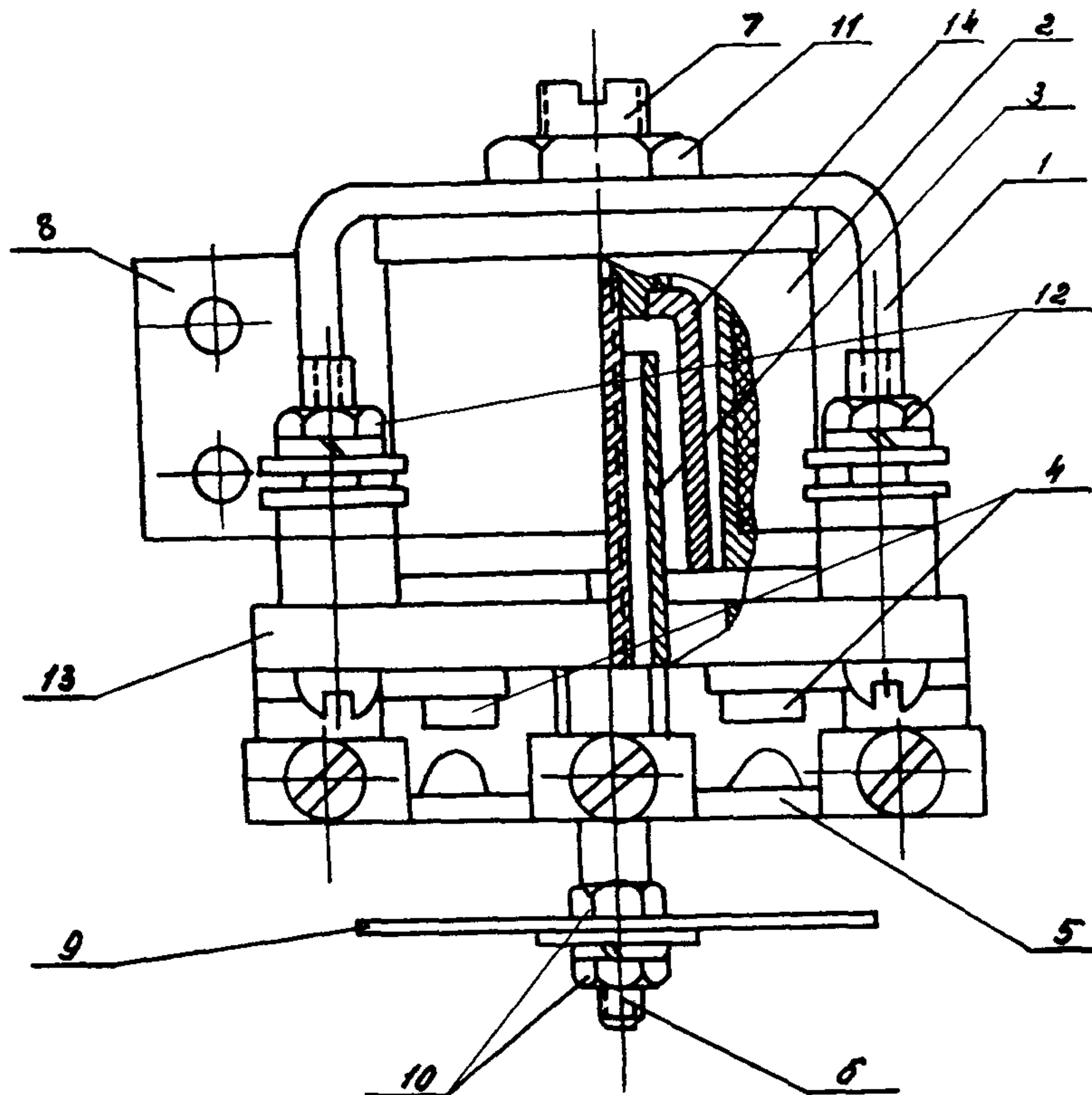
Рис. 1. Общий вид реле ЭП-1:
