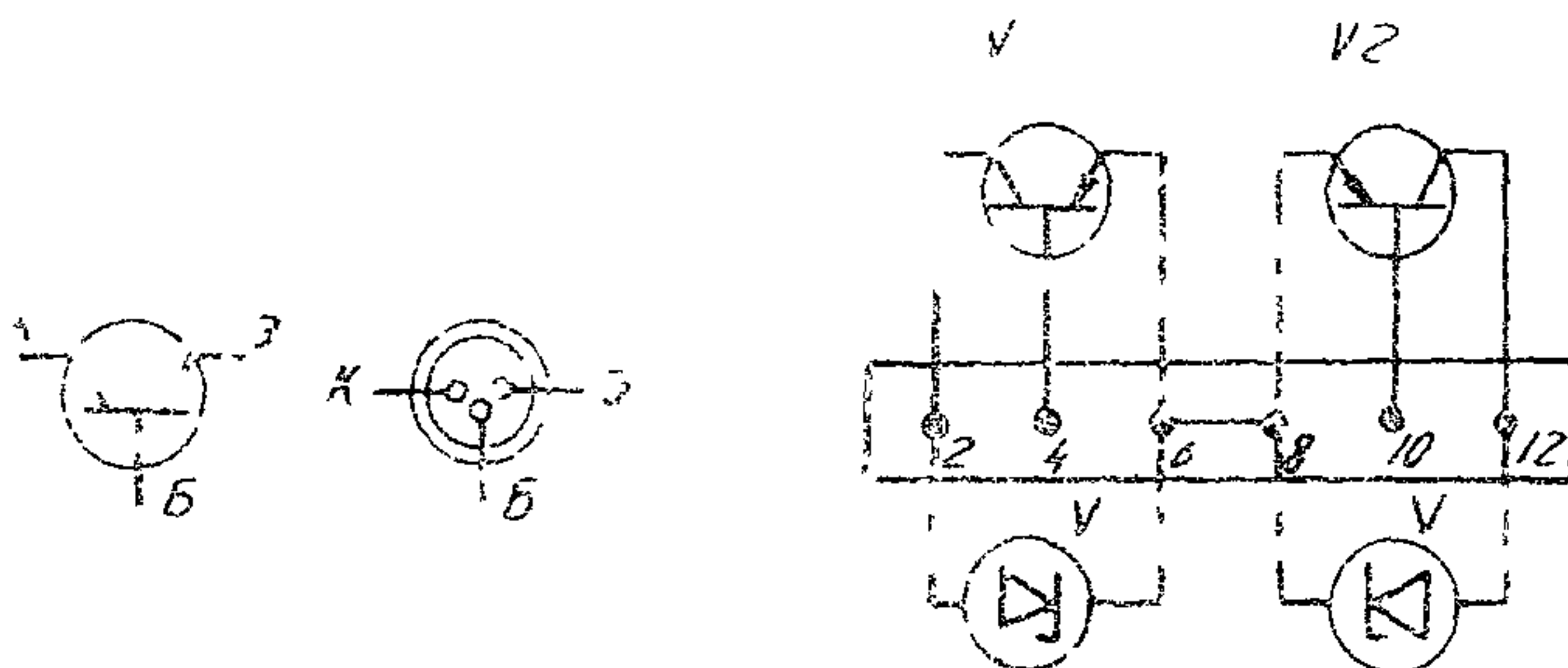
Рис. 28. Цоколевка и монтажная планка крепления транзисторов V1, V2 реле РИС-Э2М, РИС-Э2М-0,2
