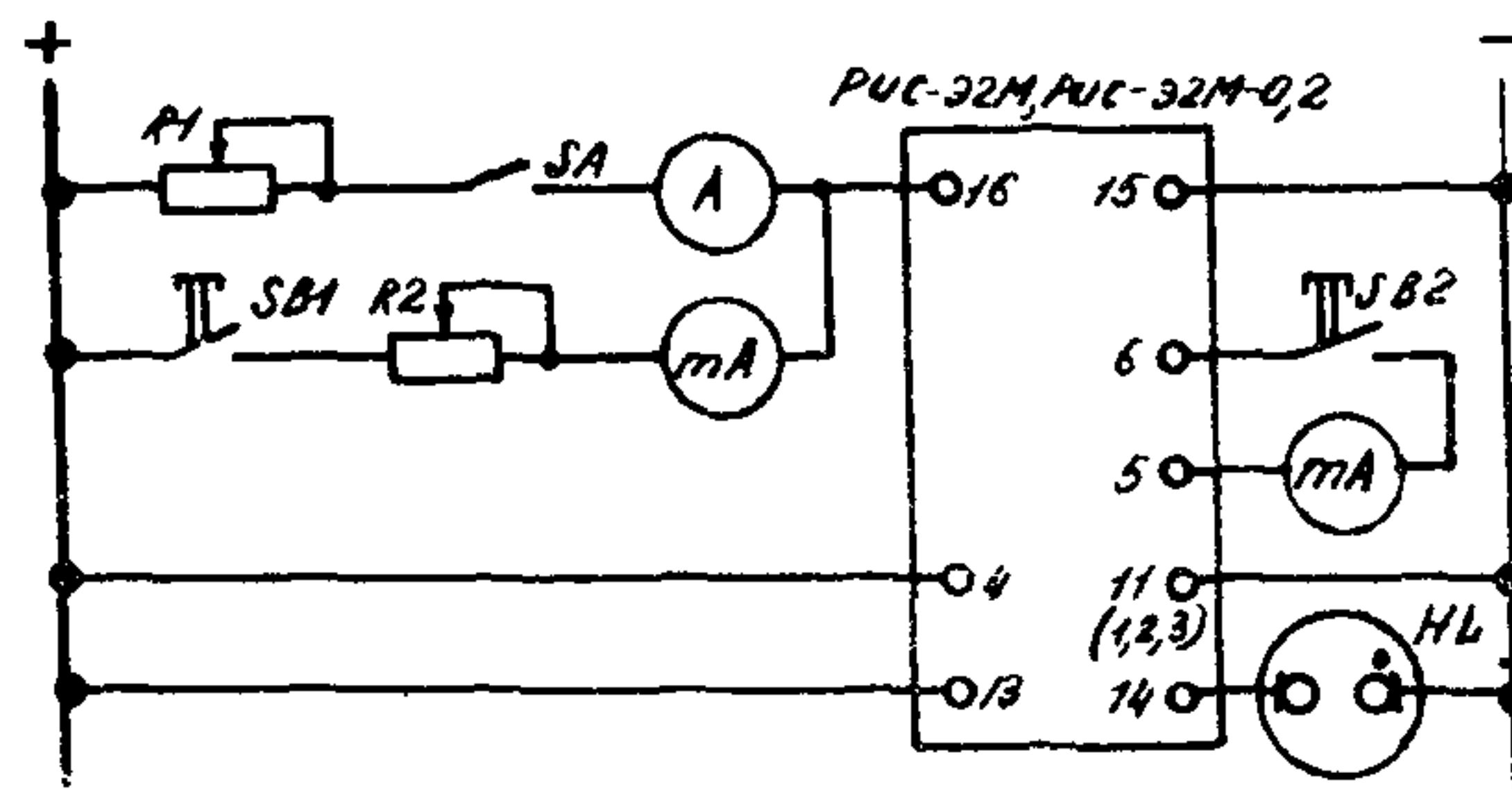
Рис. 23. Схема настройки реле РИС-ЭЗМ, РИС-ЭЗМ-0,2
