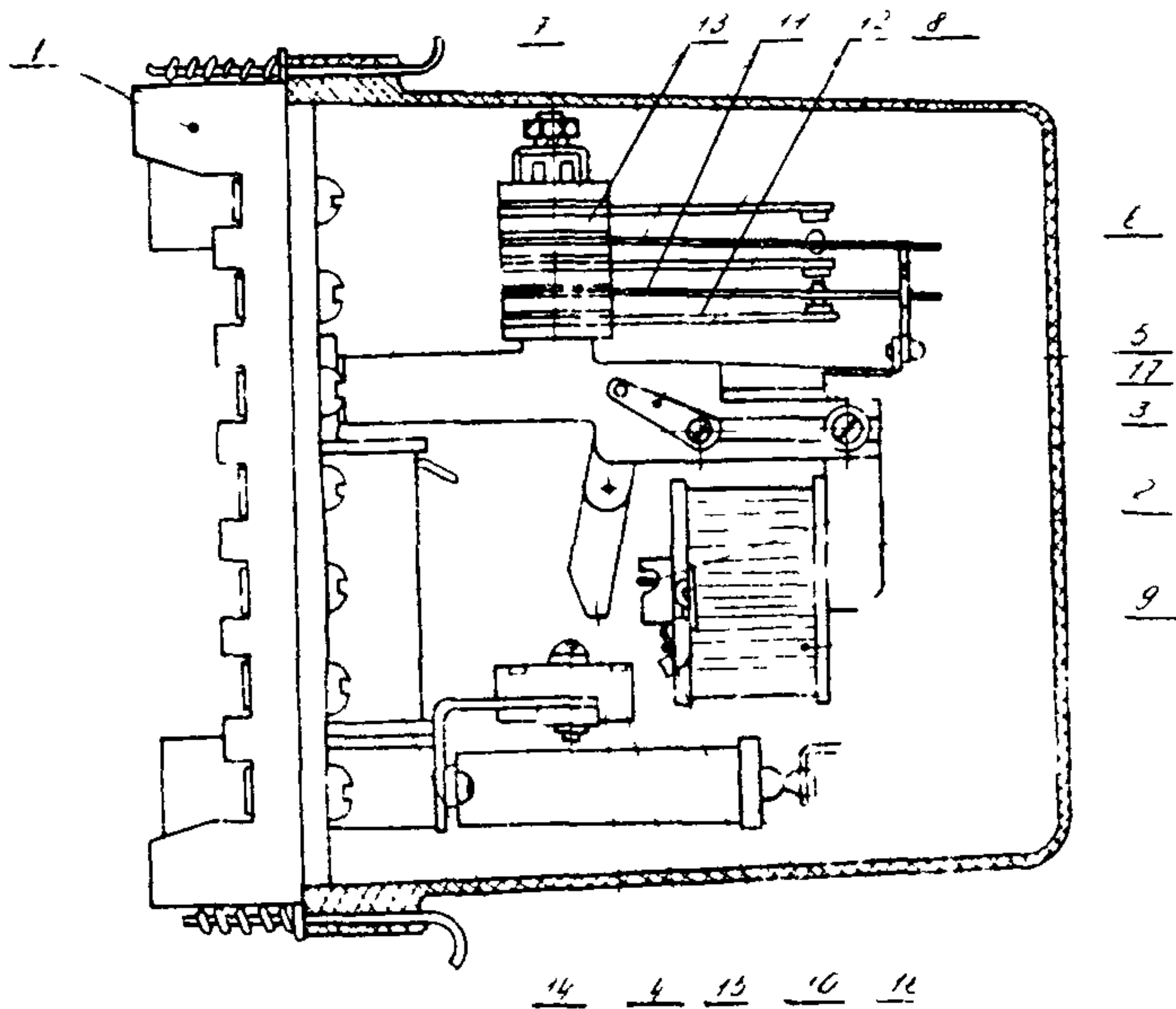
Рис. 9. Общий вид реле РР-32
