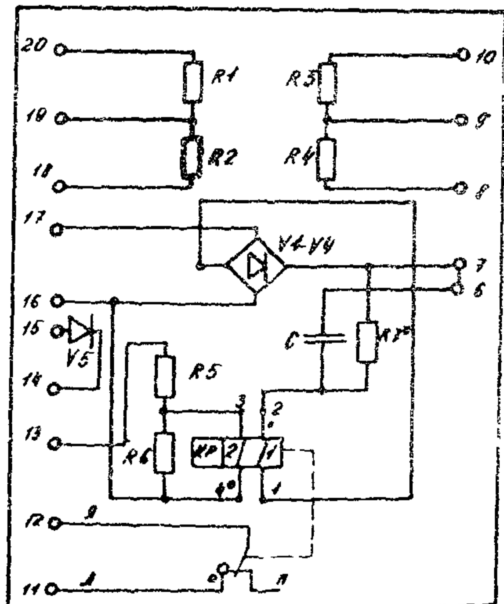
Рис. 15. Принципиальная схема реле РИС-33М
