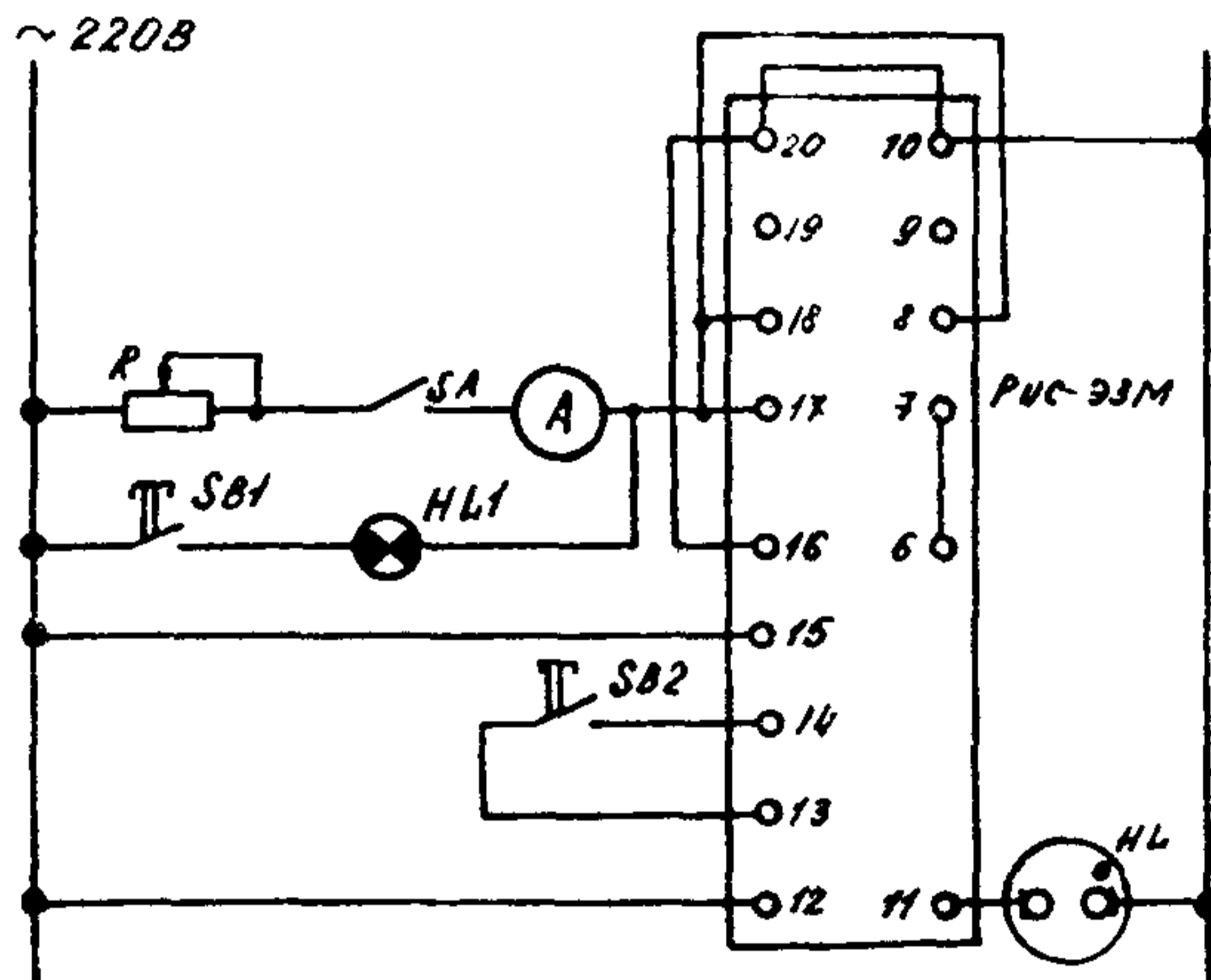
Рис. 24. Схема настройки реле РИС-33М
