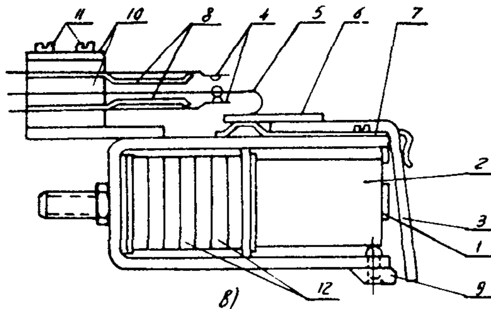
Рис. 8. Общий вид реле серии КДР:
