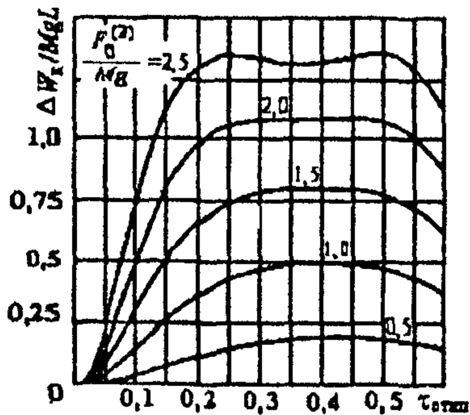
а) при 2L/a = 0,5 ;
