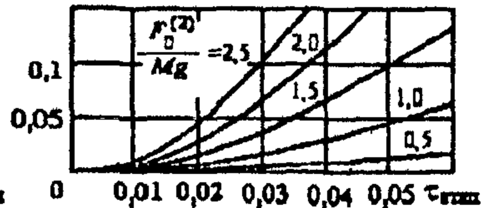
г) при 2L/a = 3,1 ;
