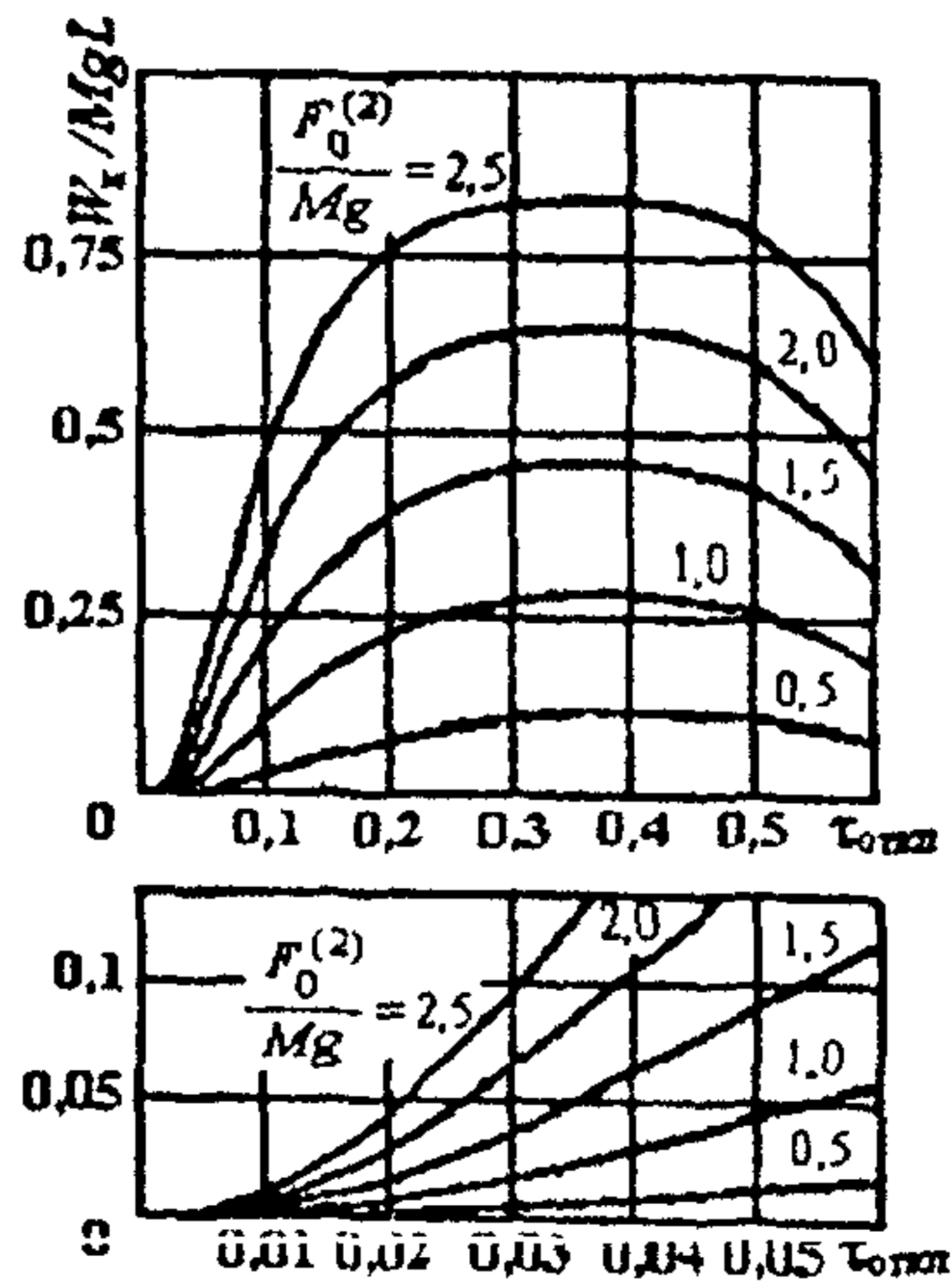
ж) при 2L/a = 5,7
