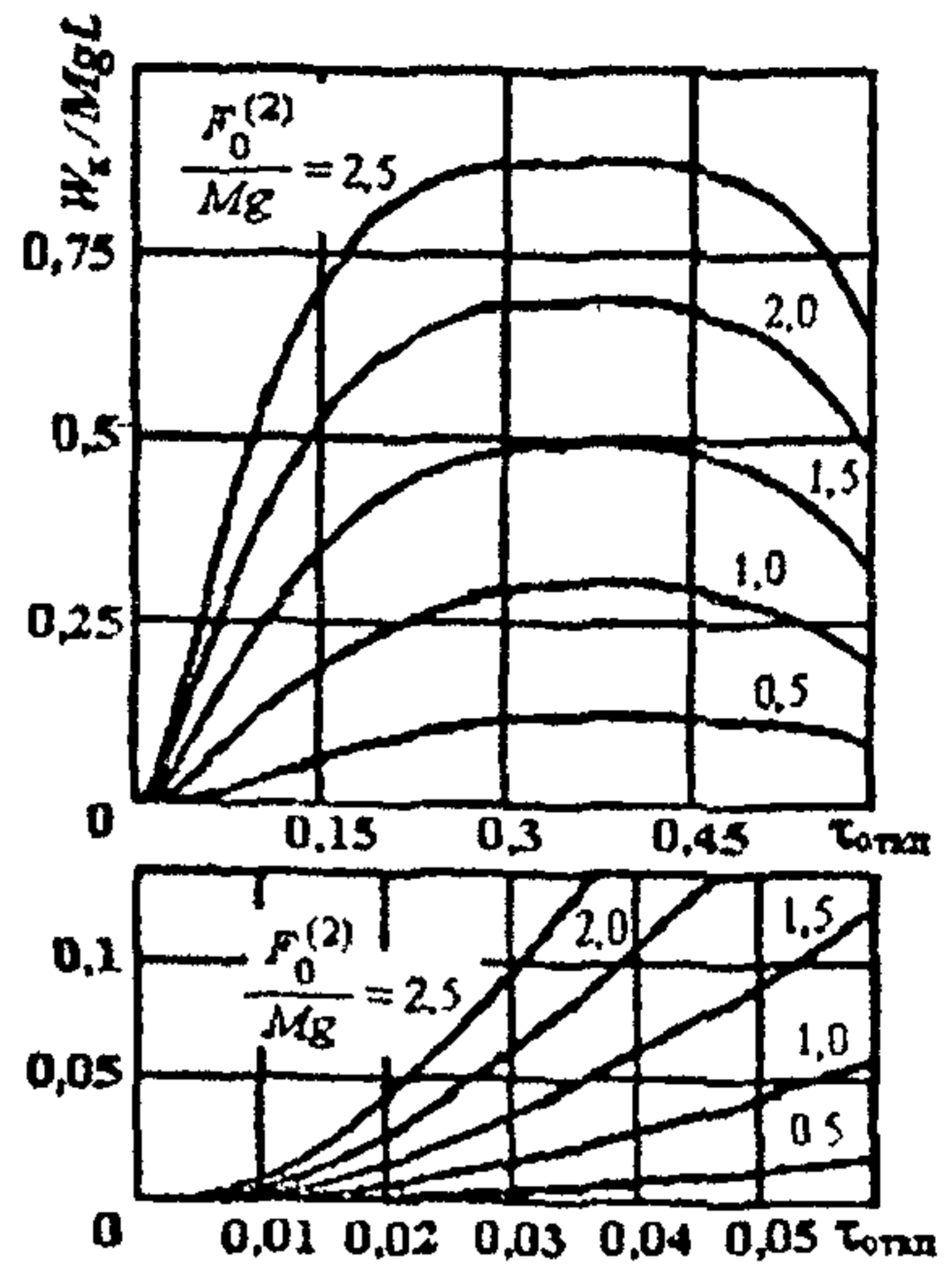
е) при 2L/a = 5,1 ;
