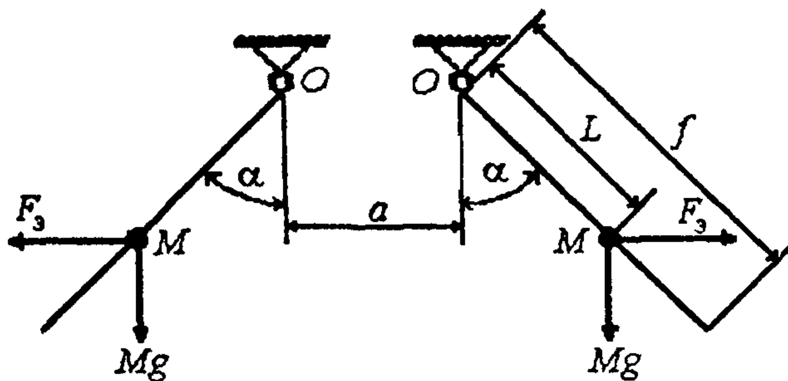
Рисунок 1 – Расчетная модель двух гибких проводников
