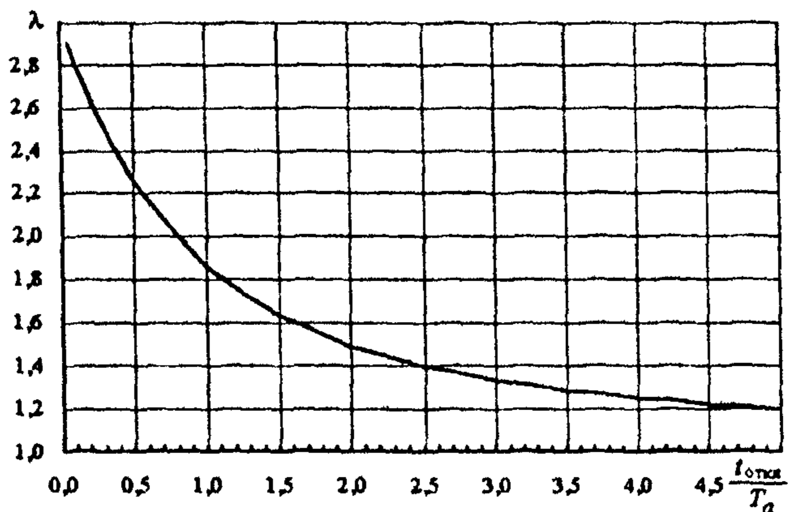
Рисунок 3 – Зависимость коэффициента \lambda от t_{откл} / T_a
