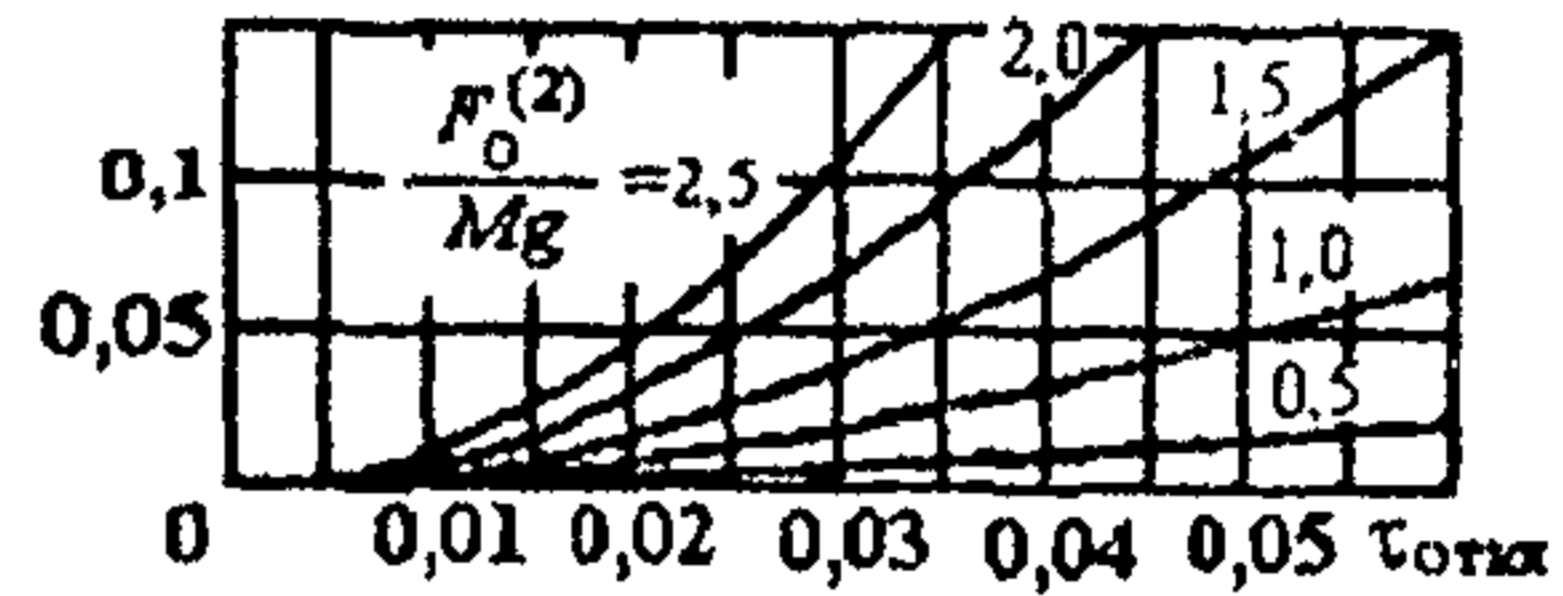
б) при 2L/a = 1,1 ;
