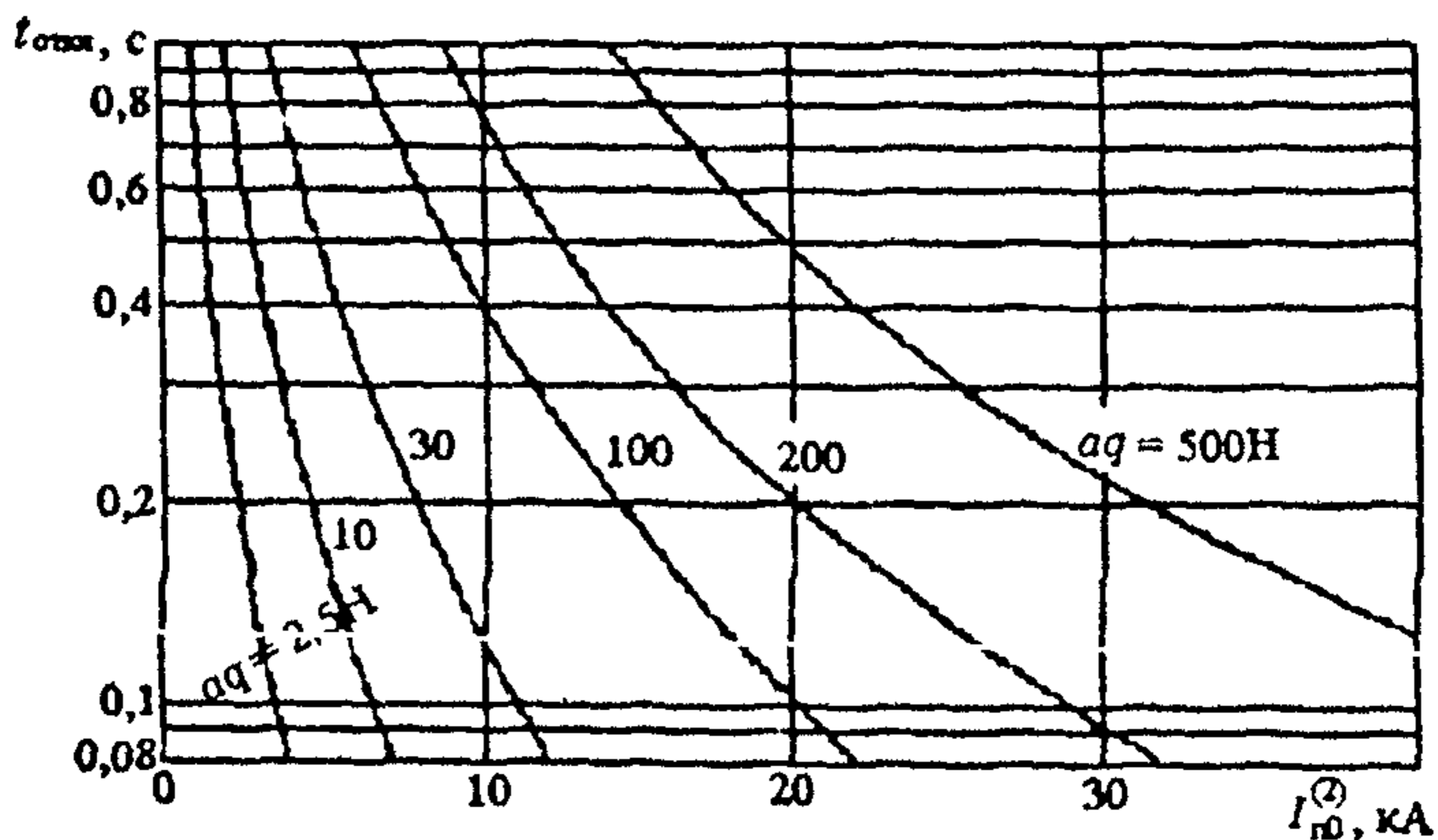
Рисунок 4 – Продолжительность КЗ, при которой p = 0,4
