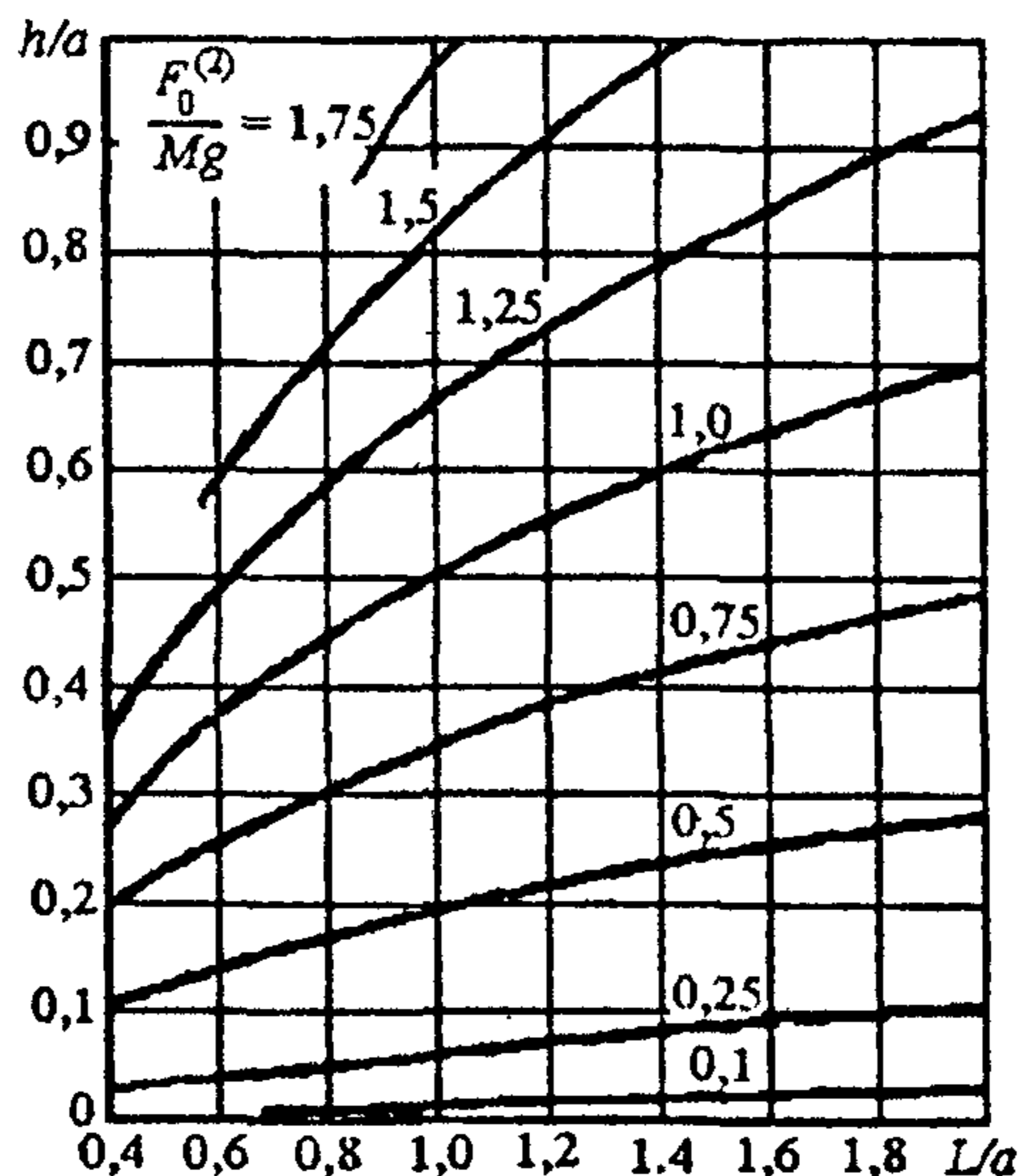
Рисунок 6 – Характеристики h/a при двухфазном КЗ
