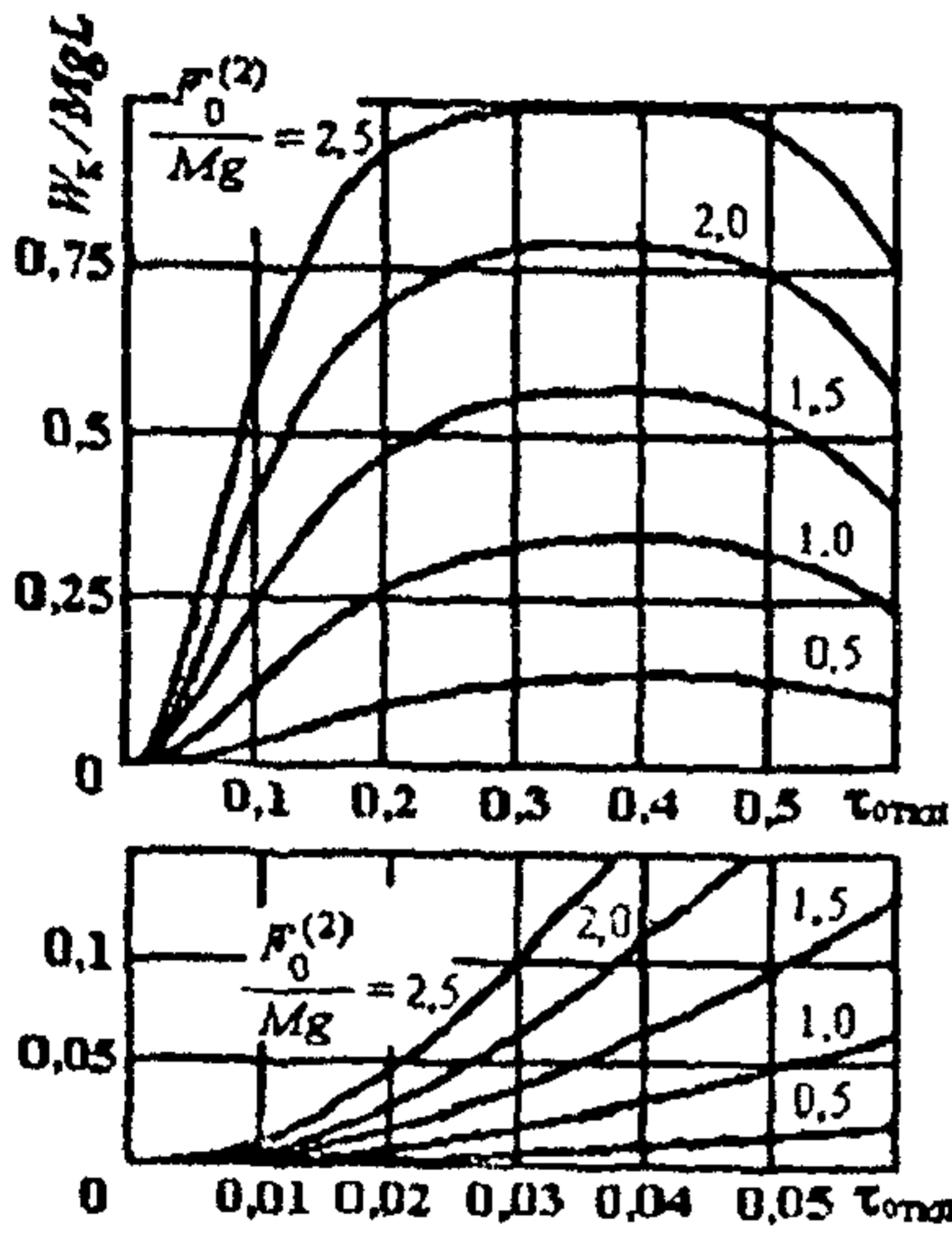
д) при 2L/a = 4,1 ;
