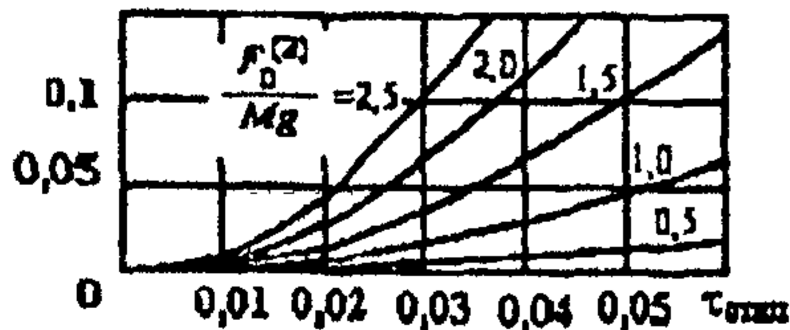
в) при 2L/a = 2,1 ;
