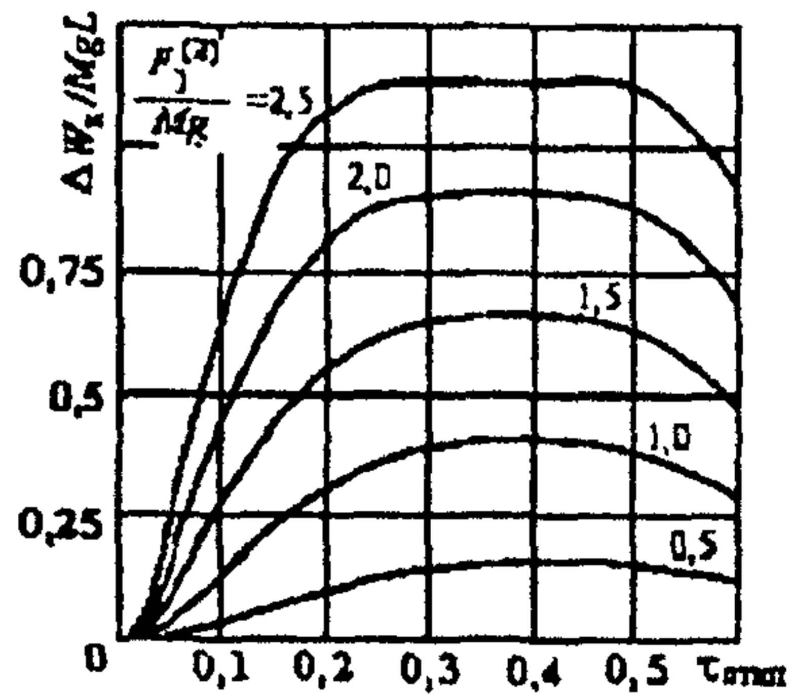
б) при 2L/a = 1,1 ;
