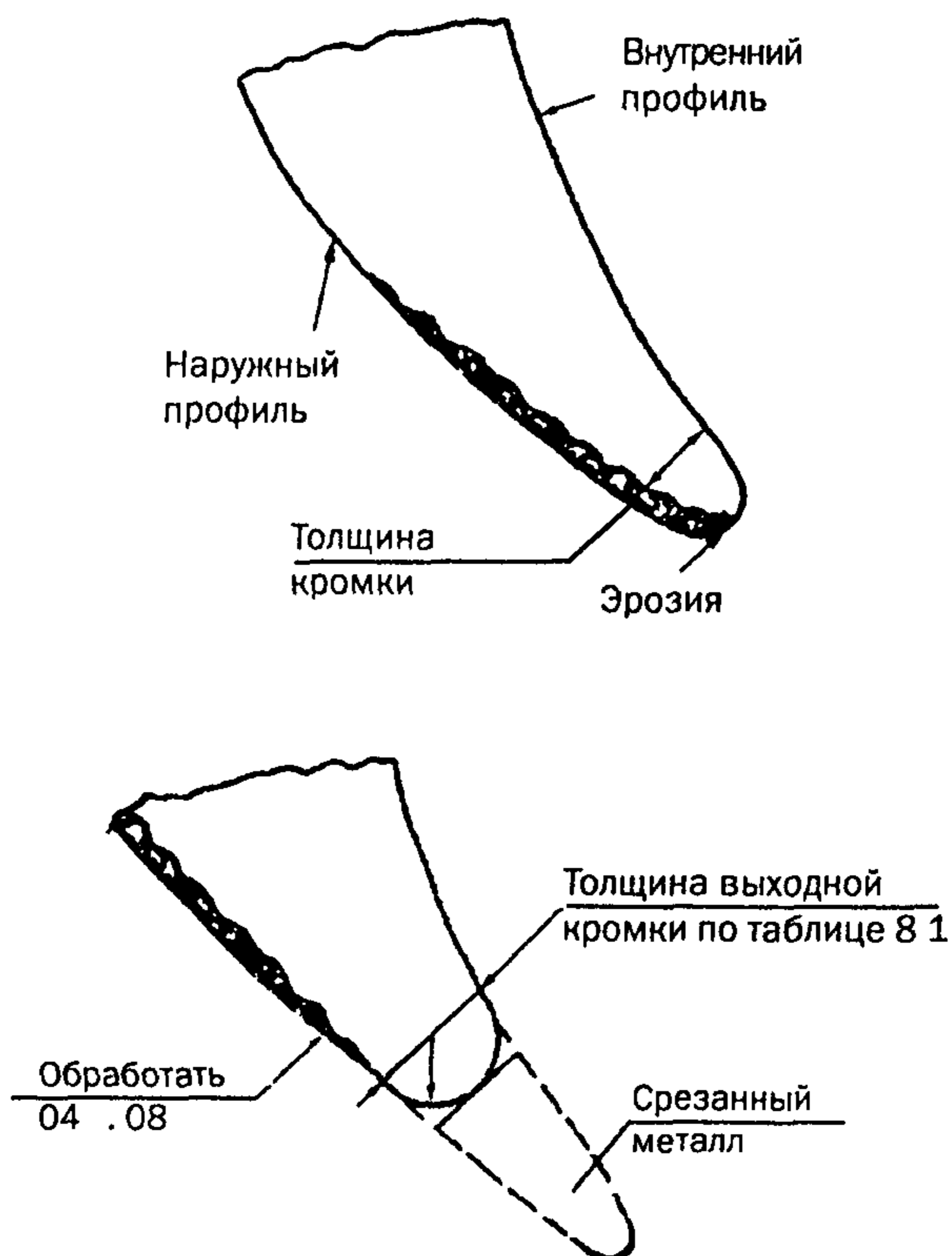
Рисунок 8.3 – Подрезка и обработка выходной кромки
