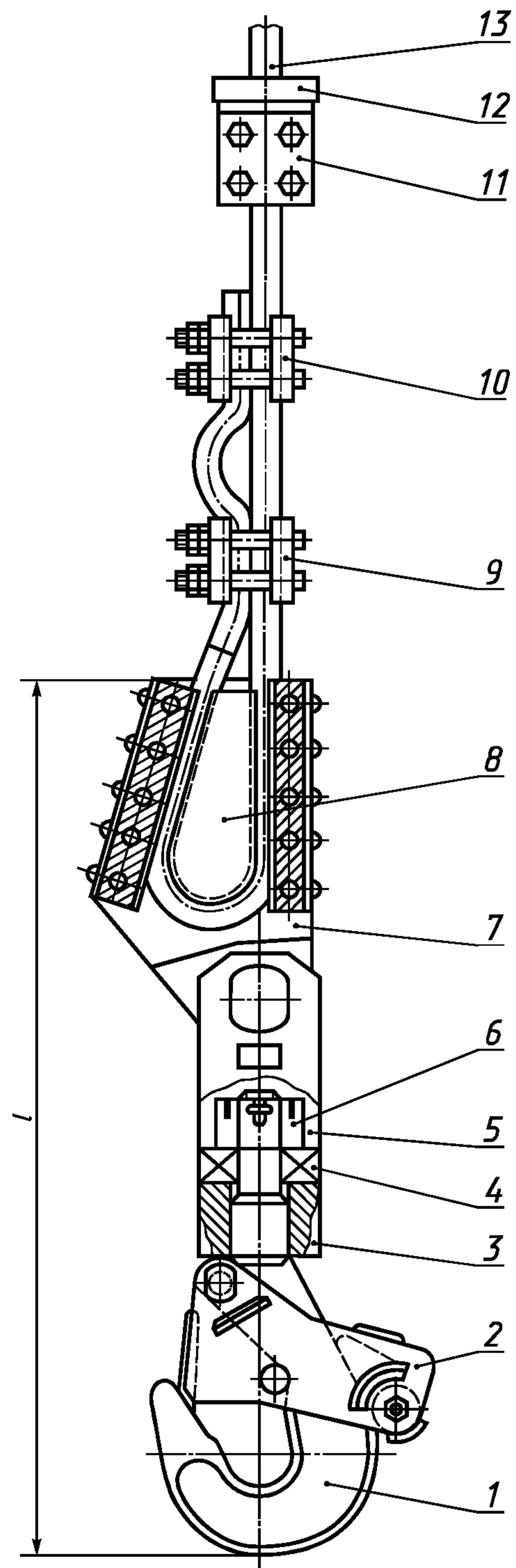
1 — крюк; 2 — защелка; 3 — траверса; 4 — упорный подшипник; 5 — щеки; 6 — гайка; 7 — клиновья втулка; 8 — клин; 9 — рабочий жимок; 10 — контрольный жимок; 11 — опорный жимок; 12 — амортизатор; 13 — подъемный канат
