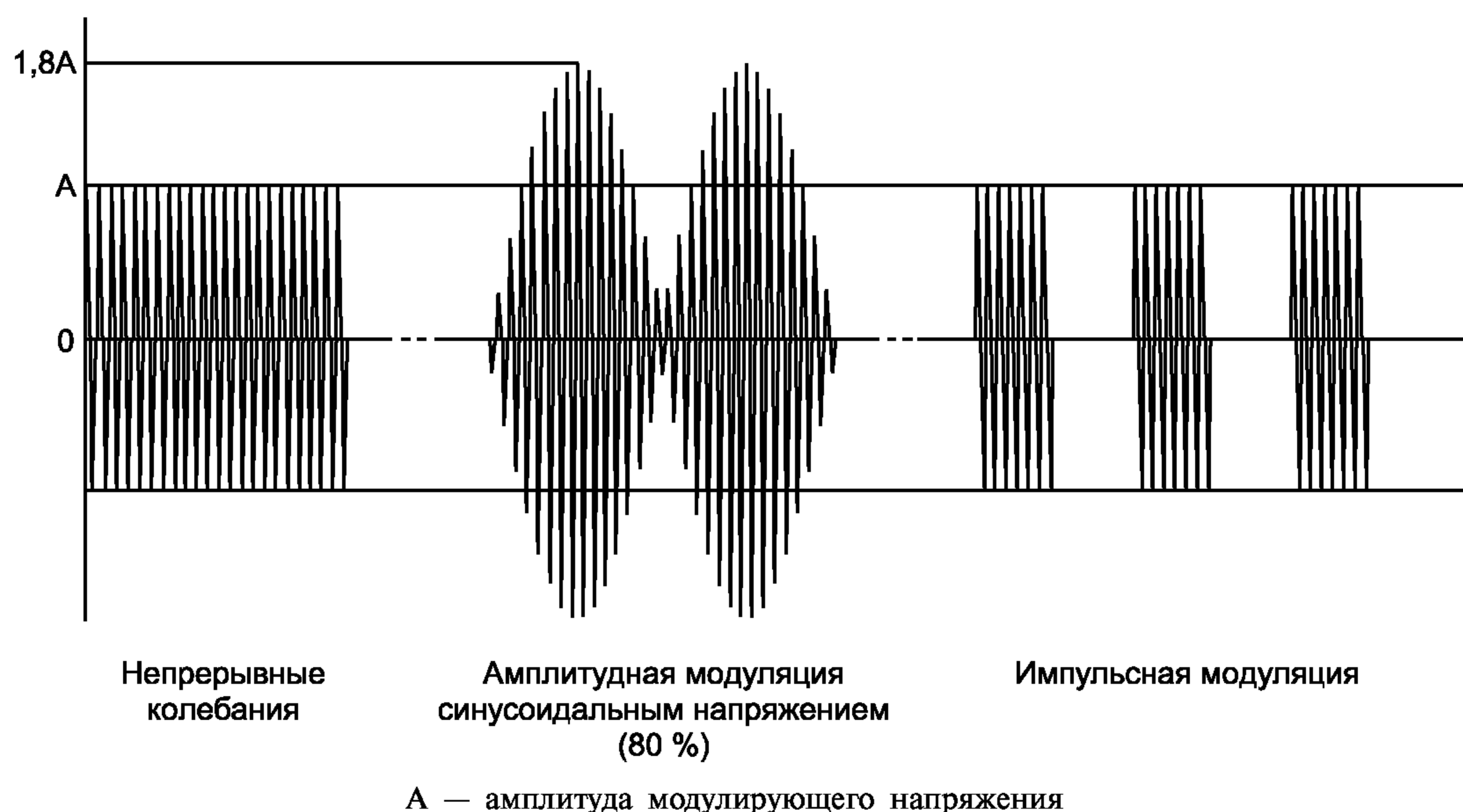
Рисунок 3 — Виды модуляции
