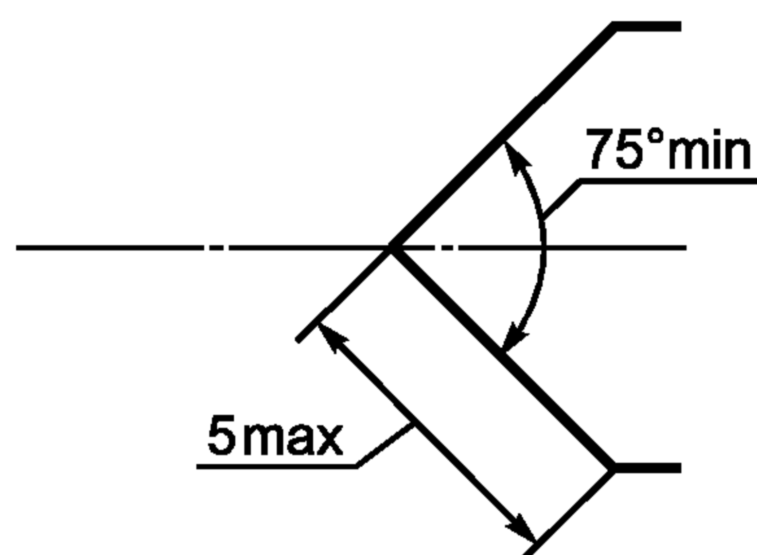
Рисунок 1 — Угол схождения боковых граней острия клинка
