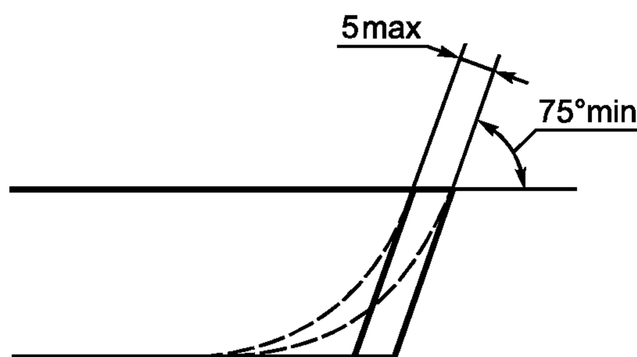
Рисунок 2 — Угол схождения обуха и лезвия клинка
