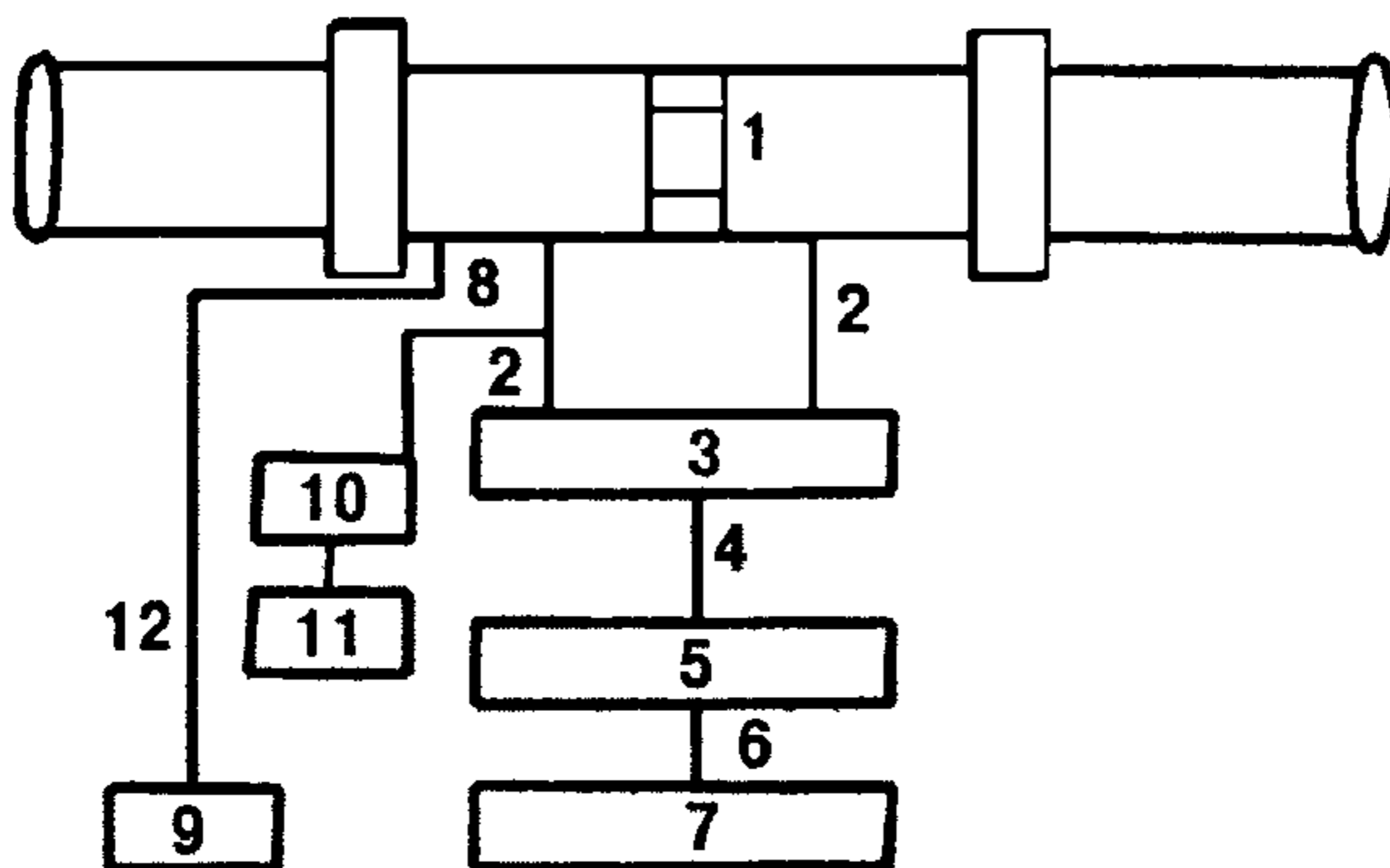
Рис. 1. Структурная схема измерительной системы с использованием локального РСИ (децентрализованная система):
