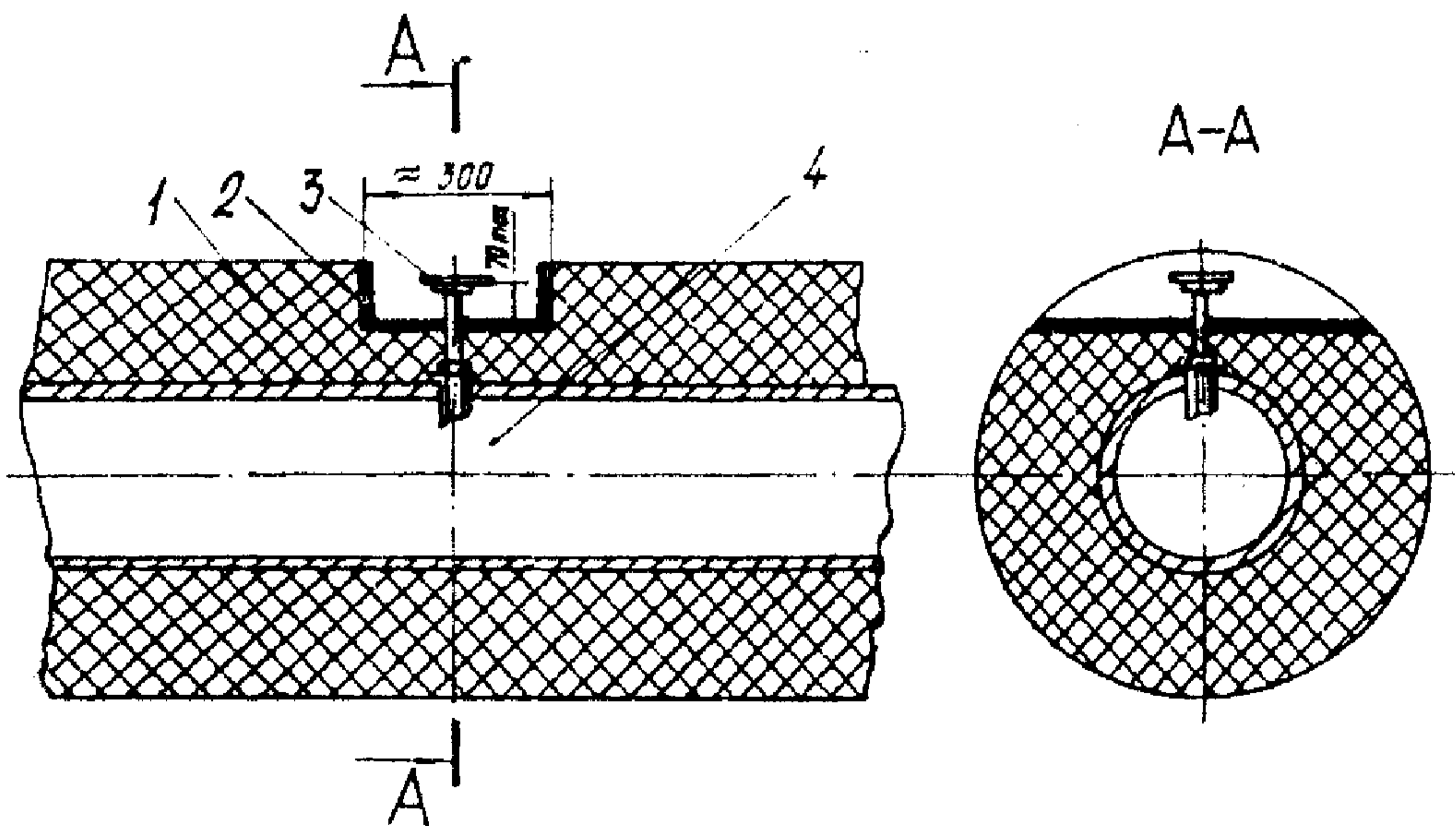
Тепловая изоляция мест установки термоэлектрических преобразователей:
