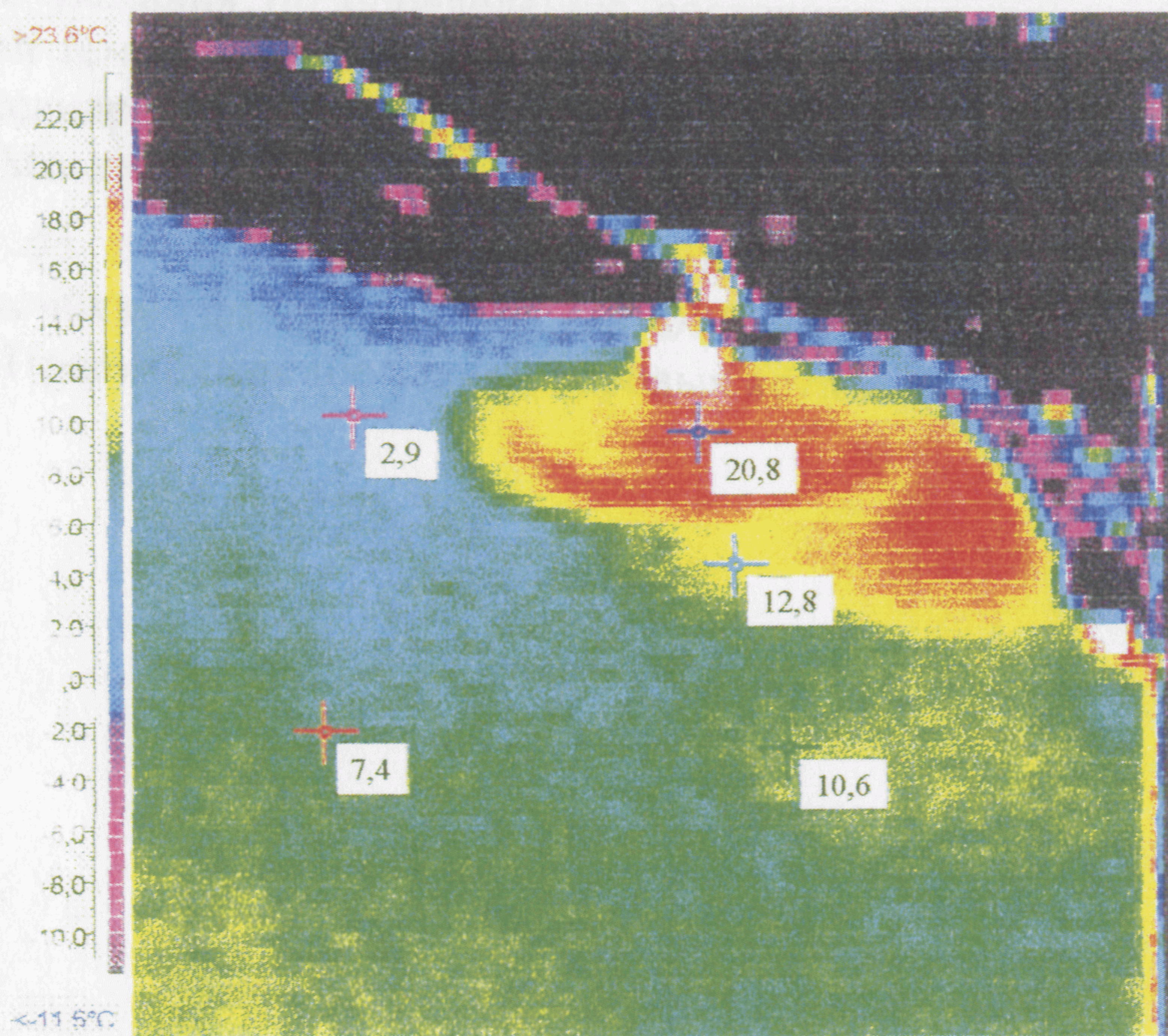
Рис.6.2 Распределение температур на поверхности пруда охладителя ТЭЦ
