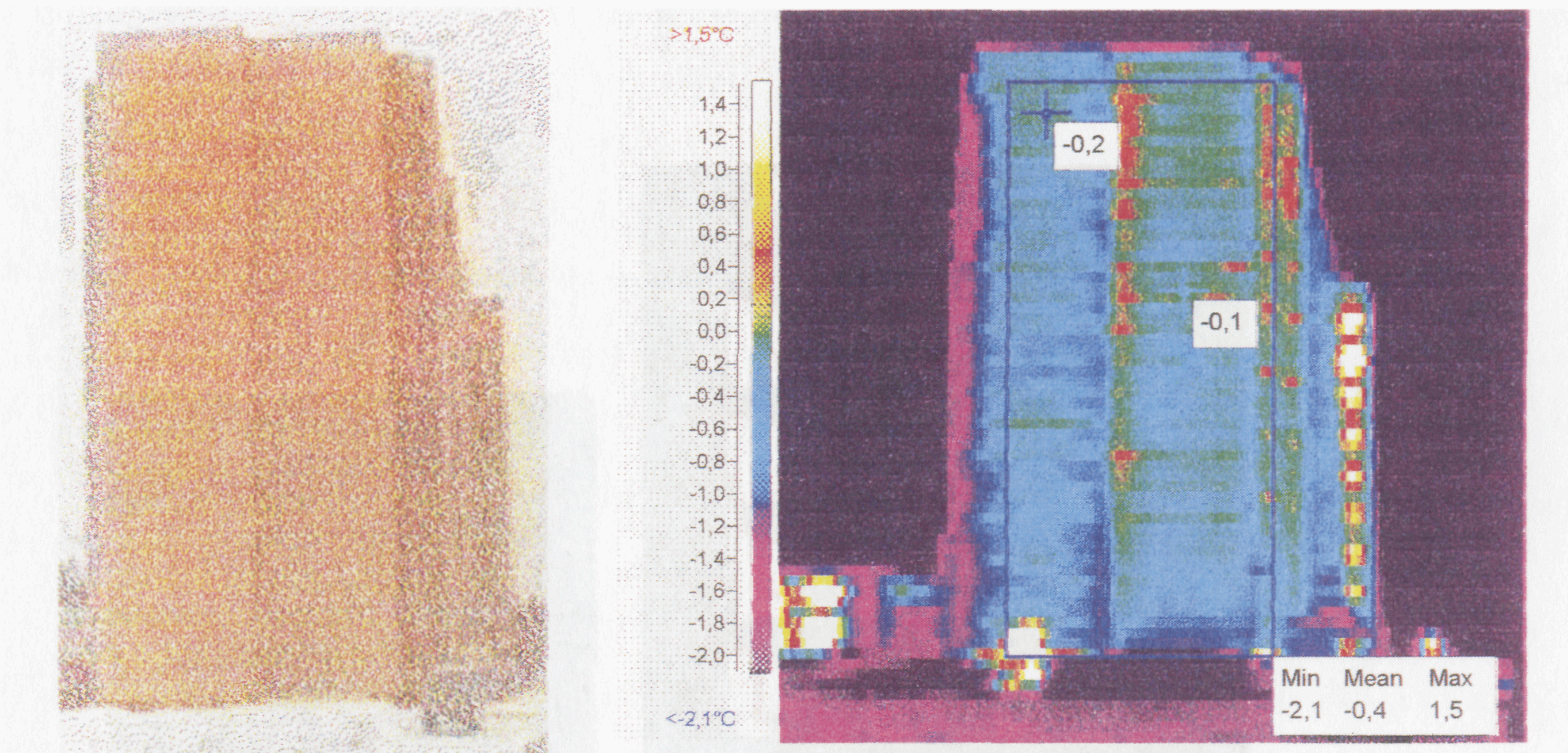
Рис. 1-9 Торцевая часть 9-ти этажного здания. Поверхность с t = -0,4^{\circ}\text{C} , можно принять за базовый участок. Красная полоса в центре здания вызвана тепловым отражением.
