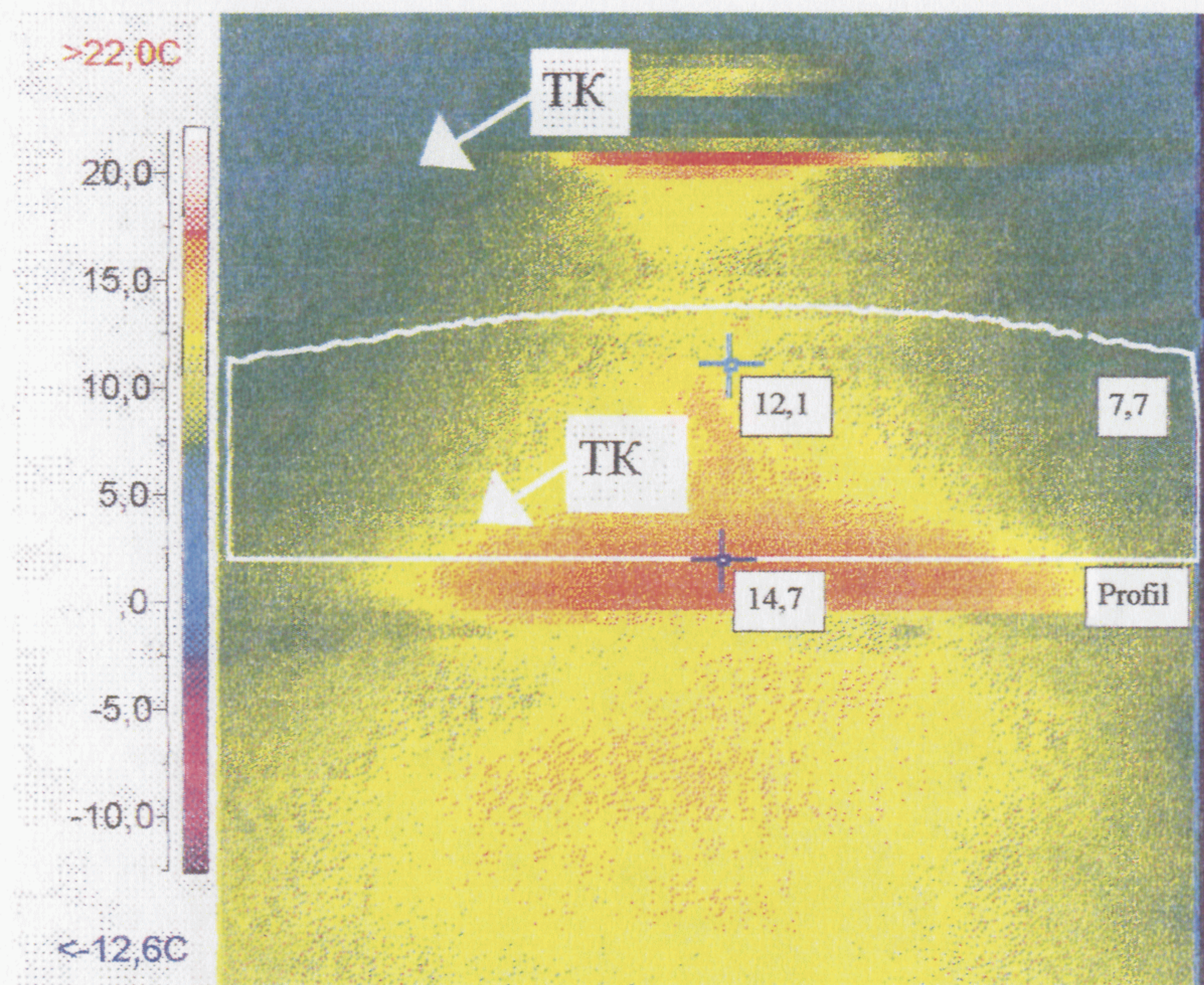
Рис. 5.9 Участок теплотрассы без дефектов
