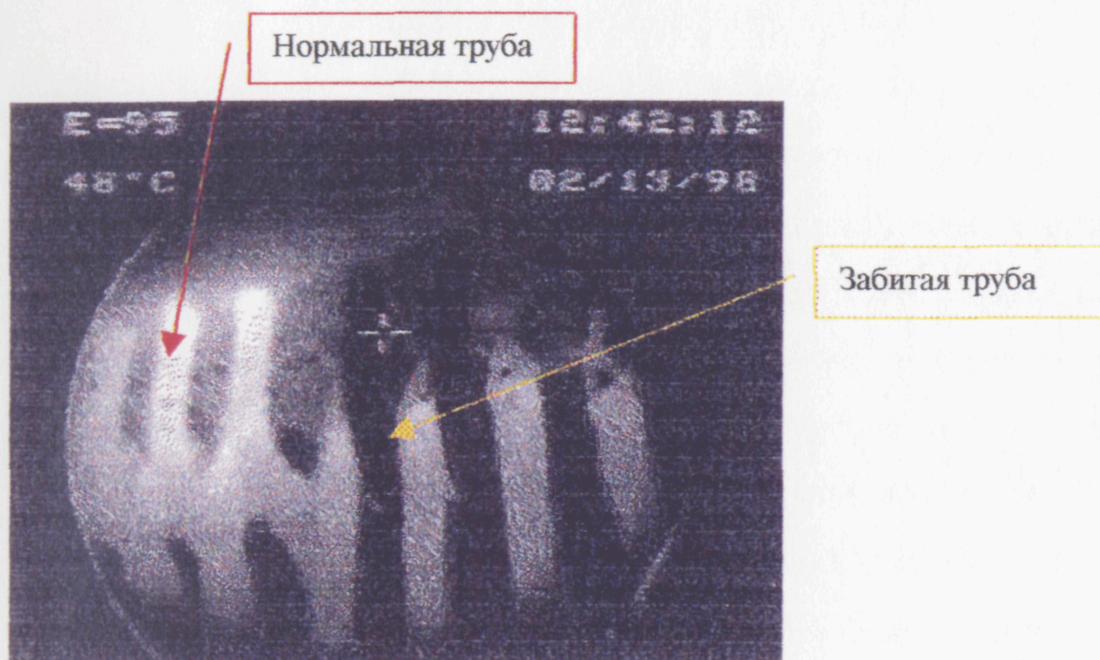
Рис. 3.1 Термограмма труб поверхностей нагрева котла.
