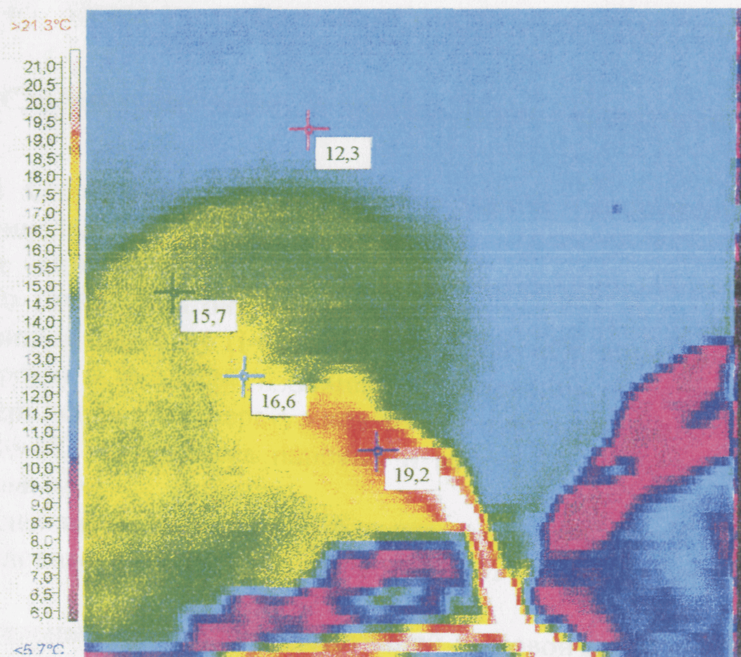
Рис. 6.1 Распределение температур на поверхности пруда охладителя ТЭЦ
