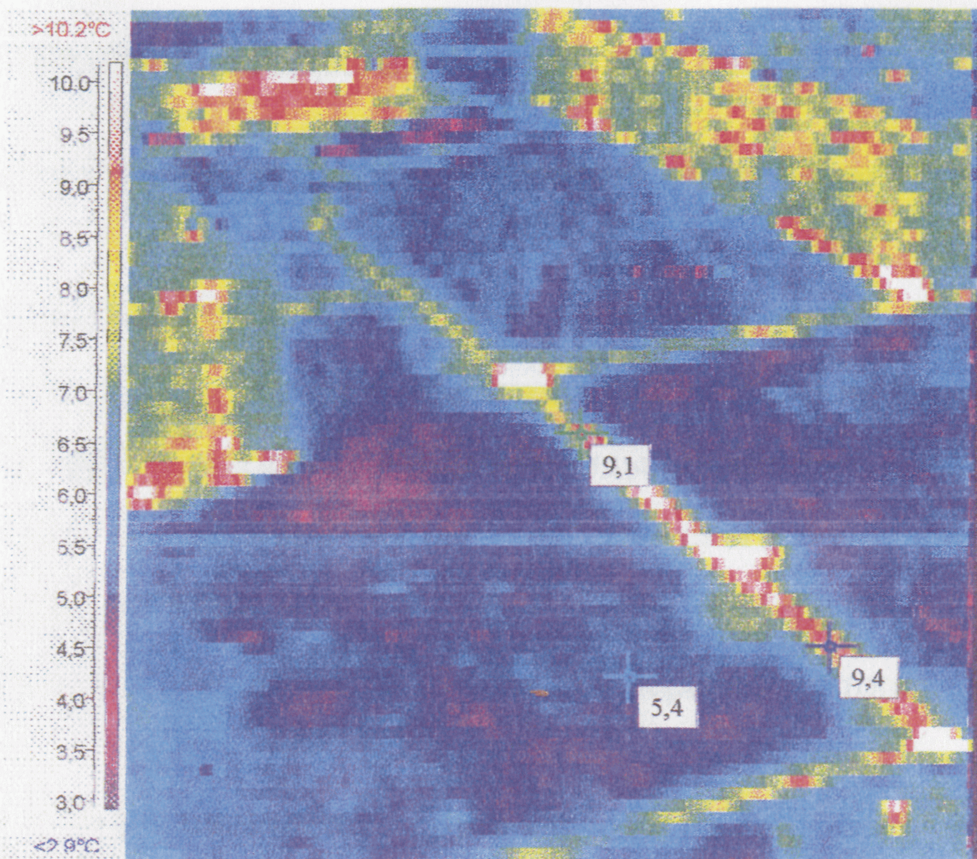
Рис. 5.10 Затопленный участок подземной теплотрассы (съемка с вертолета)
