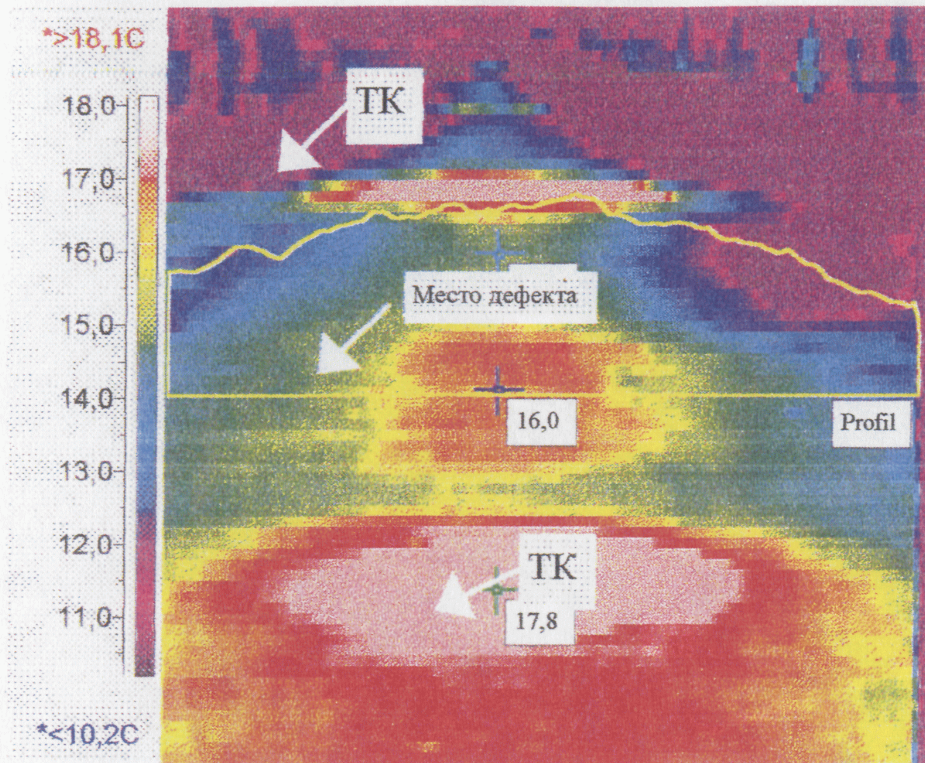
Рис. 5.8 Участок подземной теплотрассы с нарушенной изоляцией.
