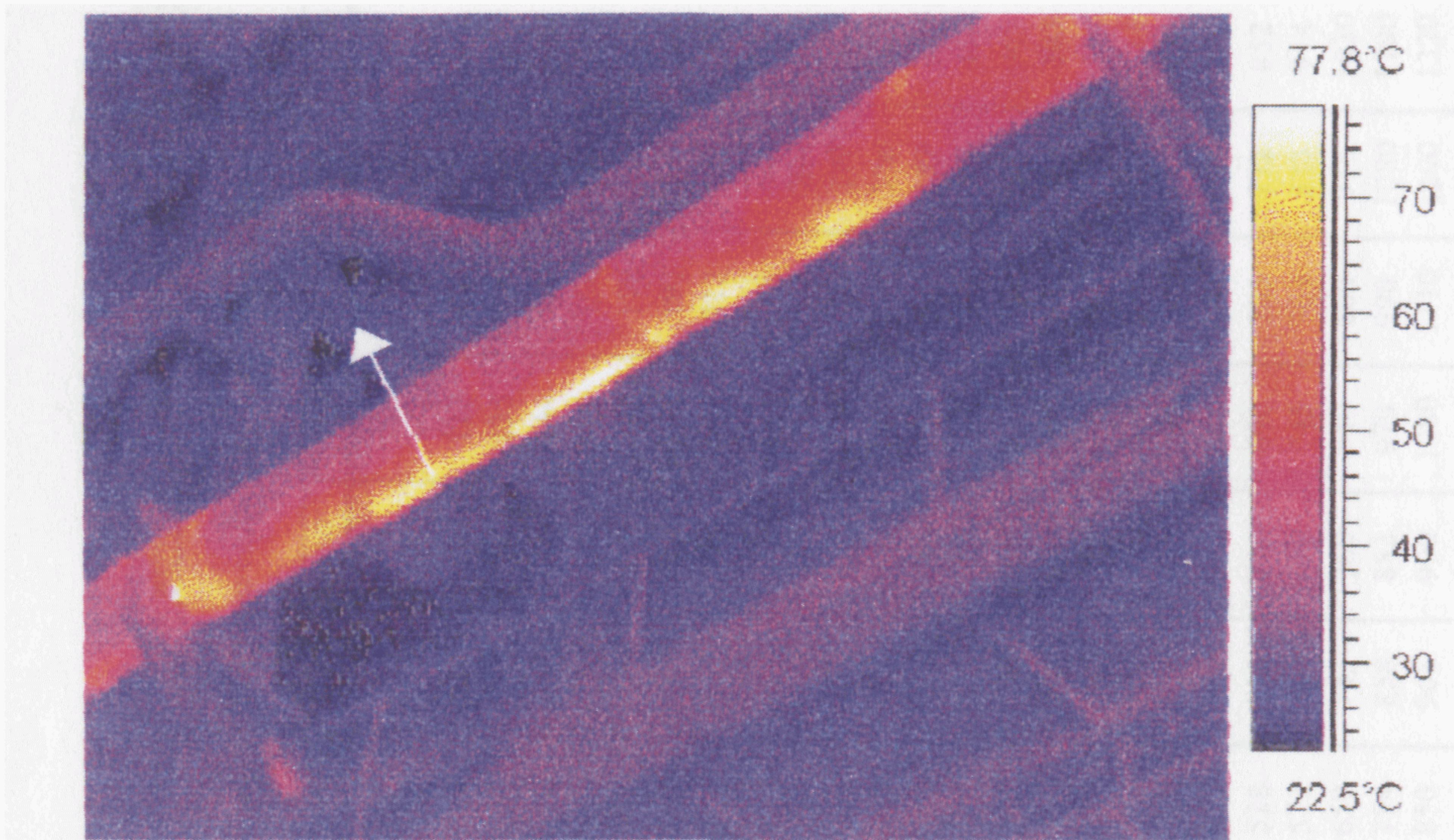
Рис.2.3 Участок паропровода с повышенными теплотерями.
