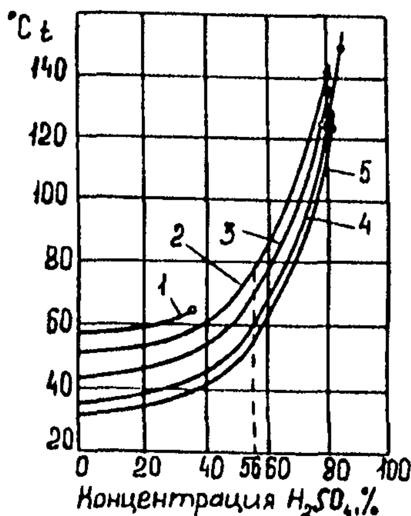
Рис. 6. Зависимость концентрации серной кислоты от температуры дымовых газов различных топлив: 1 — торф; 2 — подмосковный уголь; 3 — мазут и сушенка подмосковного угля, 4 — кизеловский уголь и промпродукт; 5 — тощий уголь
