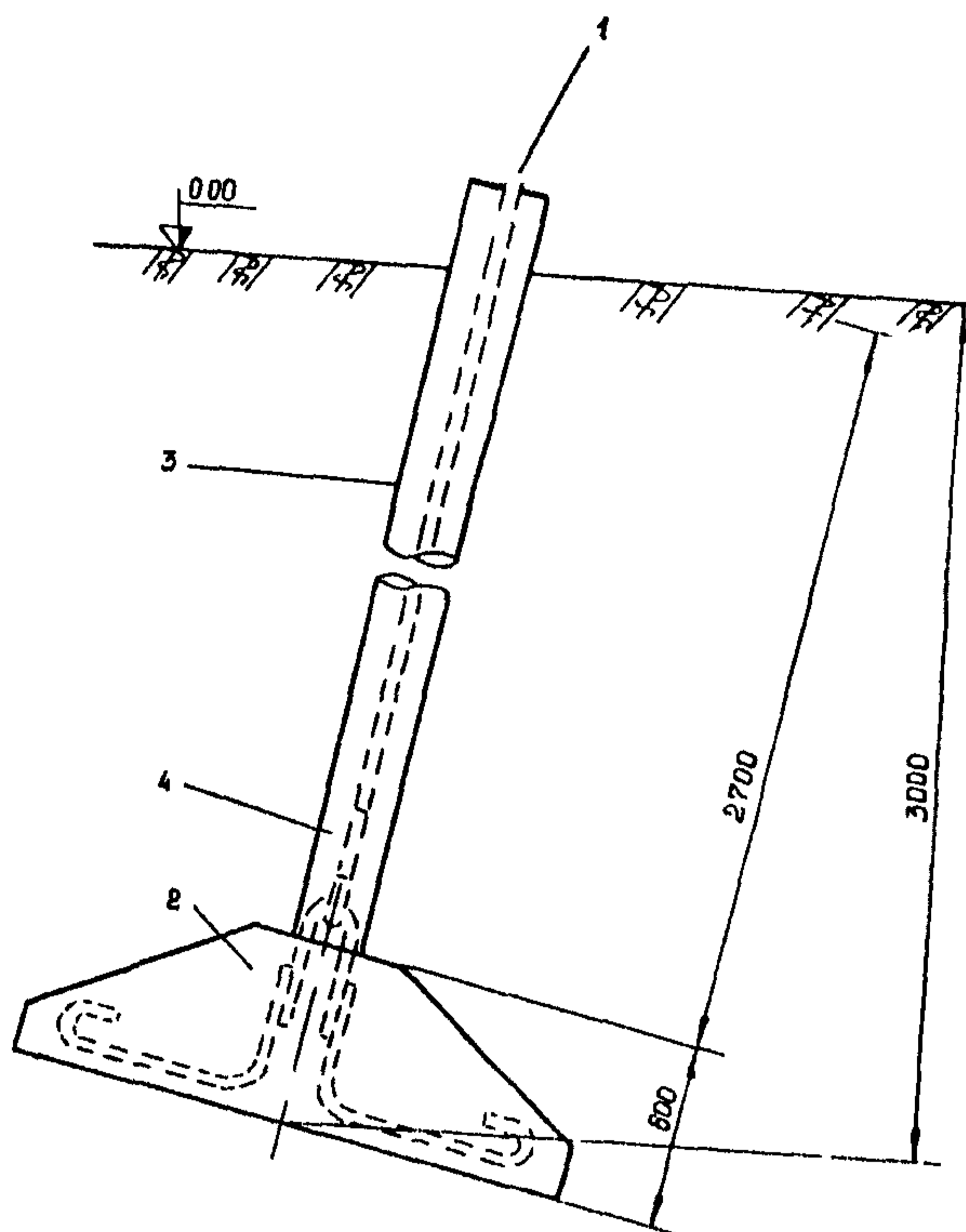
Рис. 7. Анкерное крепление вантовой оттяжки металлической дымовой трубы:
