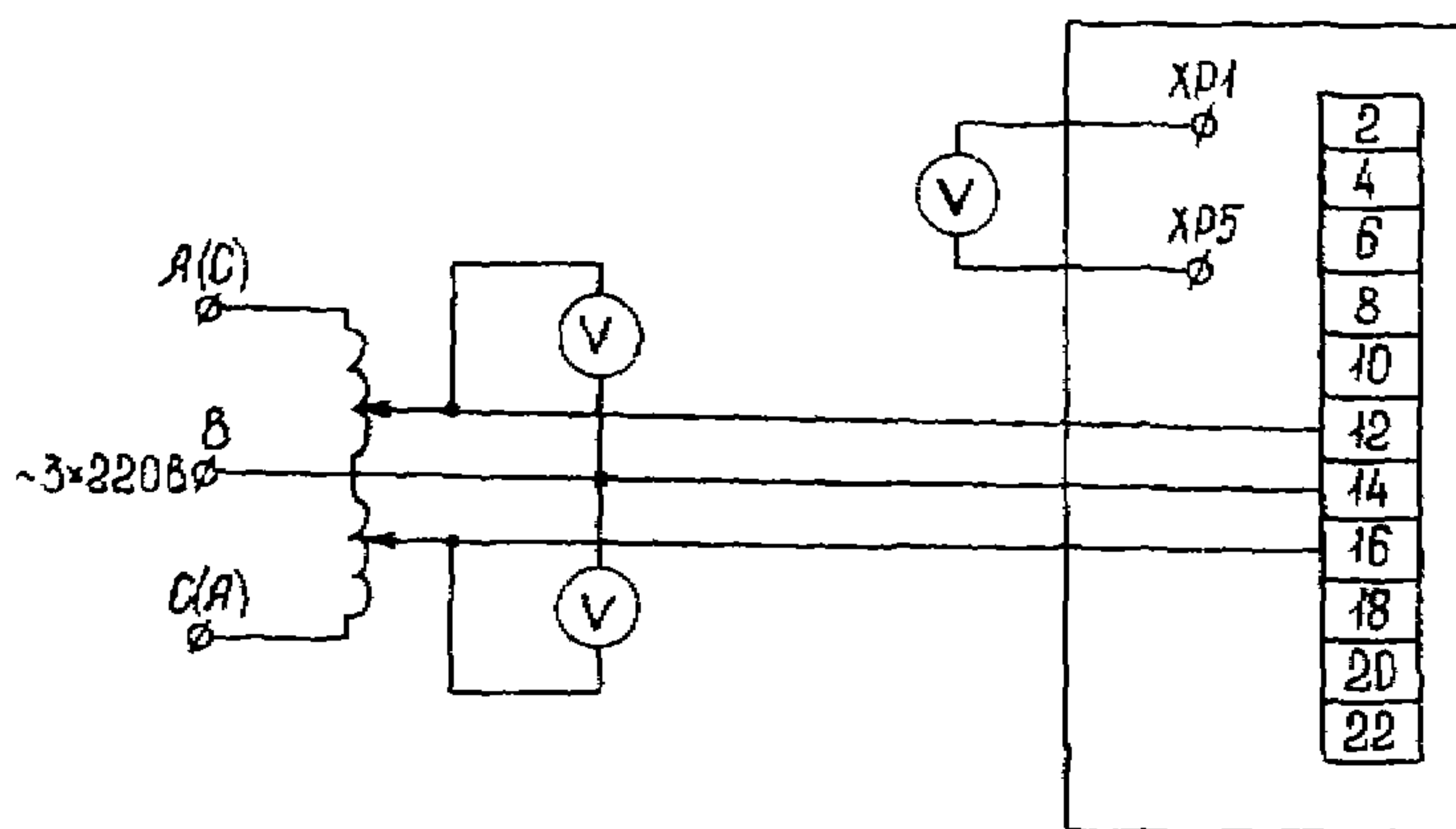
Рис. 4. Схема для испытания фильтра обратной последовательности
