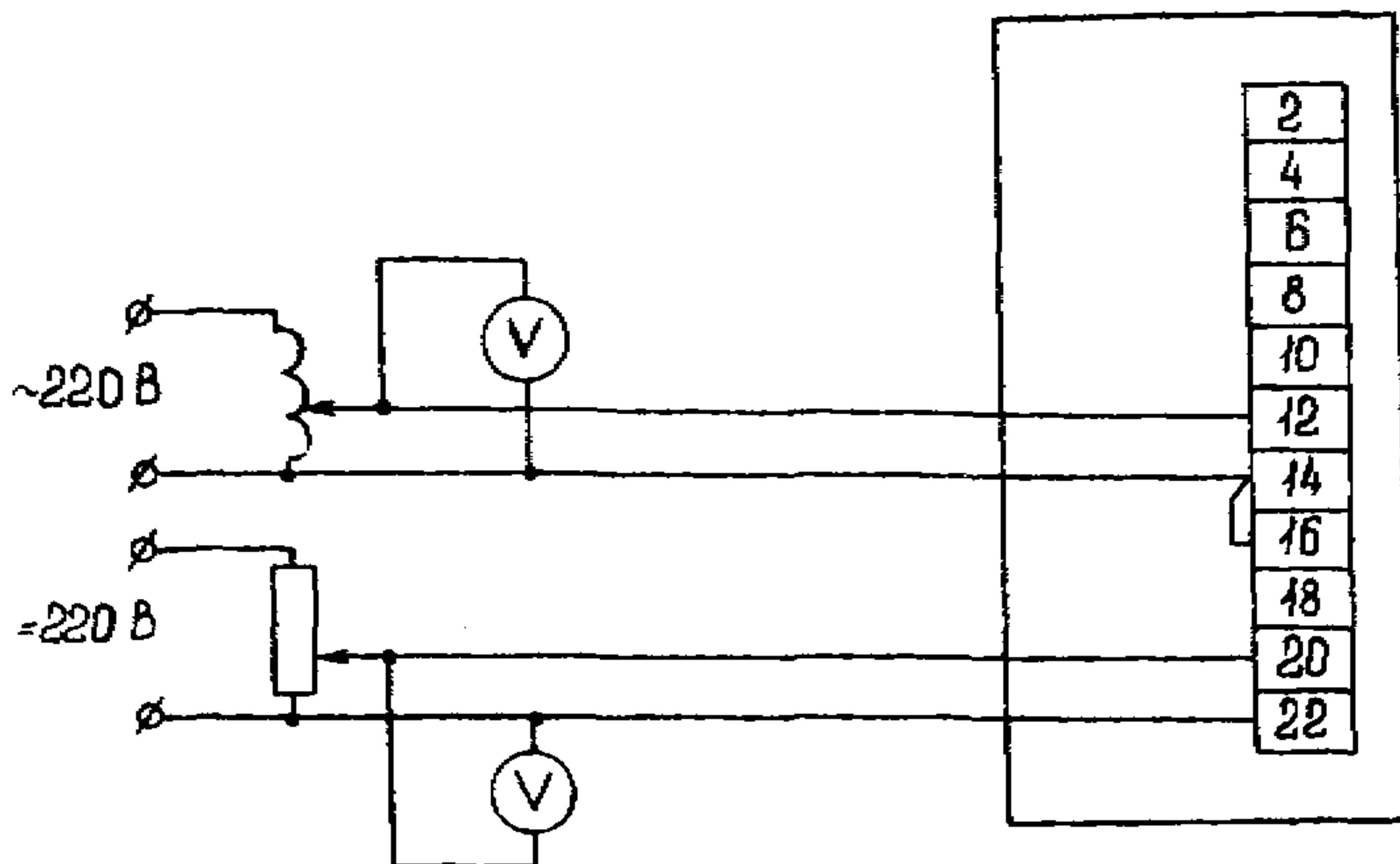
Рис. 3. Схема испытаний реле
