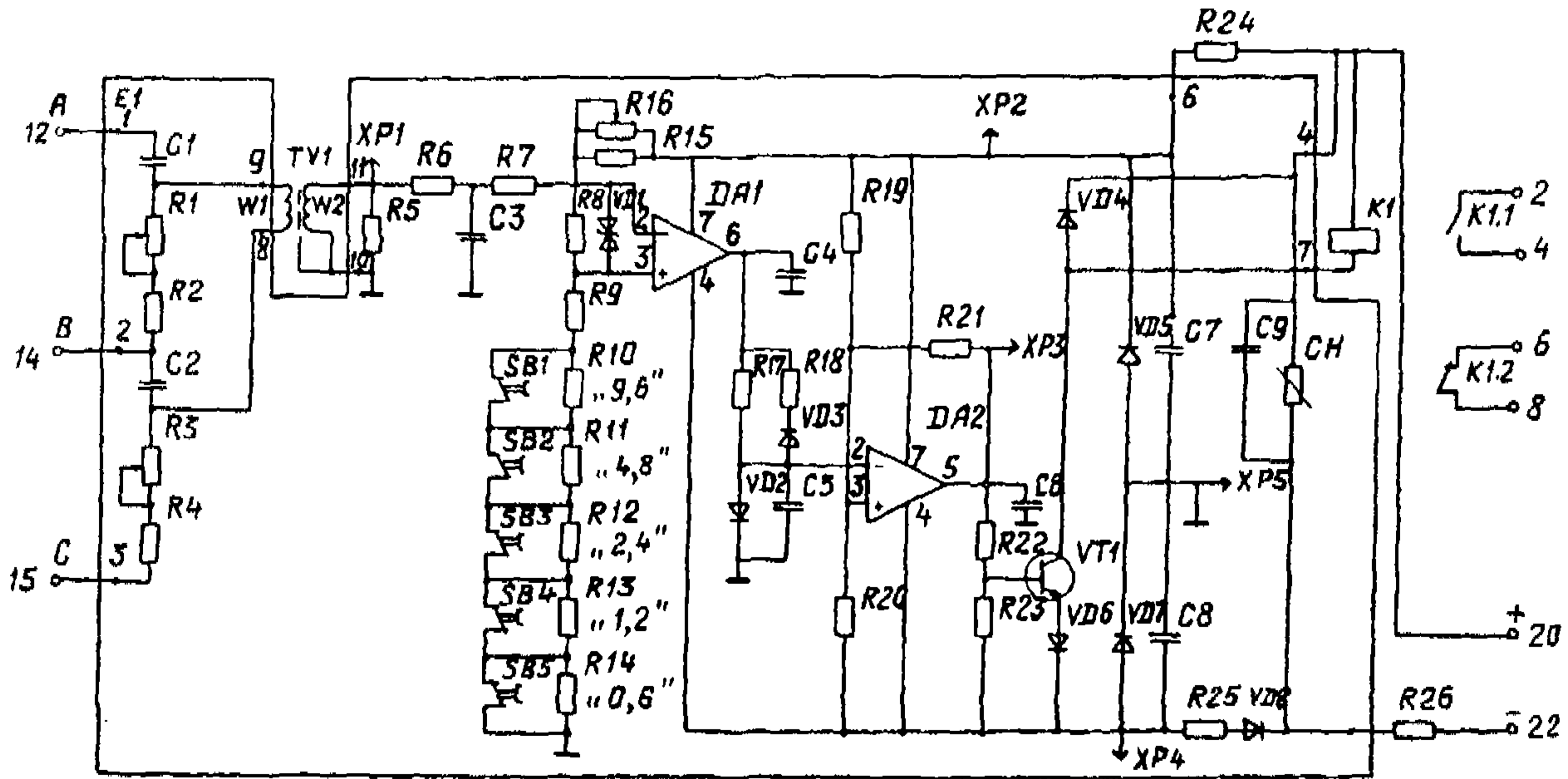
Рис. 2. Принципиальная схема реле
