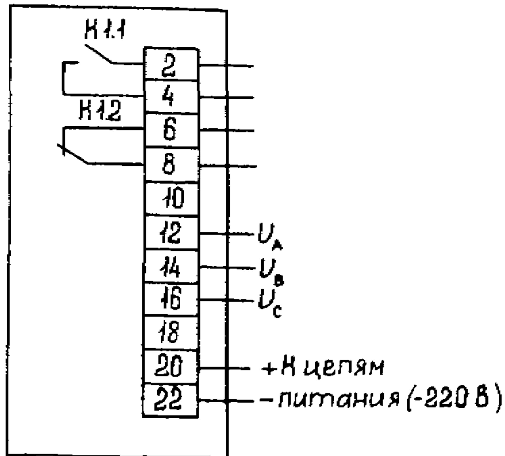
Рис. 1. Схема подключения реле
