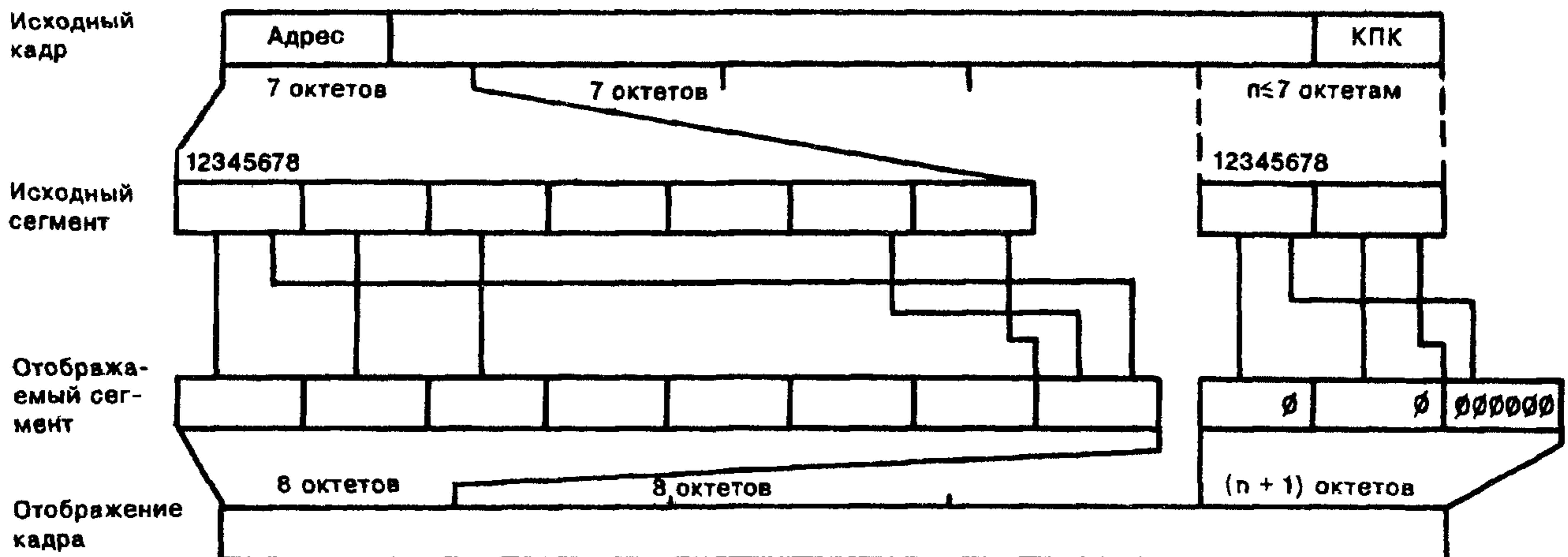
Рисунок 1 — Переход от исходного кадра к отображению кадра
