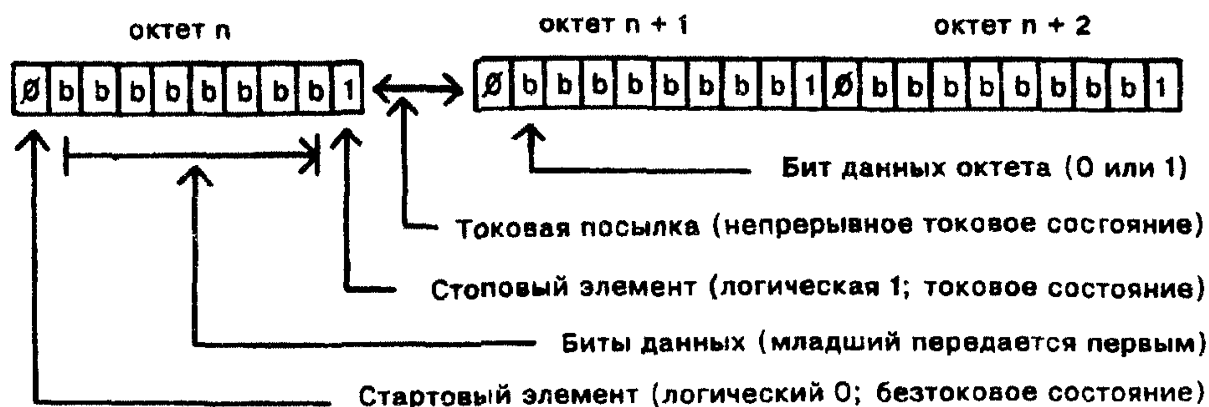
Рисунок 2 — Типичная передача октета при стартстопной передаче
