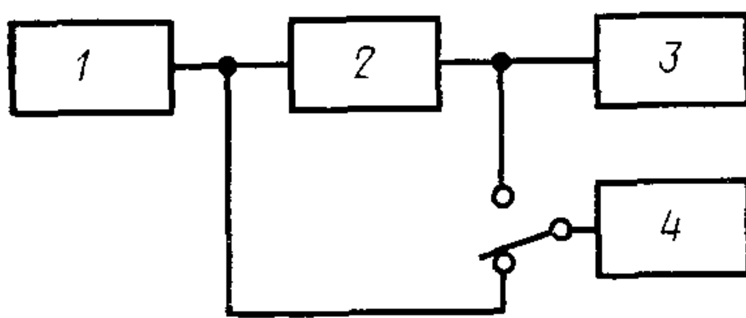
1—поверяемый генератор; 2—режекторный фильтр; 3—анализатор гармоник; 4—вольтметр
