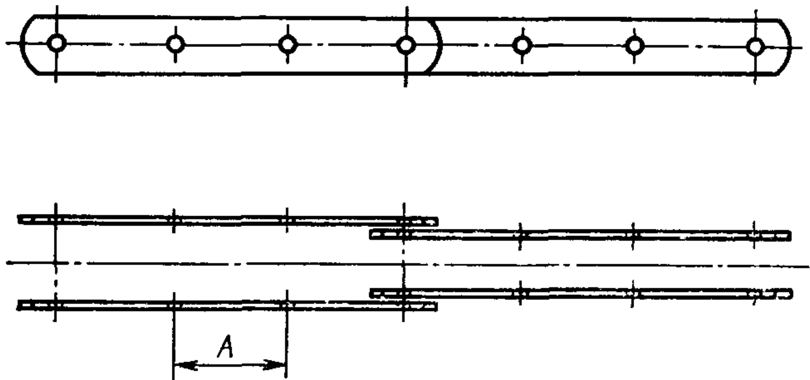
Тип 2.2
