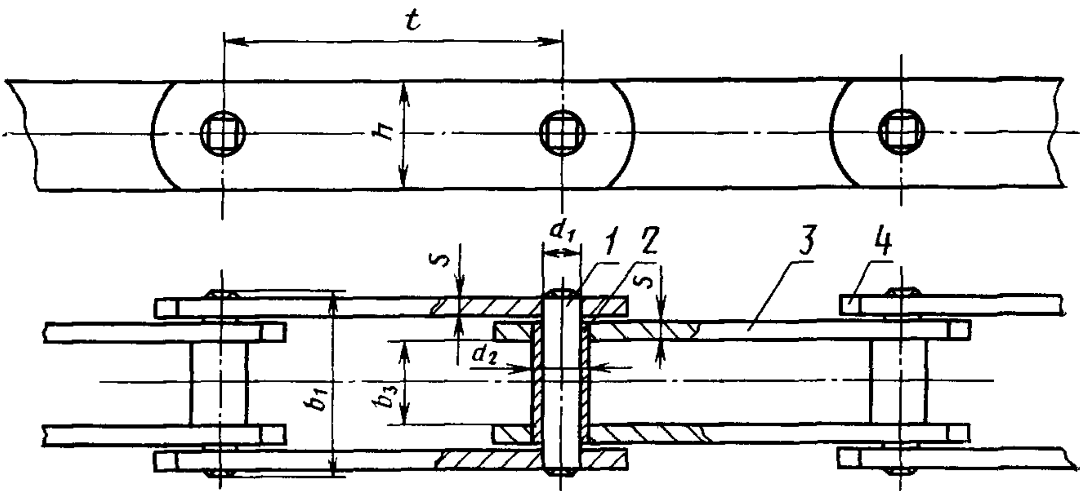
Исполнение 1
