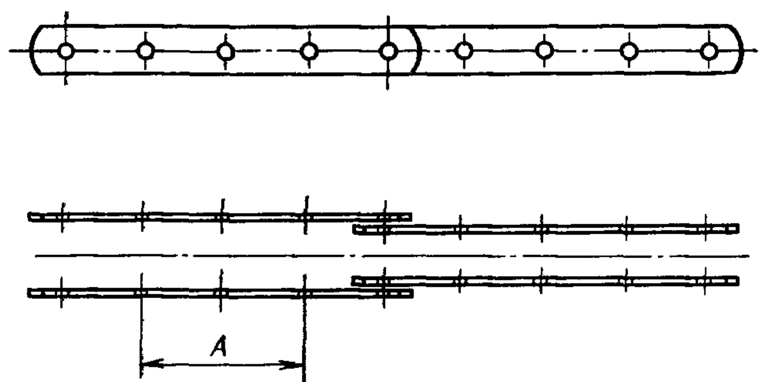
Тип 2.3
