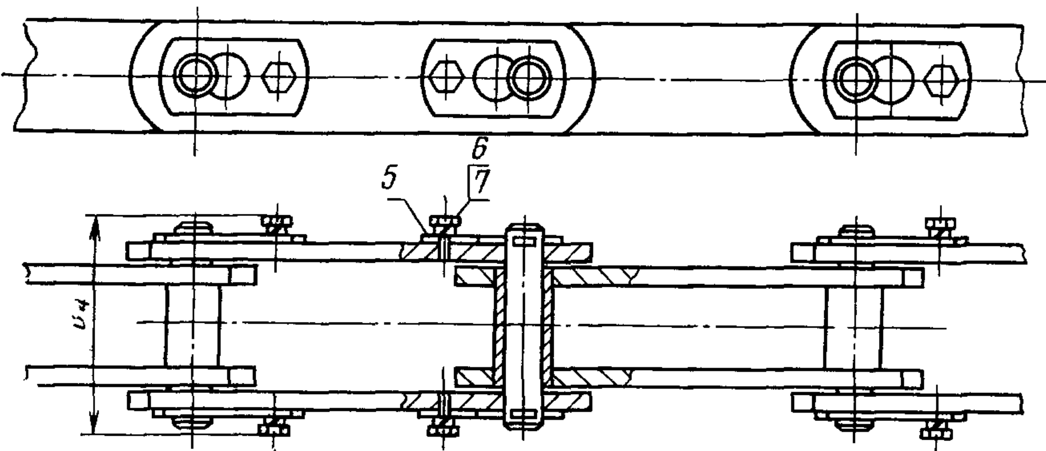
Исполнение 2
