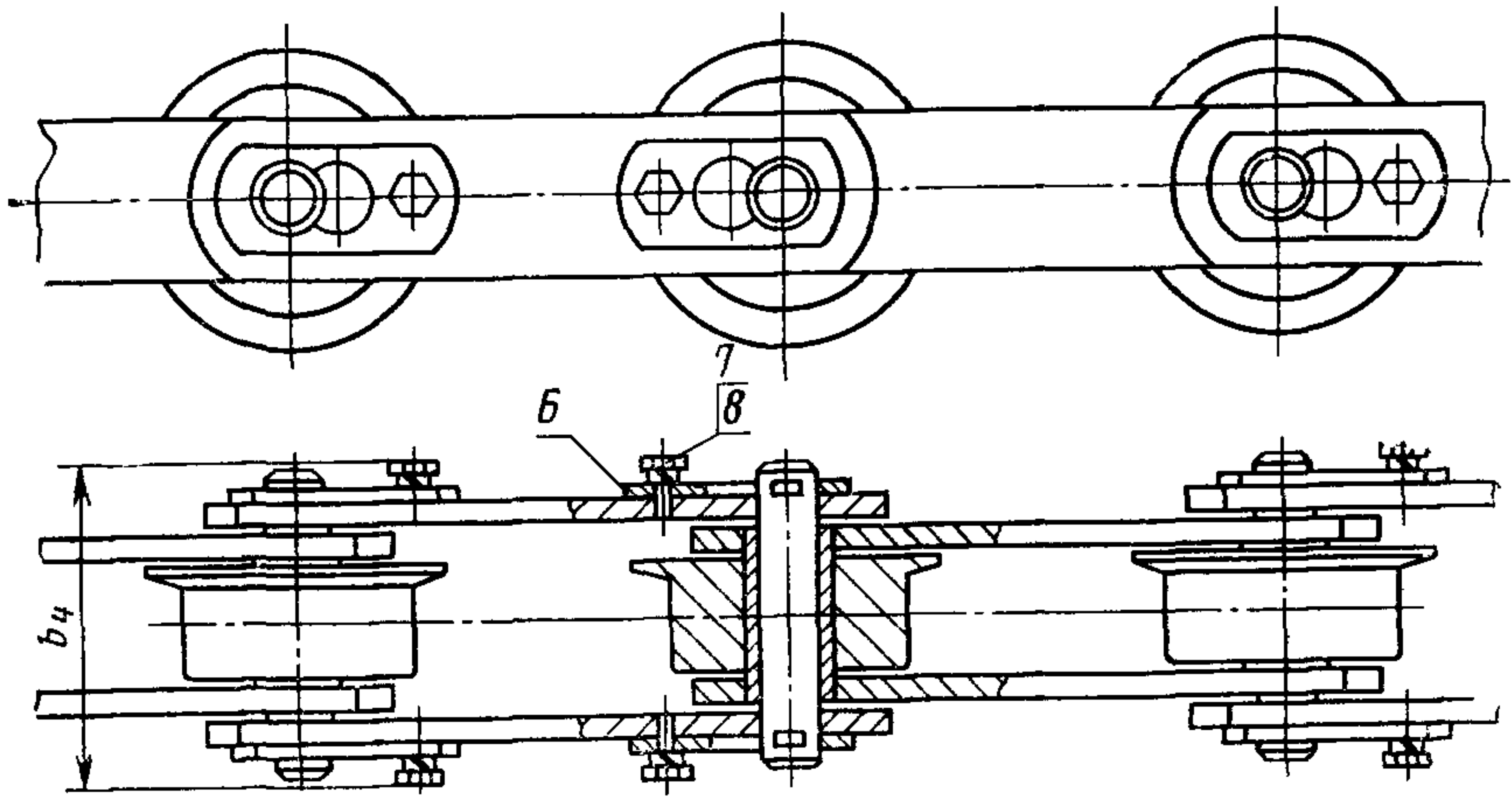
Исполнение 2
