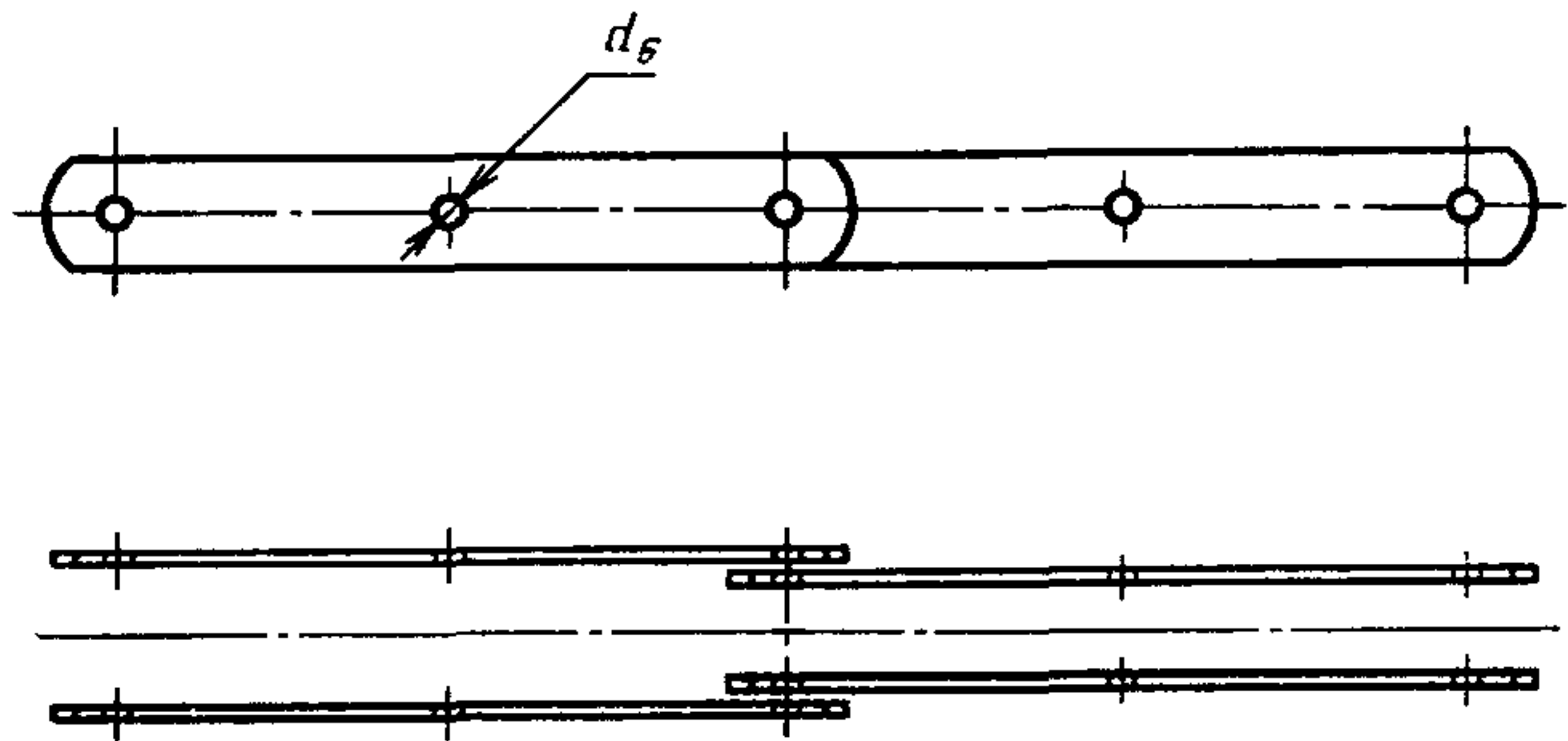
Черт. 5 Тип 2.1
