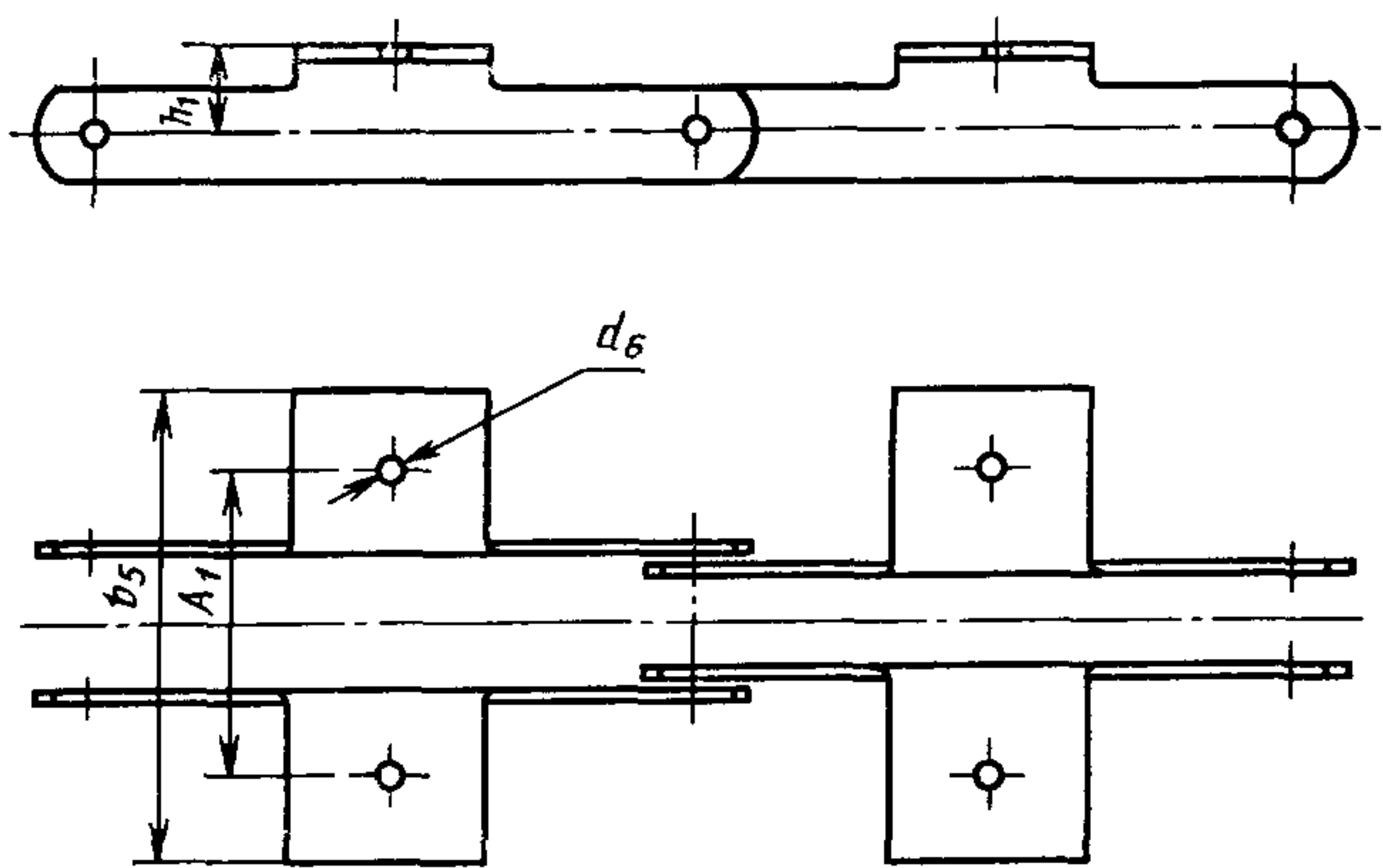
Тип 1.1
