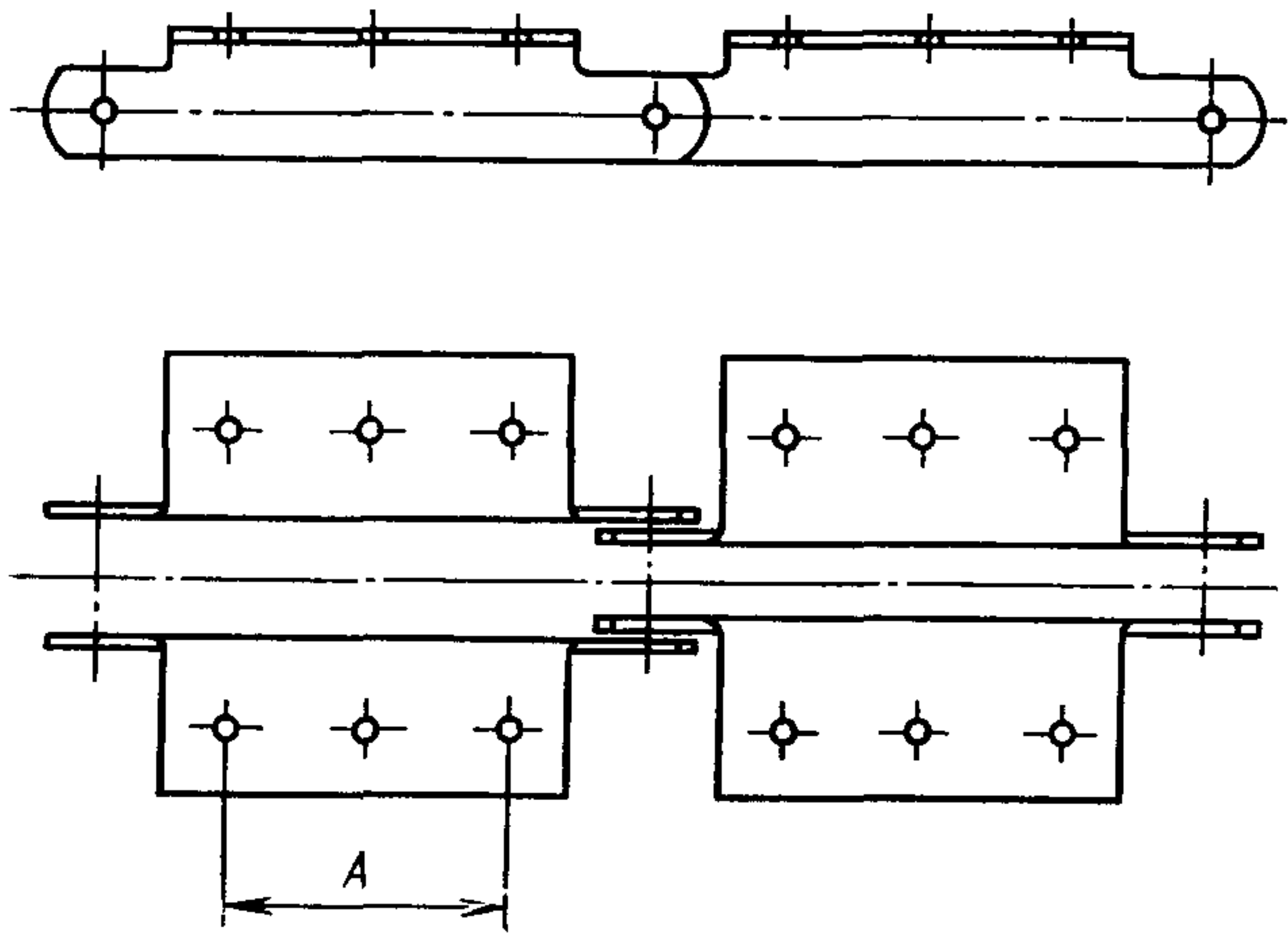
Черт. 5 Тип 2.1
