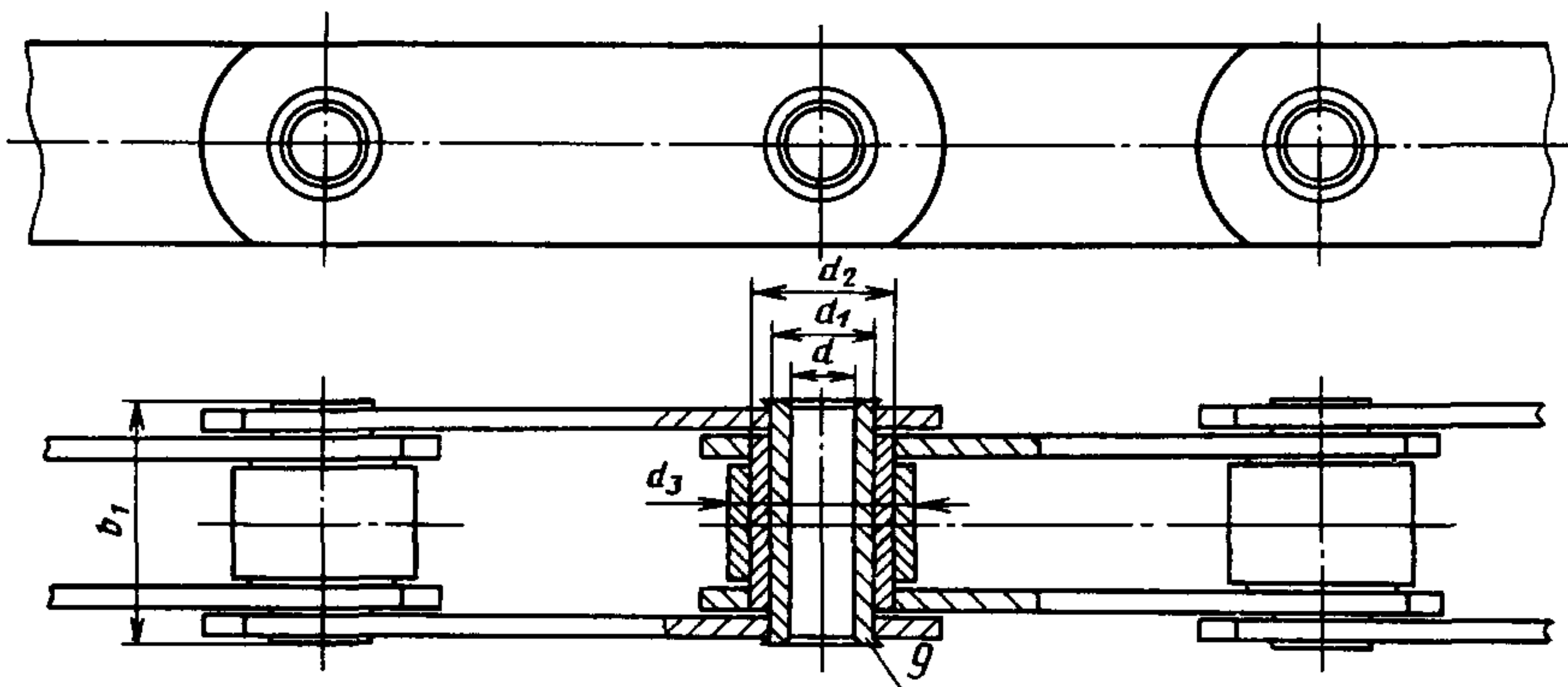
Исполнение 3
