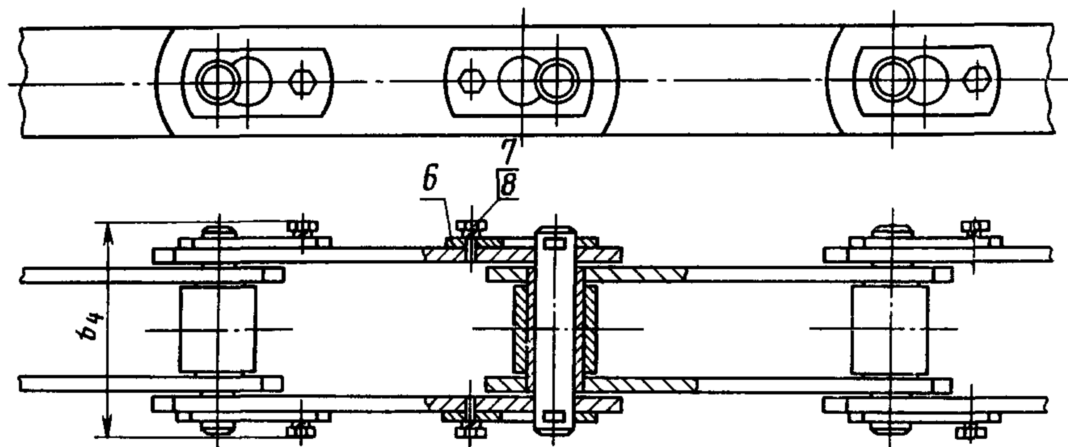
Исполнение 3
