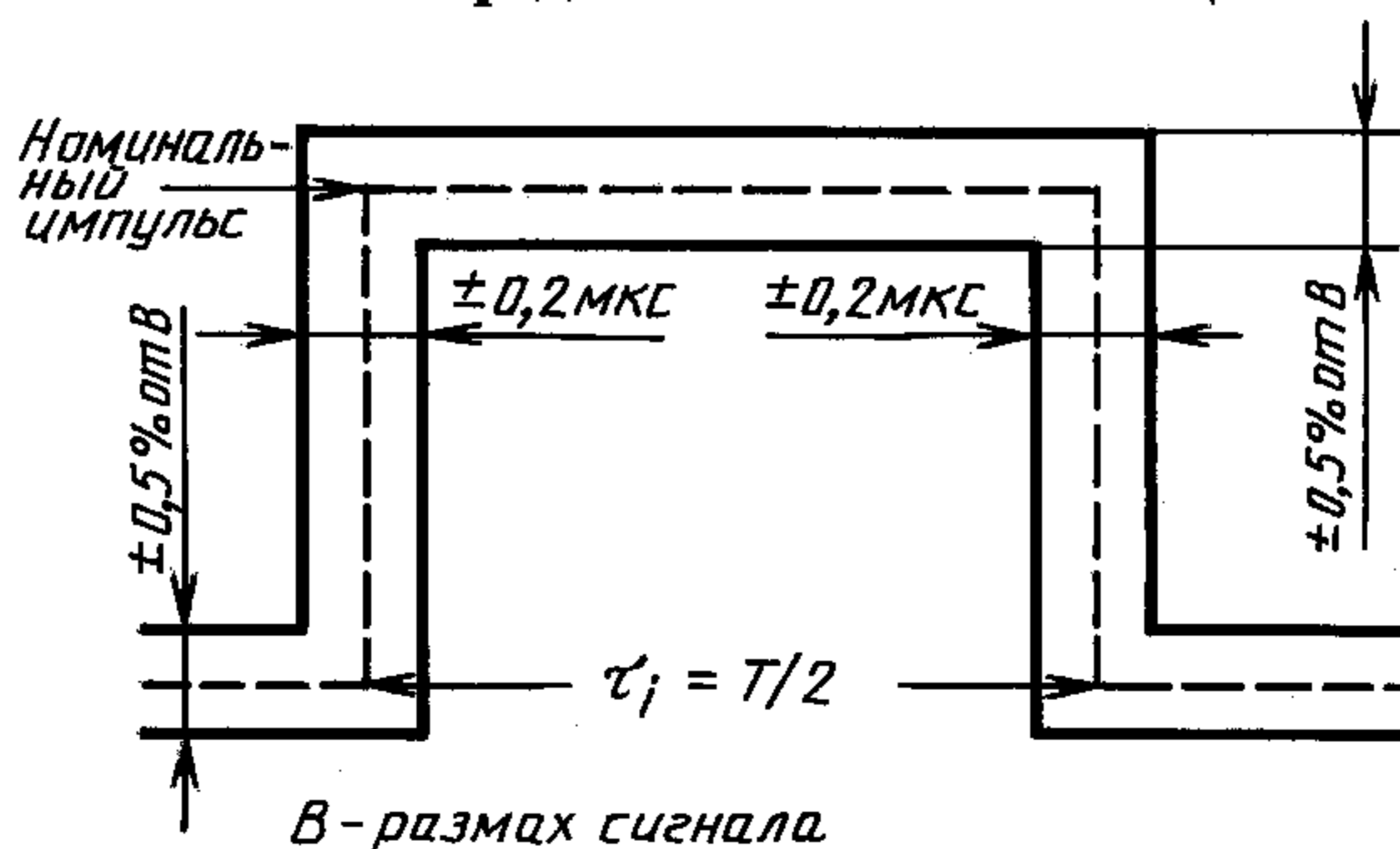
Маска передаваемого сигнала ОЦК
