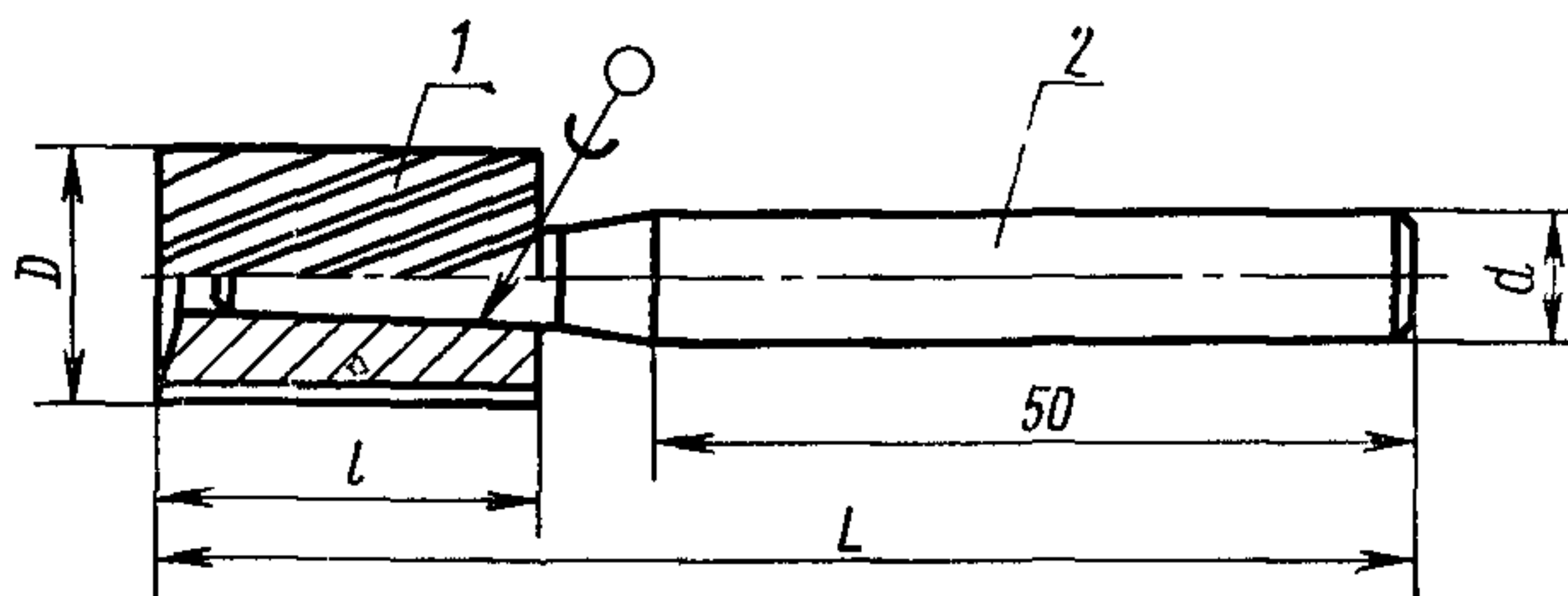
1—коронка, 2—оправка
