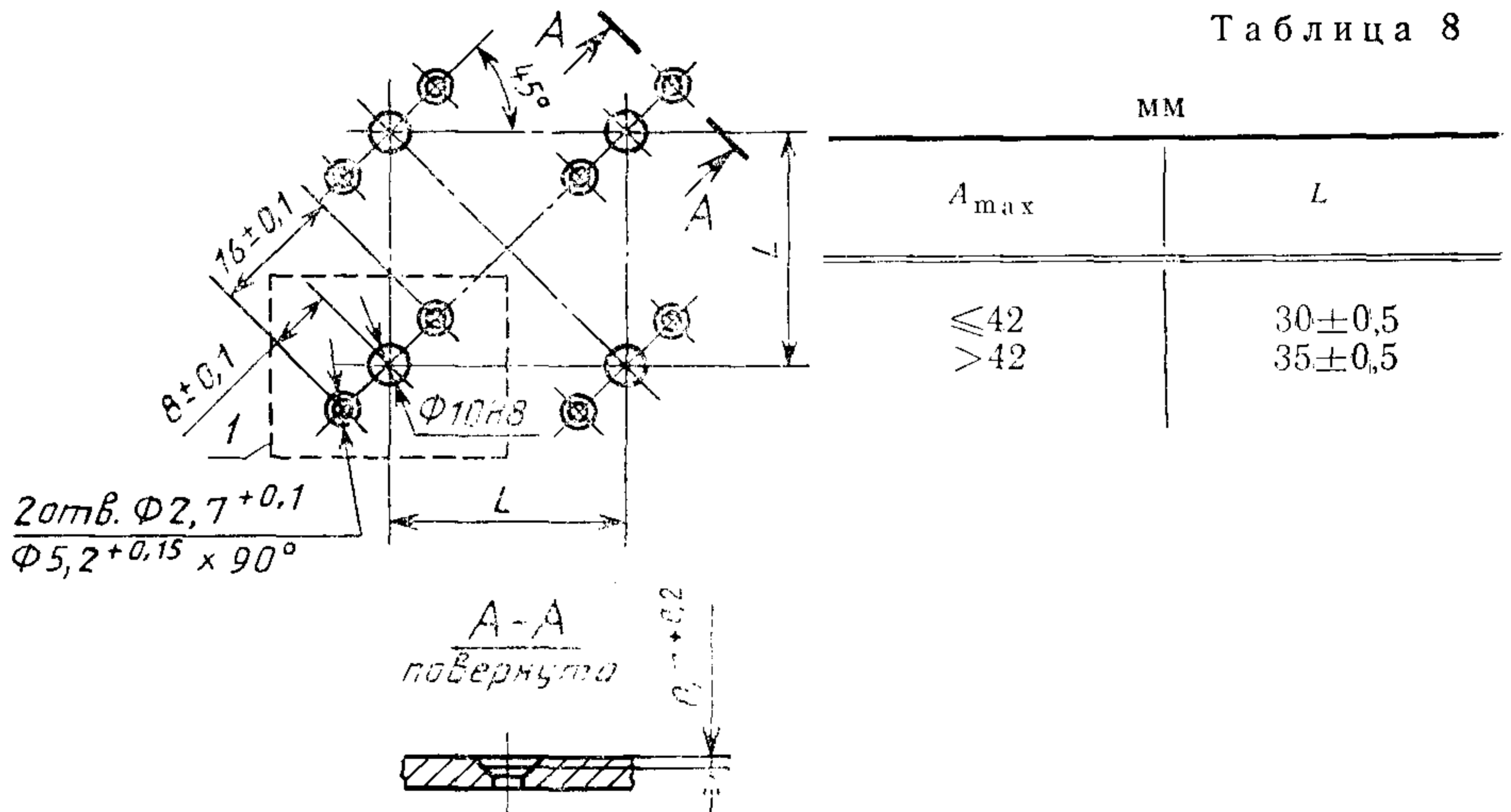
Разметка для крепления переключателей
