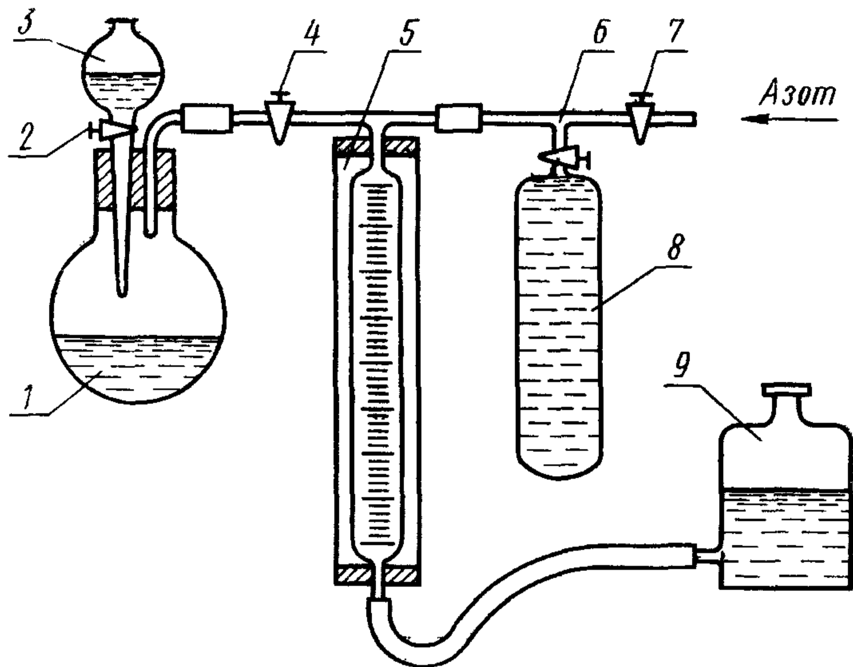
1—реакционная колба вместимостью 25—30 см 3 , 2, 4, 6, 7 — краны; 3—капельная воронка, 5—измерительная бюретка вместимостью 100 см 3 с водяной рубашкой, 8 — поглотительная склянка; 9 — уравнильный сосуд
