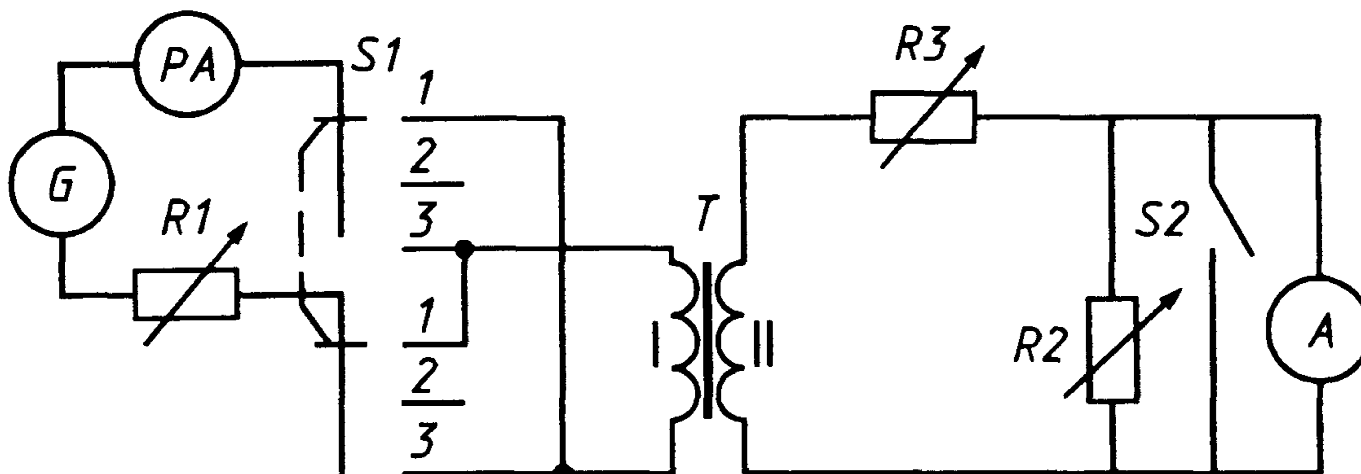
Рисунок 1 — Схема для измерений в разомкнутой магнитной цепи
