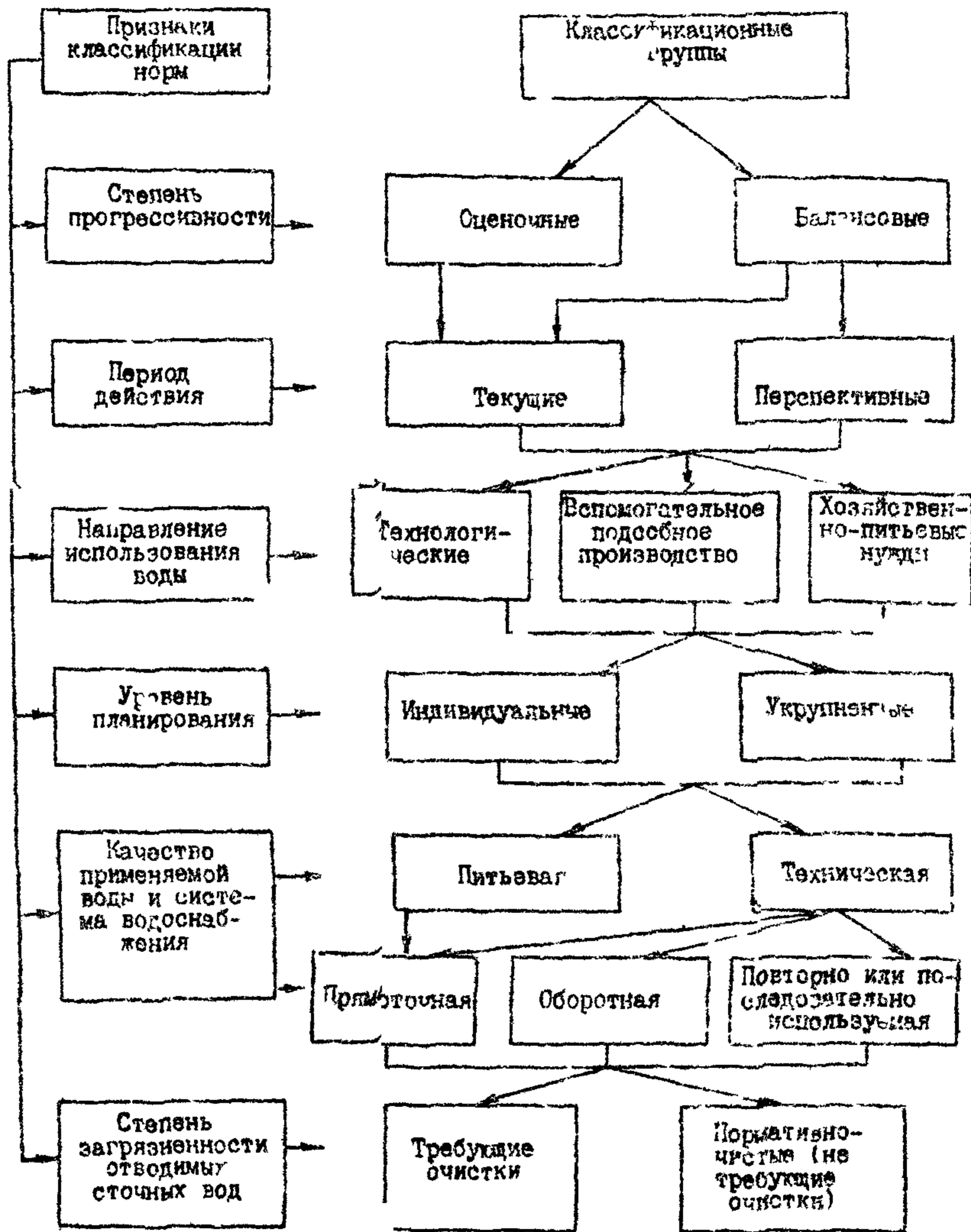
Рис. I. Классификация норм водопотребления и водосотведения на предприятиях теплоэнергетики
