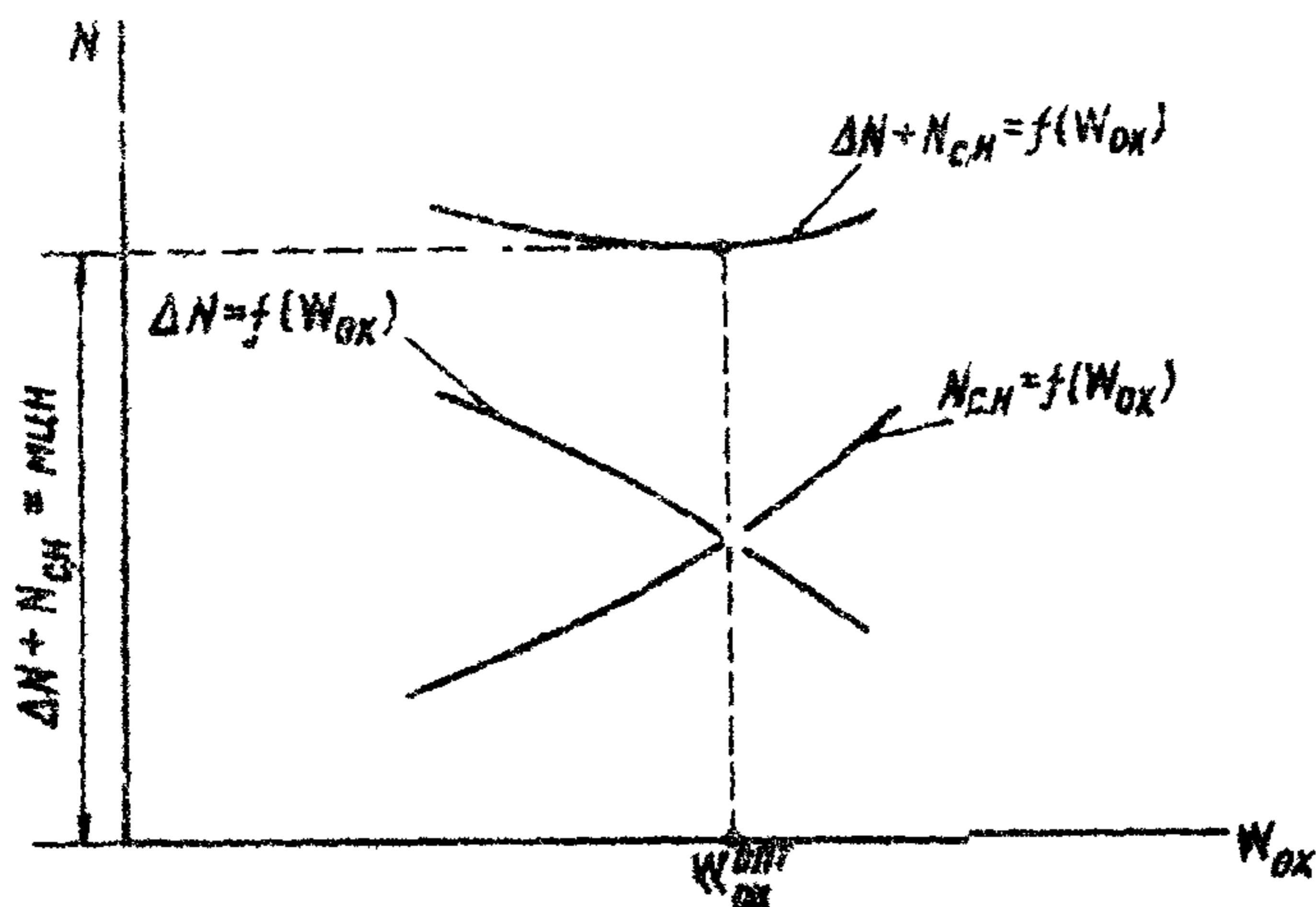
Рис.4. Определение оптимального расхода охлаждающей воды: \Delta N - недовыработка электроэнергии турбиной; N_{сн} - затраты электроэнергии на перекачку охлаждающей воды
