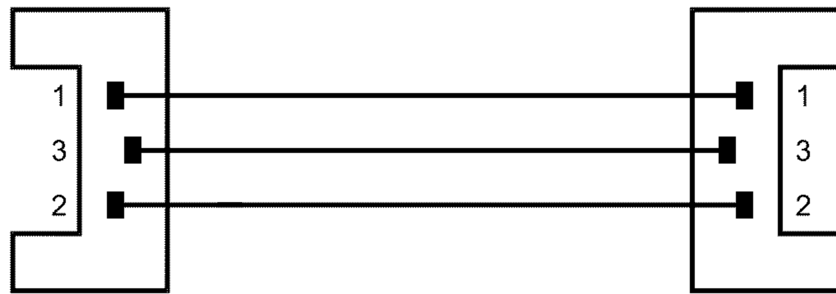
Рисунок Е.2 — Схема соединений кабеля шины
