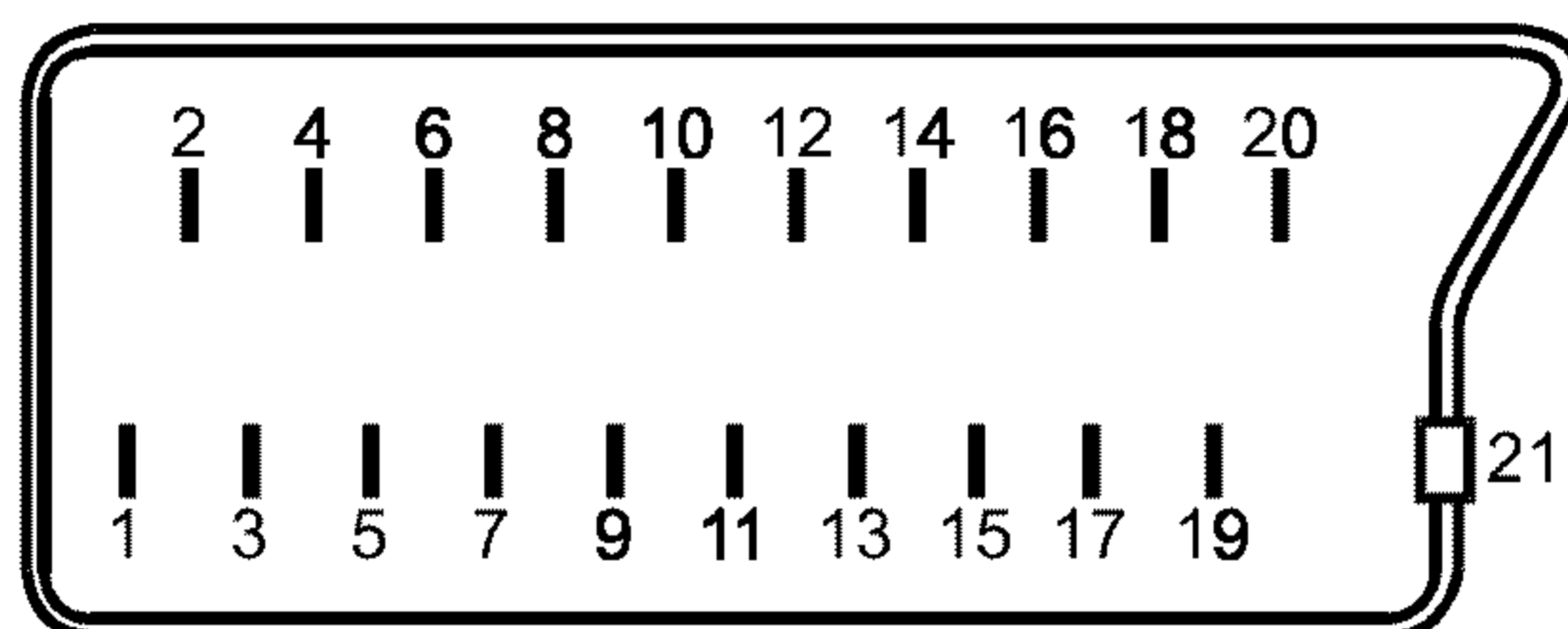
Рисунок В.1 — Расположение и нумерация контактов соединителя
