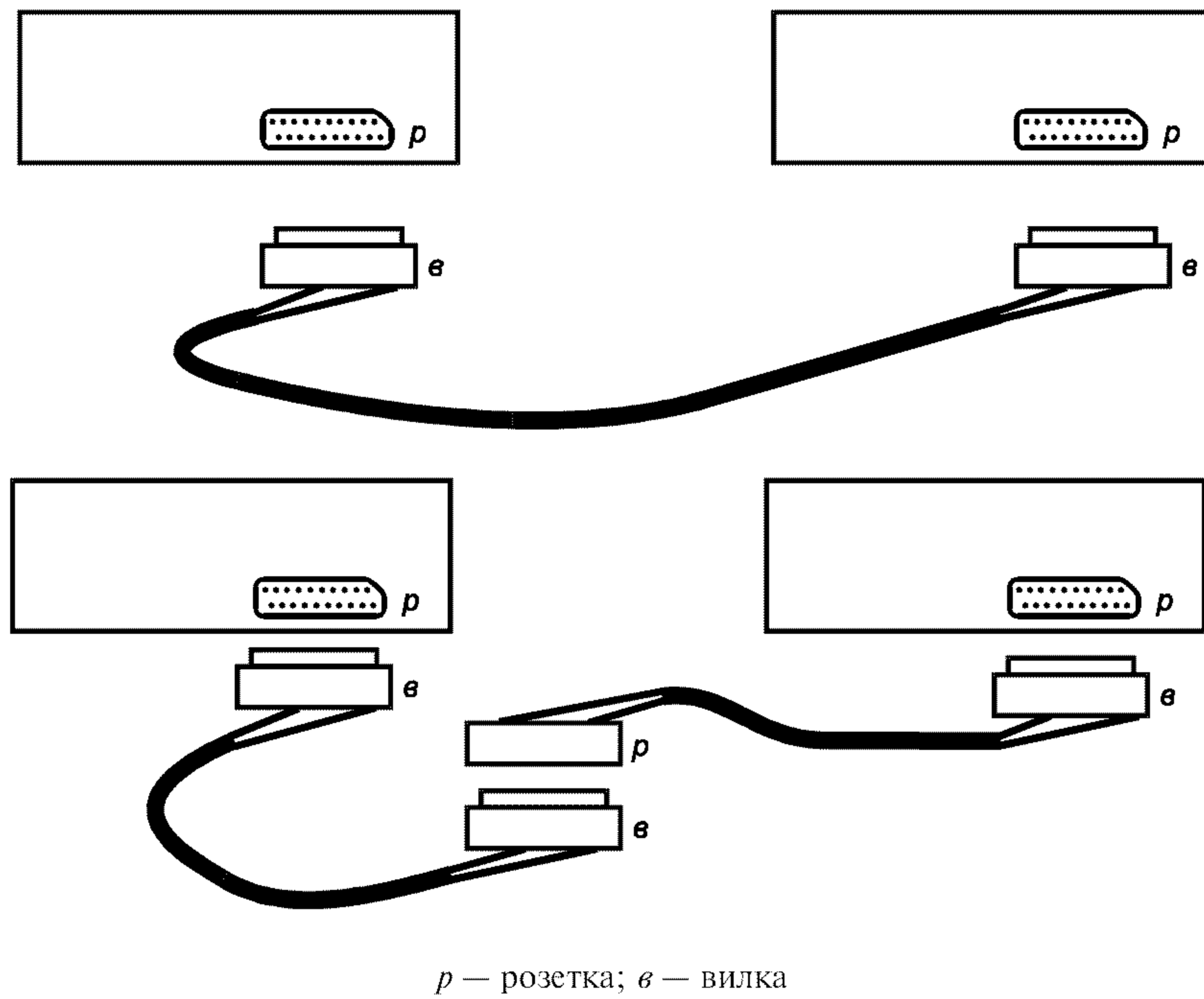
Рисунок Г.1 — Виды соединительных шнуров
