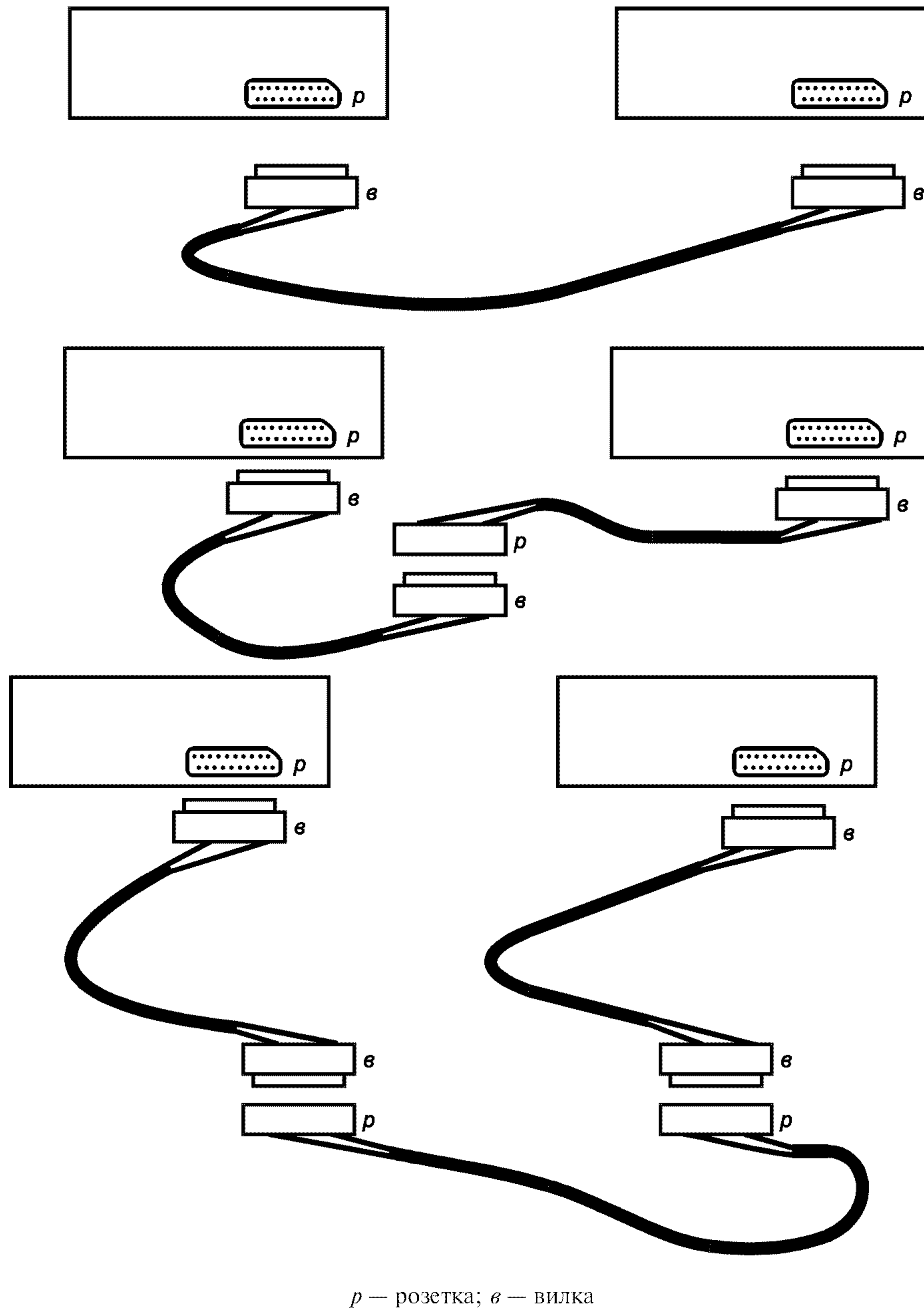
Рисунок В.2 — Виды соединительных шнуров
