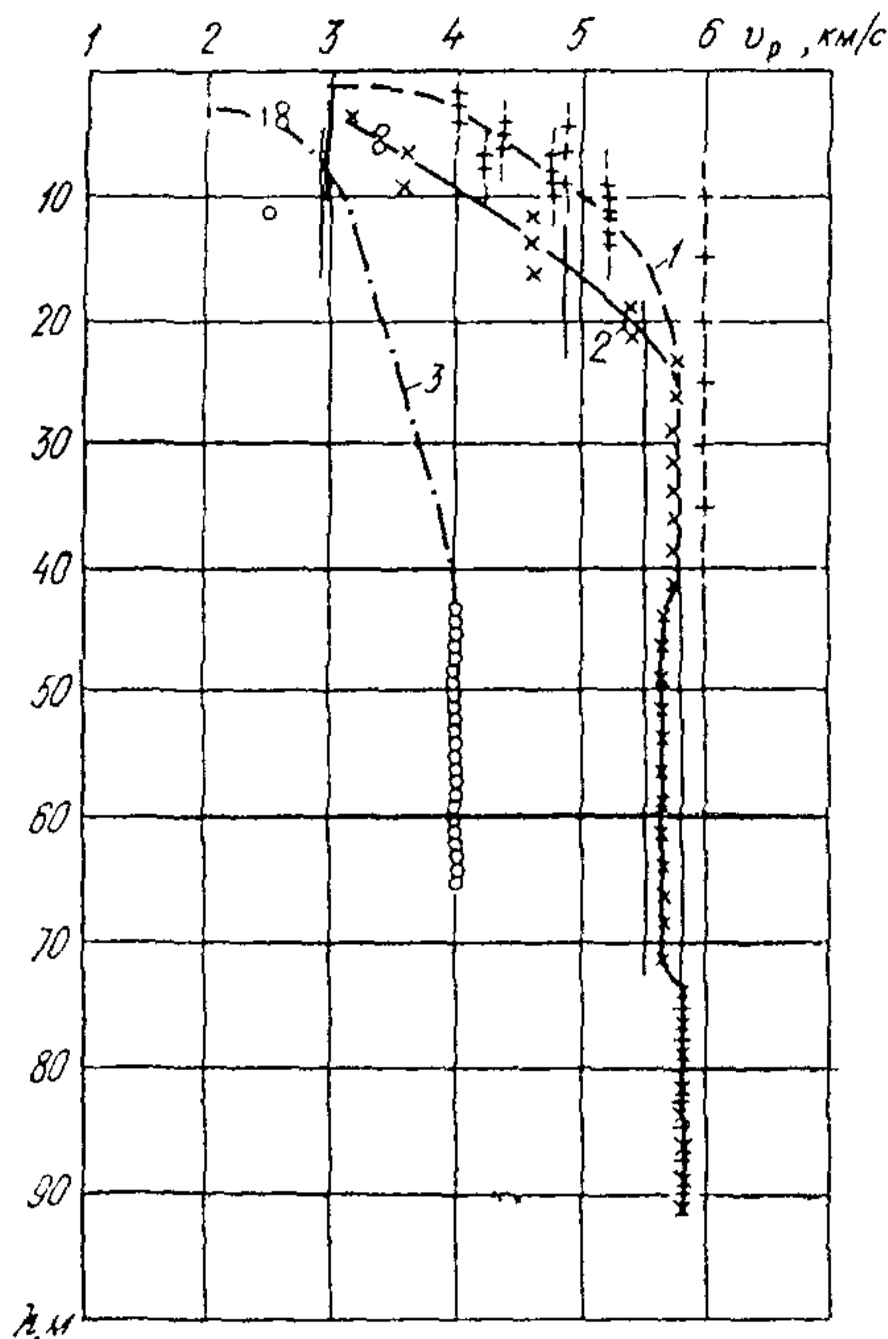
Рис. 4-1. Изменение скорости продольных волн v_p с глубиной h в гранитоидном массиве основания Тельмамского гидроузла
