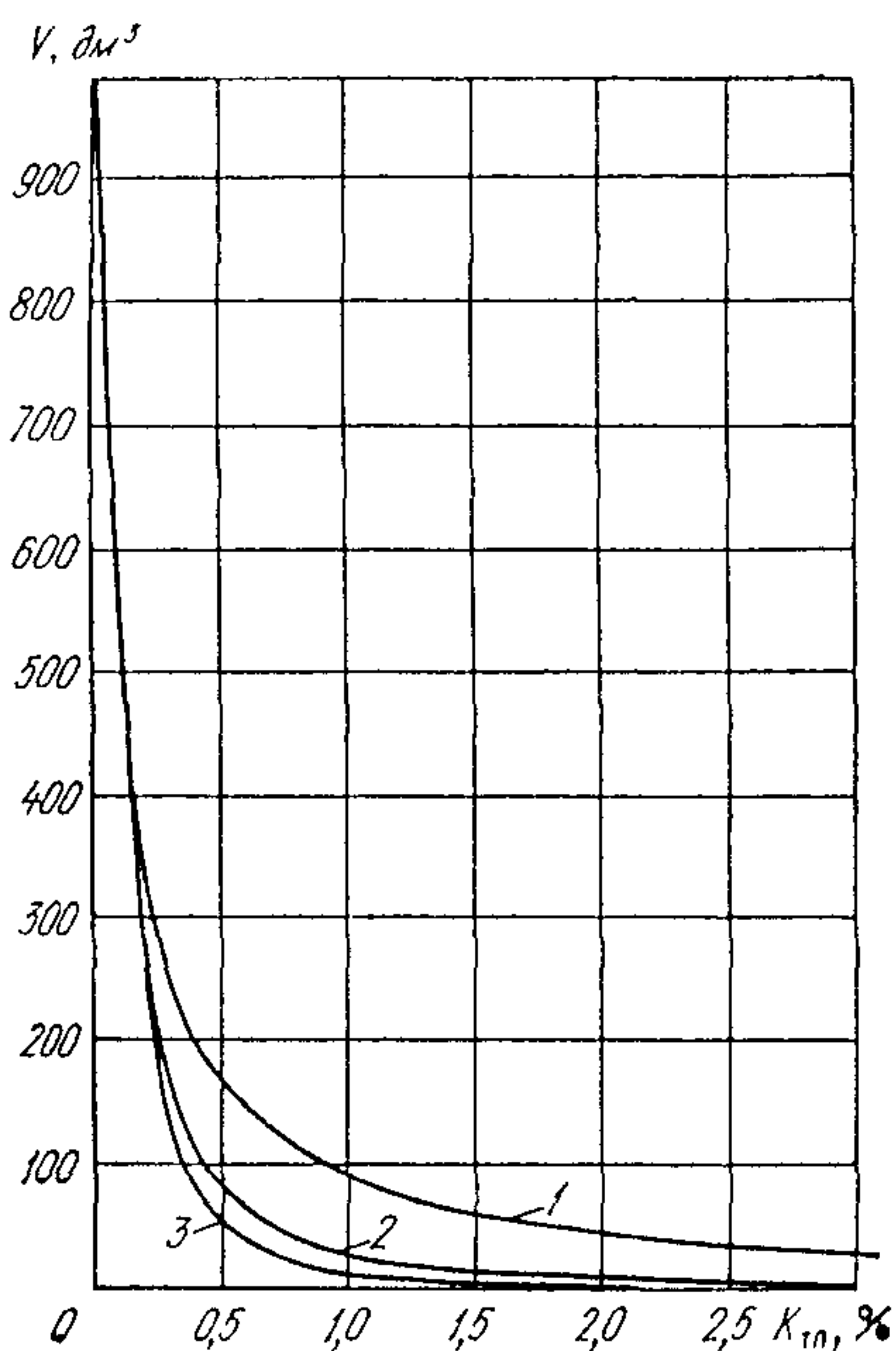
Рис. 4-3. Расчетная зависимость объема блоков горных пород V от коэффициента трещинной пущности K_{\text{ТП}}
