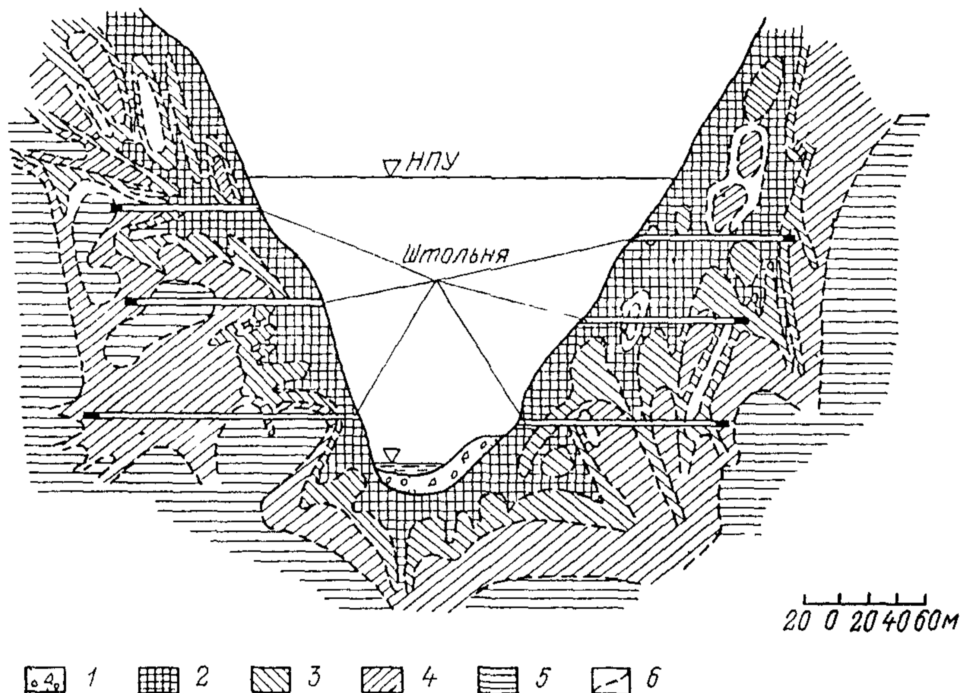
Рис 6 3 Сейсмогеологический разрез скального массива на участке плотины Токтогульской ГЭС
