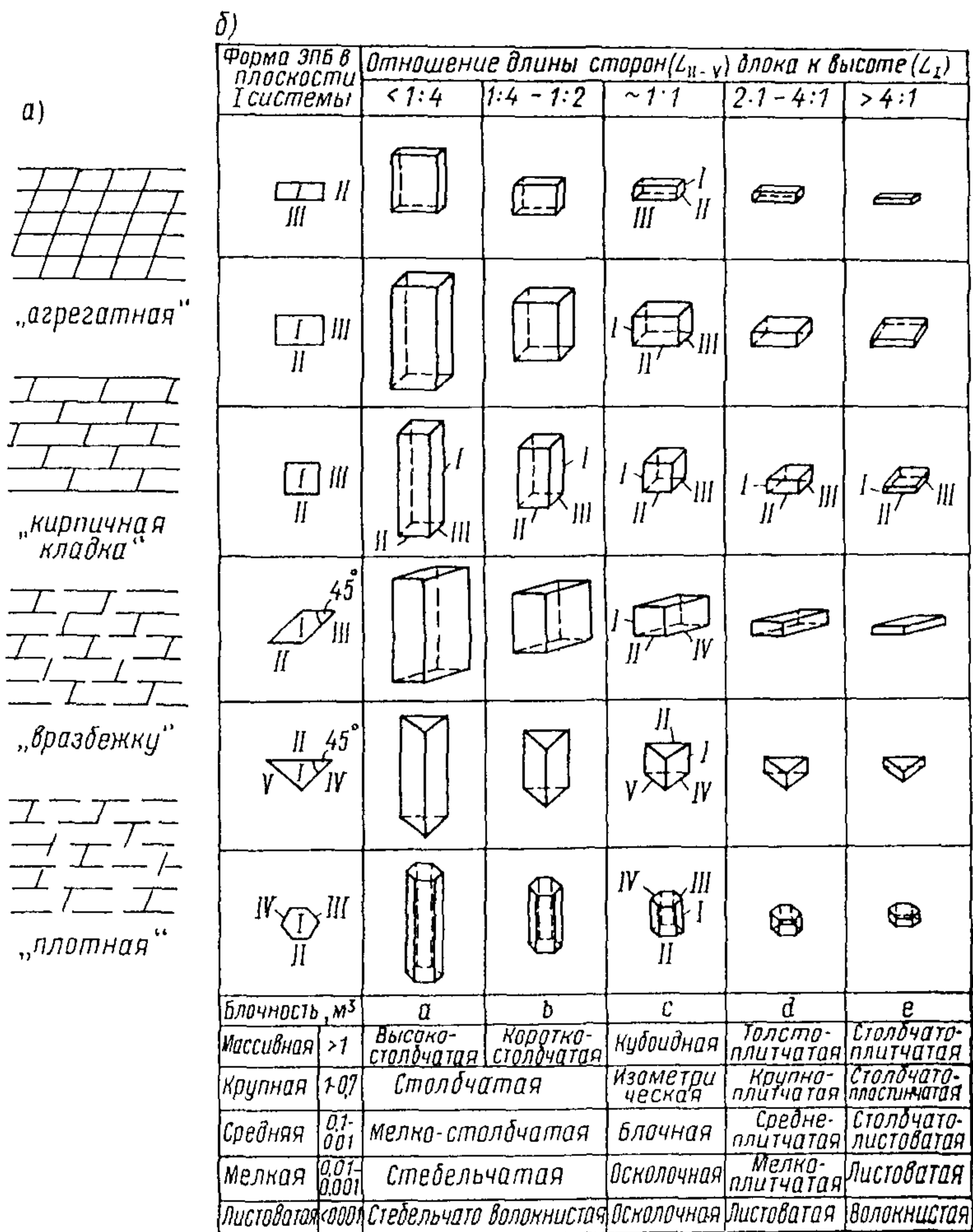
Рис. 3. Форма связи блоков в массиве (а) и классификация их форм (б) (по Л. Мюллеру [42] с дополнениями).
