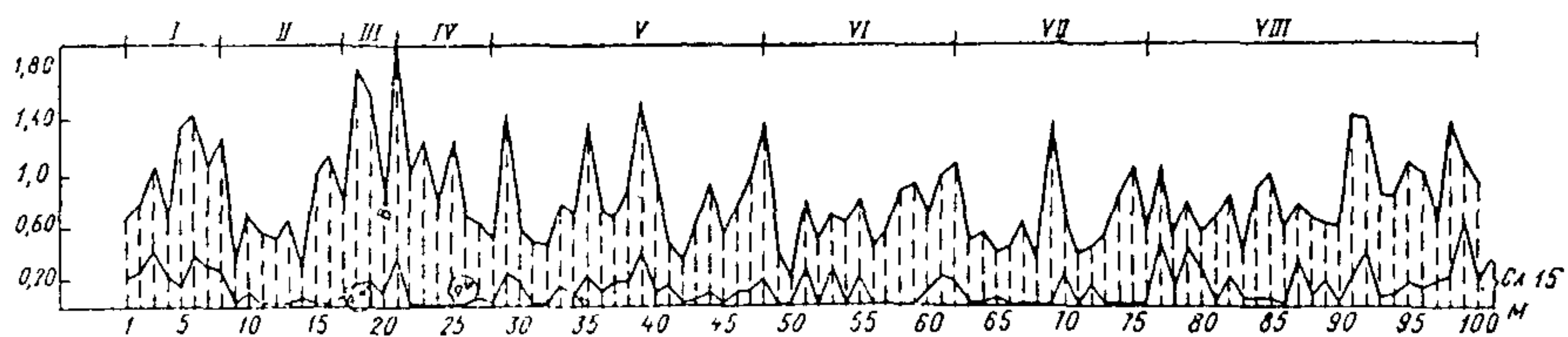
Рис. 3-1. Коннексиа разреза известняков на участке арочной плотины Кассеб А, В, 8а, 9а — маркирующие горизонты; I—VIII — номера пачек.
