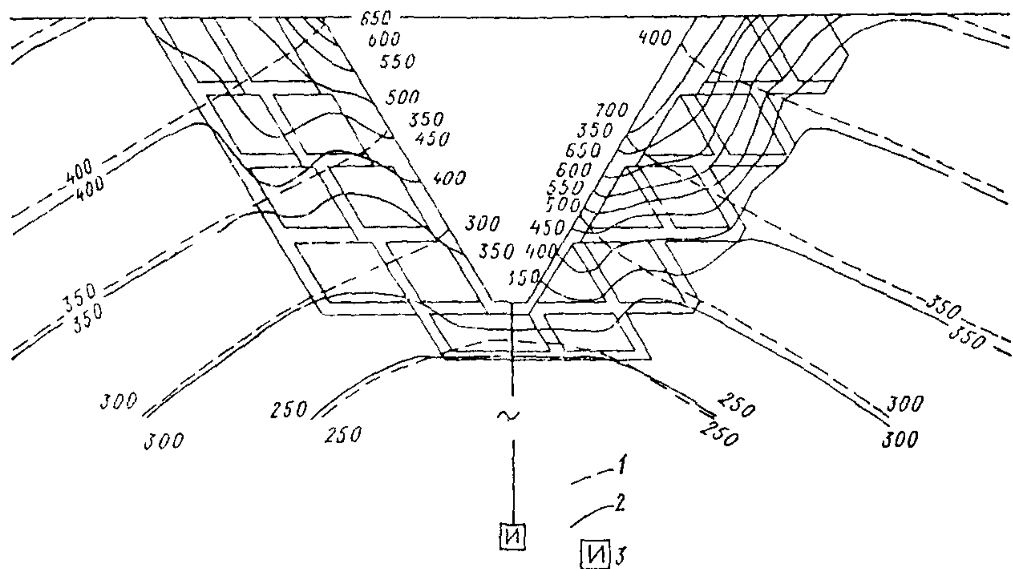
Рис 6.5 Исследование волновой картины в скальных основаниях при землетрясениях. Поле изохрон в модели каньона с зонально-блочным строением бортов и положением эпицентра в каньоне
