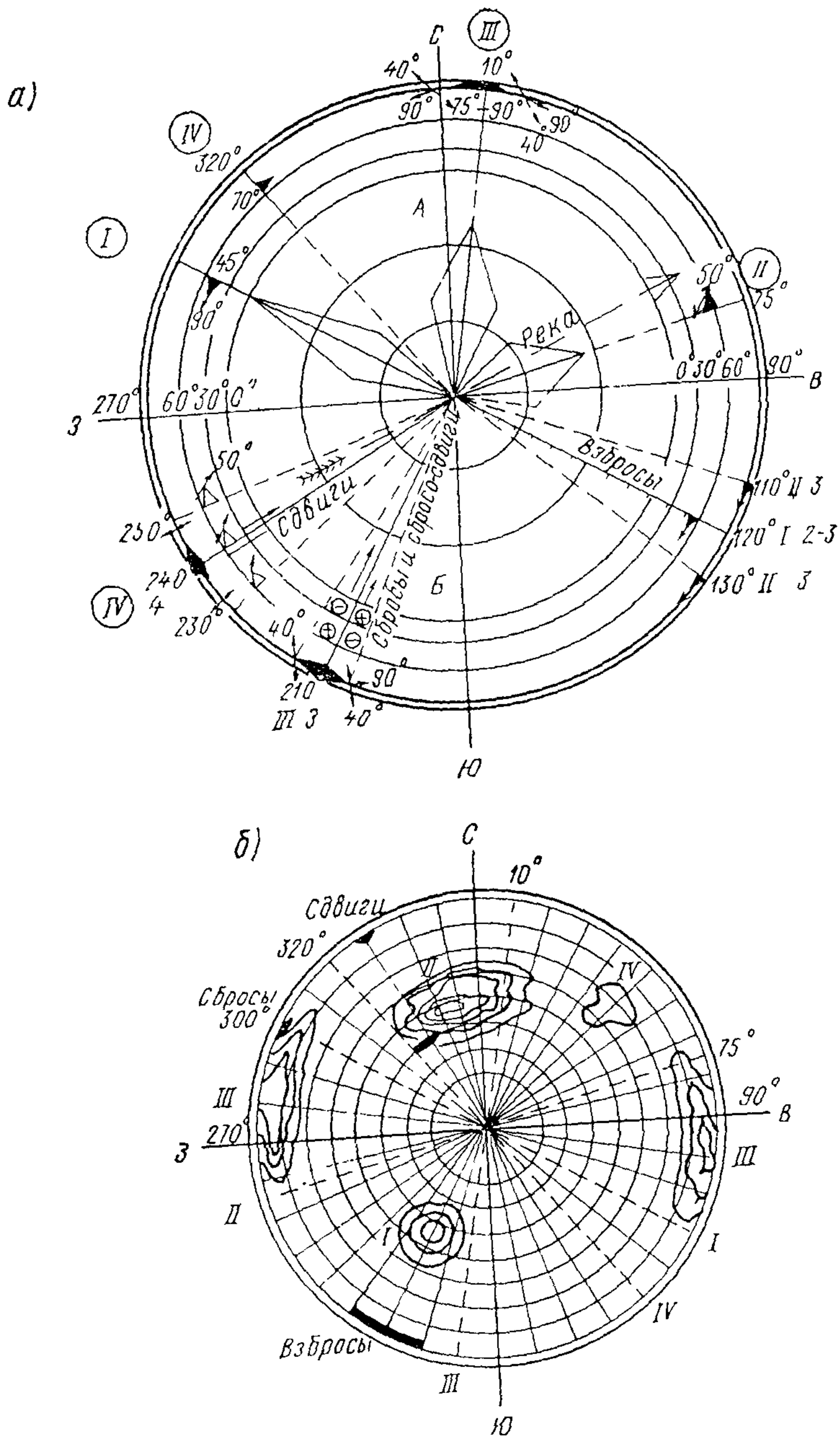
Рис. 3-7. Диаграммы ориентации трещин и тектонических разрывных смещений в массиве основания Стрыйского гидроузла а — круговая роза: А — трещин; Б — тектонических разрывных смещений (по А. М. Гурееву); б — круговая точечная (проекция равнопромежуточная — полюсная); I—IV — основные системы тектонических нарушений.
