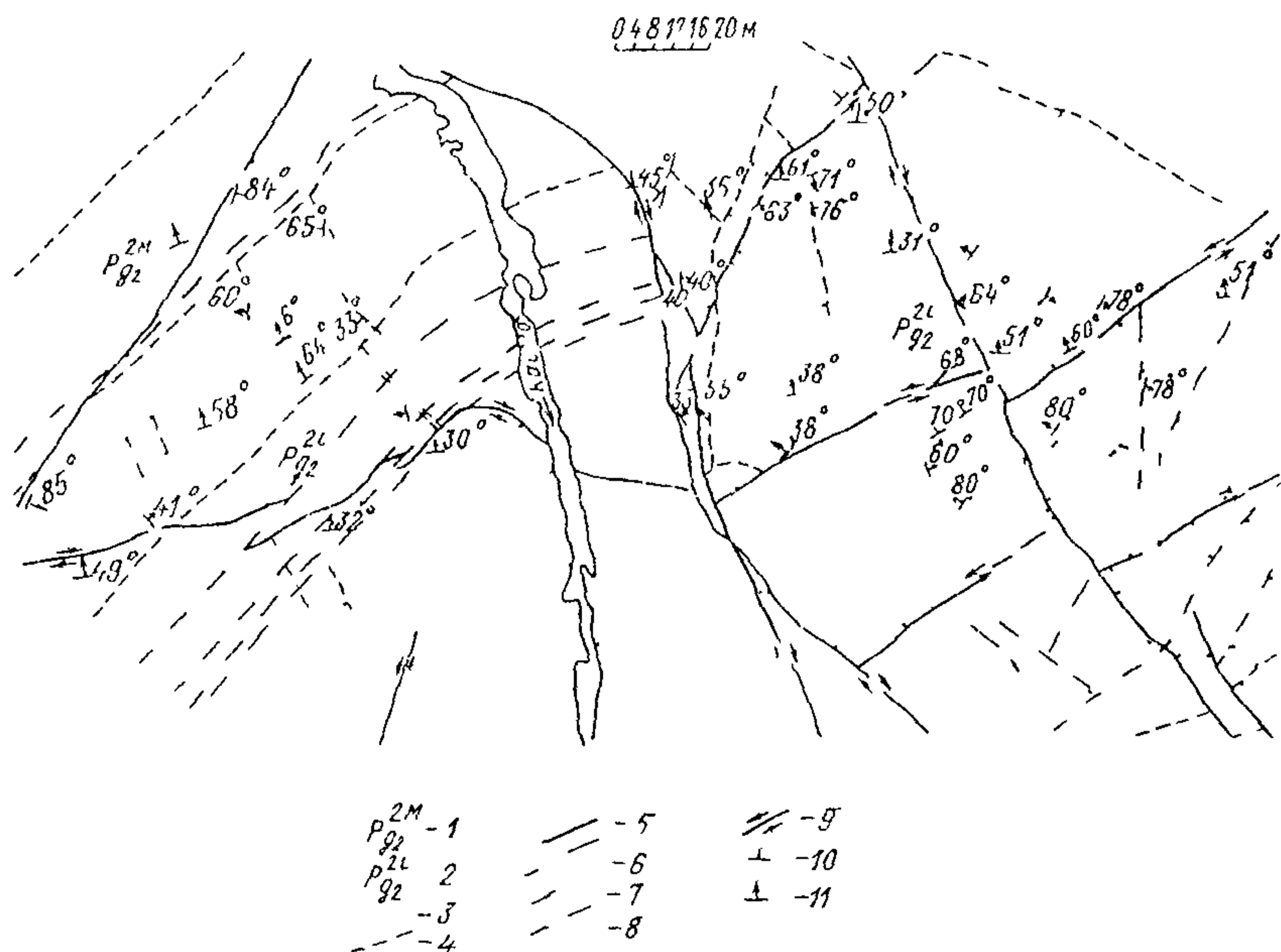
Рис 5.4 Структурная схема участка основания арочной плотины Кассеб
