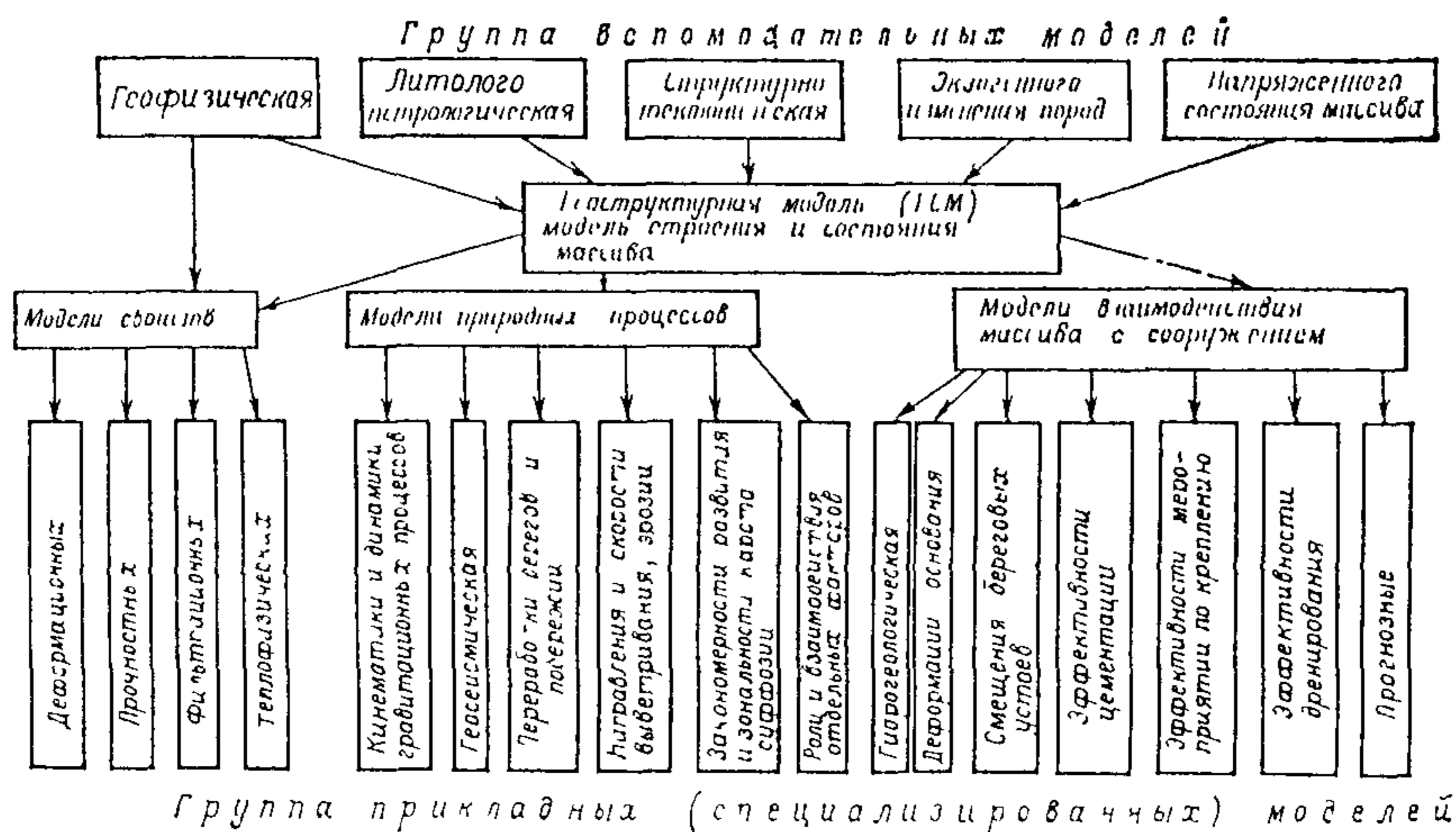
Рис. 1 Принципиальная схема инженерно-геологической модели основания гидротехнического сооружения.
