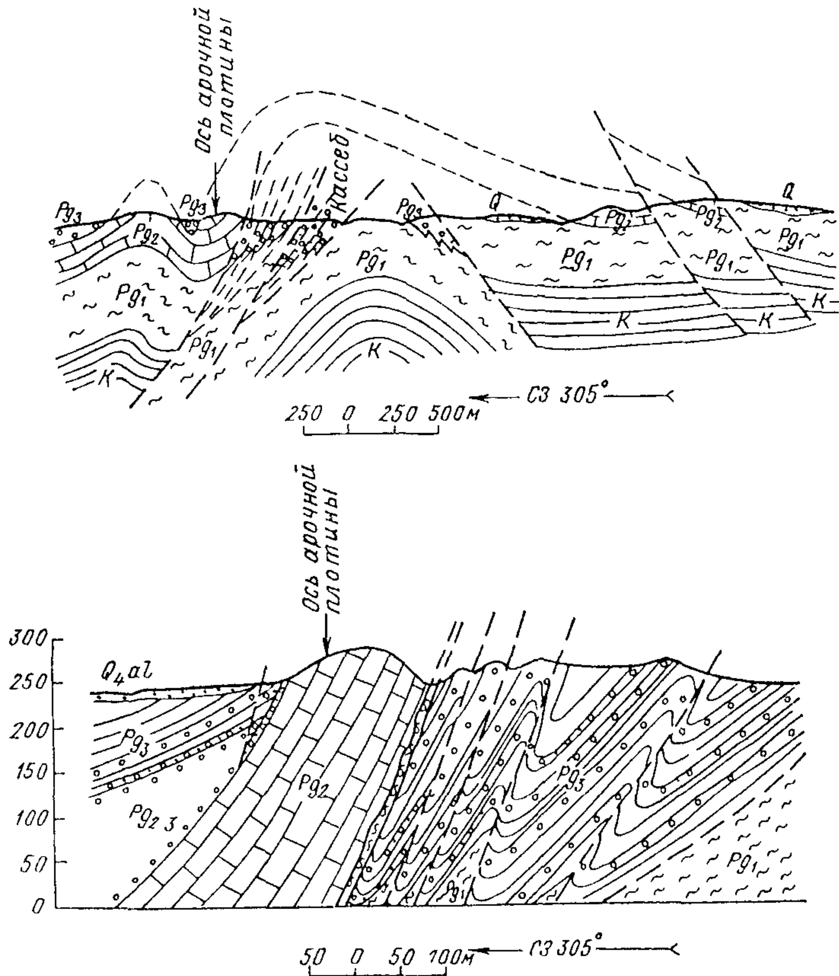
Рис 5.2 Схематический геологический разрез вдоль долины Уэд-Кассеб
