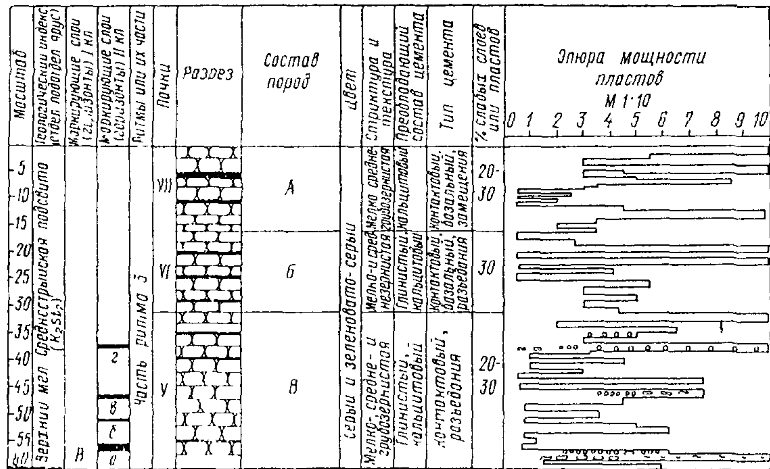
Рис. 4-2. Фрагмент сводного литолого-стратиграфического разреза основания плотны на р. Стрый
