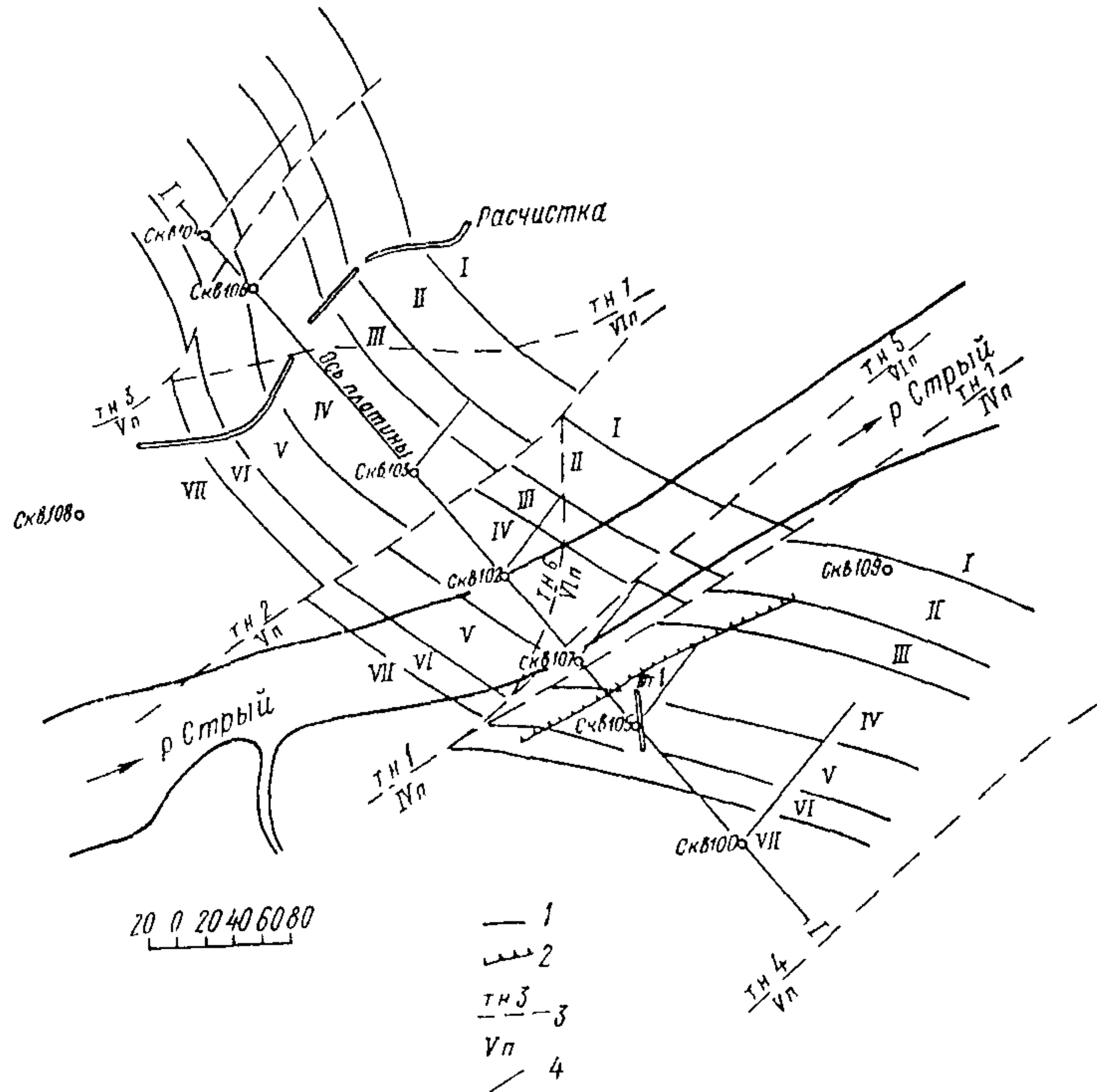
Рис 5-8. Структурно-литологическая карта участка створа «Ровин»
