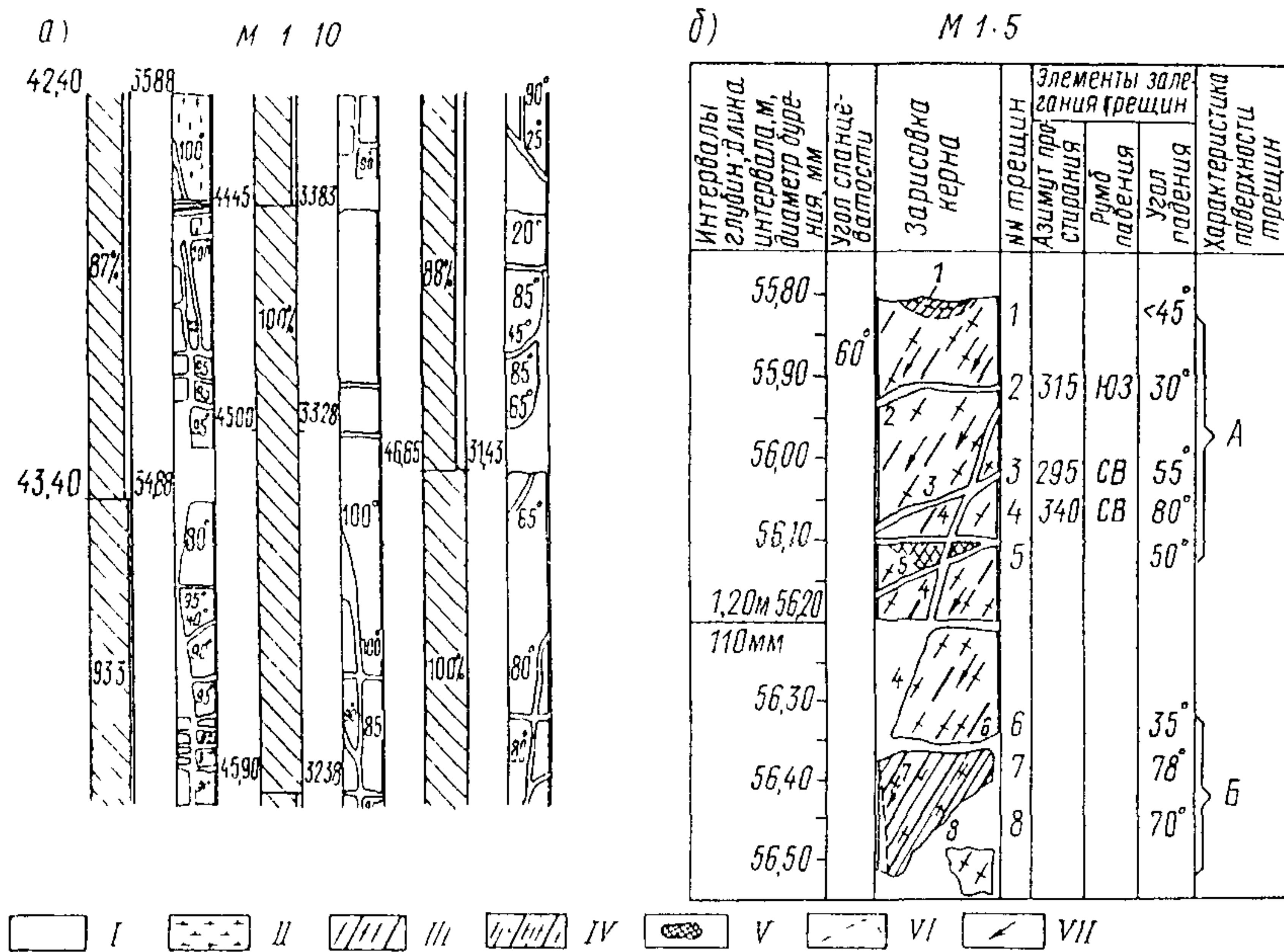
Рис 3-4 Типы зарисовок трещин в ядре буровых скважин
