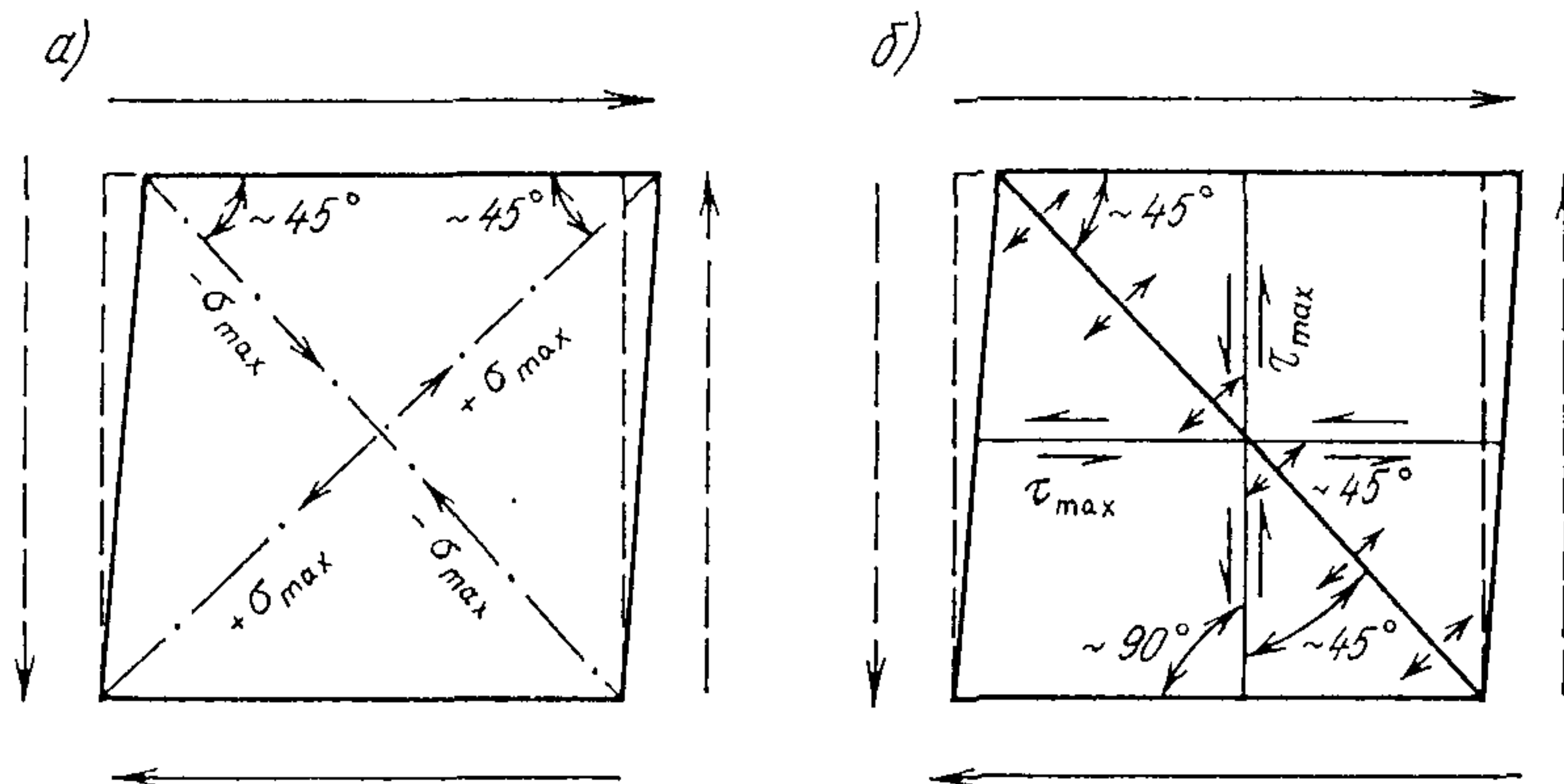
Рис 1-2. Образование трещин при сдвиге (схема напряжений)
