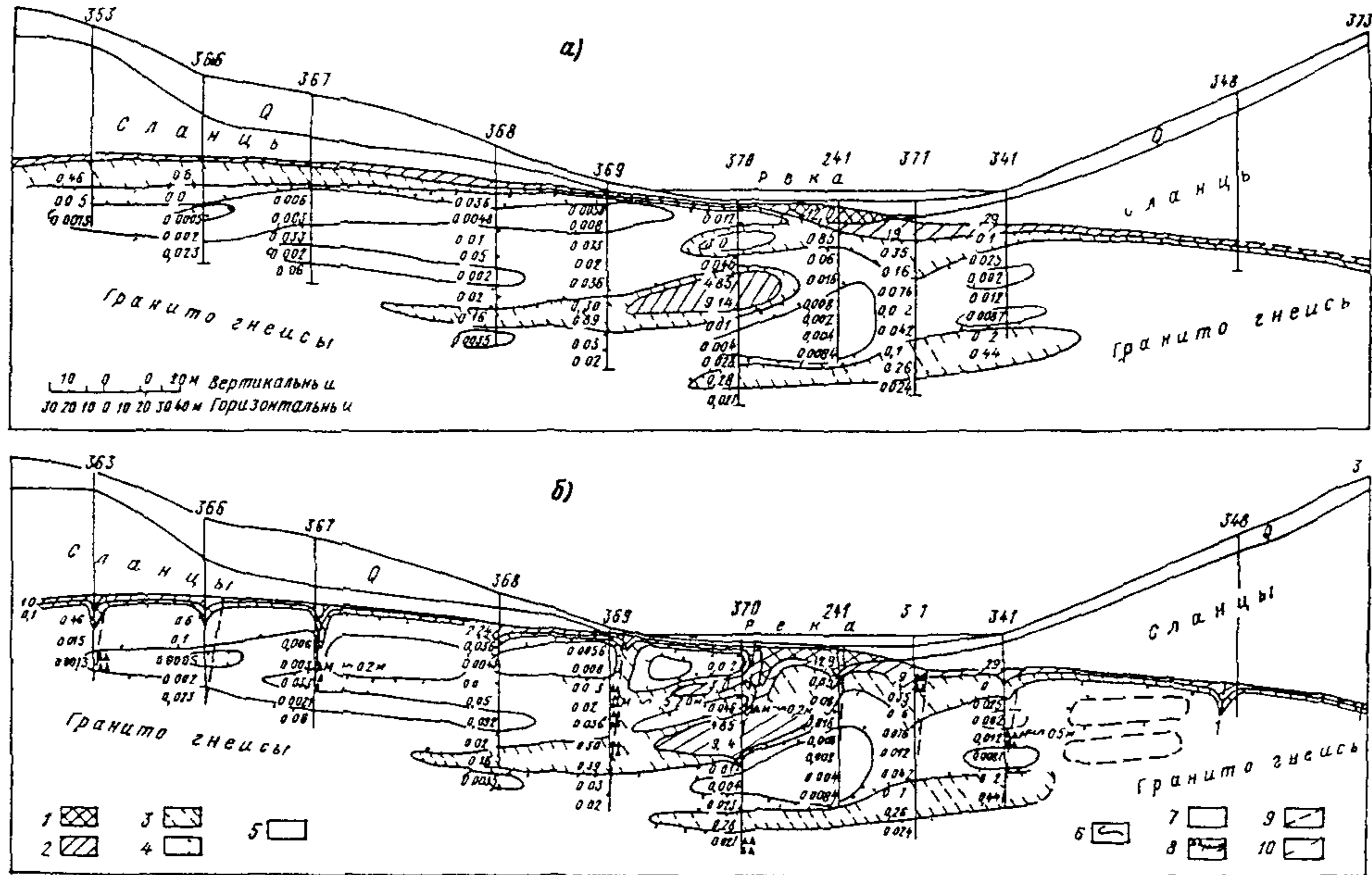
Рис 4 13 Этапы «формализованной» (а) и «геоструктурной» (б) интерпретаций данных удельных водопоглощений q , л/мин 1 — более 10 2 — 1—10 3 — 1—0,1 4 — 0,1—0,01, 5 — 0,01—0,001 6 — изолинии водопроницаемости, 7 — то же предполагаемые 8 — дробленый керна на интервалах длиной м 9 — мелкие сбросы V—VI порядков 10 — то же предполагаемые
