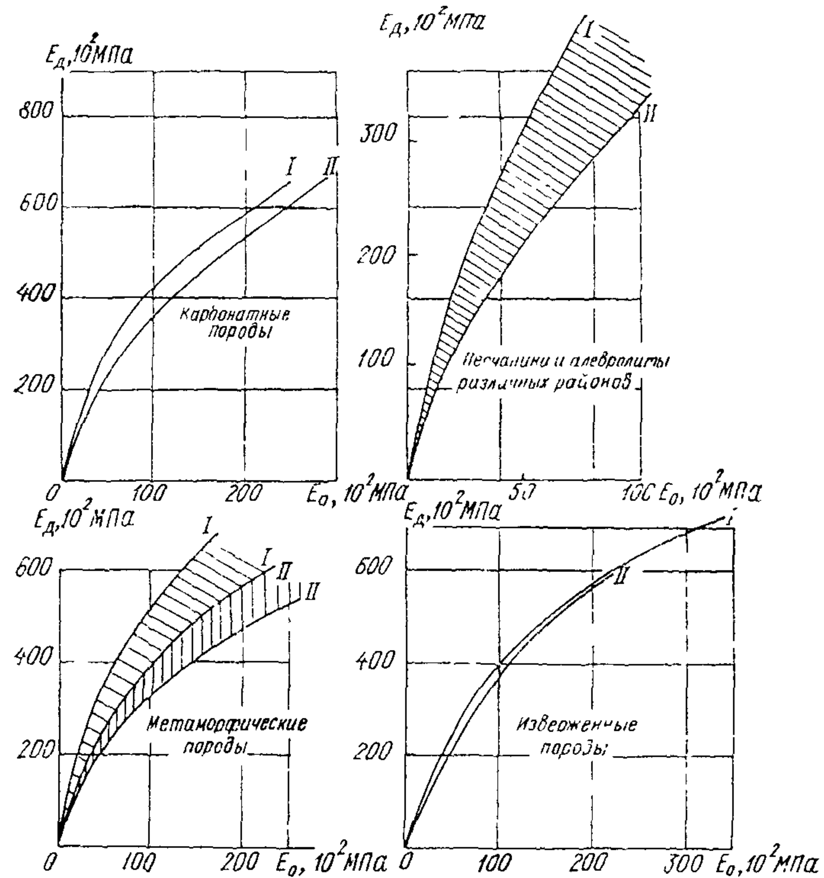
Рис. 4-8. Осредняющие взаимосвязей E_d(E_0) (и области наиболее вероятных значений) для различных скальных пород, рекомендуемые А. И. Савичем I, II — значения E_0 , определенные соответственно по первому и по второму циклам нагружения.
