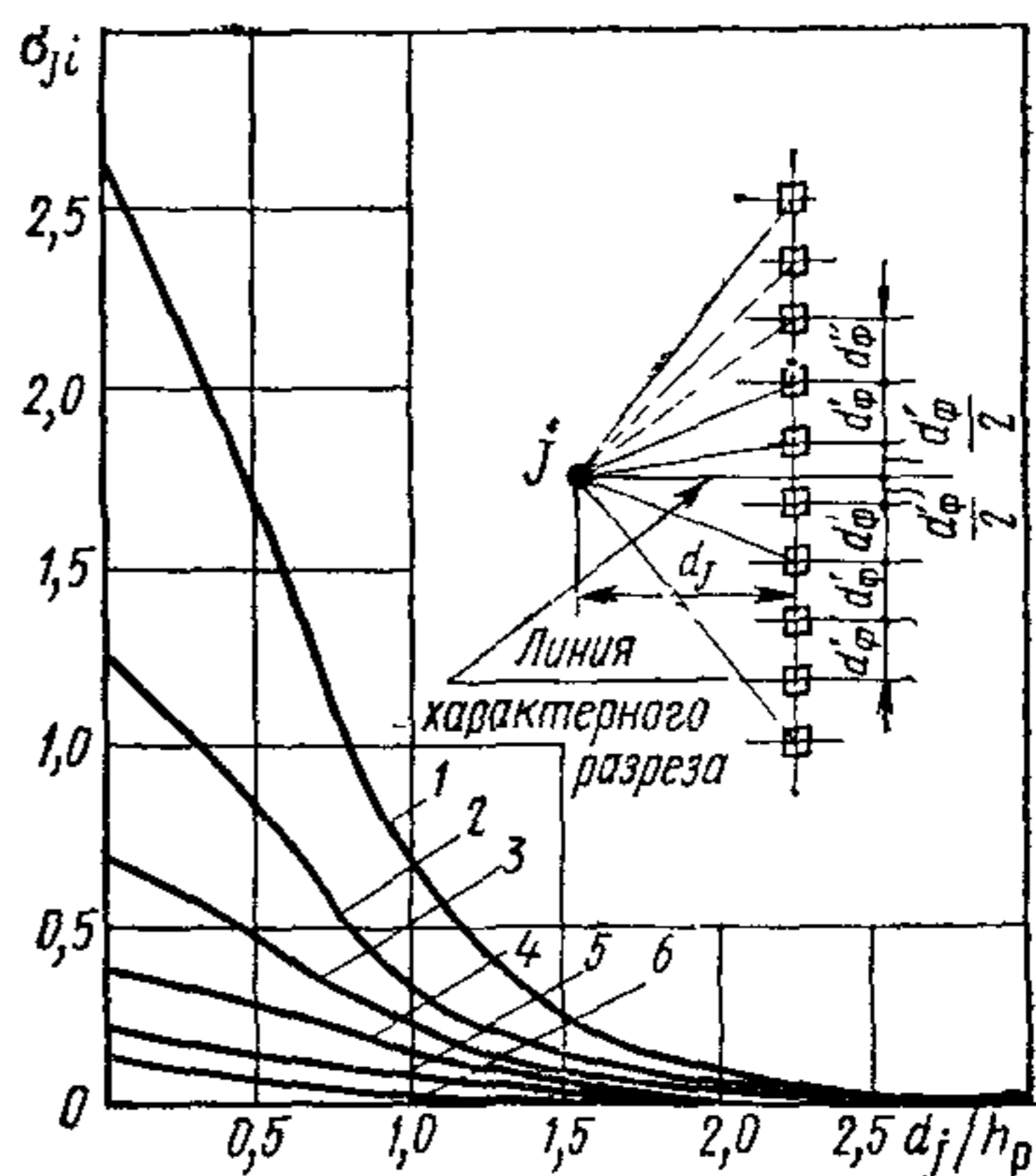
Рис. 14. Зависимость световой компоненты \sigma_{ij} ряда зенитных фонарей со световыми проемами, м: 1,5 \times 1,7 ; 1,5 \times 2,9 ; 1,5 \times 3,9 ; 1,5 \times 5,9 в точках характерного разреза между зенитными фонарями от d_j/h_p
