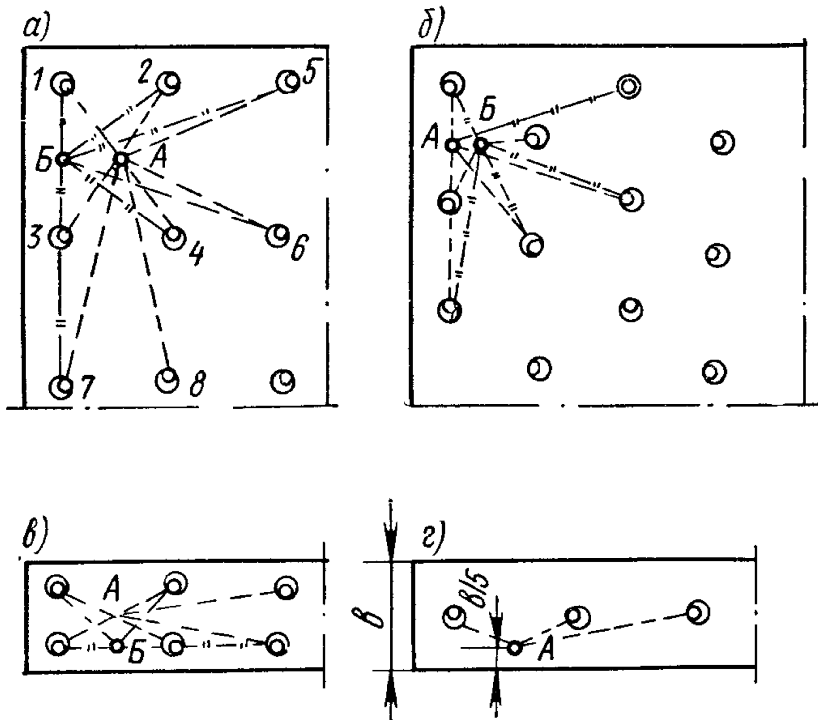
Рис. 75. Характерные расчетные точки для общего равномерного освещения
