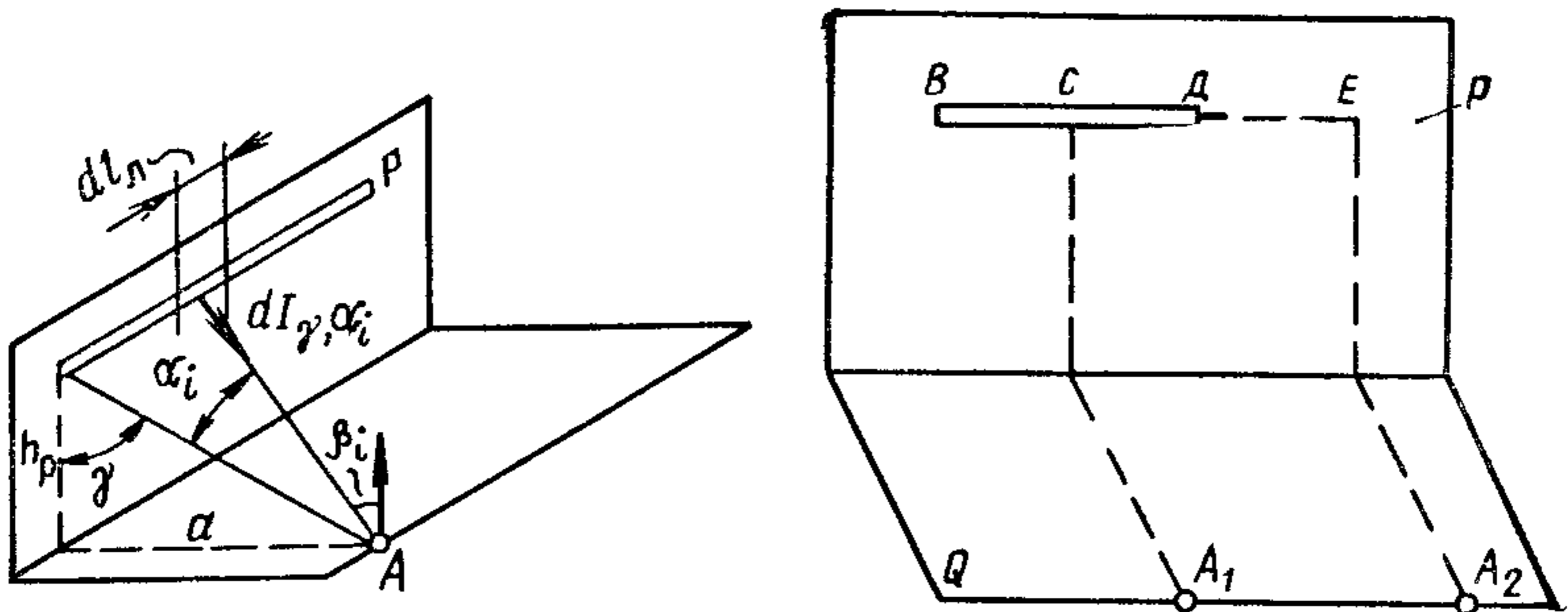
Рис. 81. Расположение прожектора относительно расчетной точки (к примеру 4)
