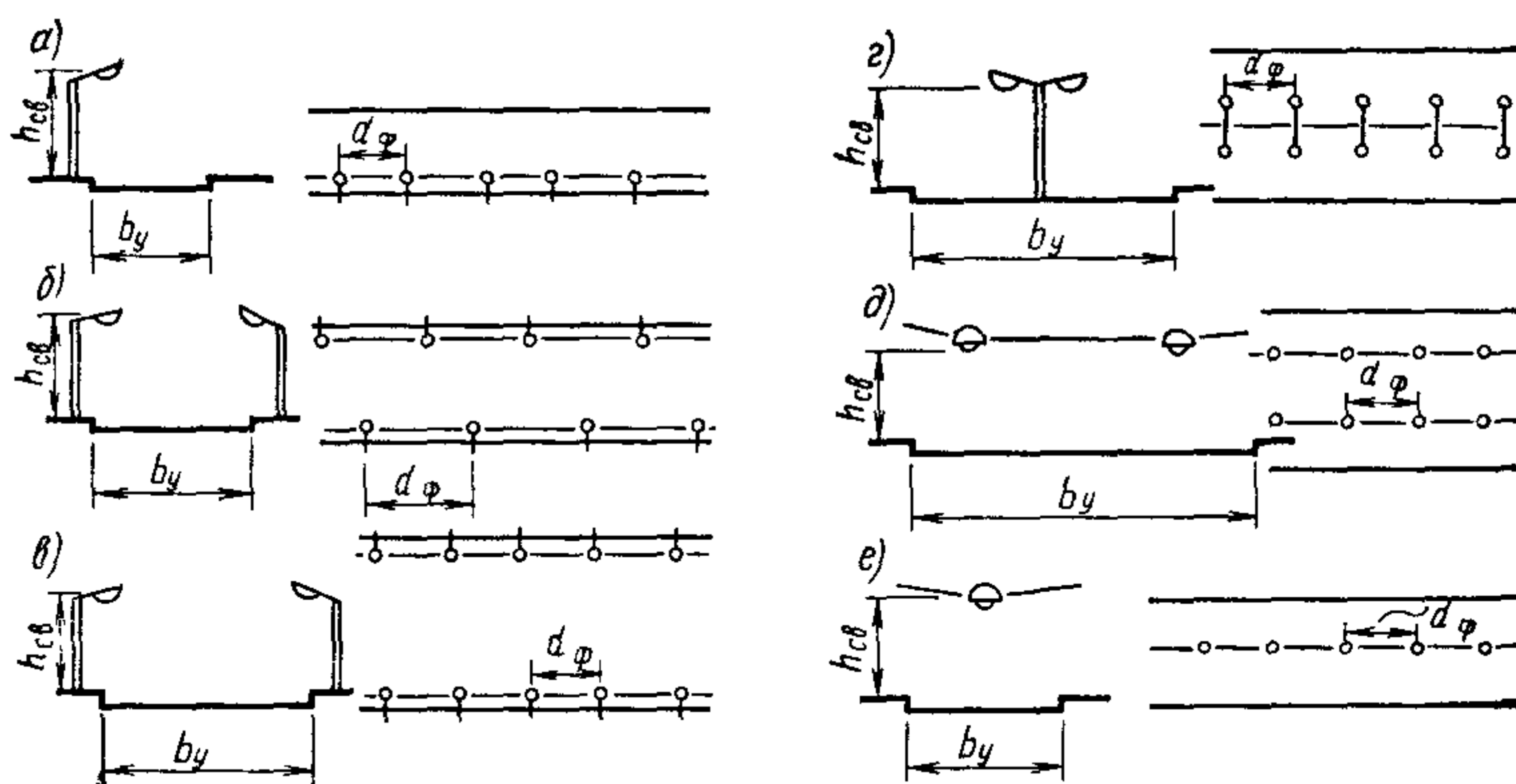
Рис. 110. Схемы размещения светильников на улицах и дорогах
