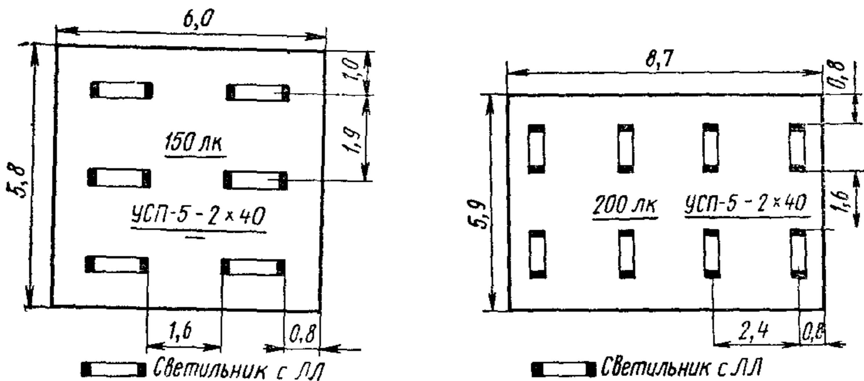
Рис. 63. Освещение кабинета массажа
