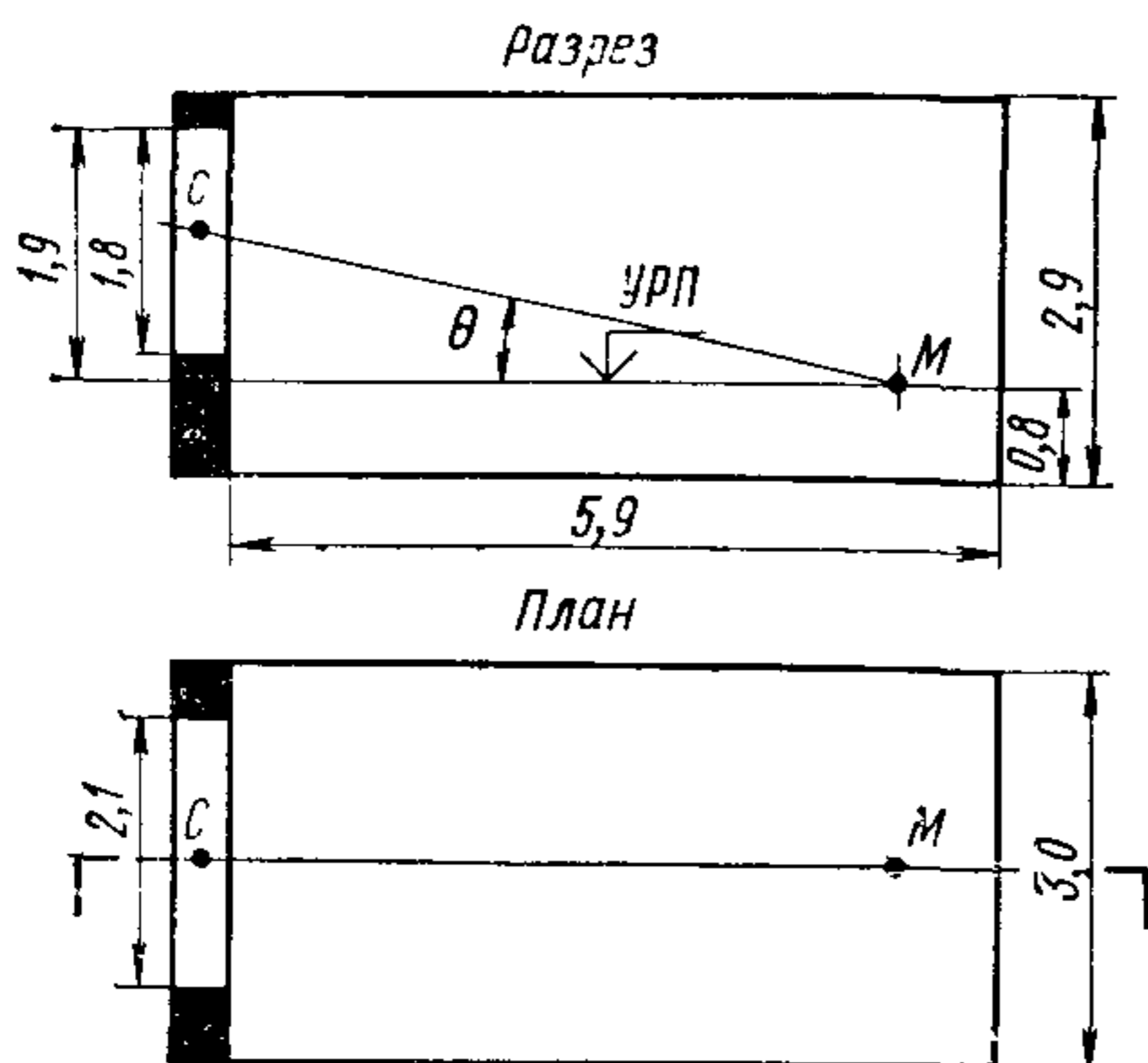
Рис. 23. План и разрез рабочего кабинета
