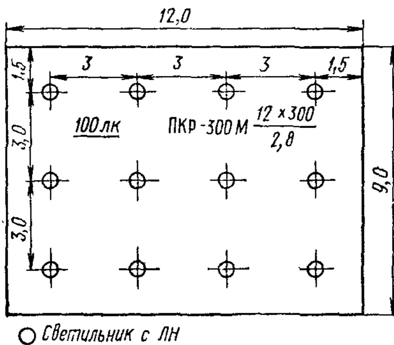
Рис. 56. Схема размещения светильников в спальне-веранде
