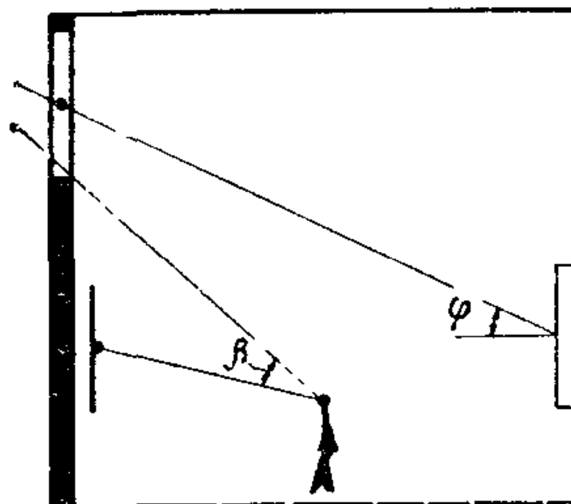
Рис. 30. Поперечный разрез выставочного помещения
