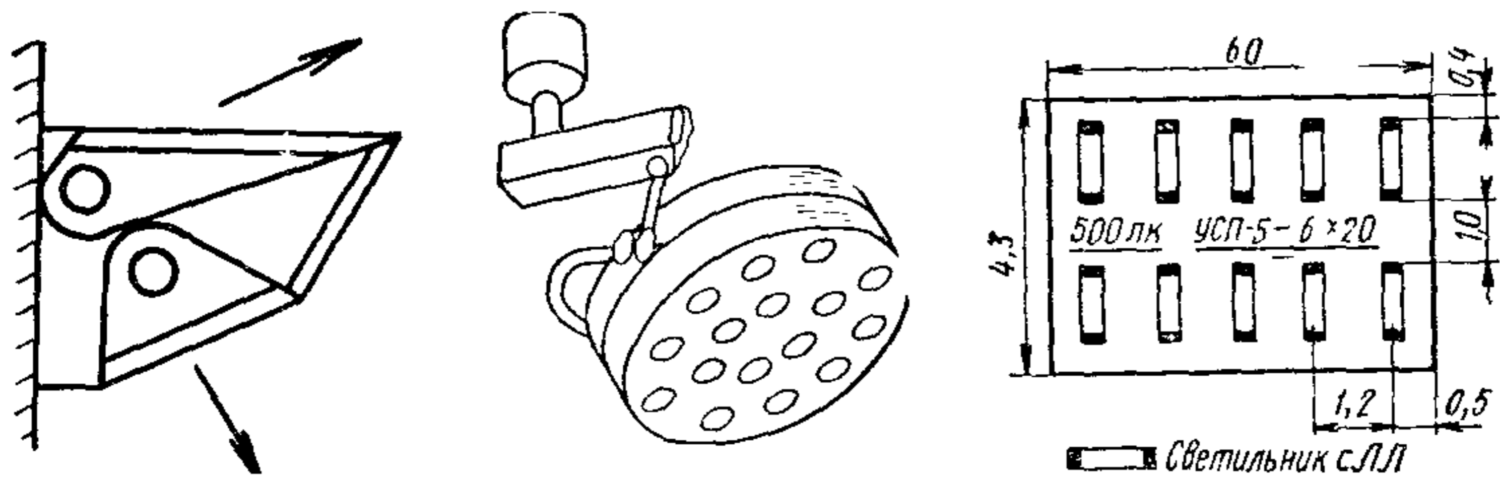
Рис. 60. Схема светильников для больничных палат
