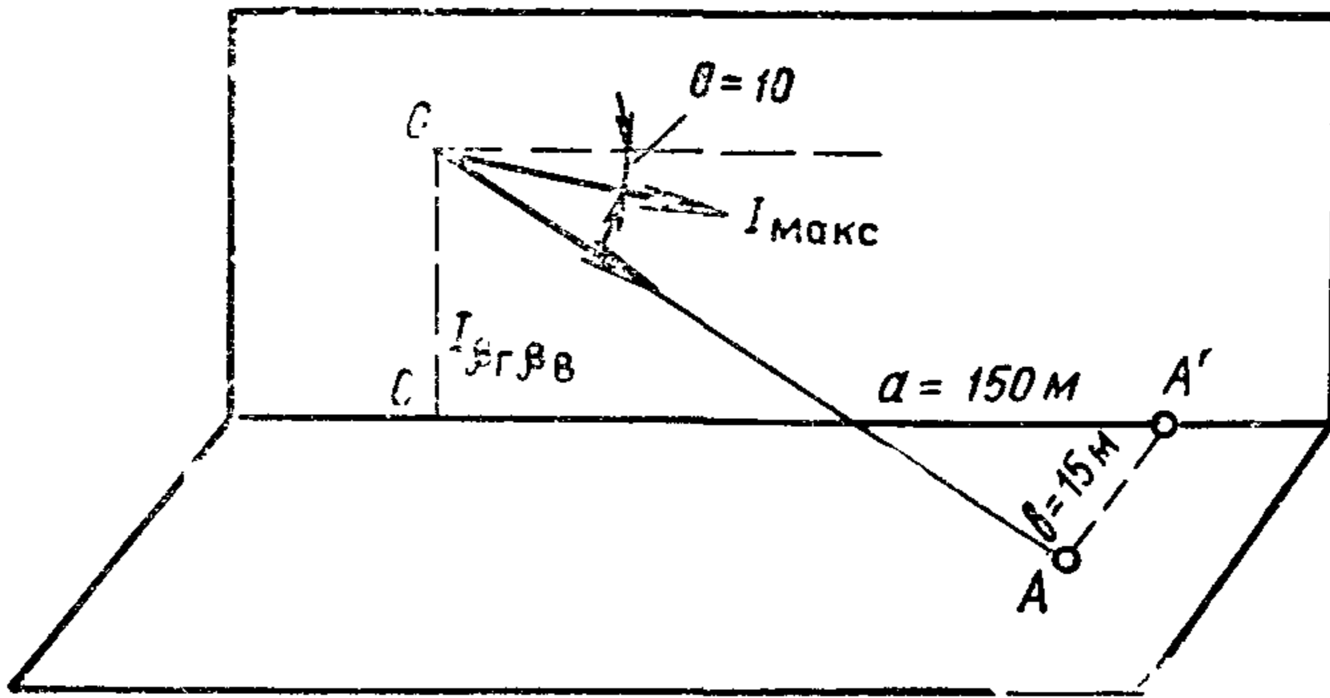
Рис. 81. Расположение прожектора относительно расчетной точки (к примеру 4)
