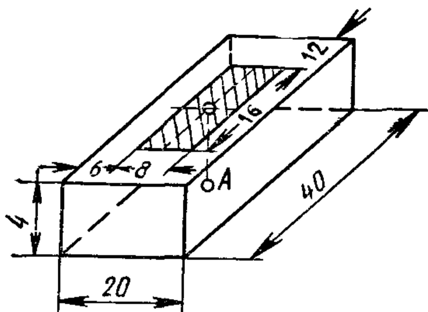
Рис. 93. Расположение светящей панели в помещении (к примеру 7)
