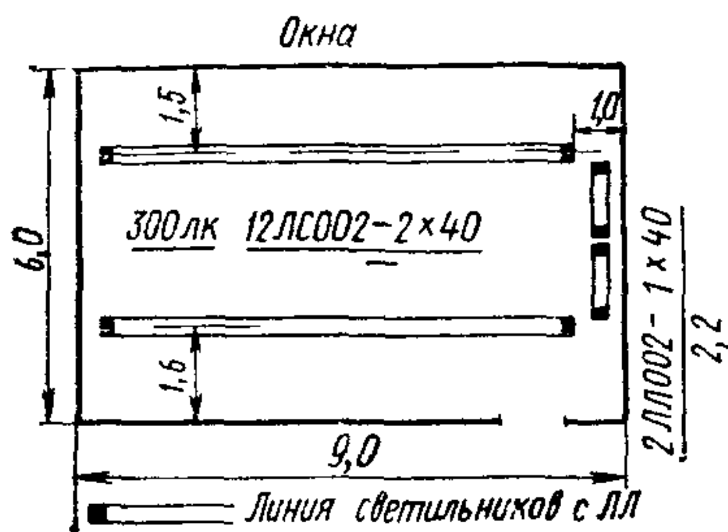
Рис. 52. Схема размещения светильников в классе
