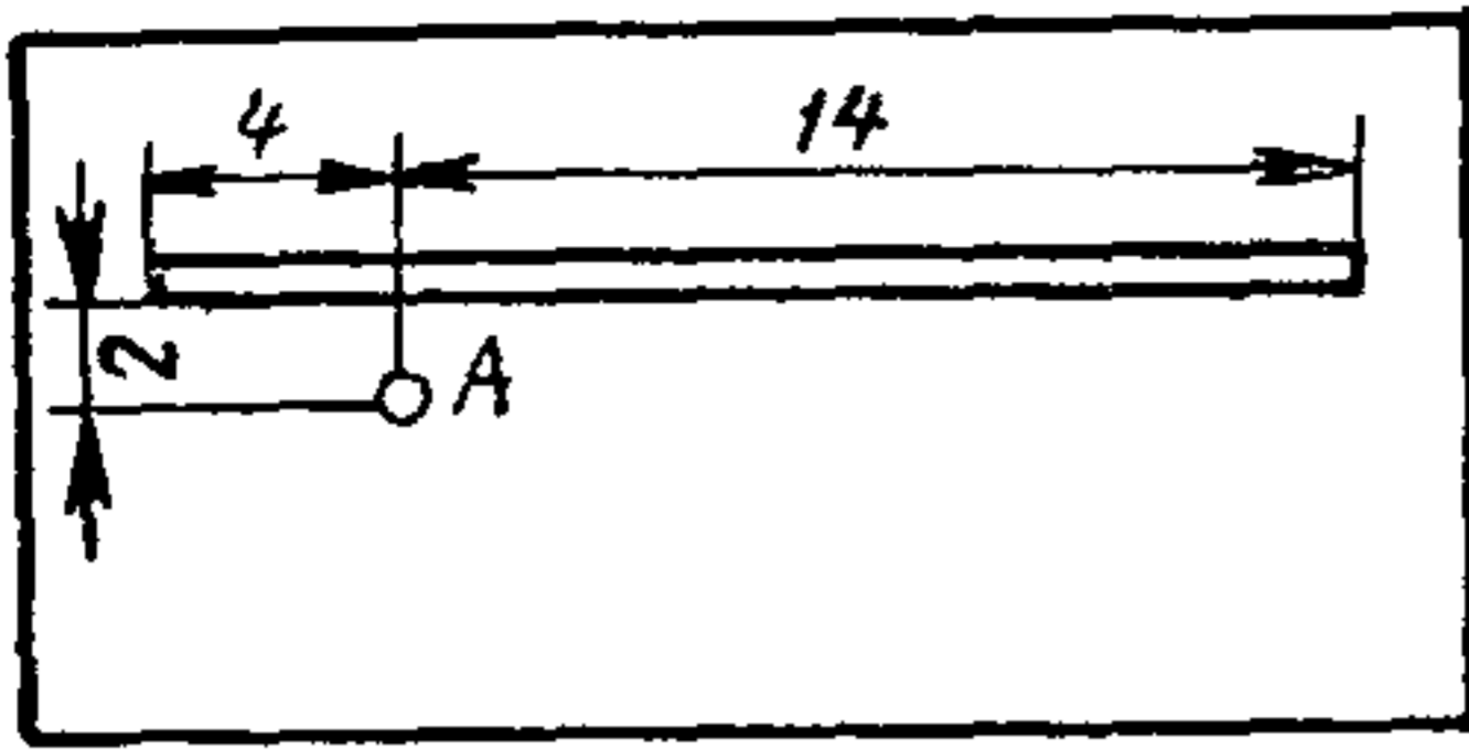
Рис. 88. Расположение светильника относительно расчетной точки (к примеру 6)
