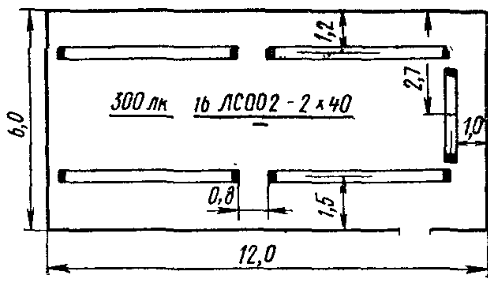
Рис. 55. Схема размещения светильников в столярной мастерской
