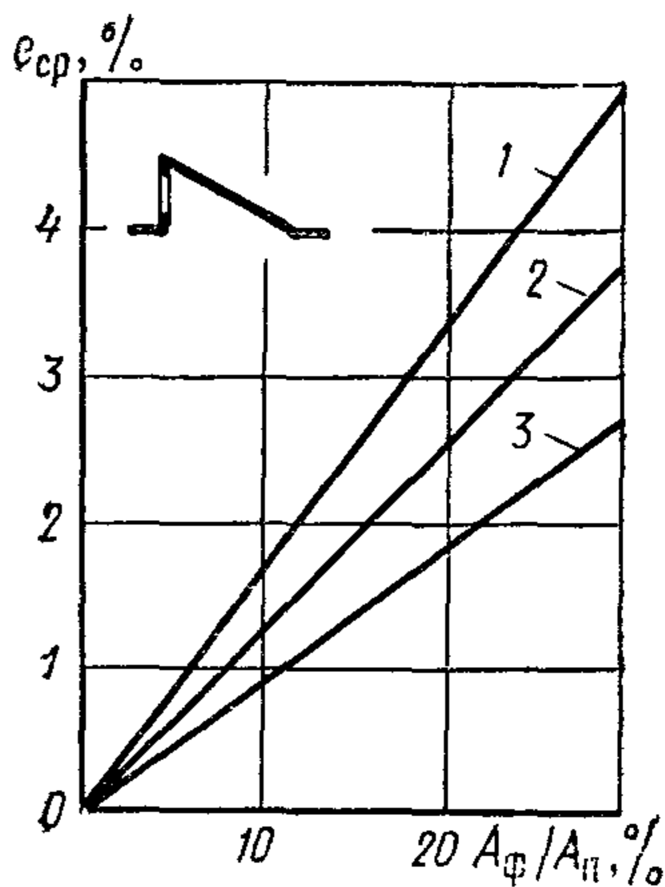
Рис. 3. График для определения среднего значения КЕО в производственных помещениях с трапециевидными фонарями
