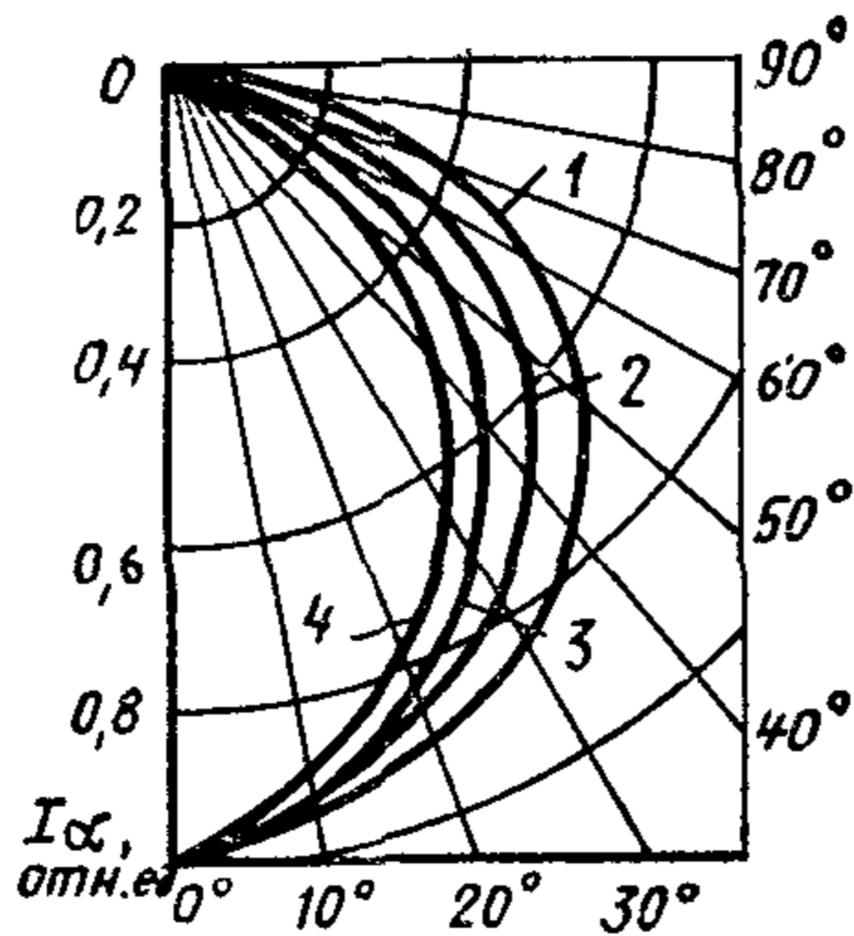
Рис. 97. Типовые кривые силы света светильников I_\alpha
