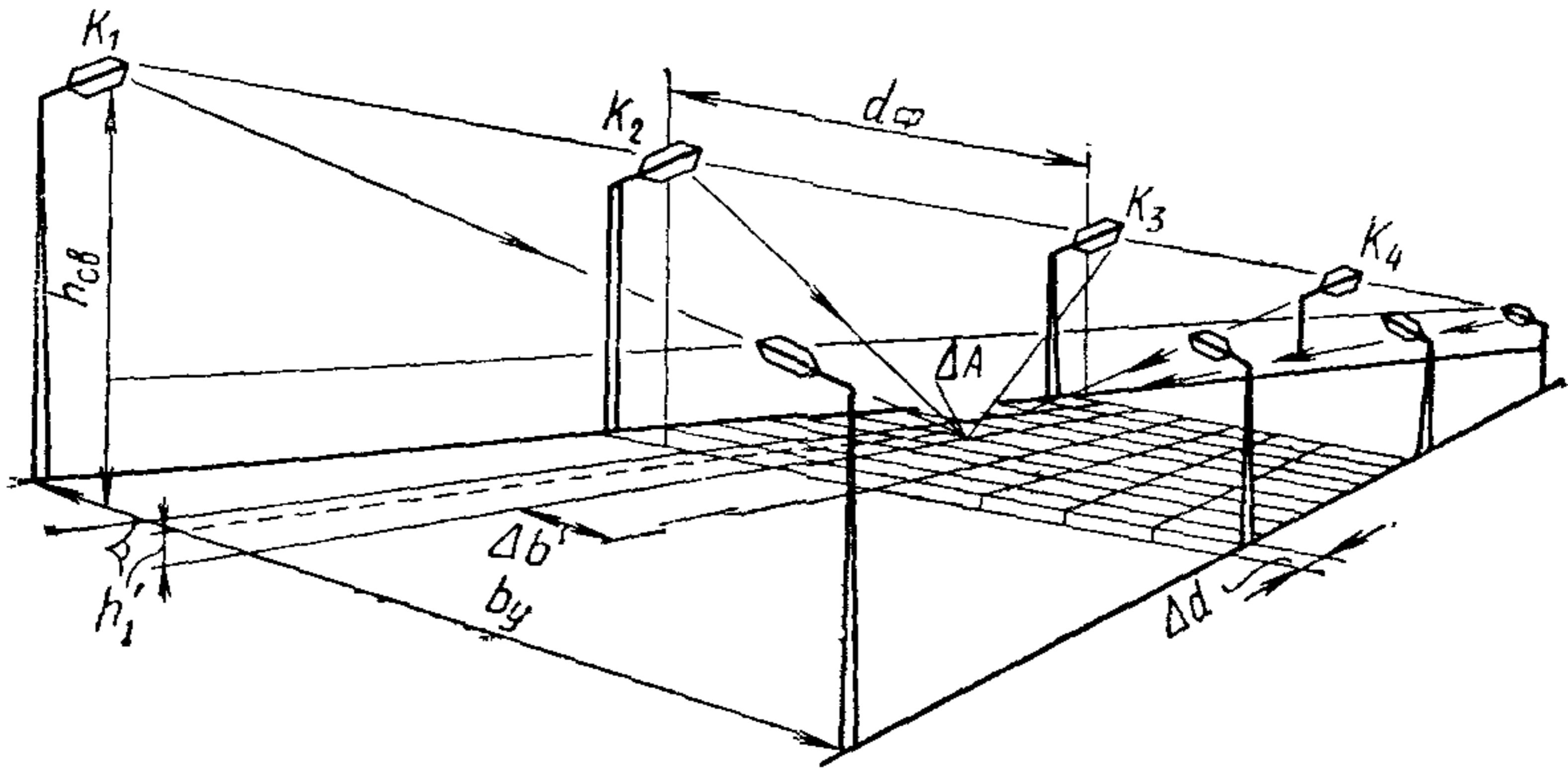
Рис. 121. К расчету параметров ОУ улицы точечным методом
