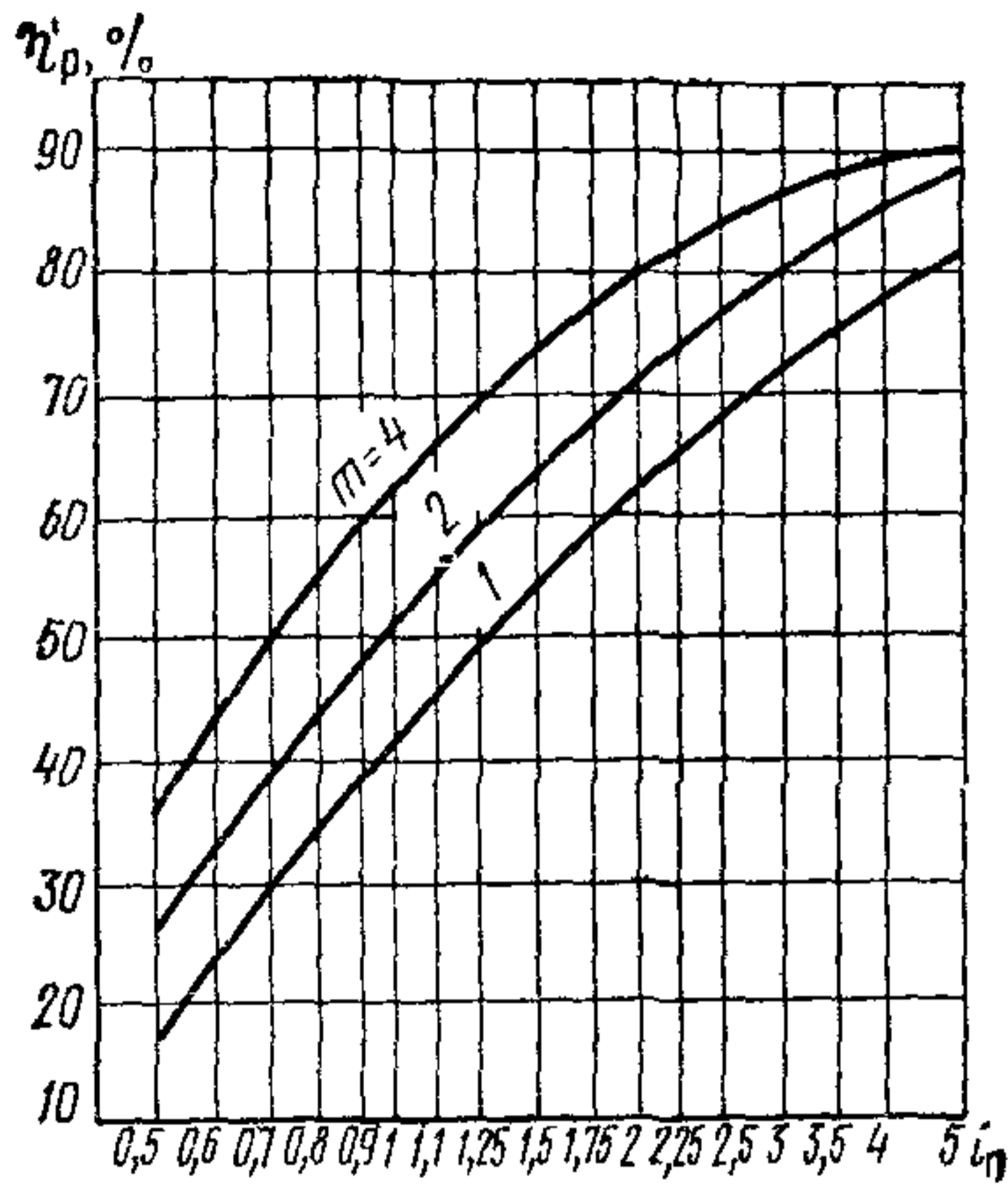
Рис. 49. График зависимости коэффициента первичного использования
