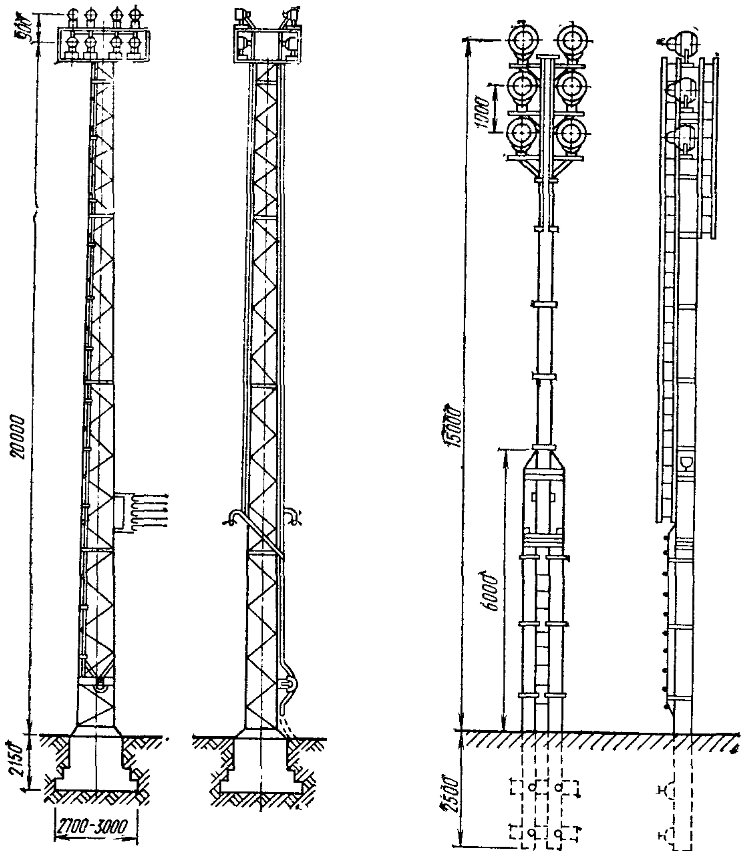
Рис. 104. Металлическая прожекторная мачта
