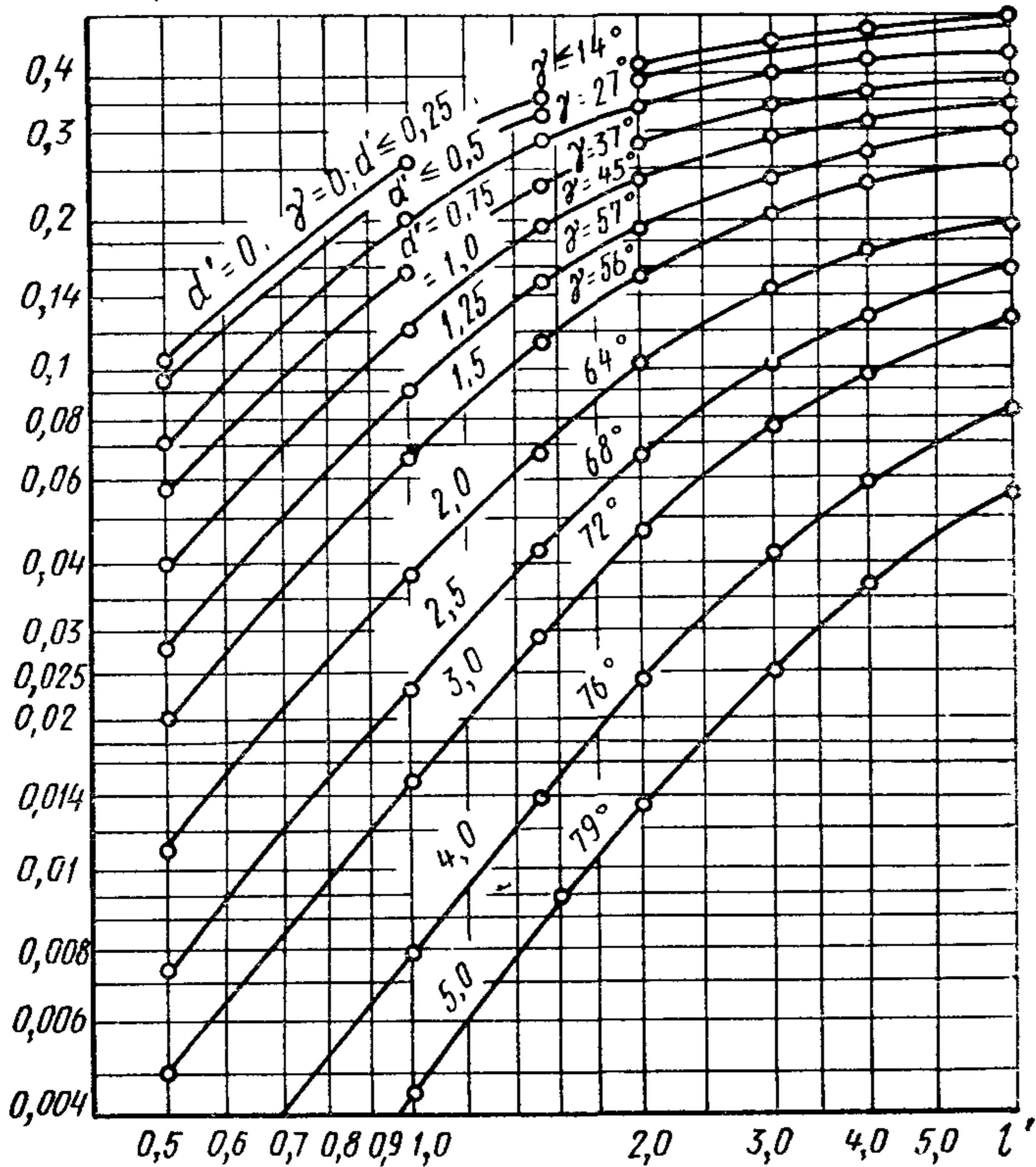
Рис. 86. Вспомогательный график для построения кривых равных значений относительной освещенности
