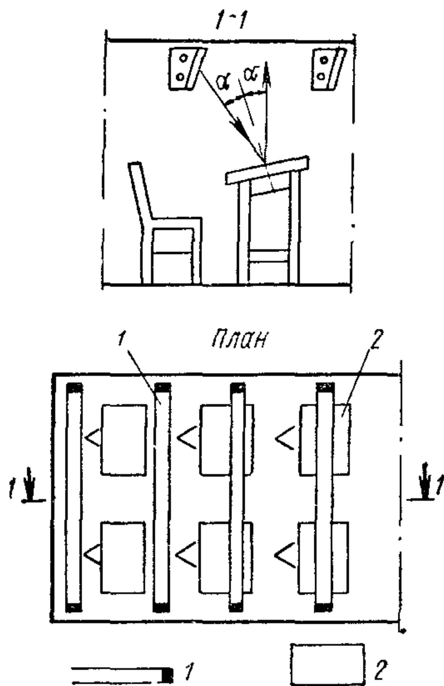
Рис. 51. Освещение столов для работы на кальке
