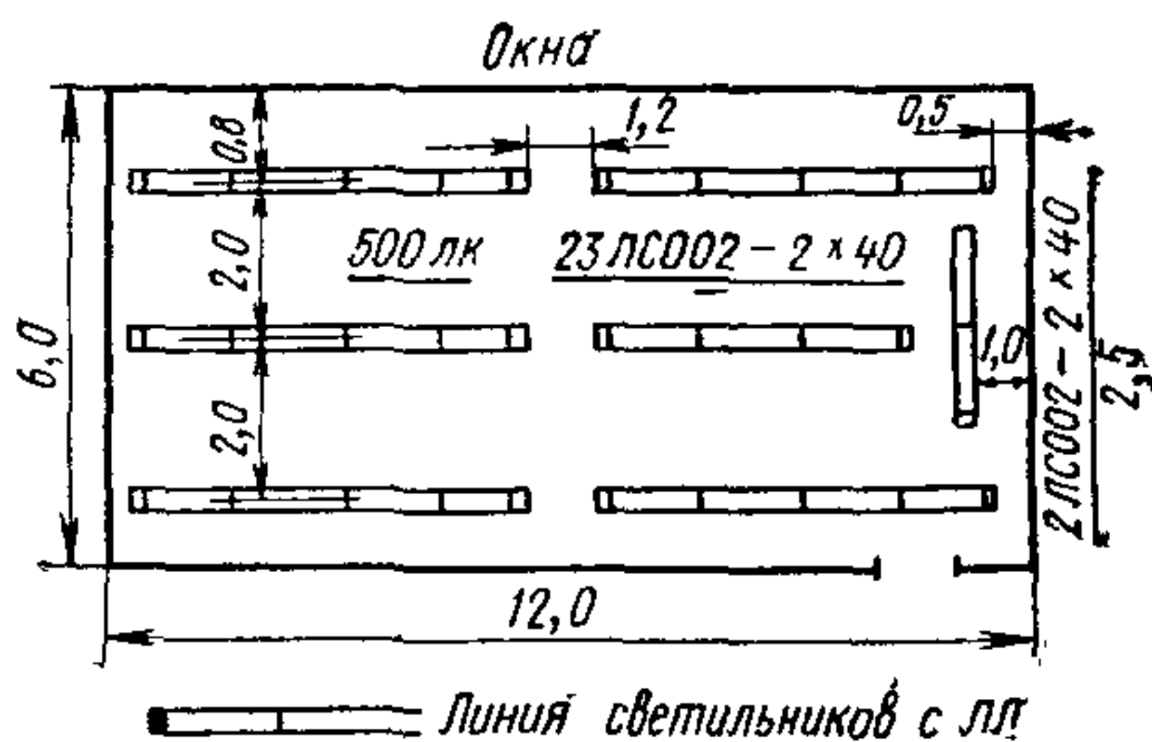
Рис. 52. Схема размещения светильников в классе
