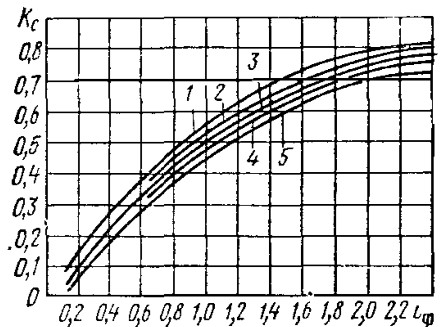
Рис. 17. График для определения коэффициента светопередачи K_c фонарей с диффузным отражением стенок шахты
