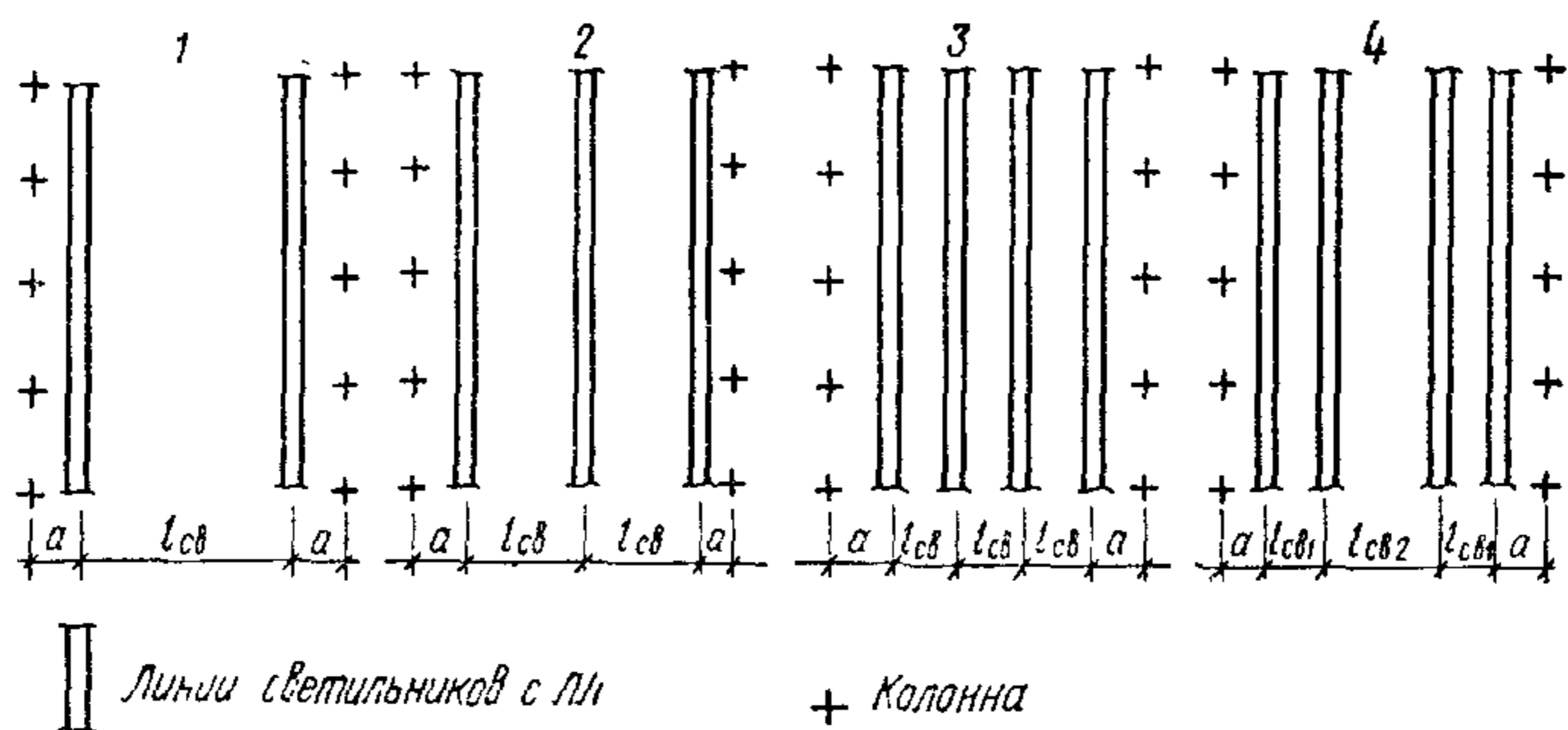
Рис. 33. Схемы размещения линий светильников с ЛЛ
