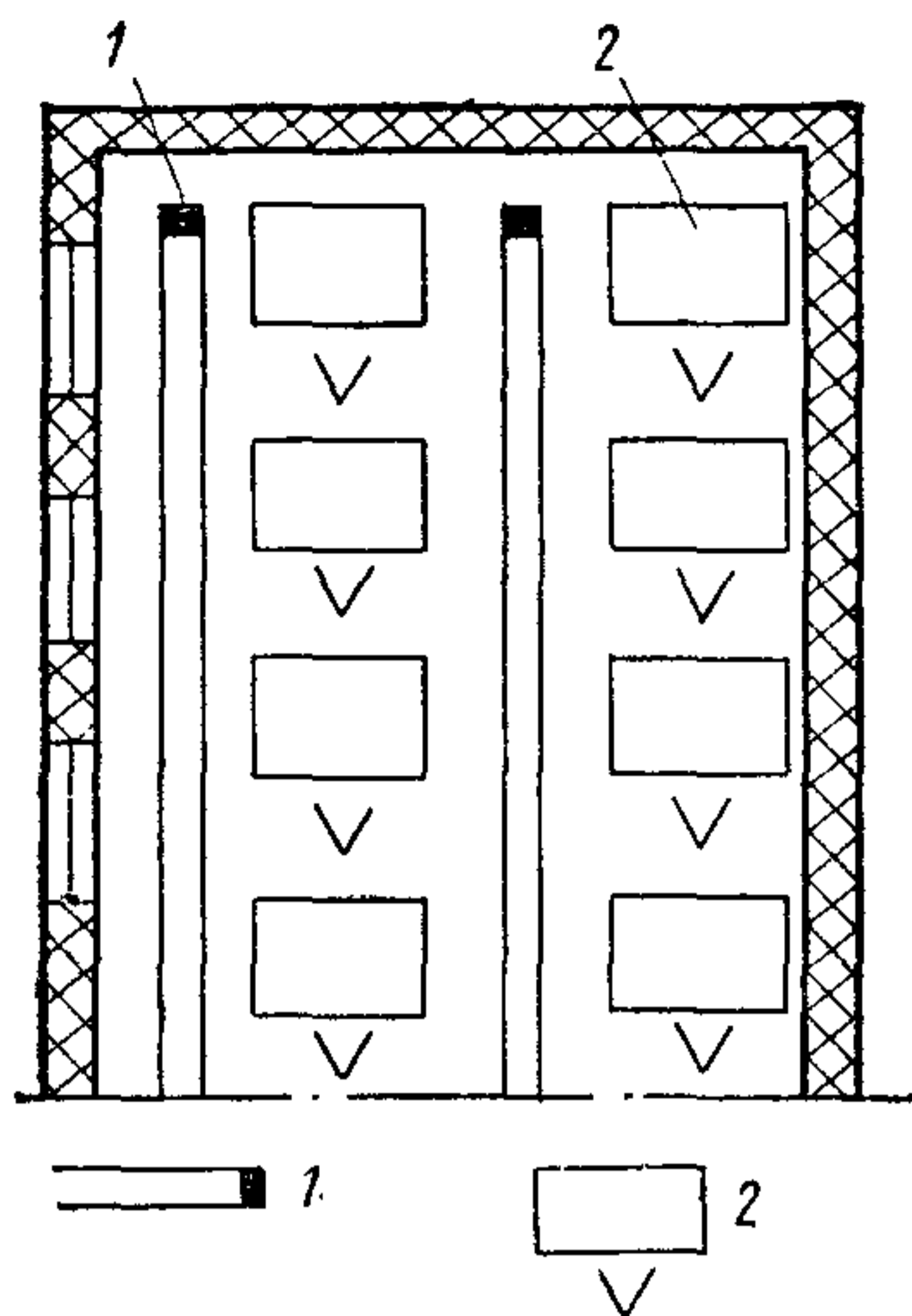
Рис. 50. Размещение светильников в помещениях конторского типа
