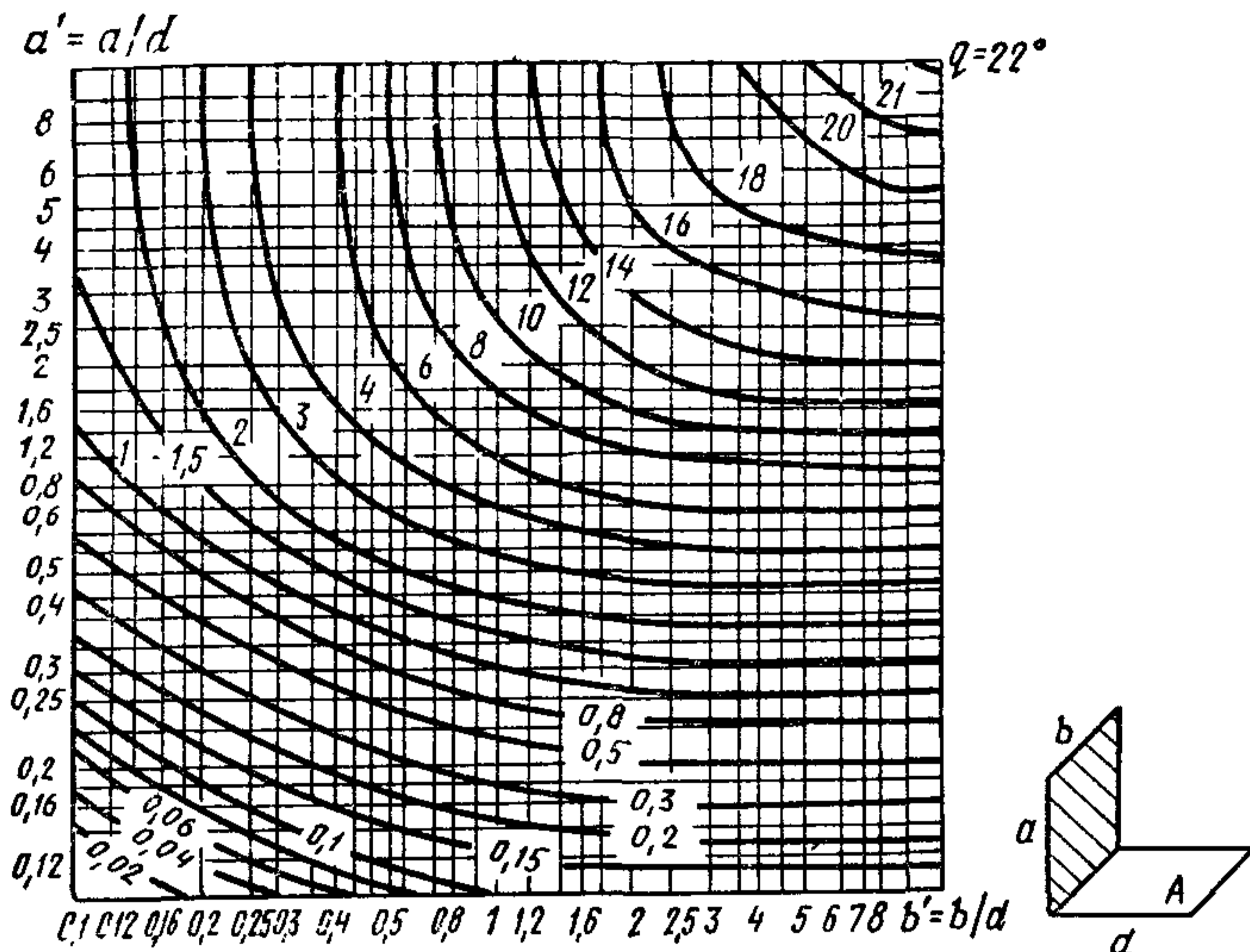
Рис. 90. Номограмма для расчета освещенности от равномерного светящего прямоугольника, перпендикулярного расчетной плоскости
