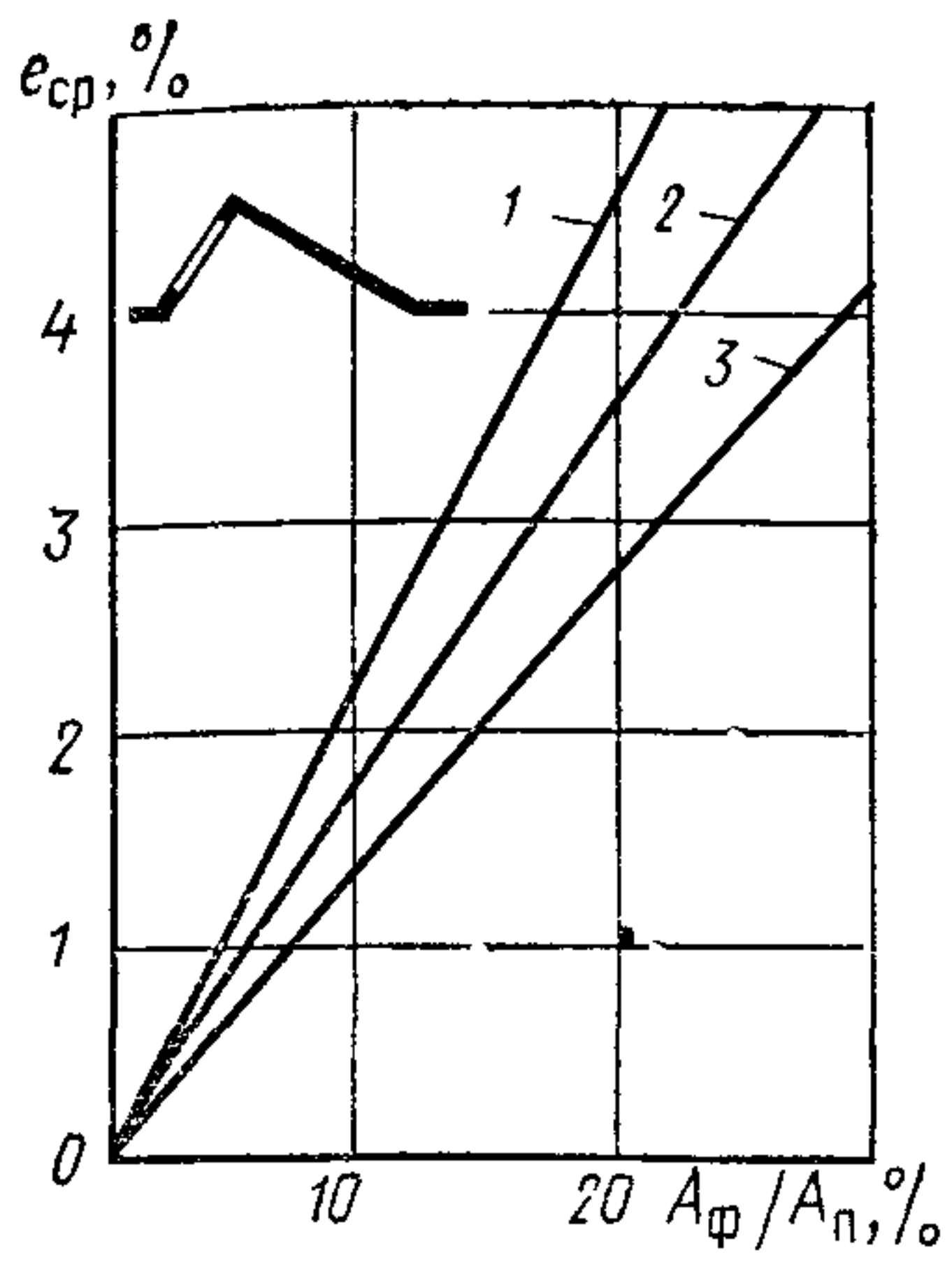
Рис. 5. График для определения среднего значения КЕО в производственных помещениях с фонарями шед, имеющими наклонное остекление 1 — три пролета и более; 2 — два пролета; 3 — один пролет
