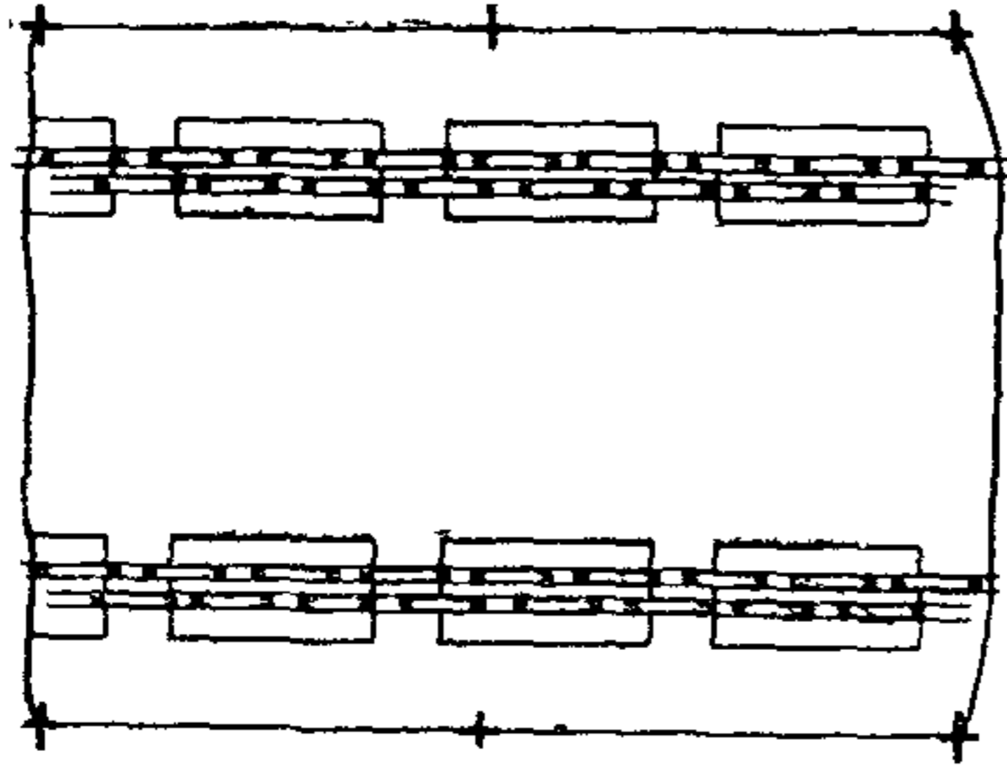
Рис. 41. Размещение светильников с ЛЛ на участке металлопокрытий, расположенном в помещении со строительным модулем 6×9 м, высотой 4 м: условные обозначения см на рис. 38 (размещение двойных линий светильников типа ПВЛП-2×40 либо светильников типа ПВЛМ-2×80 с ЛБР или ПВЛМ-ДО-2×65 по схеме 1 рис. 33)
