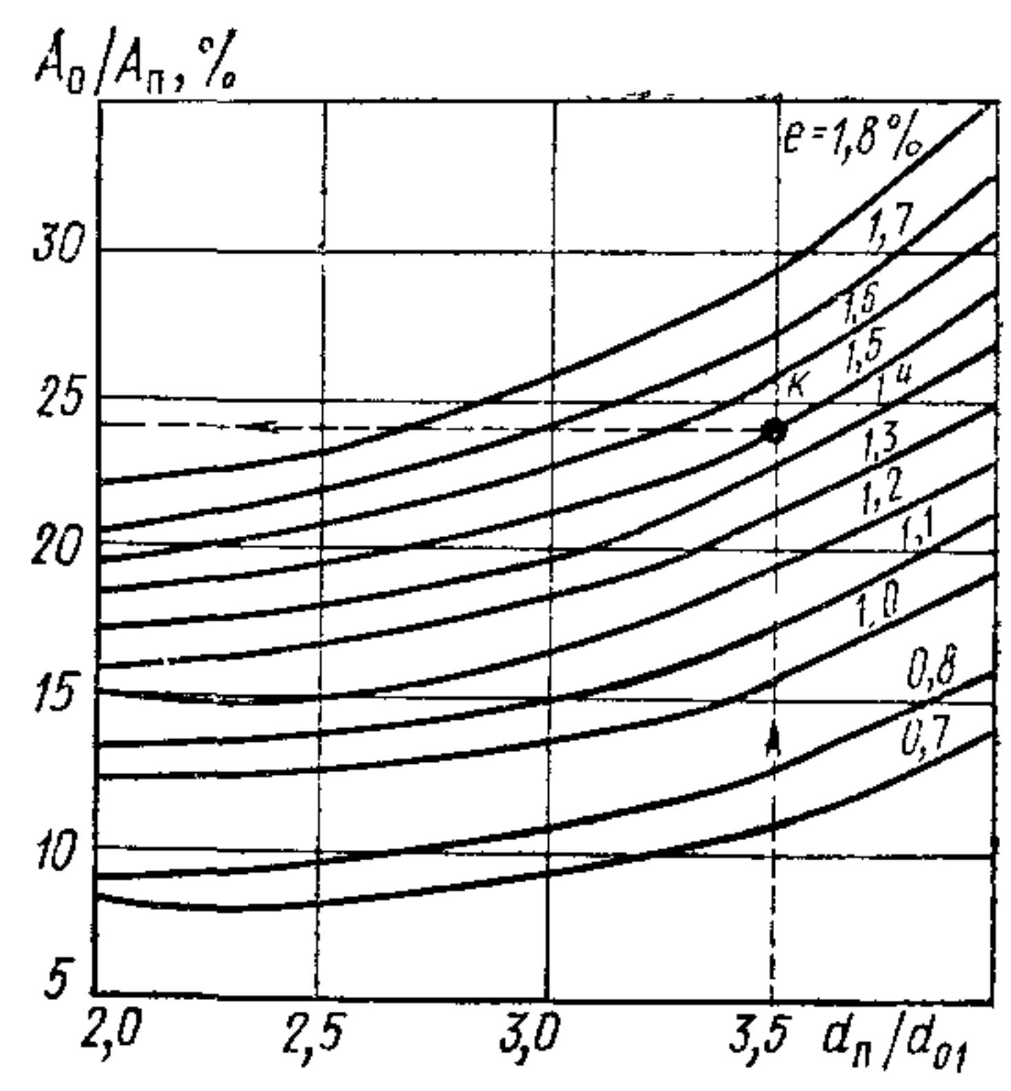
Рис. 7. График для определения КЕО при боковом освещении помещений общественных и производственных зданий
