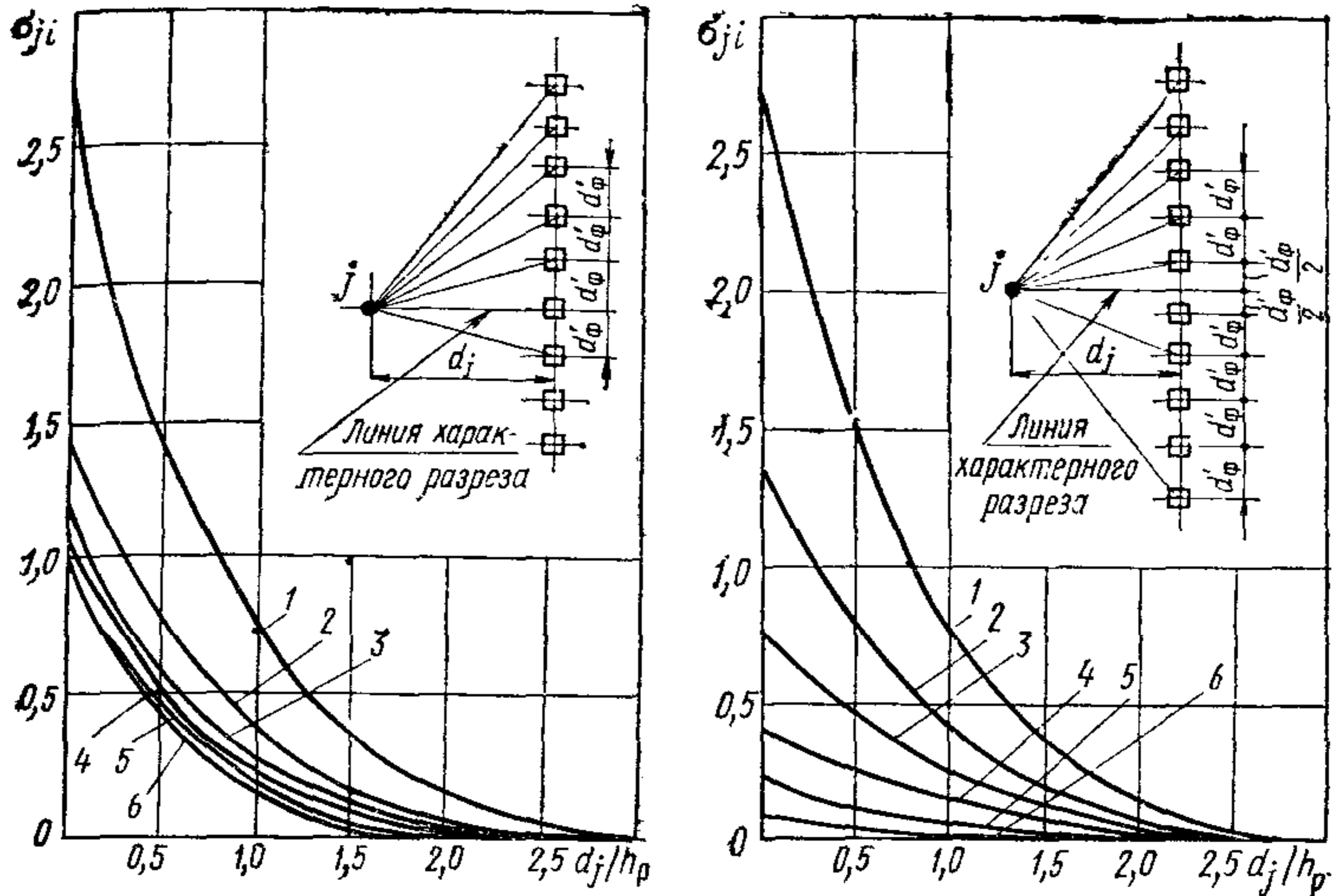
Рис. 11. Зависимость световой компоненты \sigma_{ij} ряда зенитных фонарей со световыми проемами размерами, м: 2,7 \times 2,7 ; 2,9 \times 2,9 и 2,9 \times 5,9 в точках характерного разреза по осям зенитных фонарей от d_j/h_p
