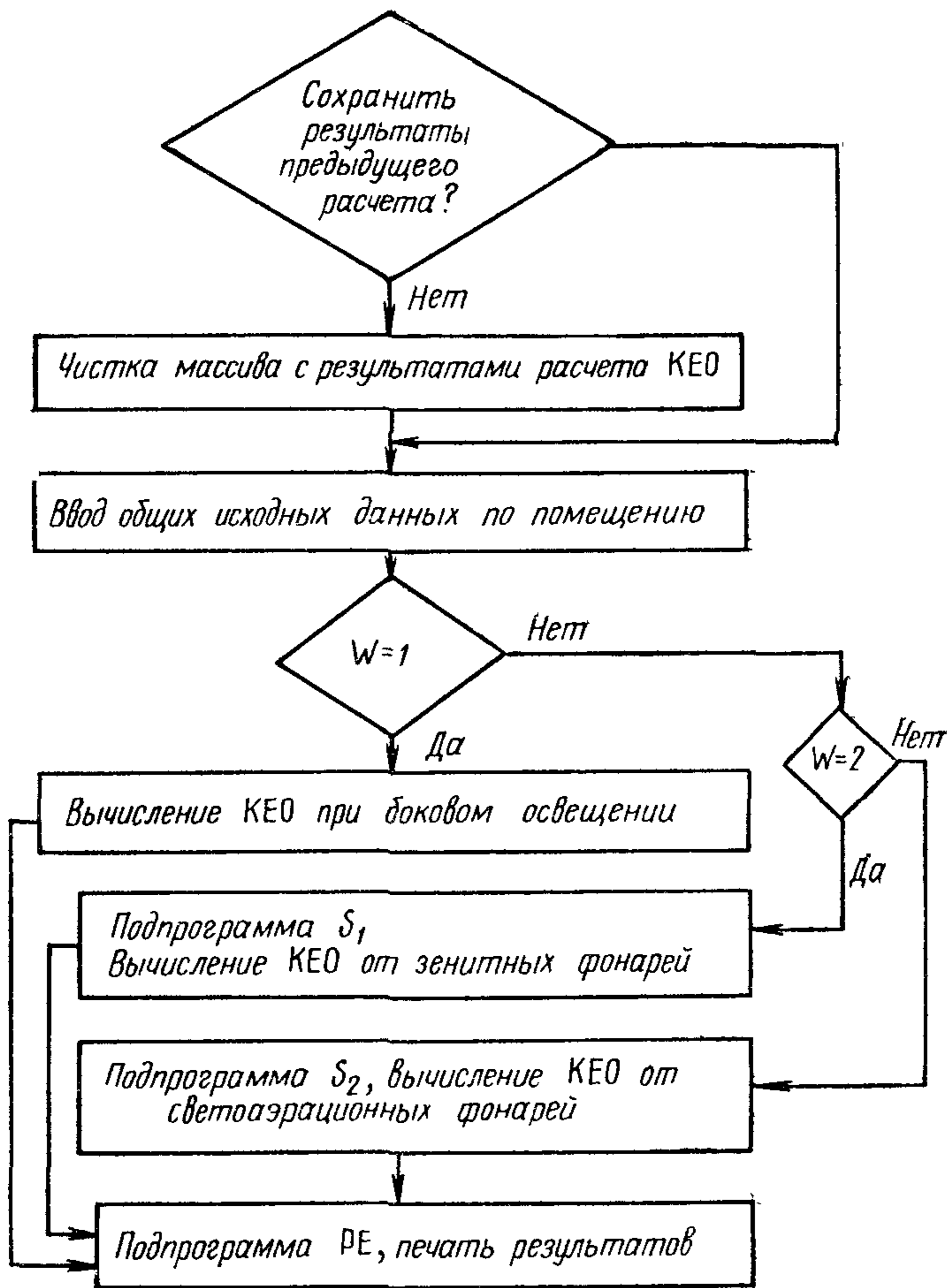
Рис. прил. 1. Укрупненная блок-схема программы
