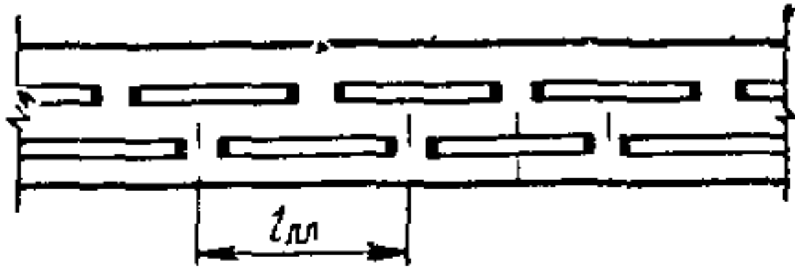
Рис. 47. Двухрядное размещение люминесцентных ламп в карнизе
