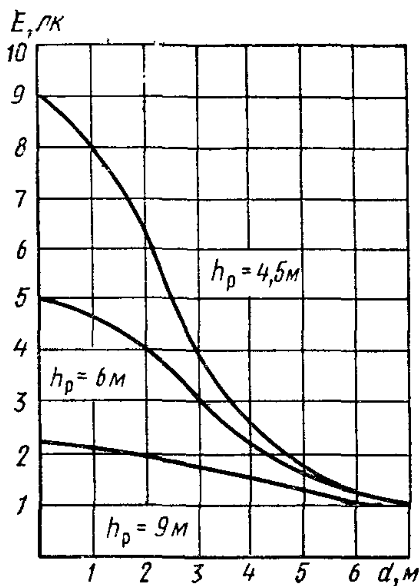
Рис. 73. Пространственные изолюксы условной горизонтальной освещенности. С светильники У, УПМ-15, УП-24, Астра 1, 11, 12
