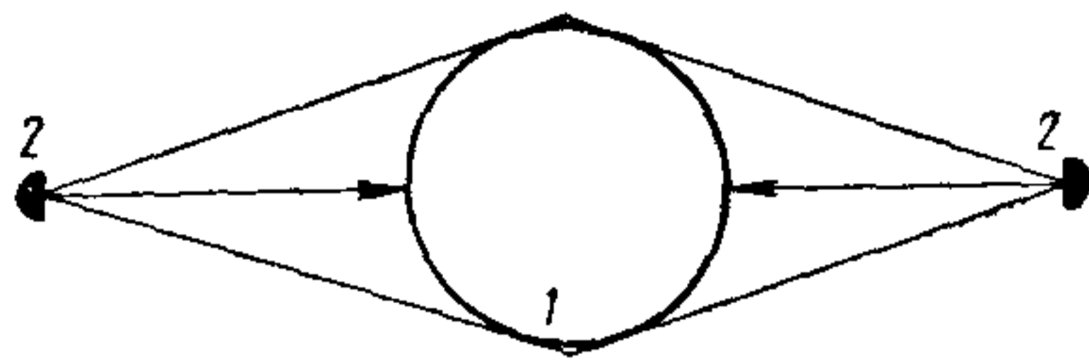
Рис. 117. Варианты освещения высоких круглых башен 1 — башня; 2 — прожекторы
