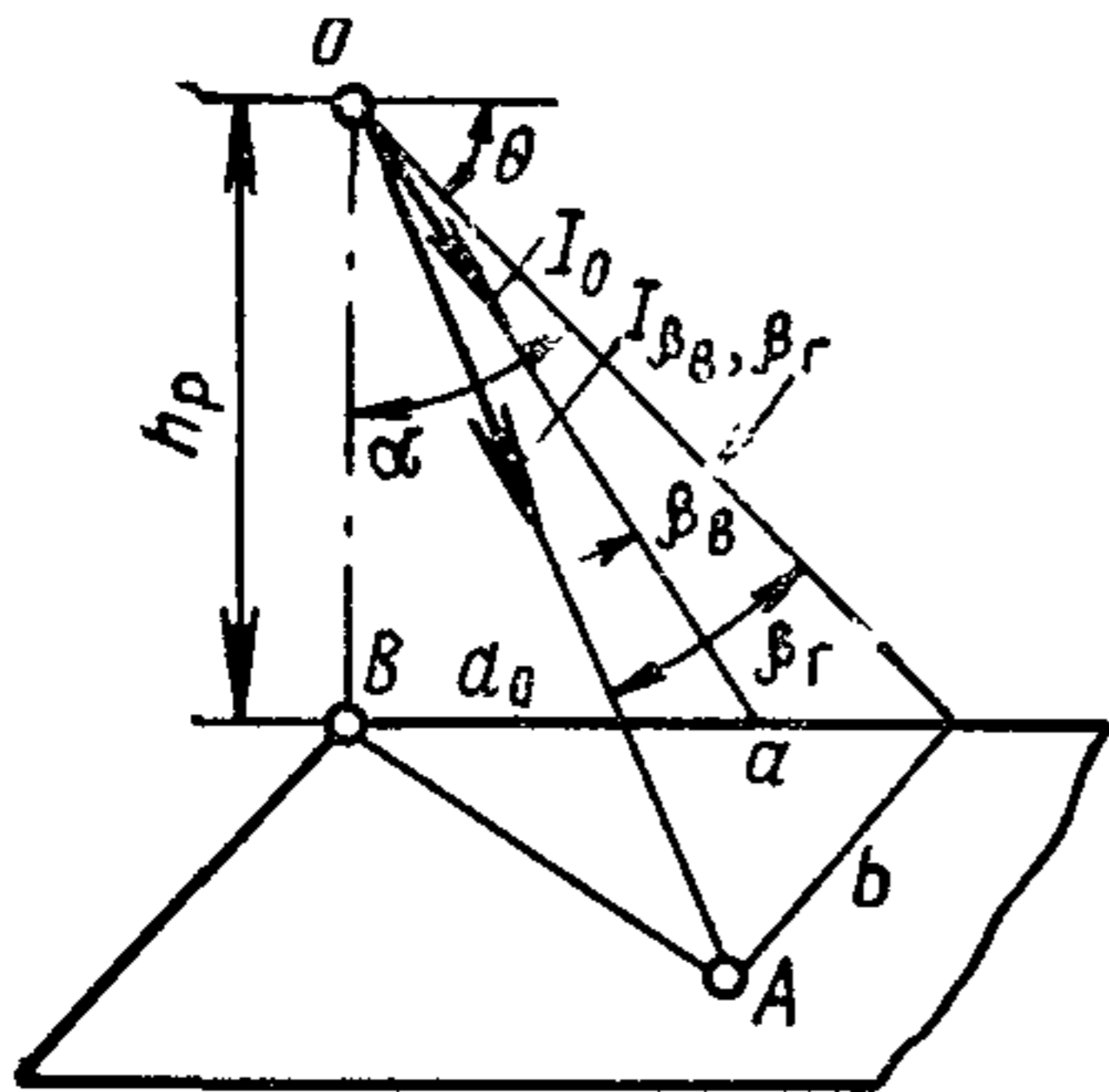
Рис. 78. К расчету освещенности от прожектора заливающего света
