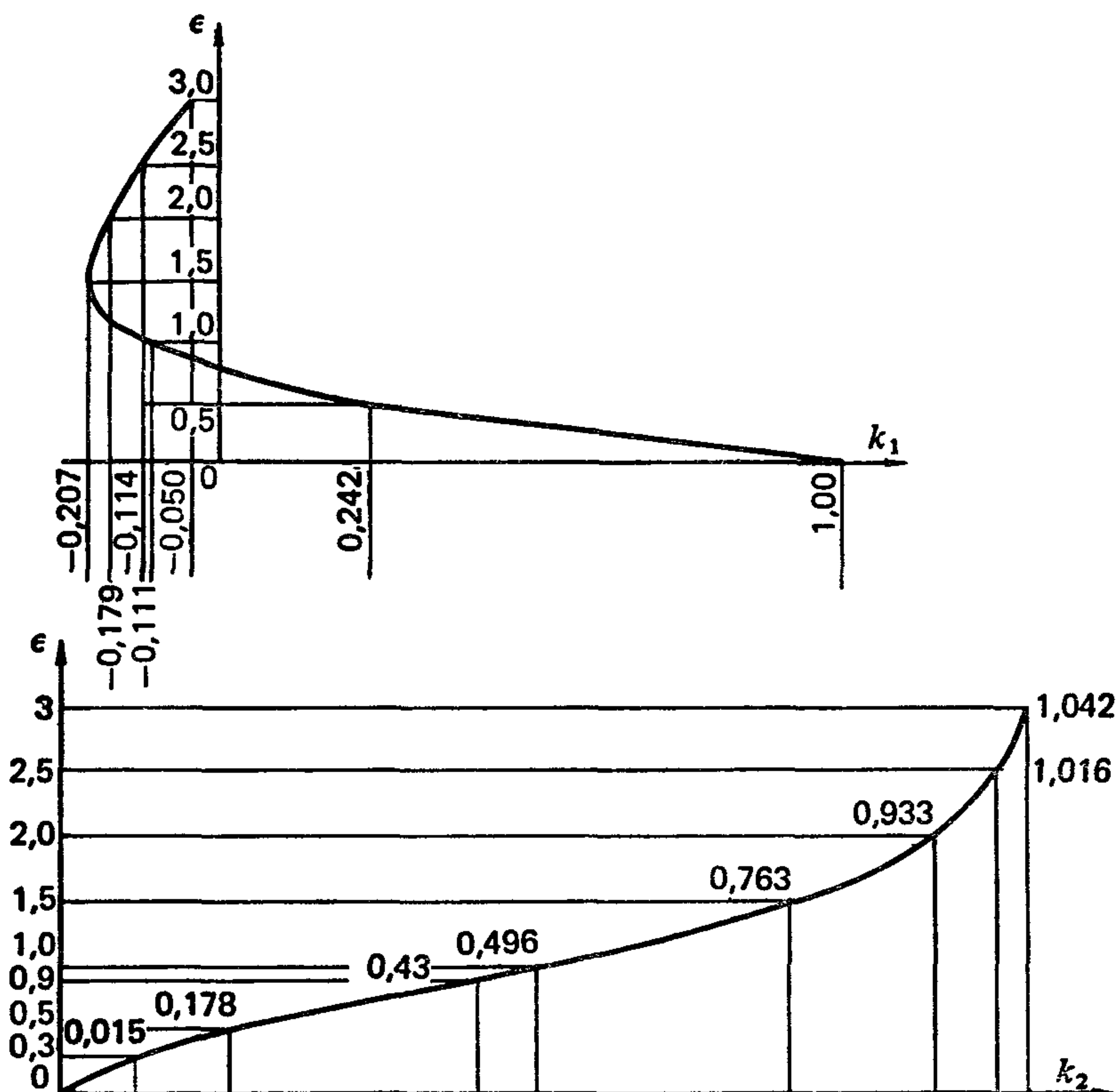
Черт. 16. Значения коэффициентов k_1, k_2
