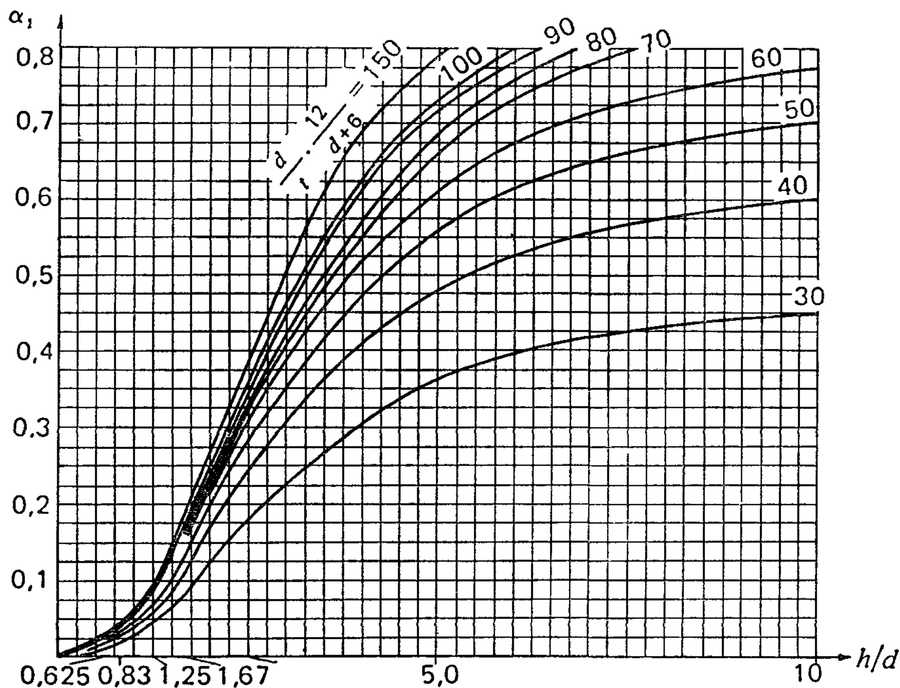
Черт. 12 (4). Значение коэффициента \alpha_1
