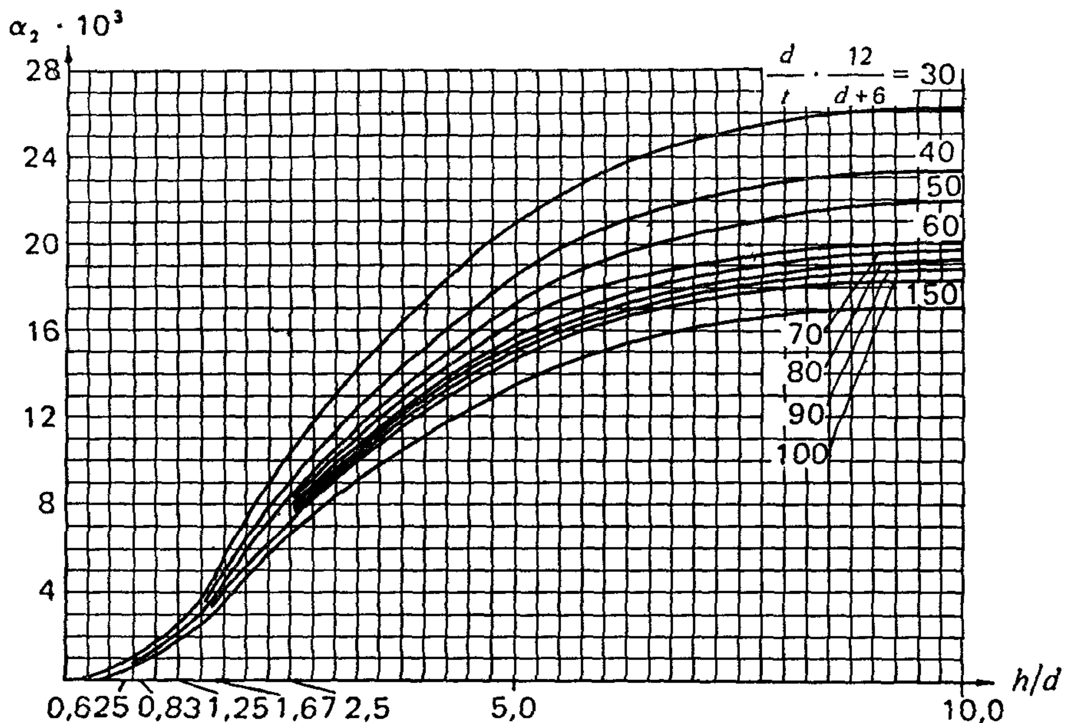
Черт. 13 (5). Значение коэффициента \alpha_2
