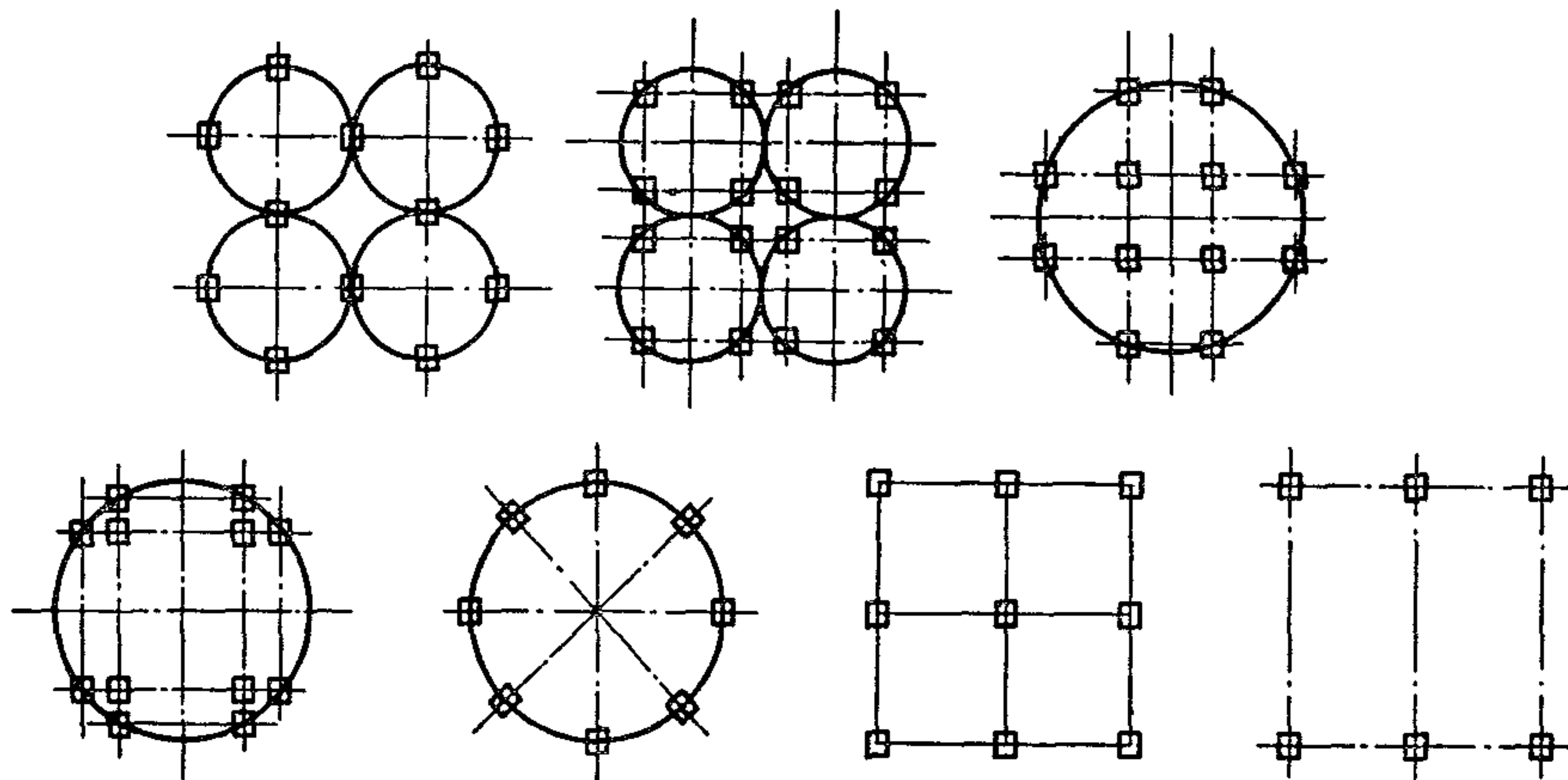
Черт. 10. Схемы расположения колонн подсилосного этажа
