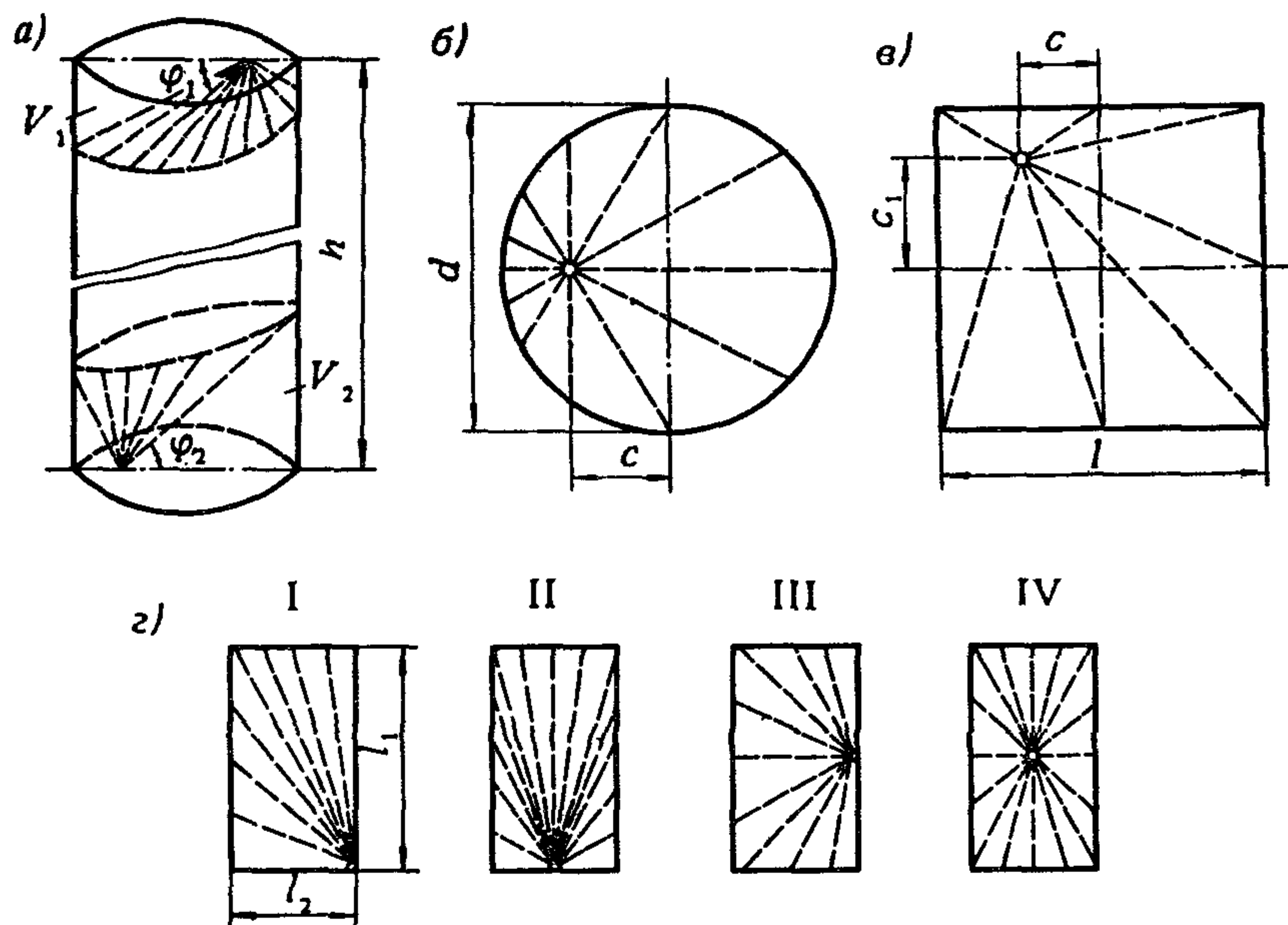
Черт. 1. Объем сыпучего материала в силосе
