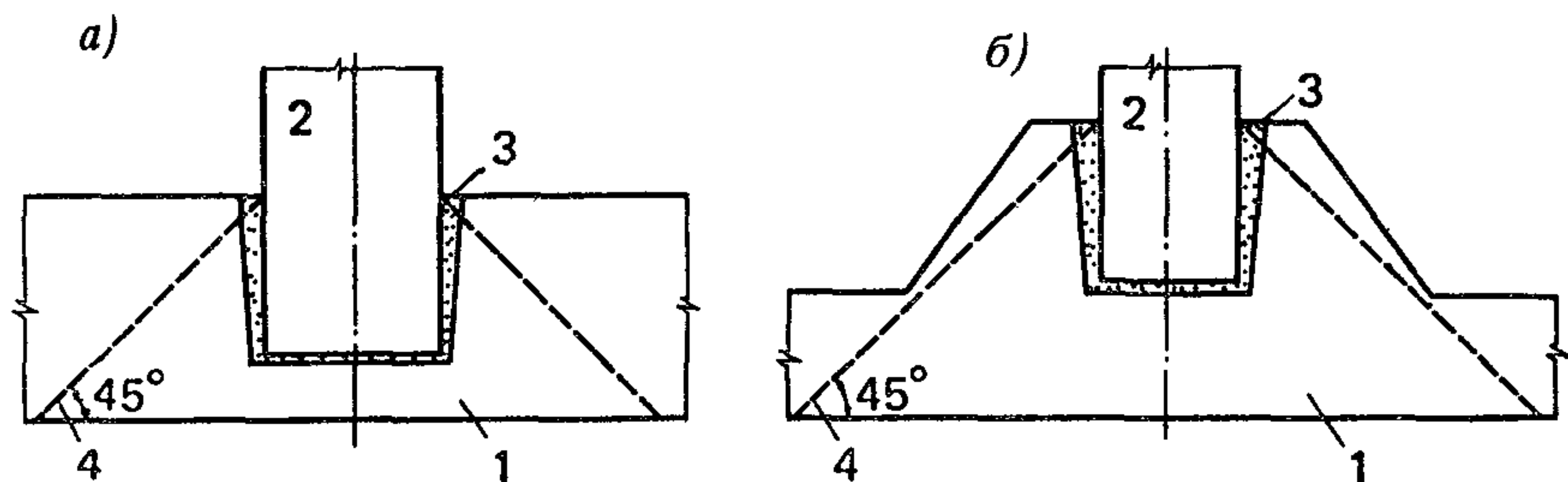
Черт. 21. Схема продавливания фундаментной плиты
