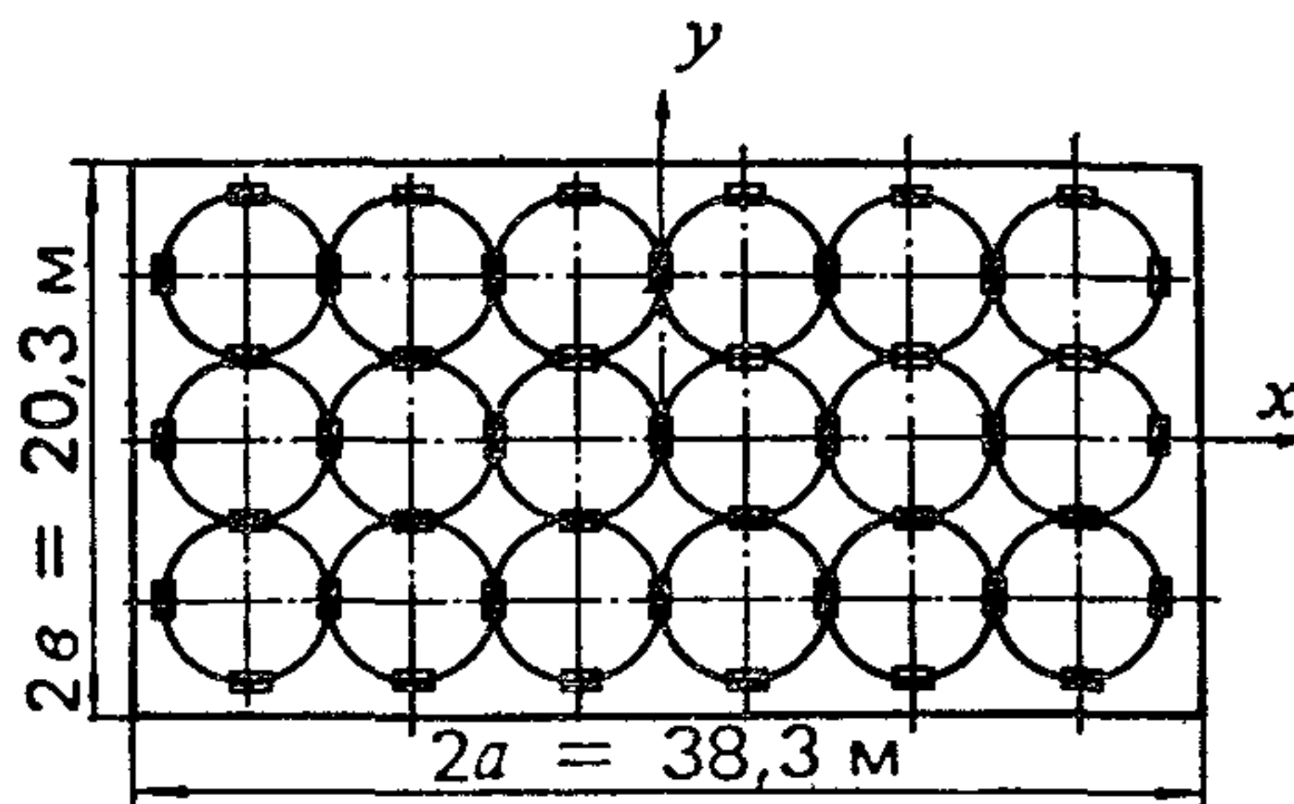
Черт. 7. Схема фундаментной плиты силосного корпуса
