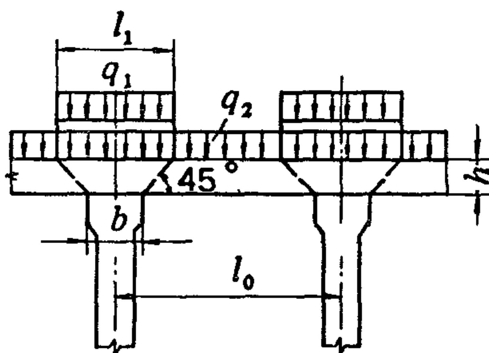
Черт. 19 (8). Передача нагрузки от балки на колонну
