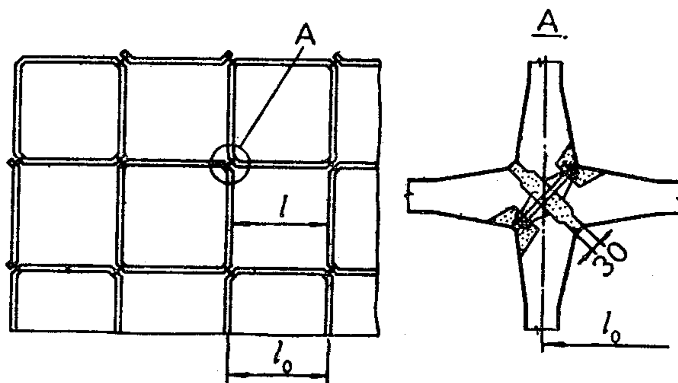
Черт. 4. Стены силосного корпуса с квадратными силосами
