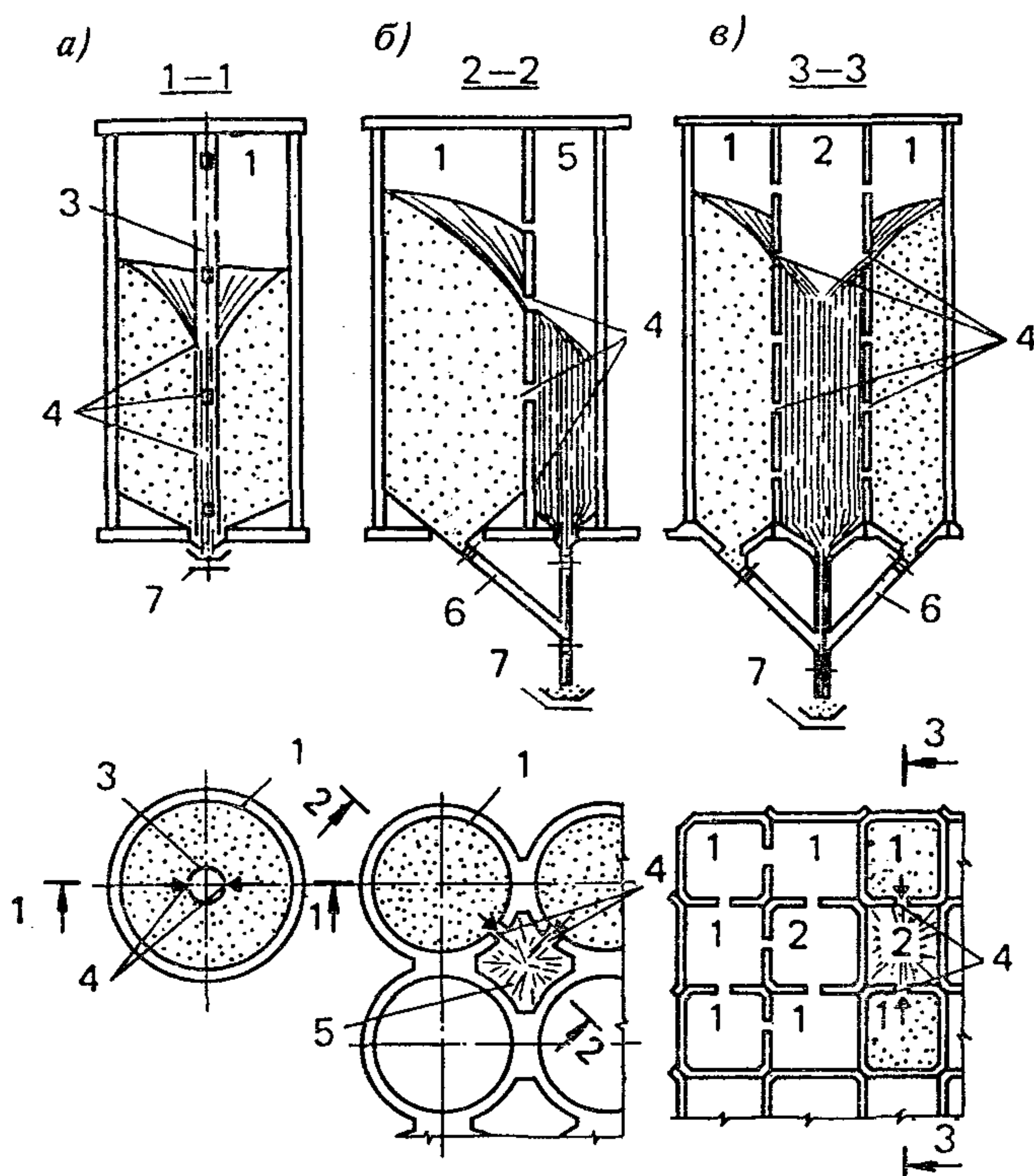
Черт. 3 (2). Выпуск сыпучего материала из силоса
