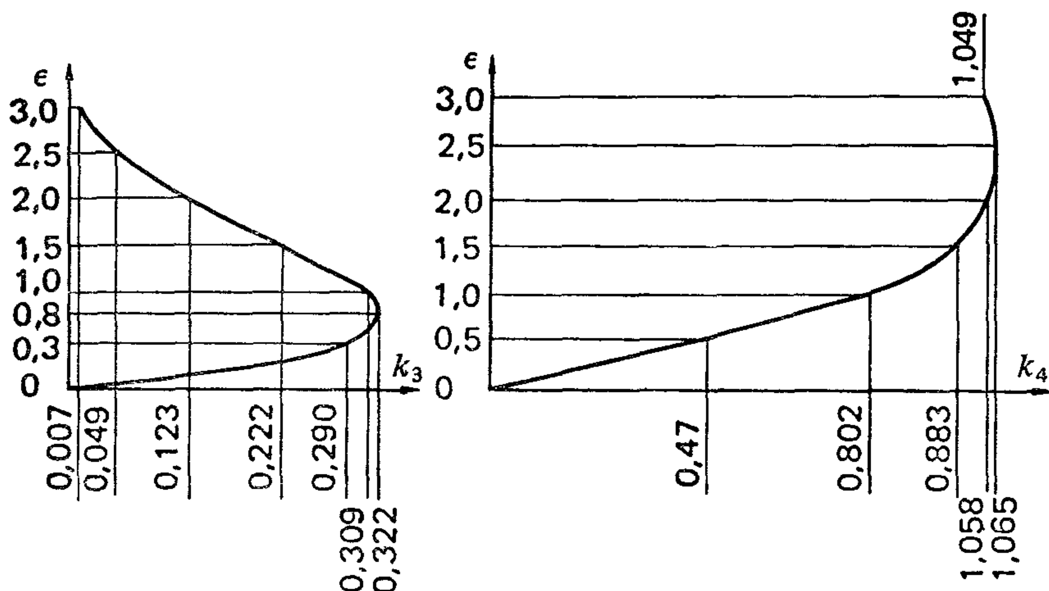
Черт. 17. Значения коэффициентов k_3, k_4
