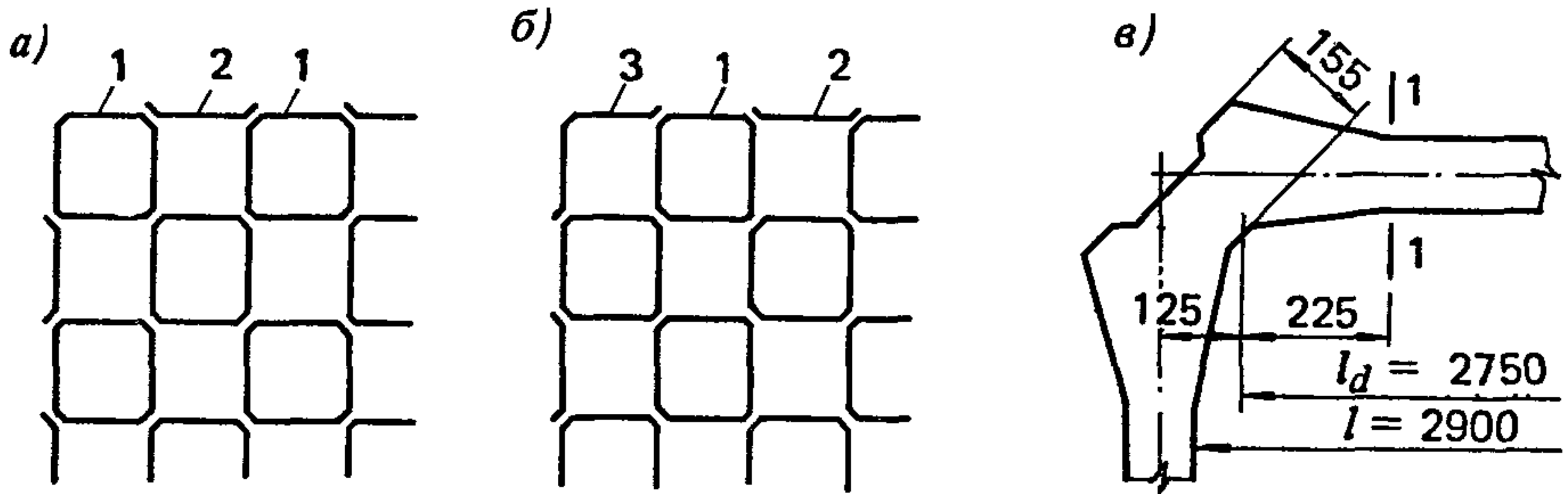
Черт. 1. План силосного корпуса (с квадратными силосами)
