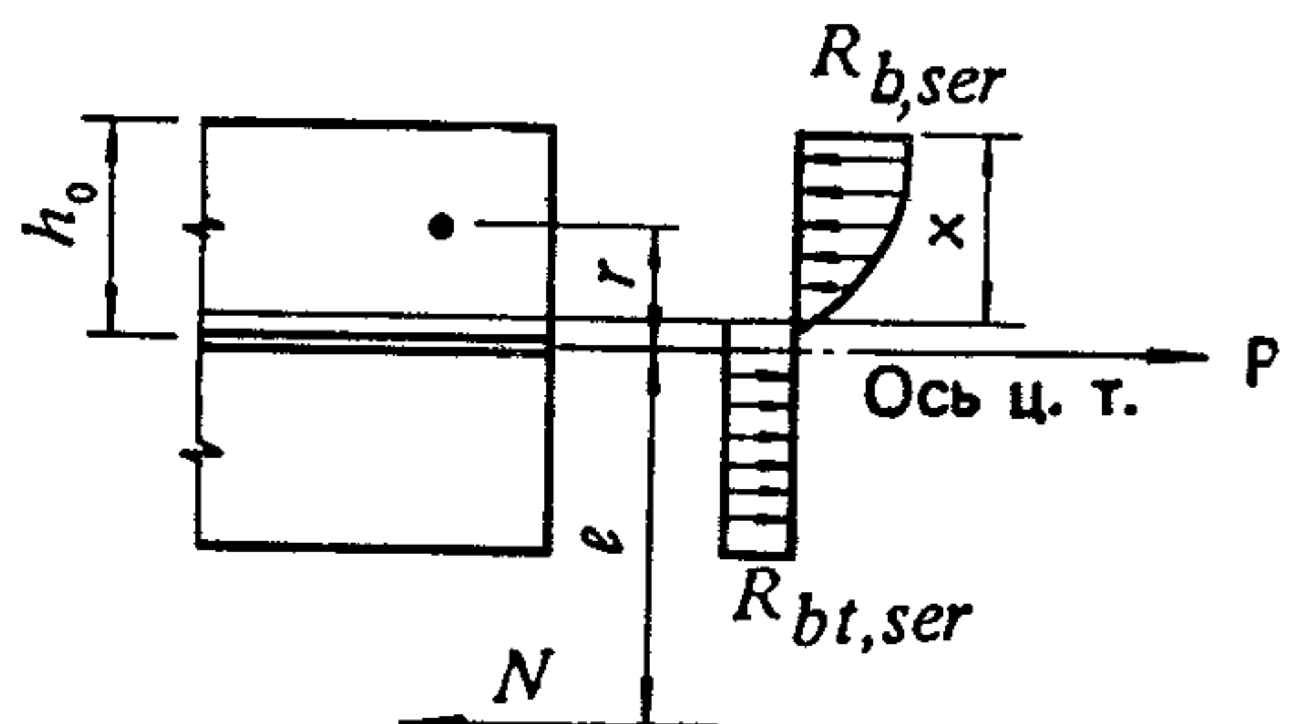
Черт. 2. Схема напряженного состояния сечения
