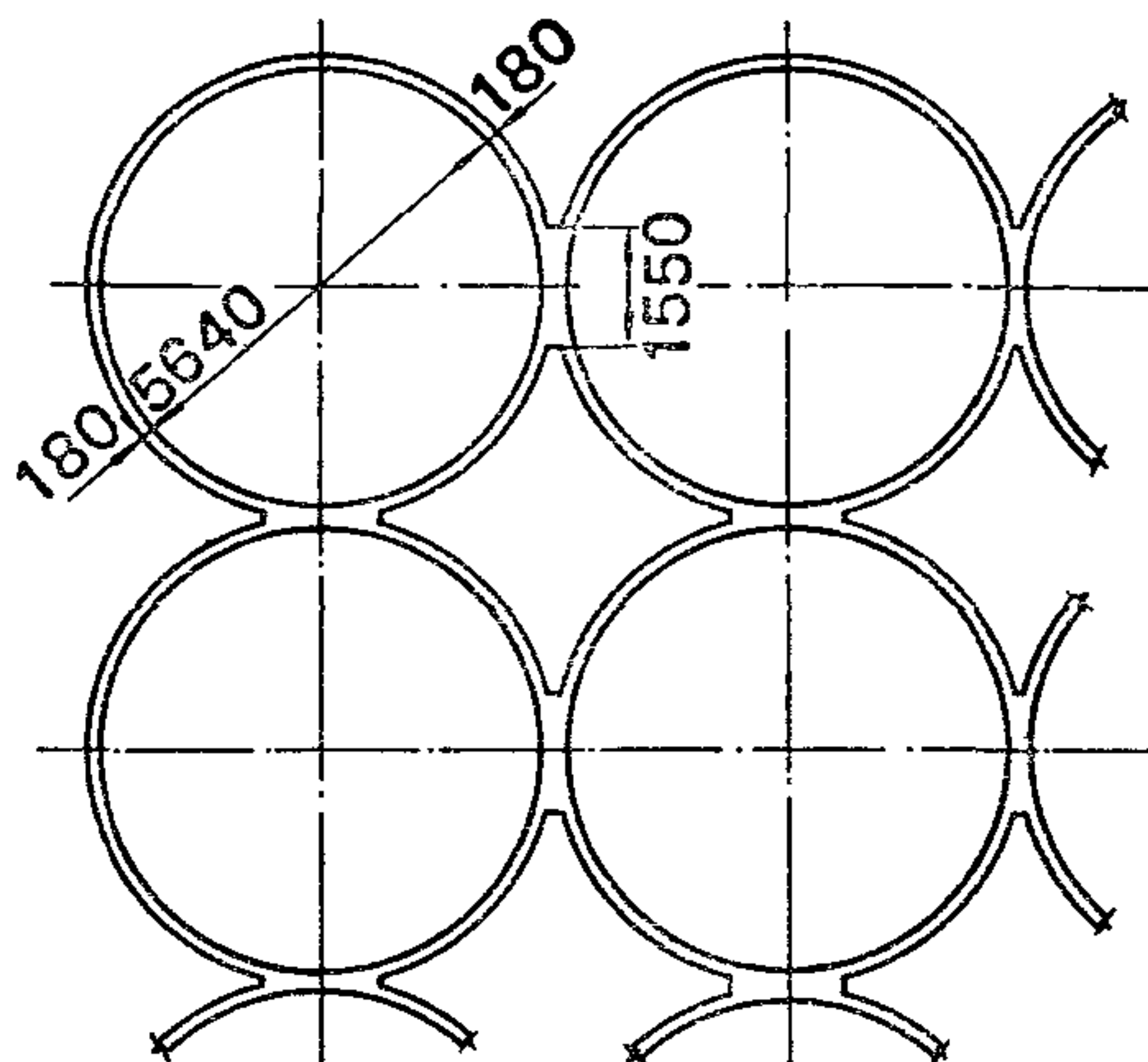
Черт. 3. План силосного корпуса с круглыми силосами
