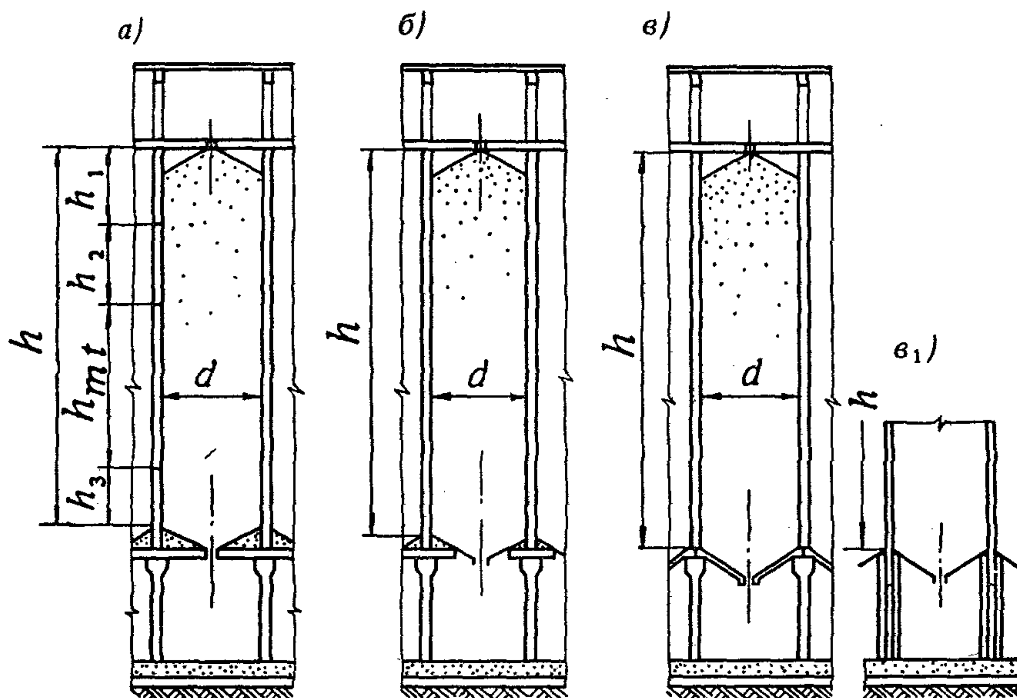
Черт. 1. Разрезы силосов
