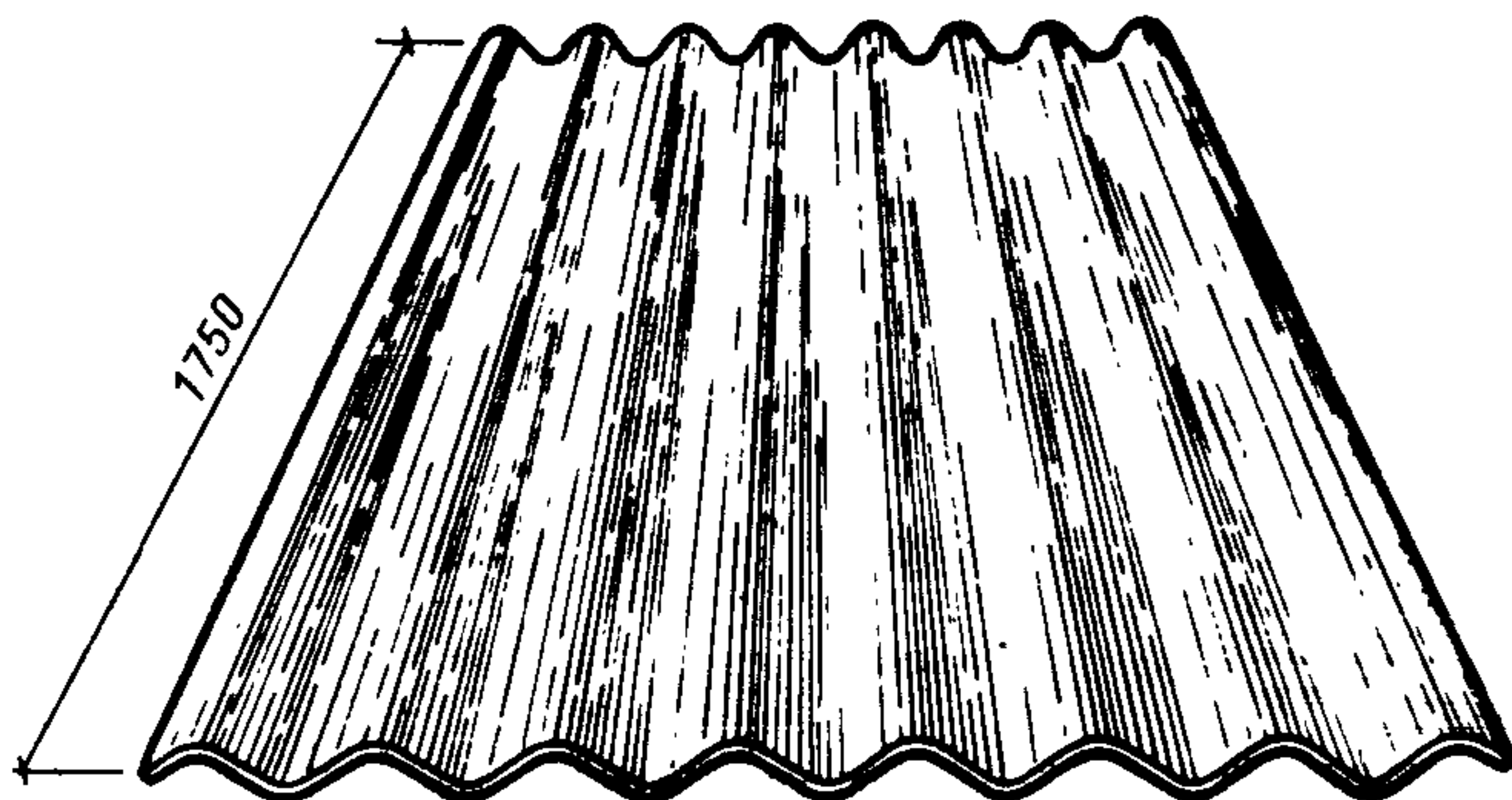
Рис. 1. Асбестоцементные волнистые листы среднего профиля 40/150
