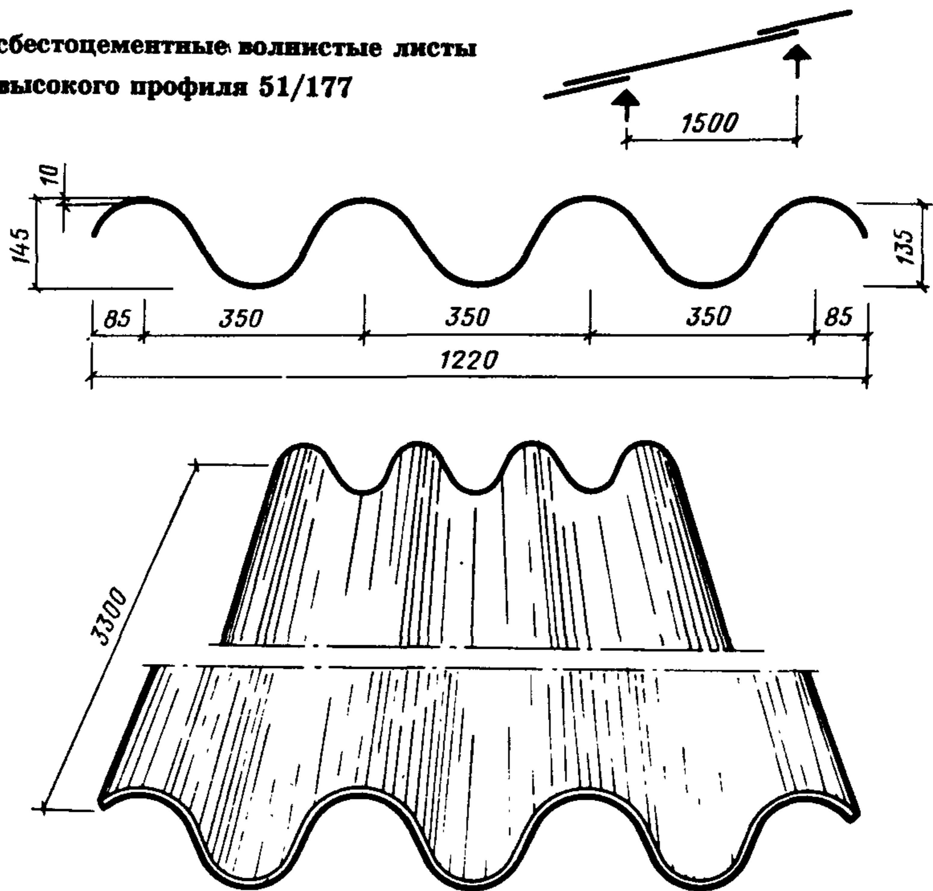
Рис. 4. Асбестоцементные волнистые листы ВК
