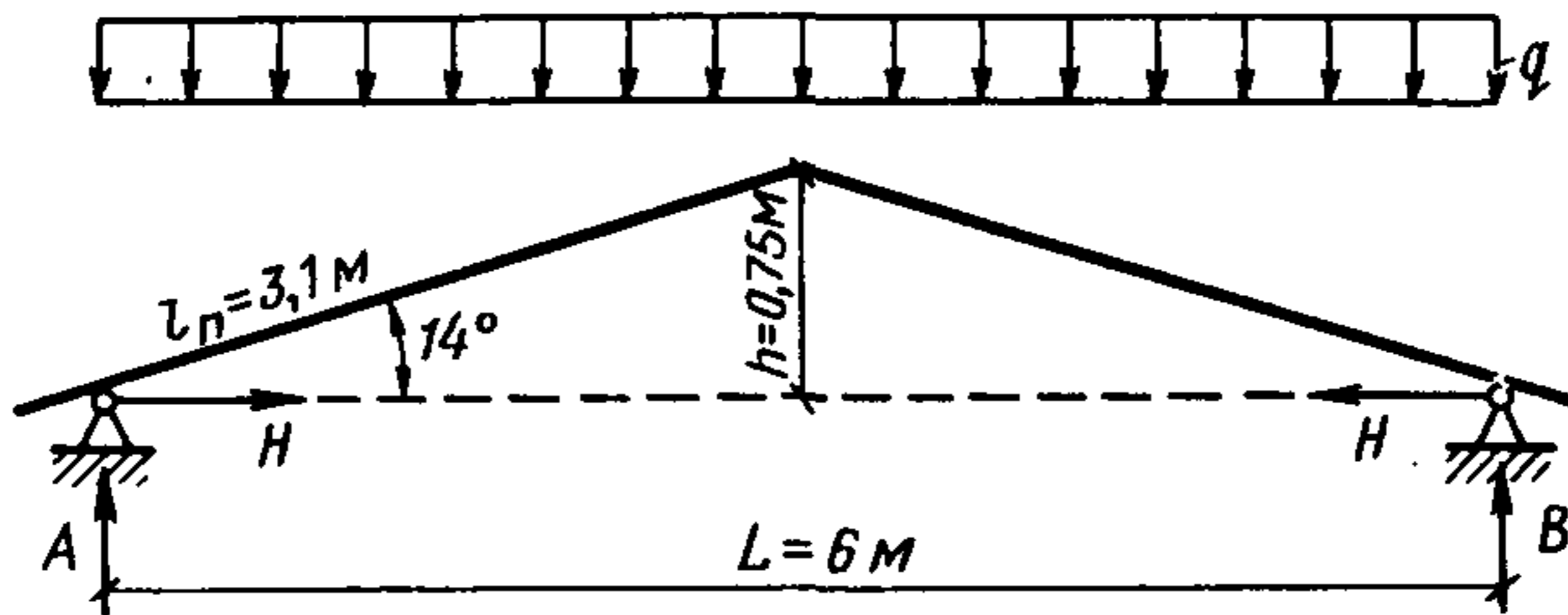
Рис. 14. Расчетная схема крыши
