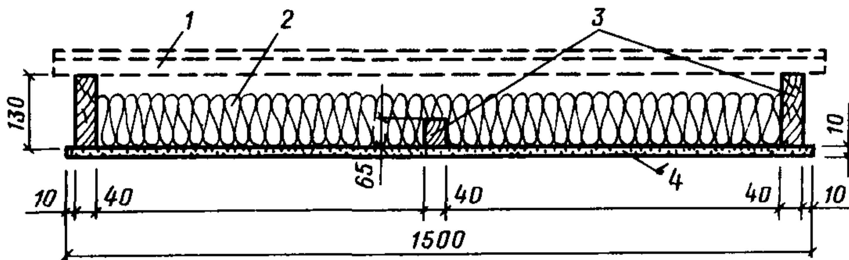
Рис. 1. Поперечное сечение плиты
