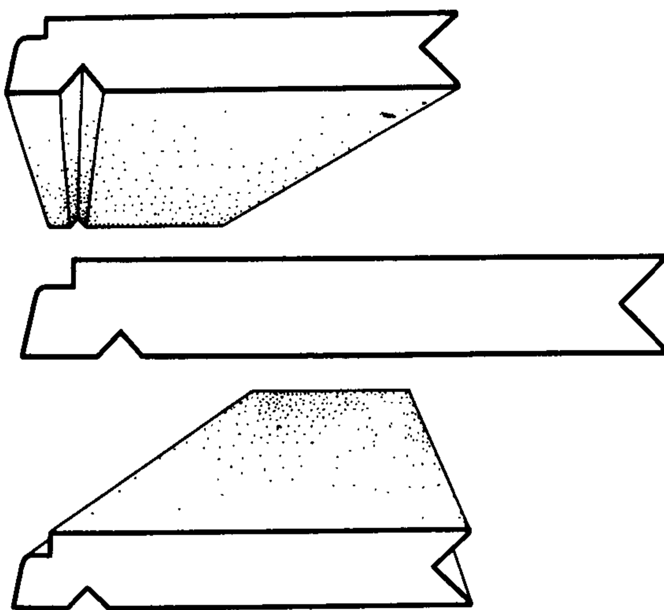
Рис. 6. Асбестоцементные экструзионные подоконные плиты
