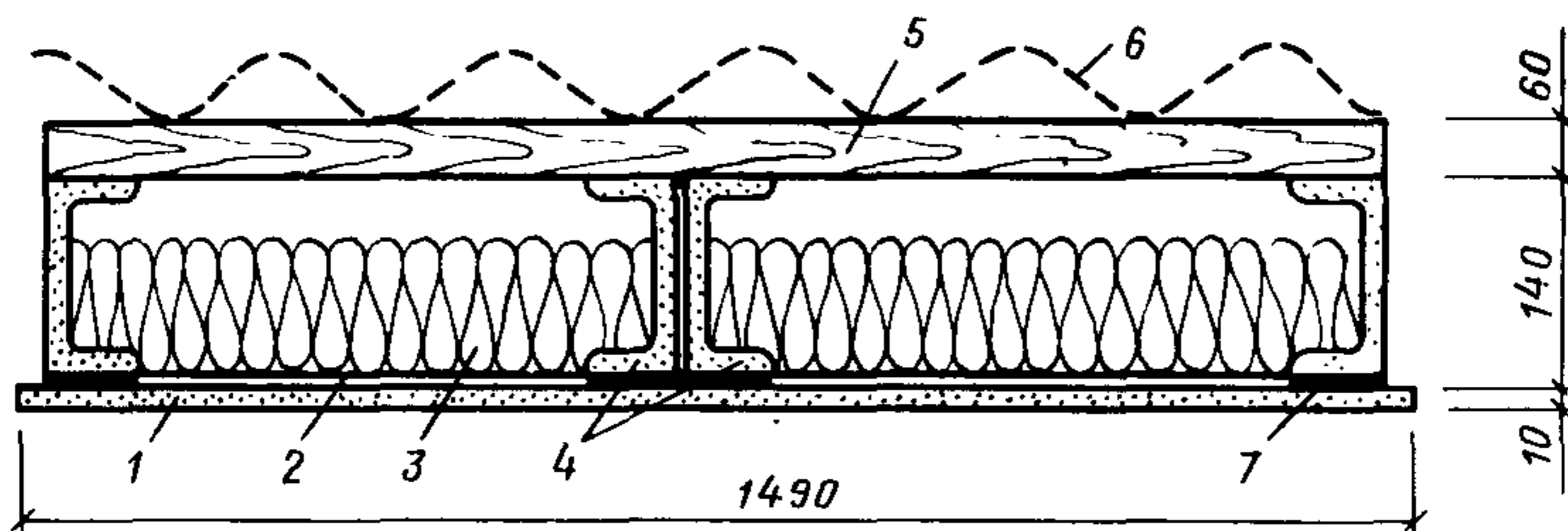
Рис. 4. Поперечный разрез плиты
