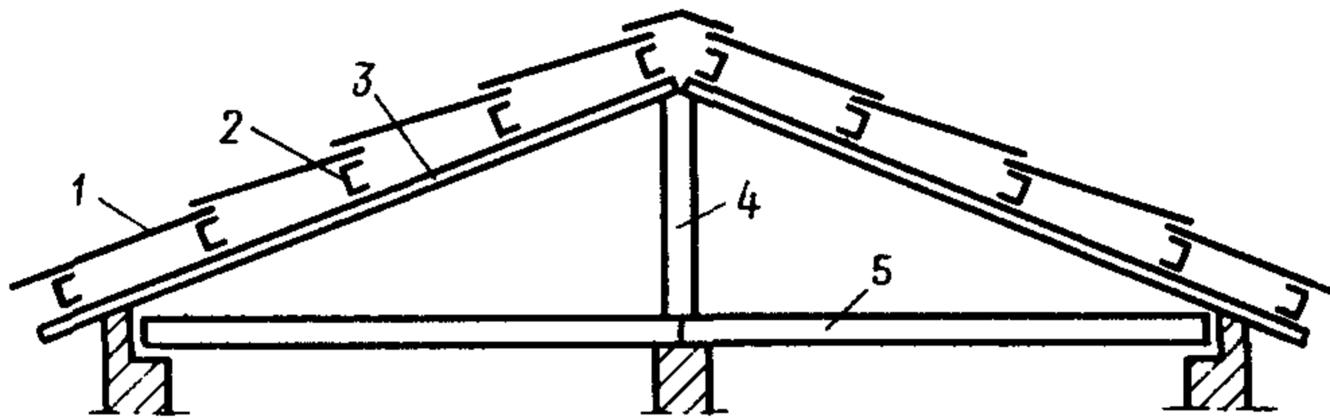
Рис. 10. Поперечный разрез крыши
