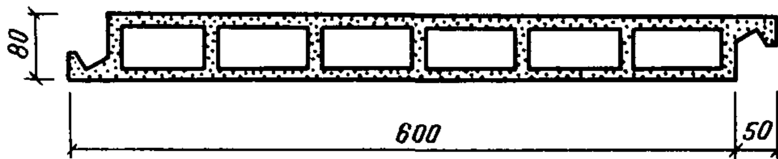
Рис. 13. Поперечное сечение плиты
