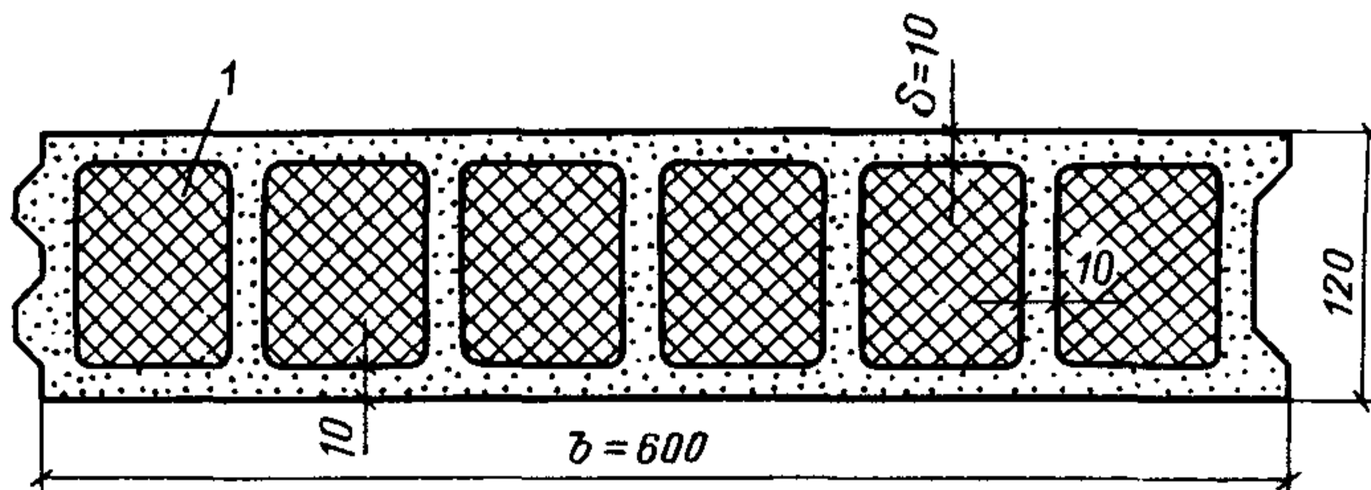
Рис. 8. Поперечное сечение экструзионной панели 1 -- утеплитель
