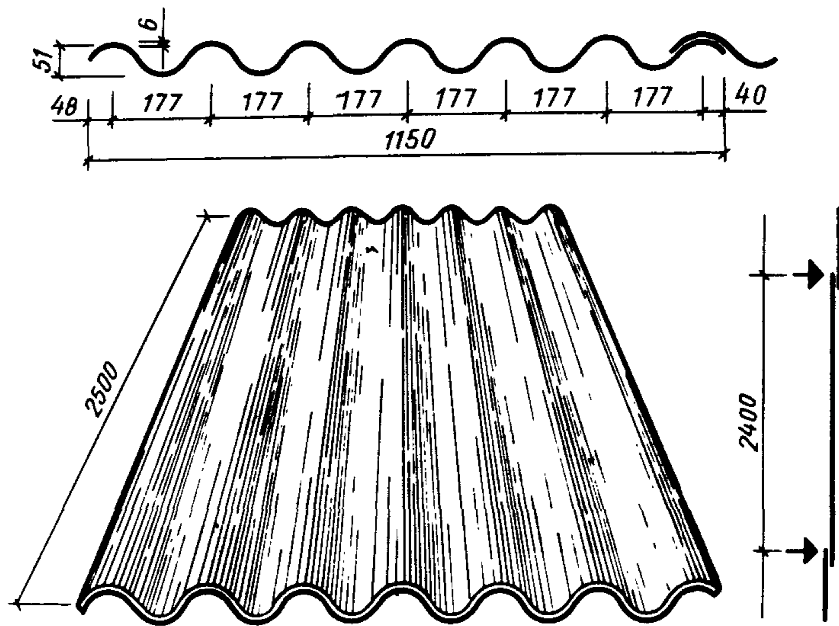
Рис. 3. Асбестоцементные волнистые листы высокого профиля 51/177
