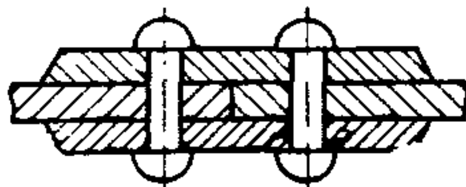
Чертеж 4
