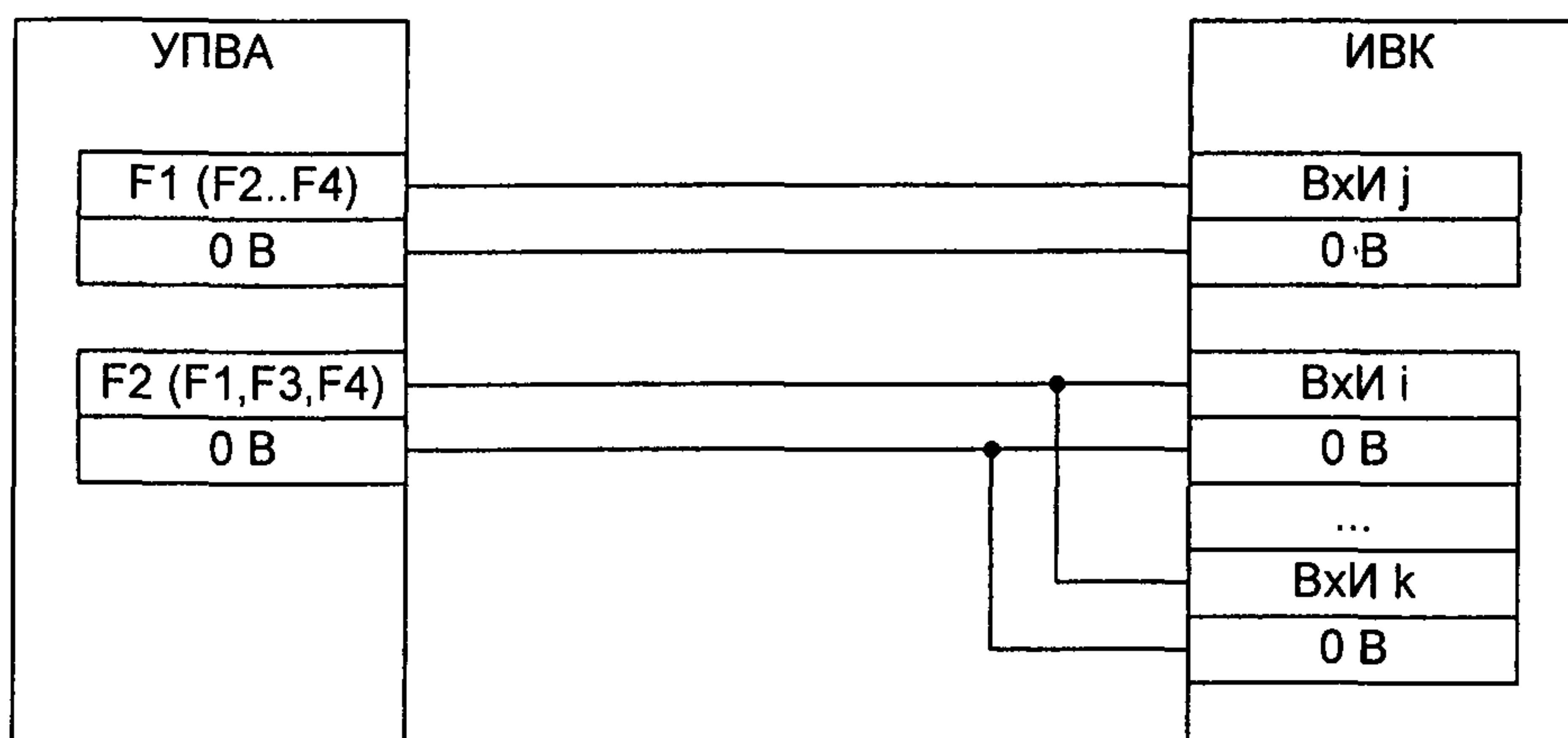
Рисунок А.6 - Схема подключения для определения погрешности ИБК при измерении отношения количества импульсов за интервал времени (несколько ЭПР (КПР))
