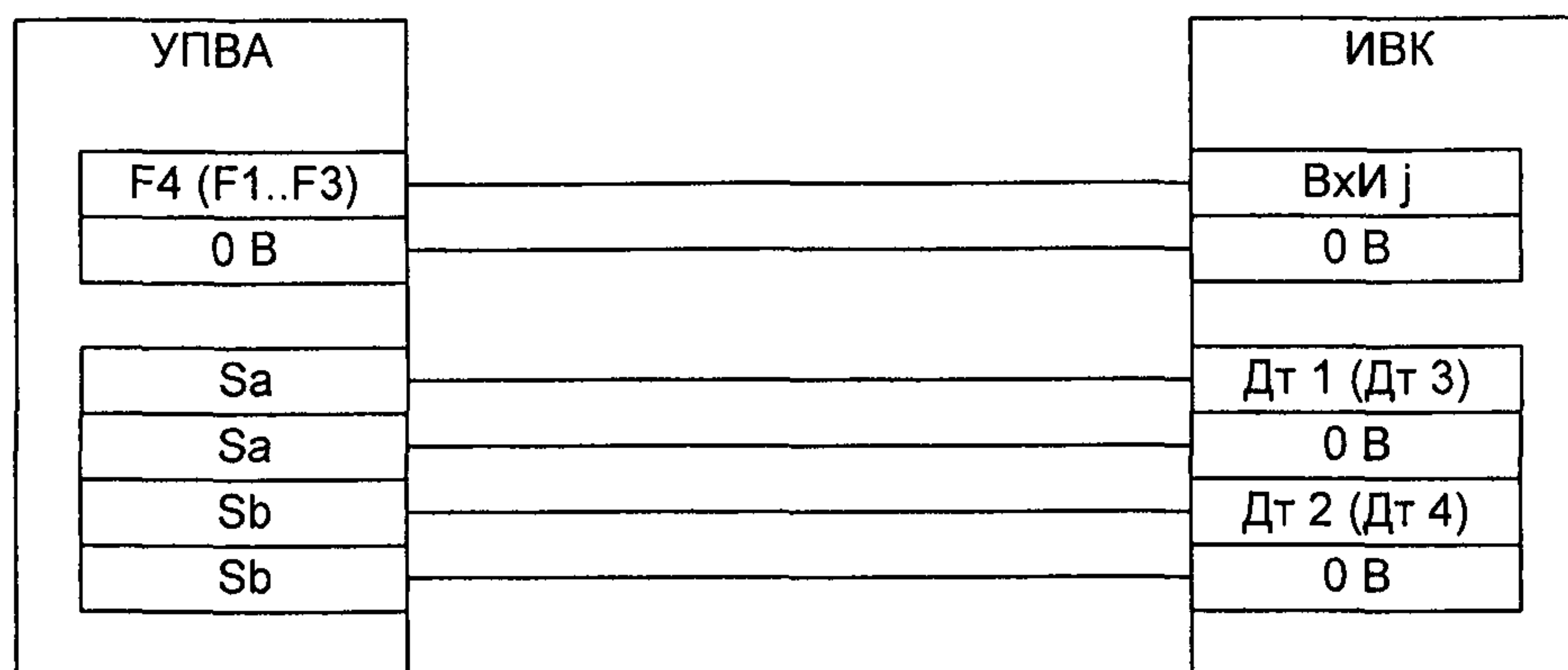
Рисунок А.4 - Схема подключения для определения погрешности ИБК при измерении количества импульсов за интервал времени
