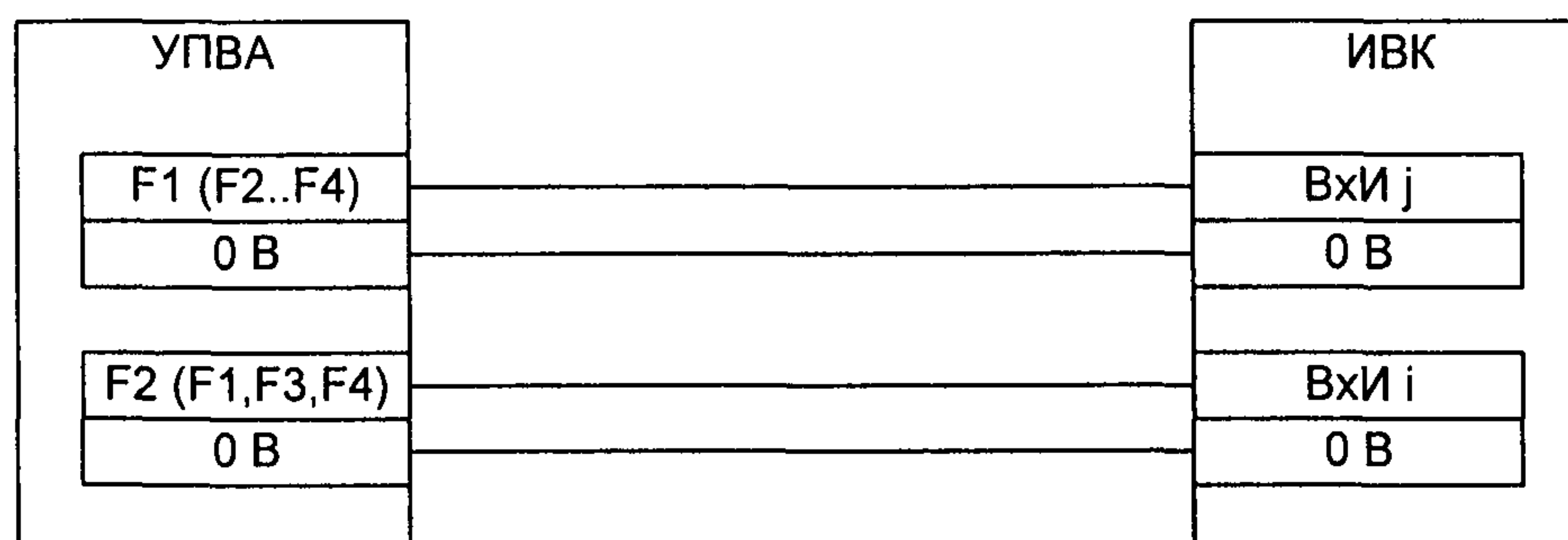
Рисунок А.5 - Схема подключения для определения погрешности ИБК при измерении отношения количества импульсов за интервал времени (один ЭПР (КПР))
