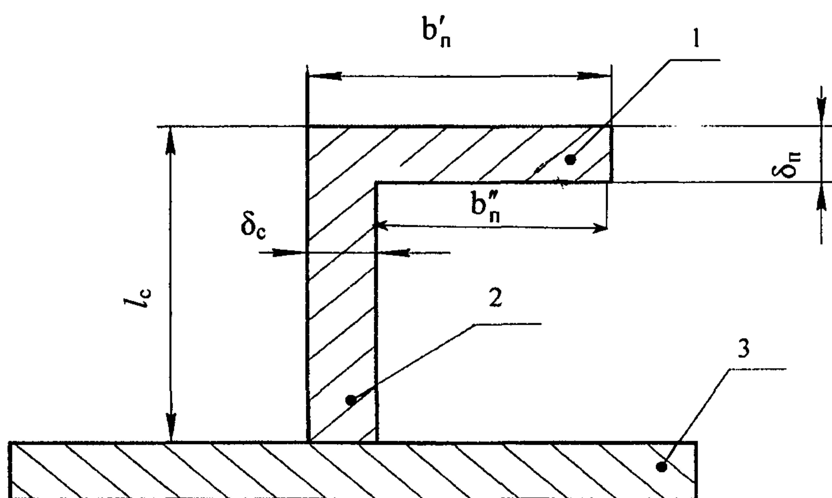
Рисунок А.13 – Рамный набор (отфланцовый профиль).
