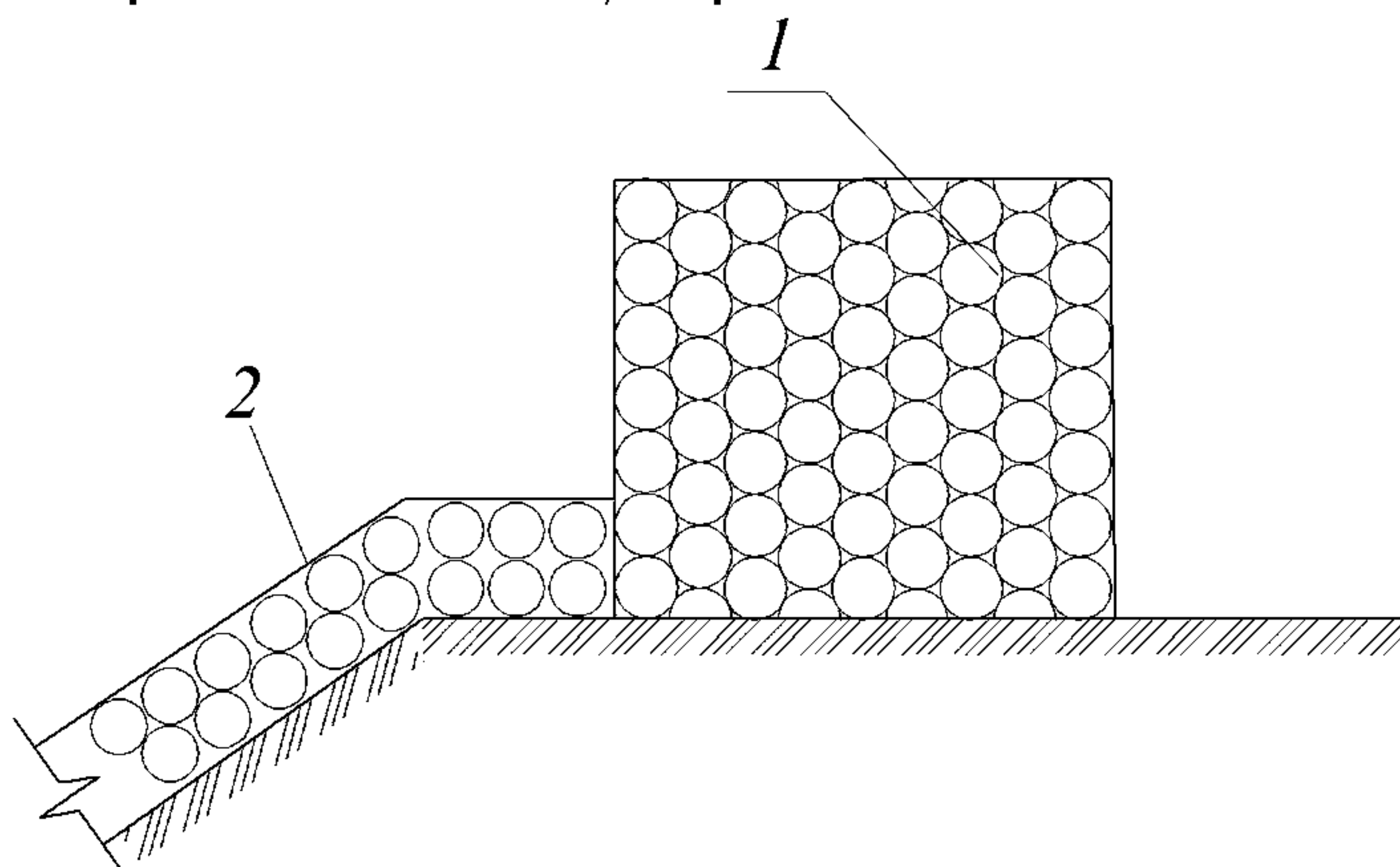
Рисунок 11 – Пример исполнения упорного элемента габионного сооружения
