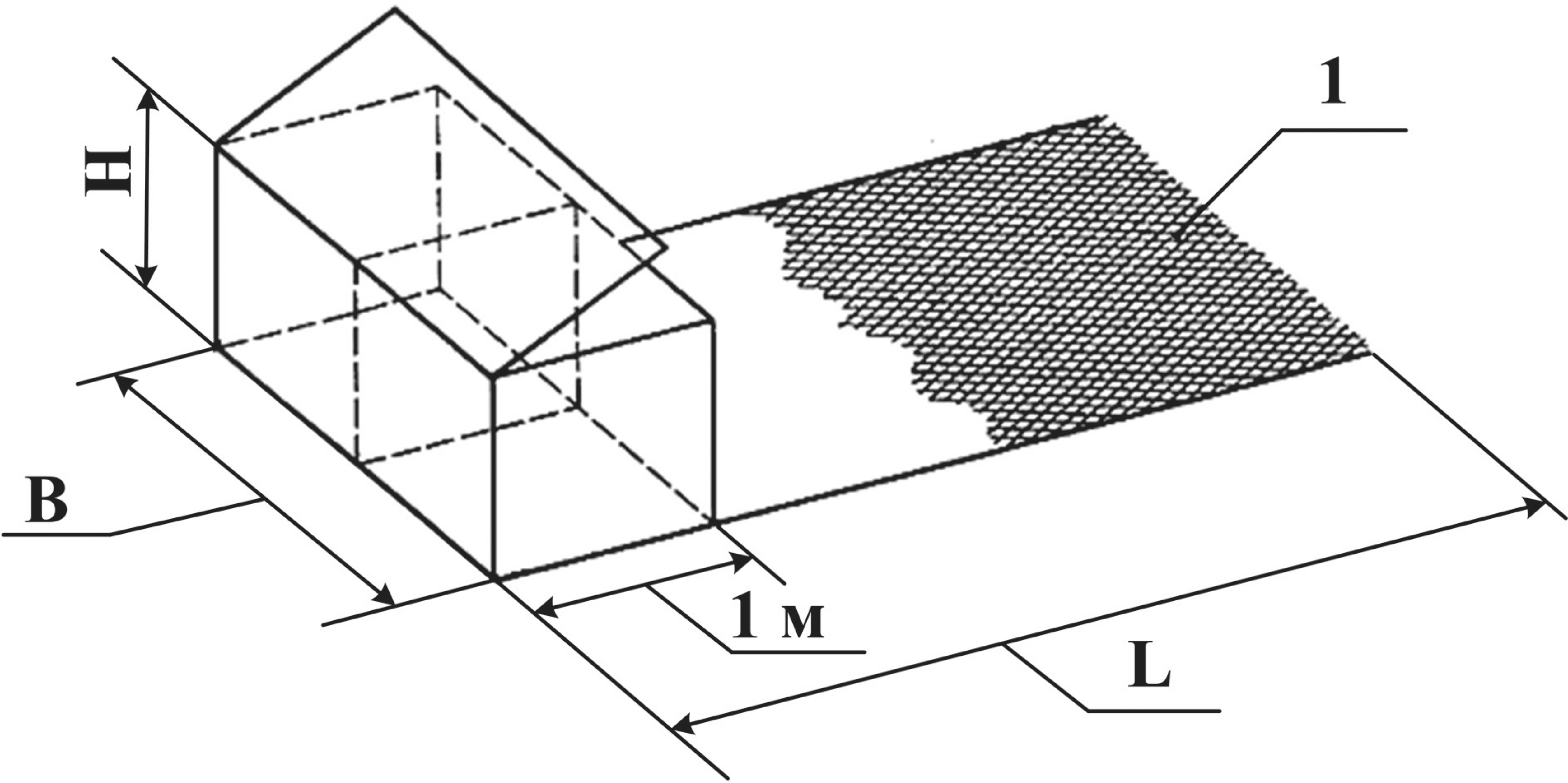
B – ширина короба и армирующей панели; L – длина армирующей панели; H – высота короба; l – армирующая панель
