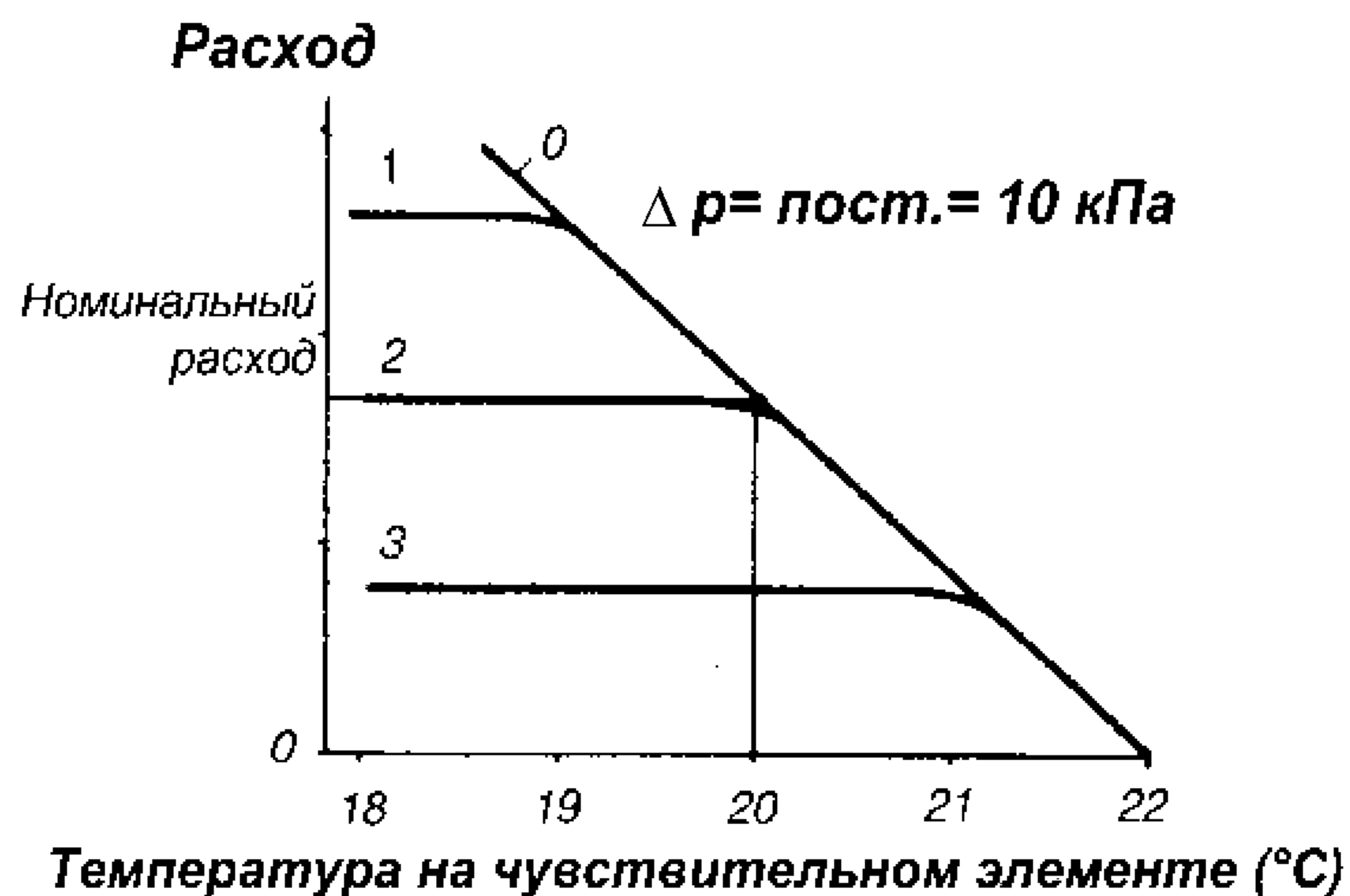
Рисунок 7.9 – Характеристики открытия термостатического вентиля с регулировкой путем ограничения хода при различных настройках (кривые 0, 1, 2, 3)
