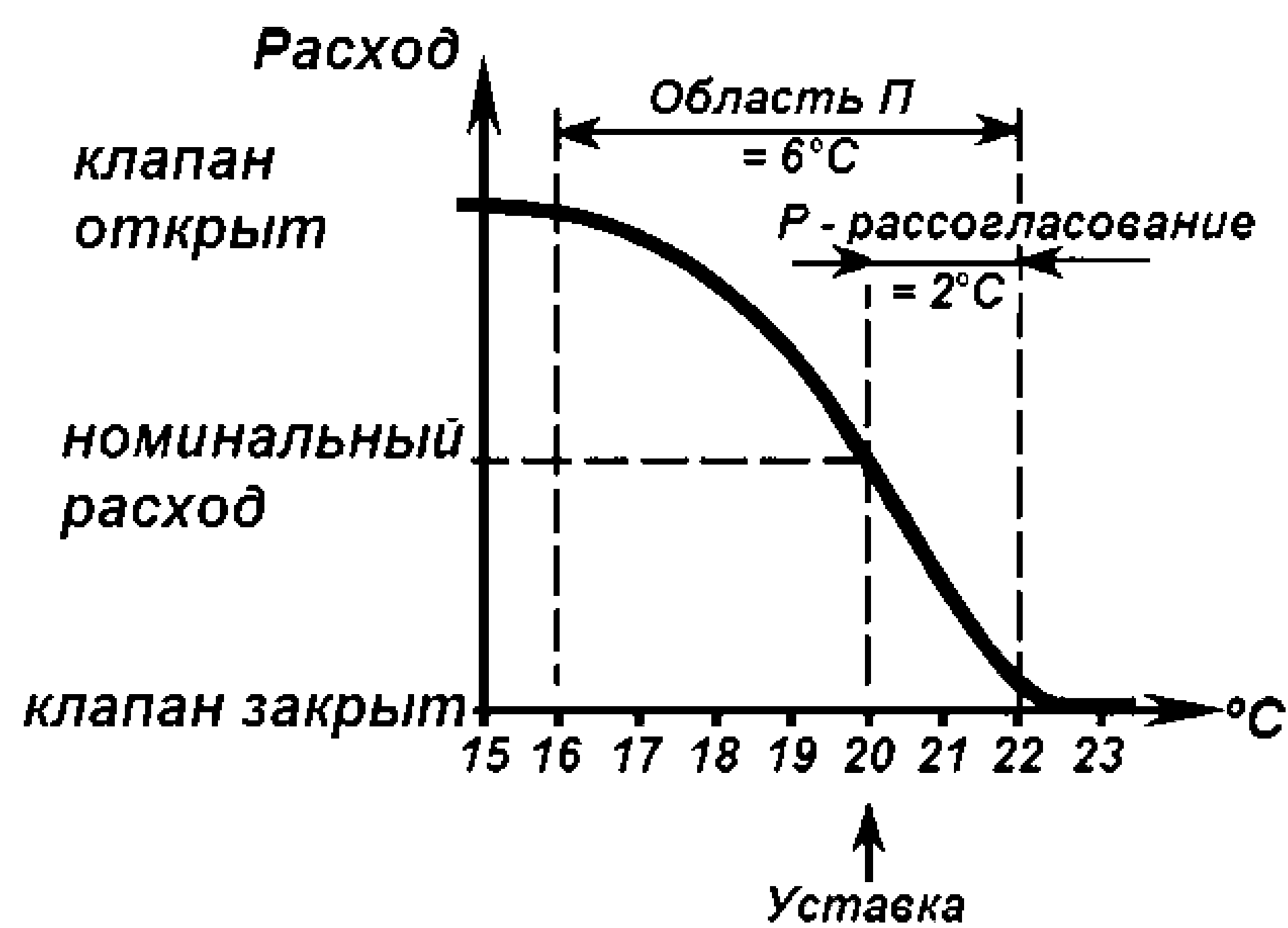
Рисунок 7.5 – Характеристика термостатического вентиля
