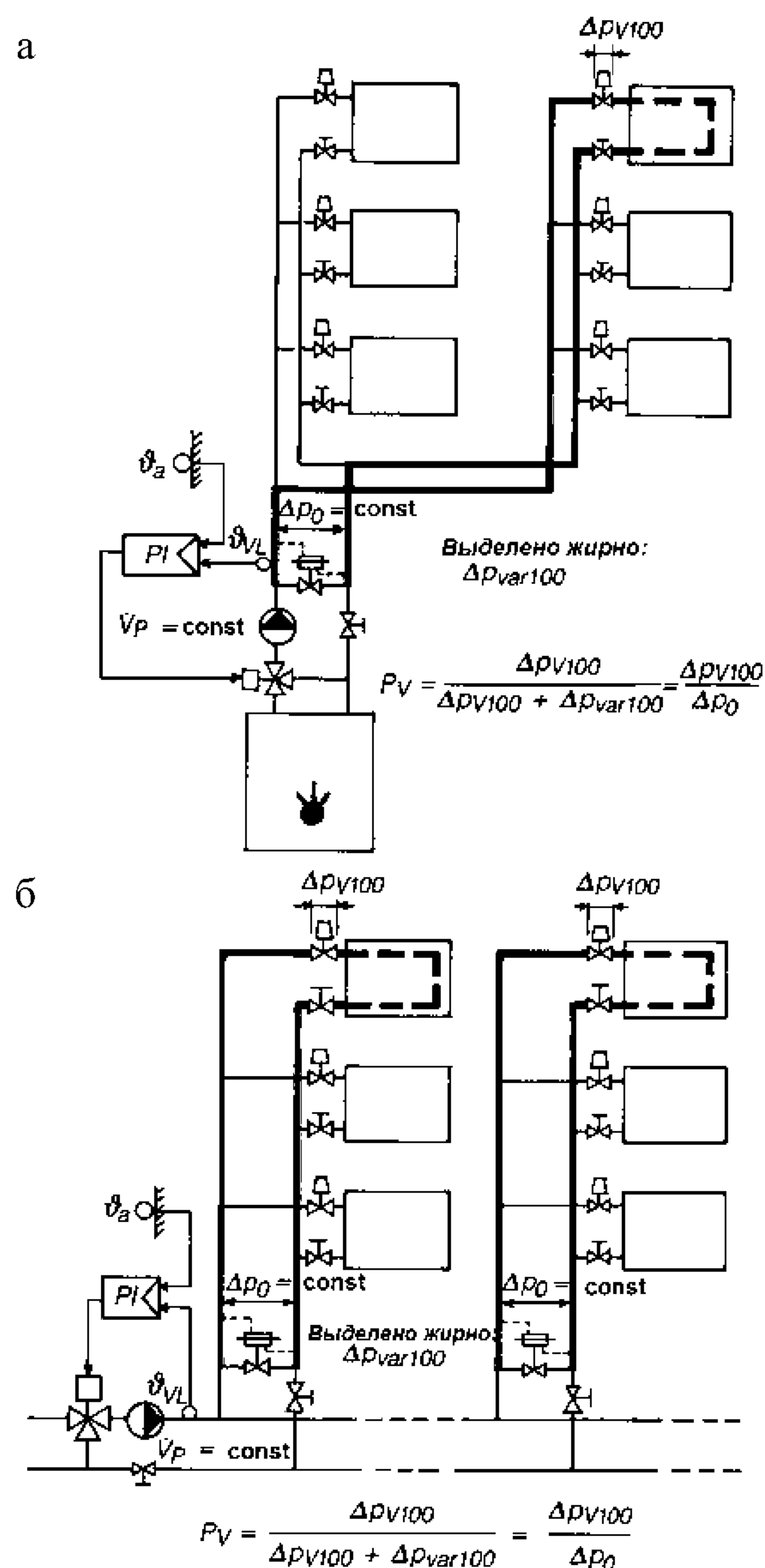
Рисунок 7.7 – Расчет авторитета клапана на примере 2-х систем
