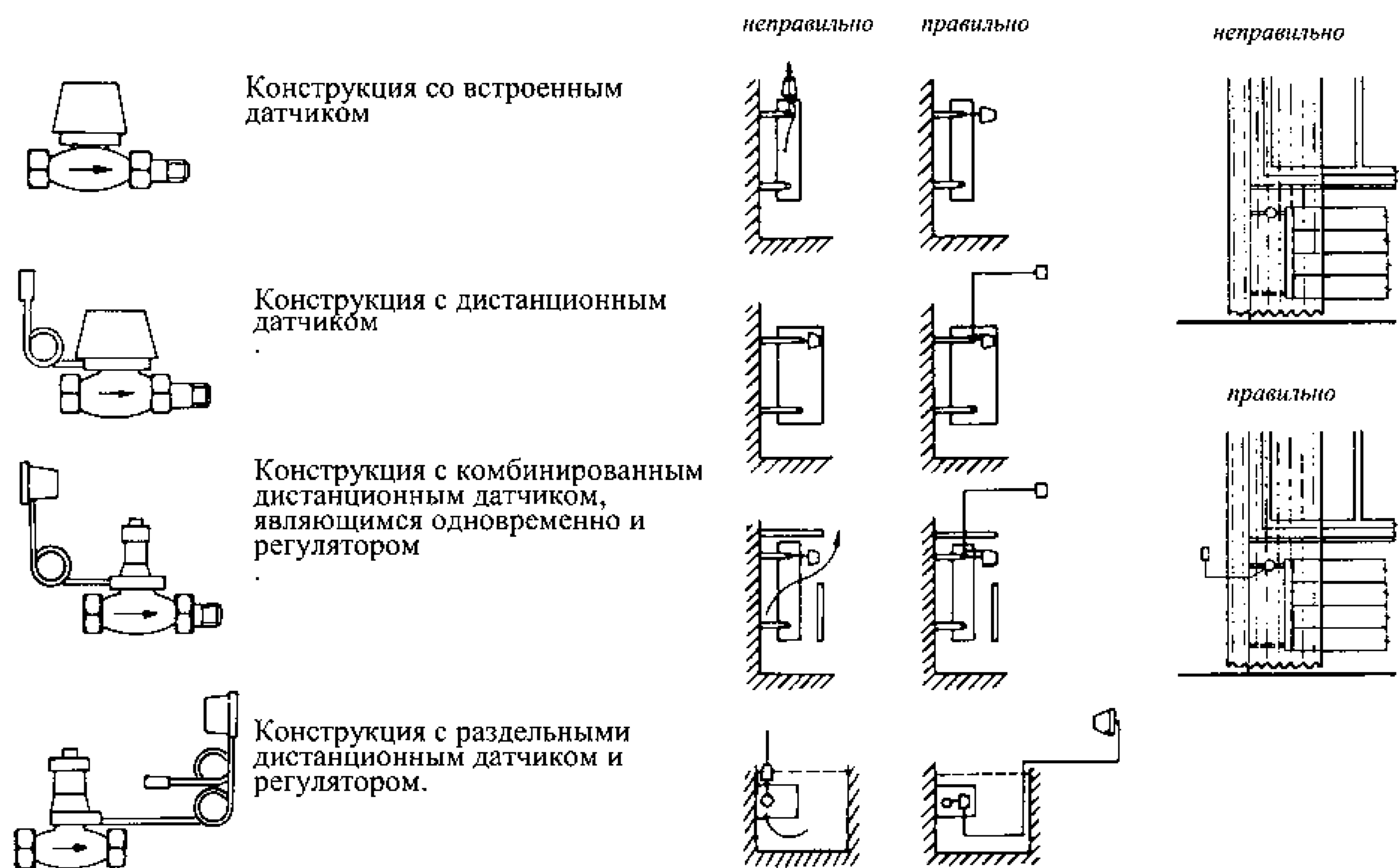
Рисунок 7.4 – Типы конструкции термостатического вентиля и варианты размещения датчика
