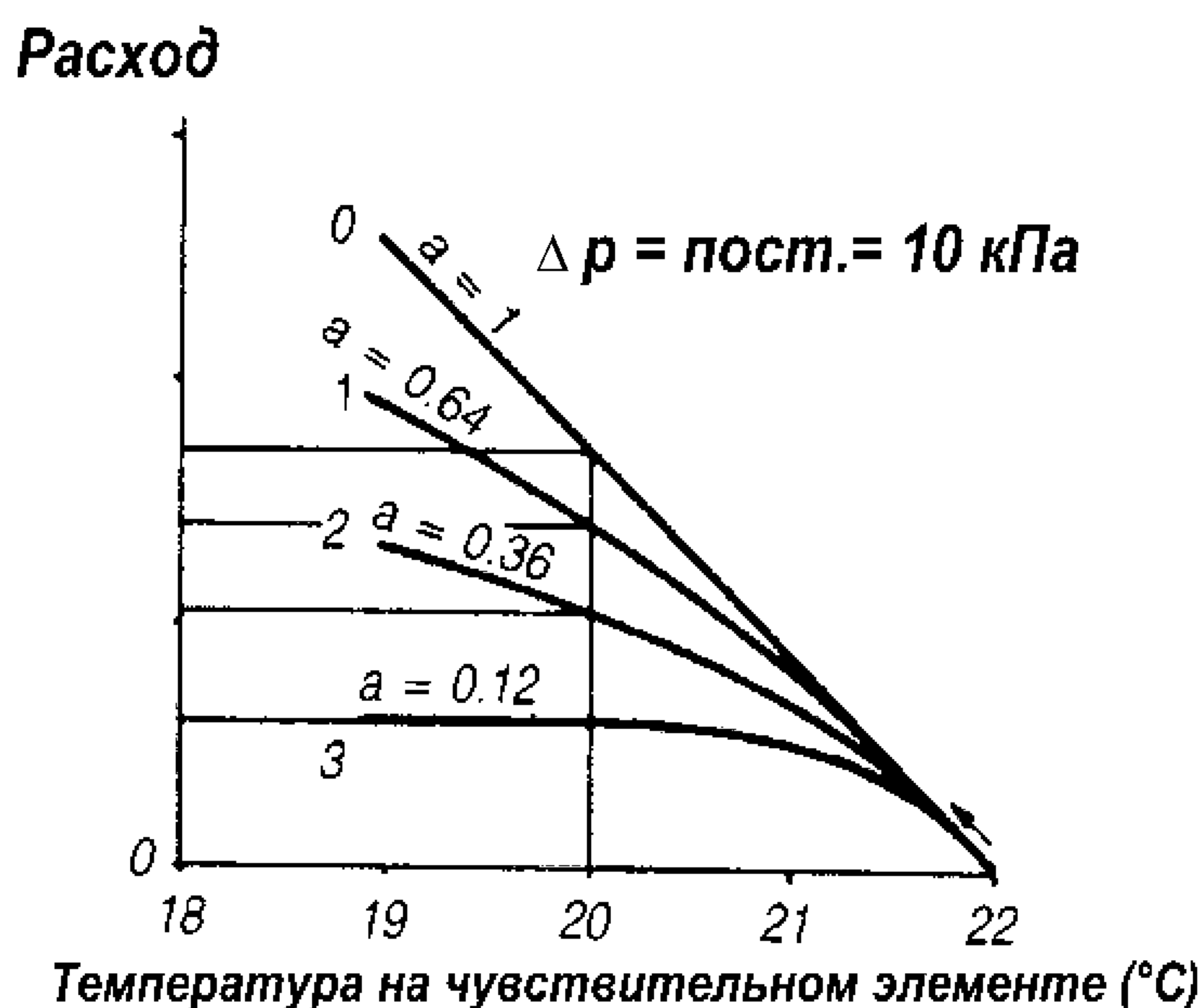
Рисунок 7.8 – Характеристики открытия термостатического клапана с регулировкой через дополнительное гидравлическое сопротивление при различных настройках (кривые 0, 1, 2, 3)
