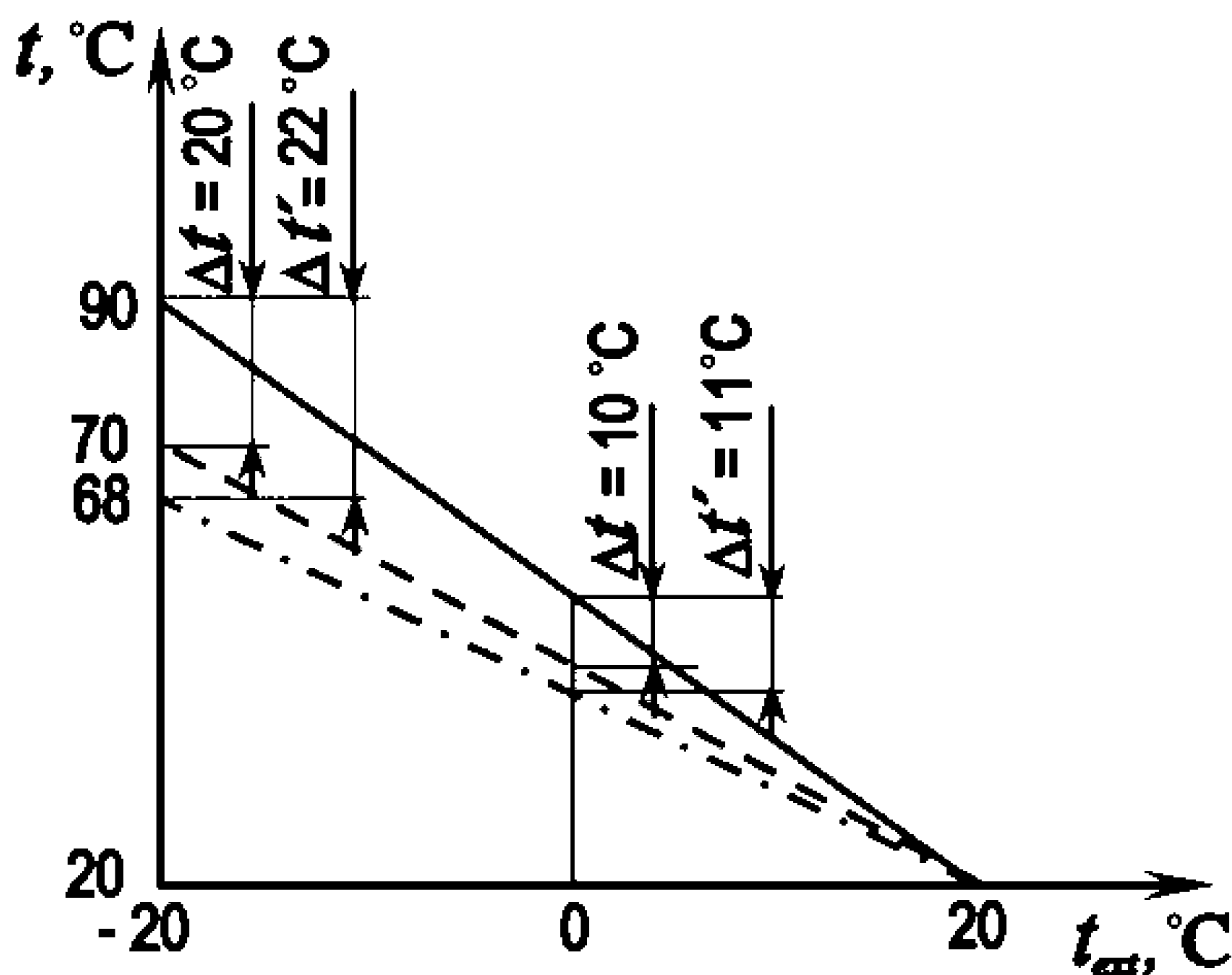
Рисунок Г.1 – Определение требуемого перепада теплоносителя в отопительном приборе
