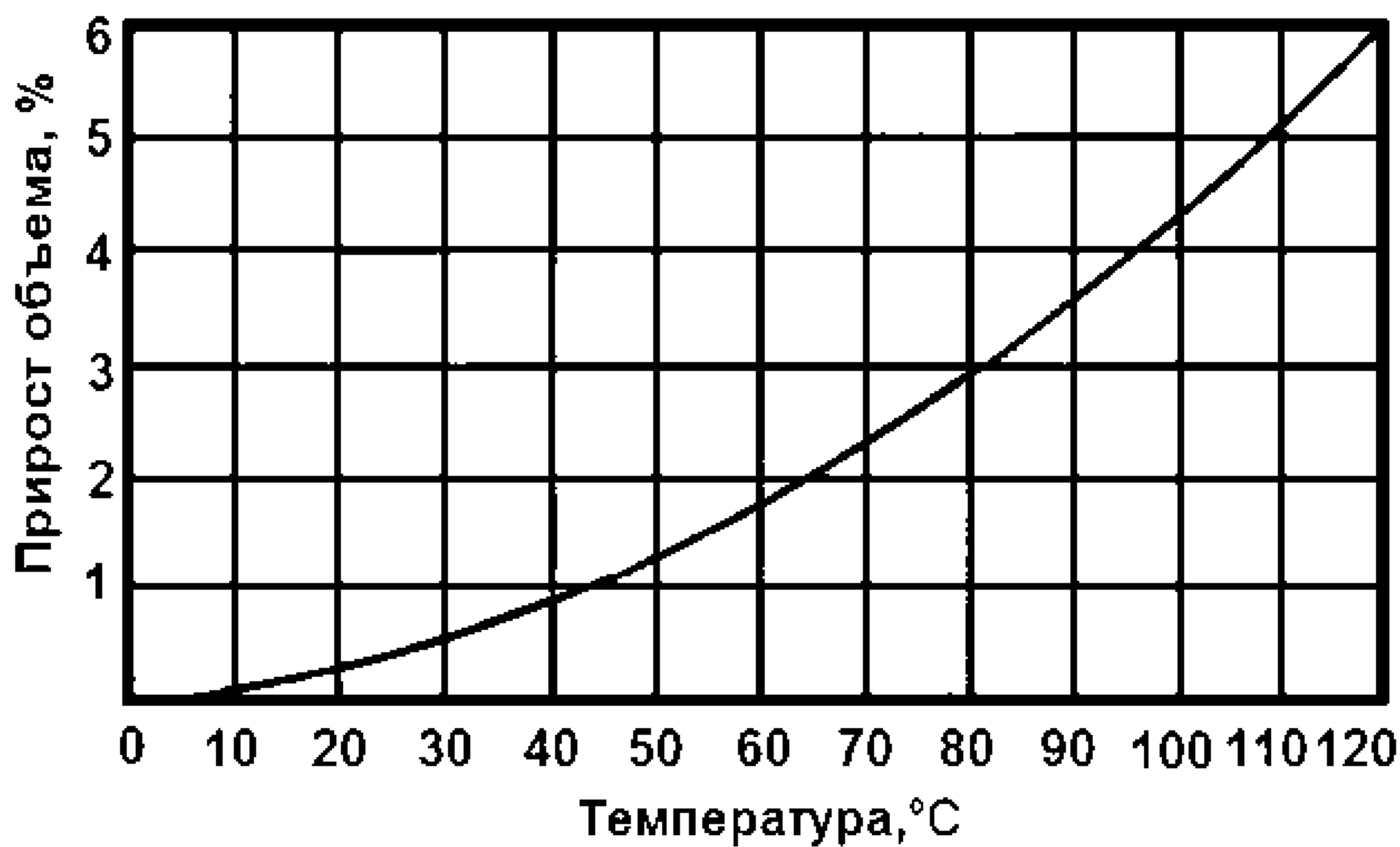
Рисунок 7.2 – Температурное расширение воды при ее нагреве (охлаждении) от 10 °С до средней температуры системы
