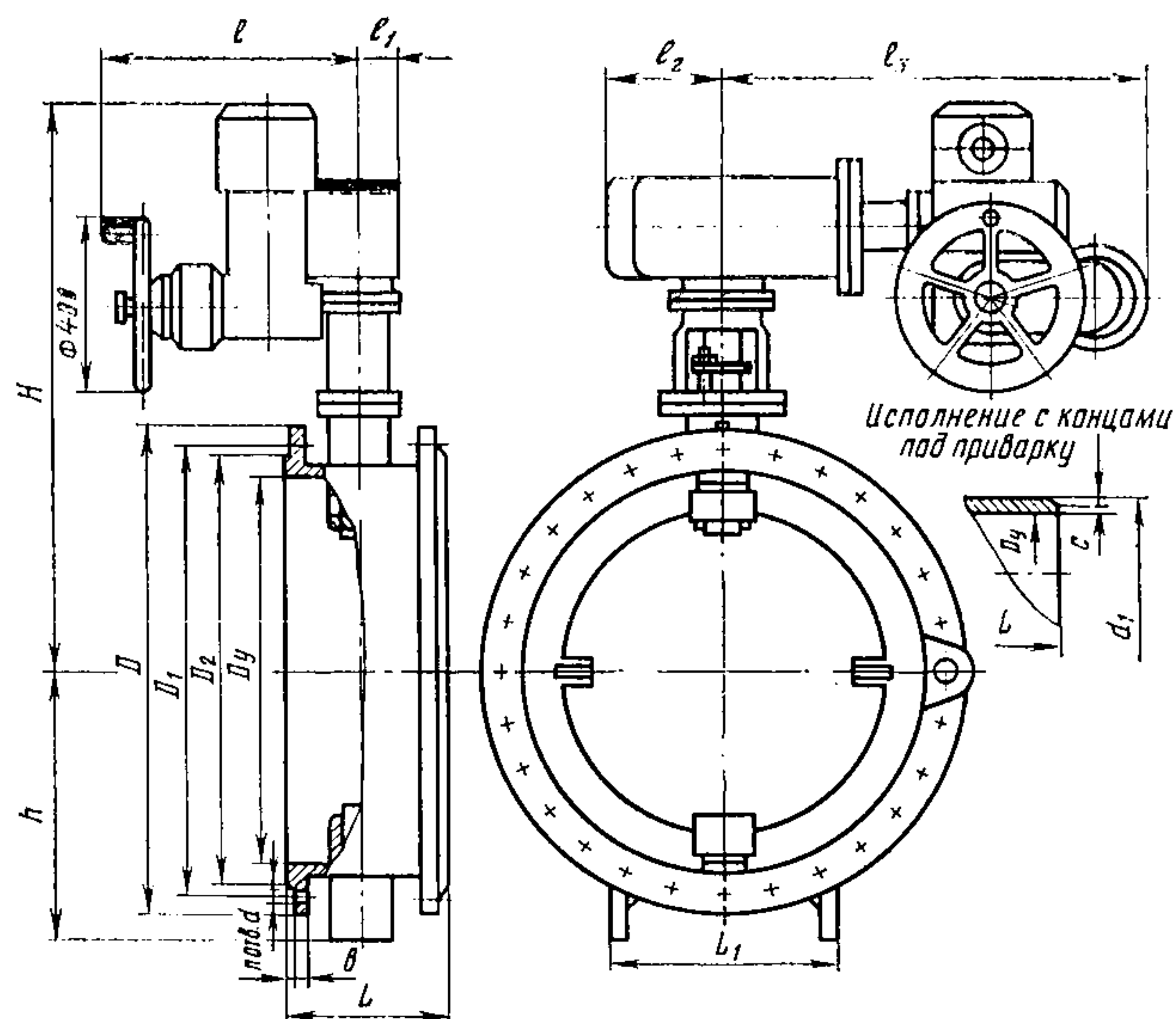
ОСНОВНЫЕ ГАБАРИТНЫЕ И ПРИСОЕДИНИТЕЛЬНЫЕ РАЗМЕРЫ (мм)
