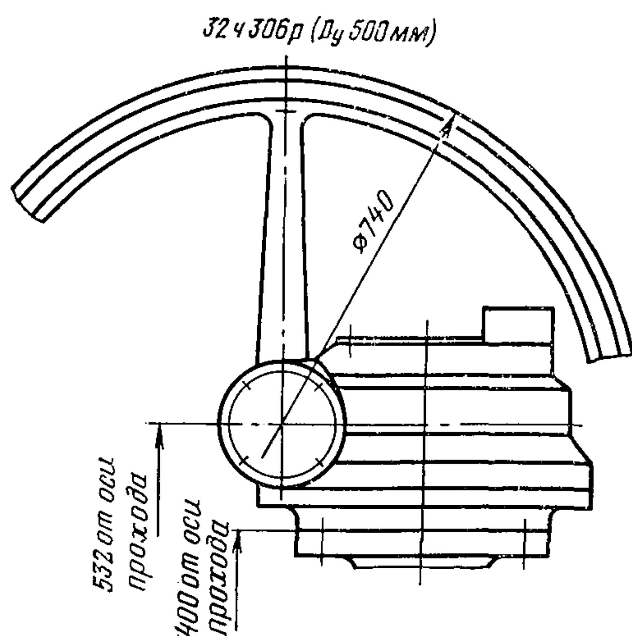
ОСНОВНЫЕ ГАБАРИТНЫЕ И ПРИСОЕДИНИТЕЛЬНЫЕ РАЗМЕРЫ (мм)
