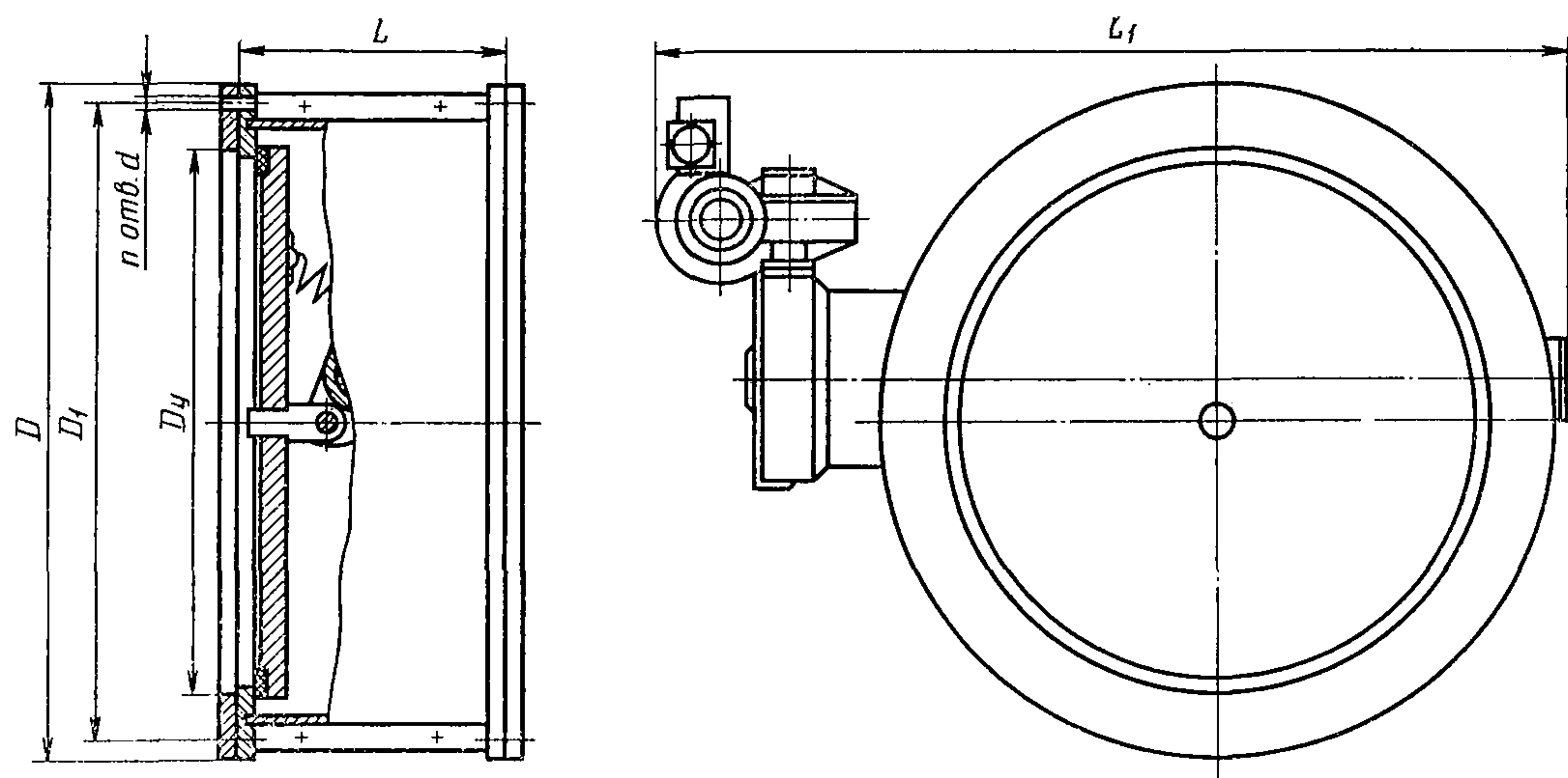
Клапан 19с941нж ( D_y 800 мм)
