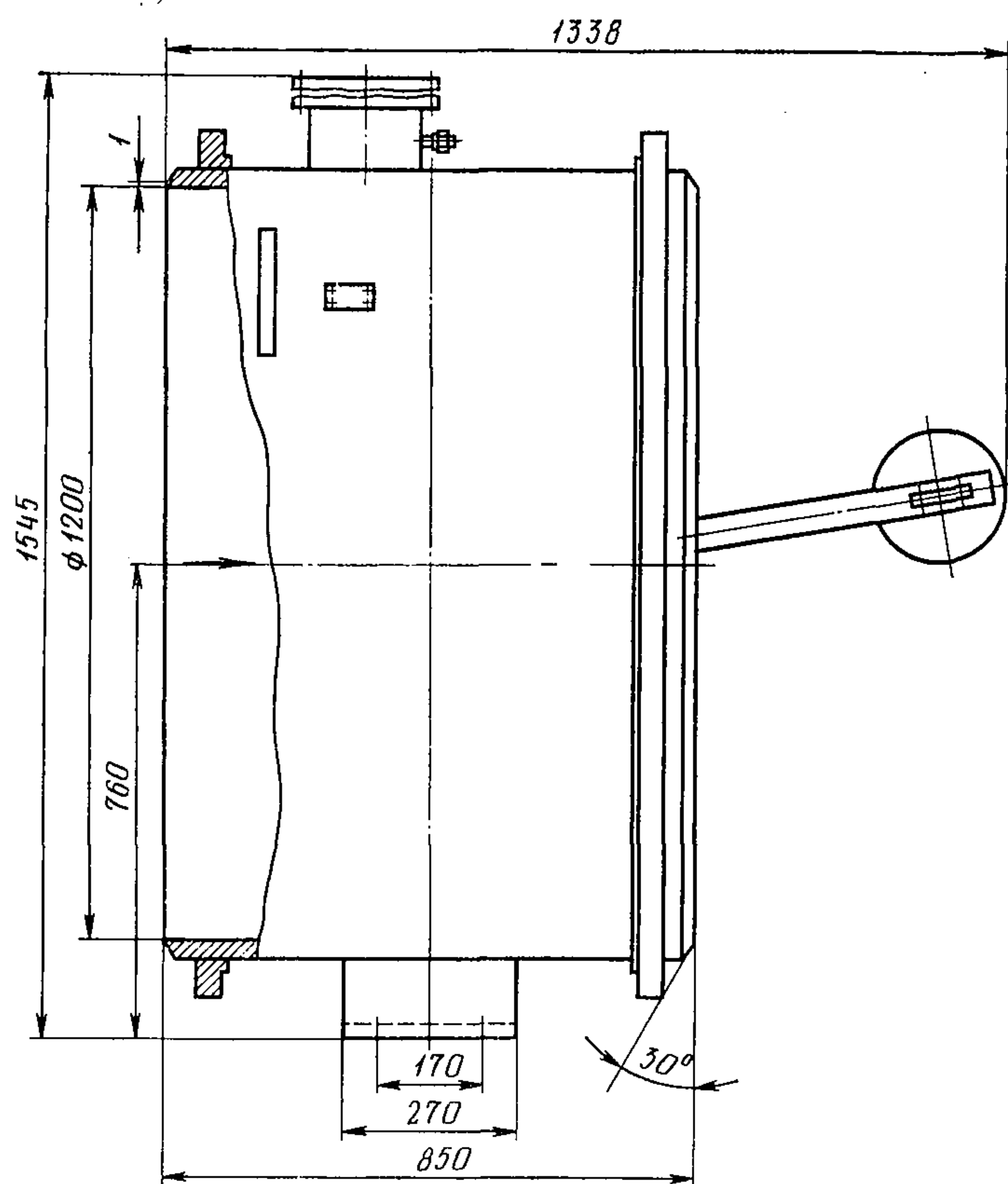
Исполнение с концами под приварку
