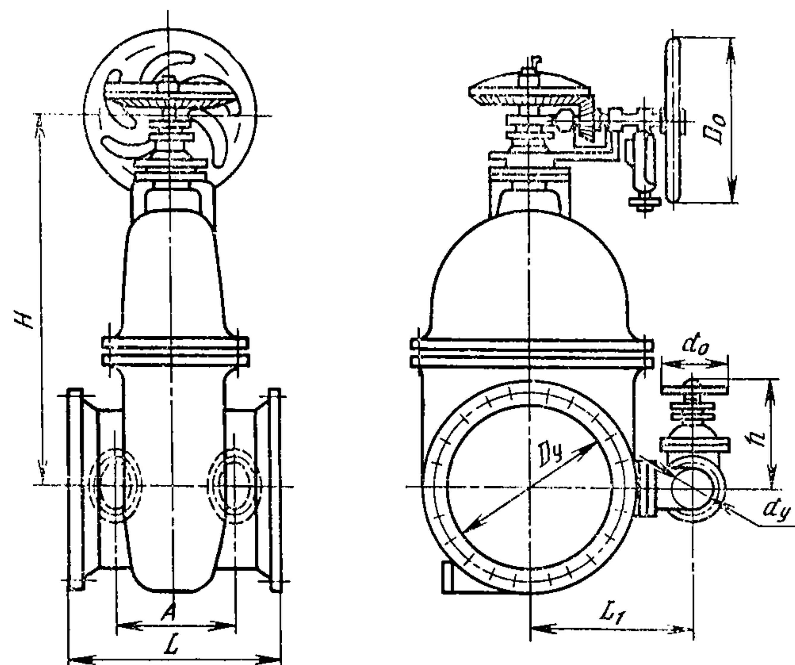
Управление ручное, маховиком через конический редуктор
