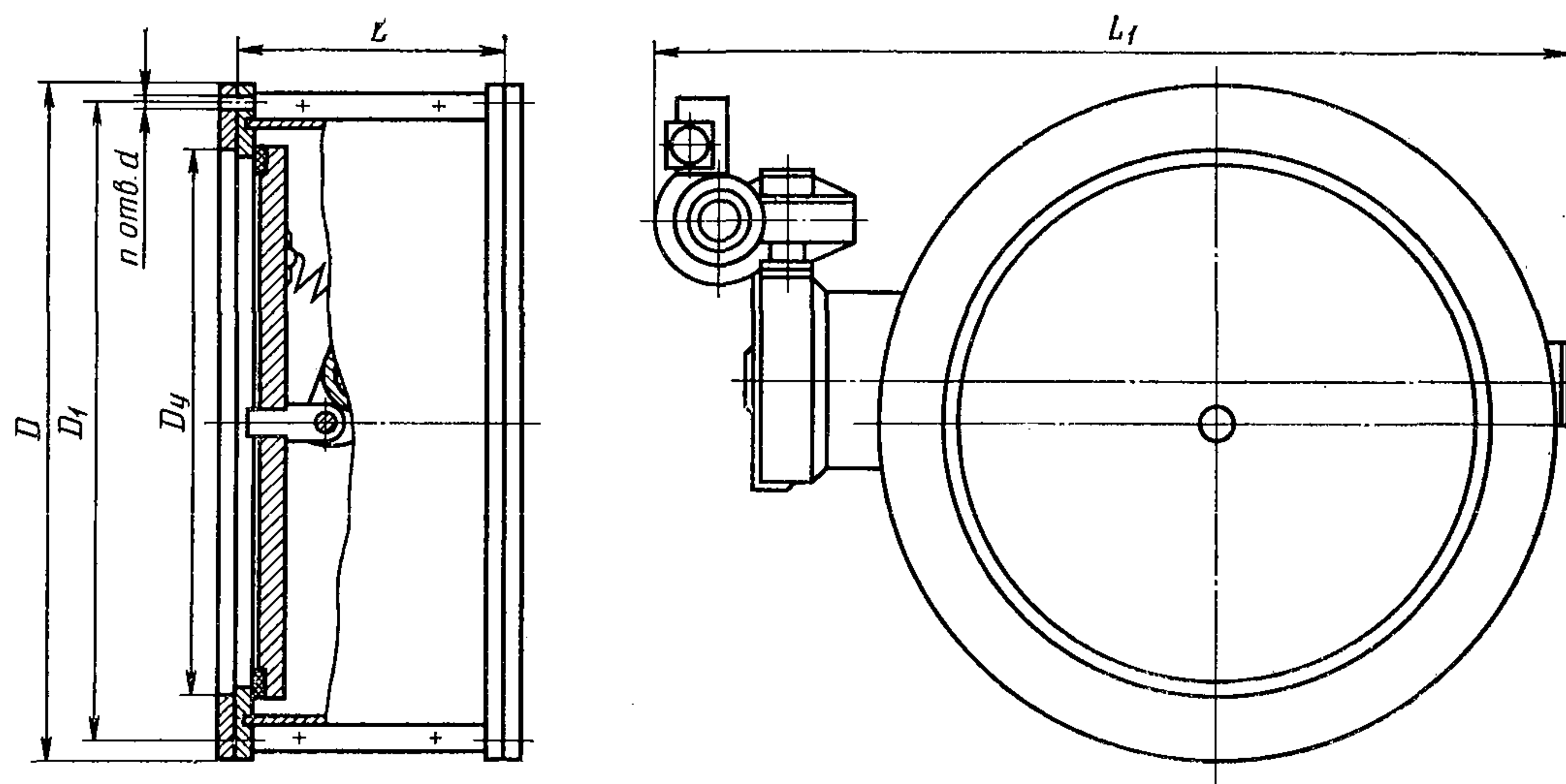
Клапан ИА 01009 ( D_y 600, 800, 1000 и 1200 мм)
