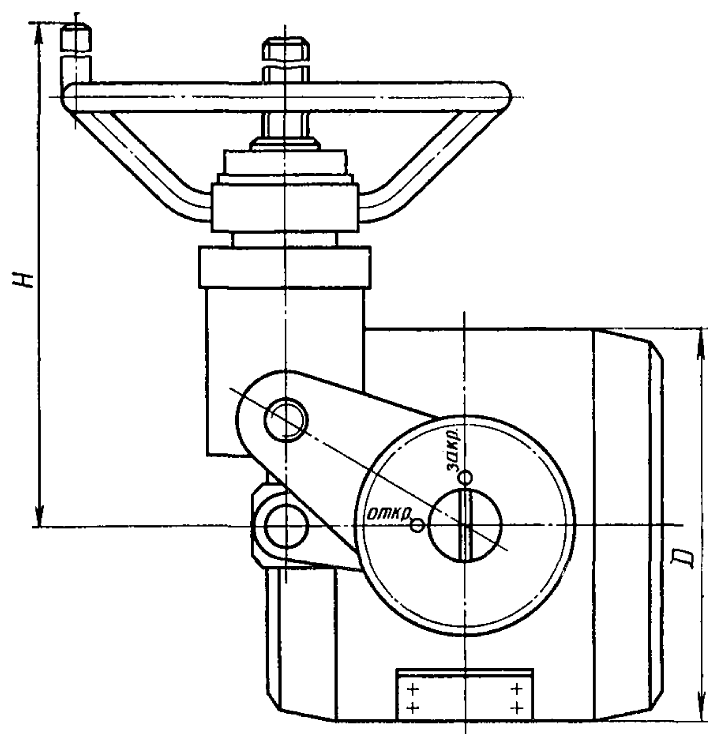
Исполнение с ручным управлением (32с30р)
