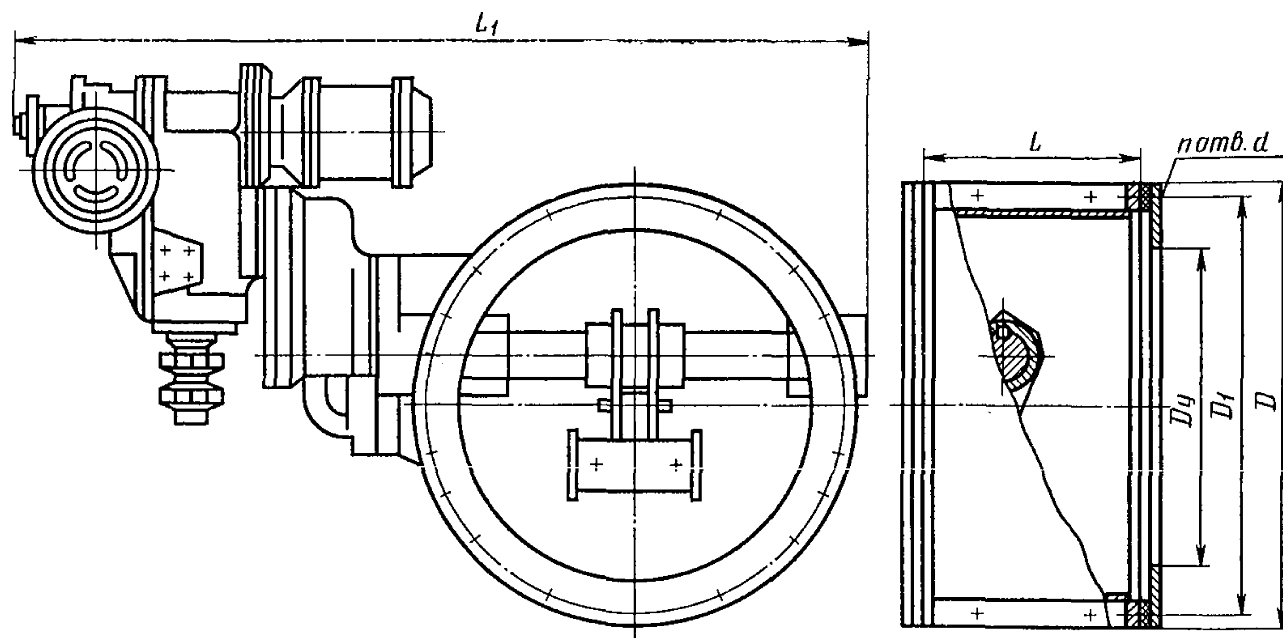
Клапан D_y 300 мм
