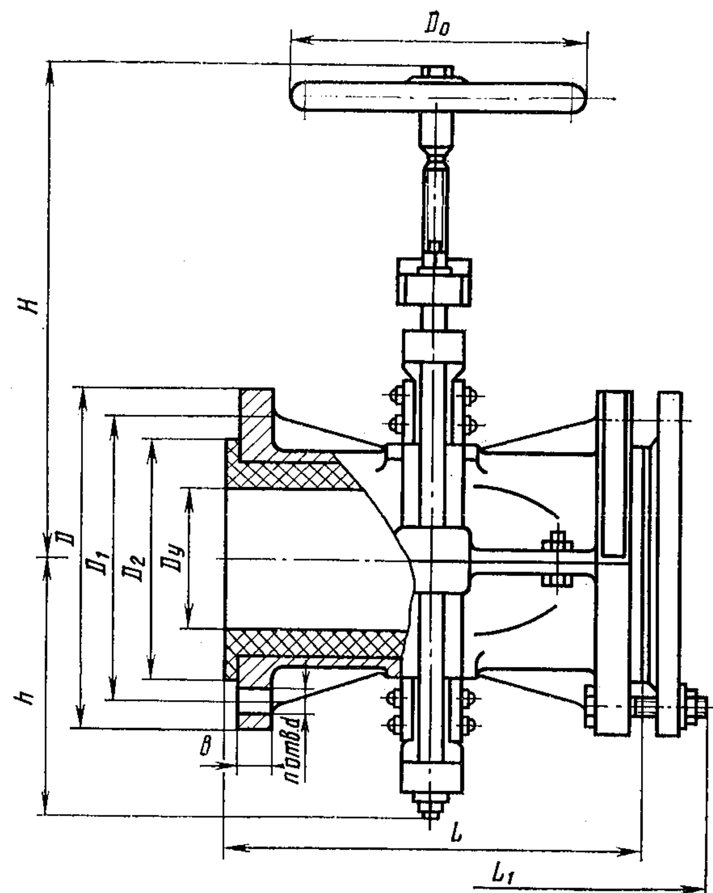
ОСНОВНЫЕ ГАБАРИТНЫЕ, ПРИСОЕДИНИТЕЛЬНЫЕ РАЗМЕРЫ (мм), КОД ОКП И МАССА (кг)
