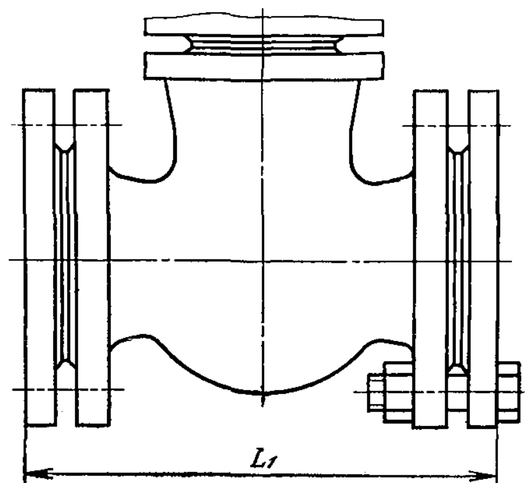
ОСНОВНЫЕ ГАБАРИТНЫЕ И ПРИСОЕДИНИТЕЛЬНЫЕ РАЗМЕРЫ (мм)
