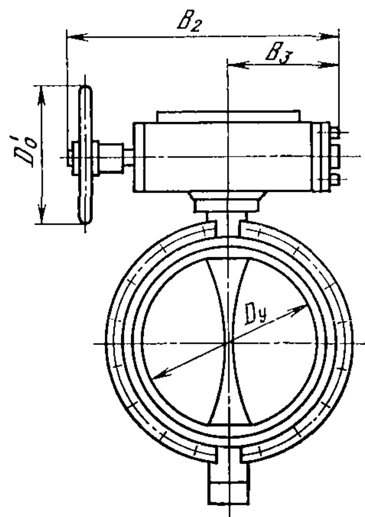
Исполнение с рычажно-винтовым редуктором
