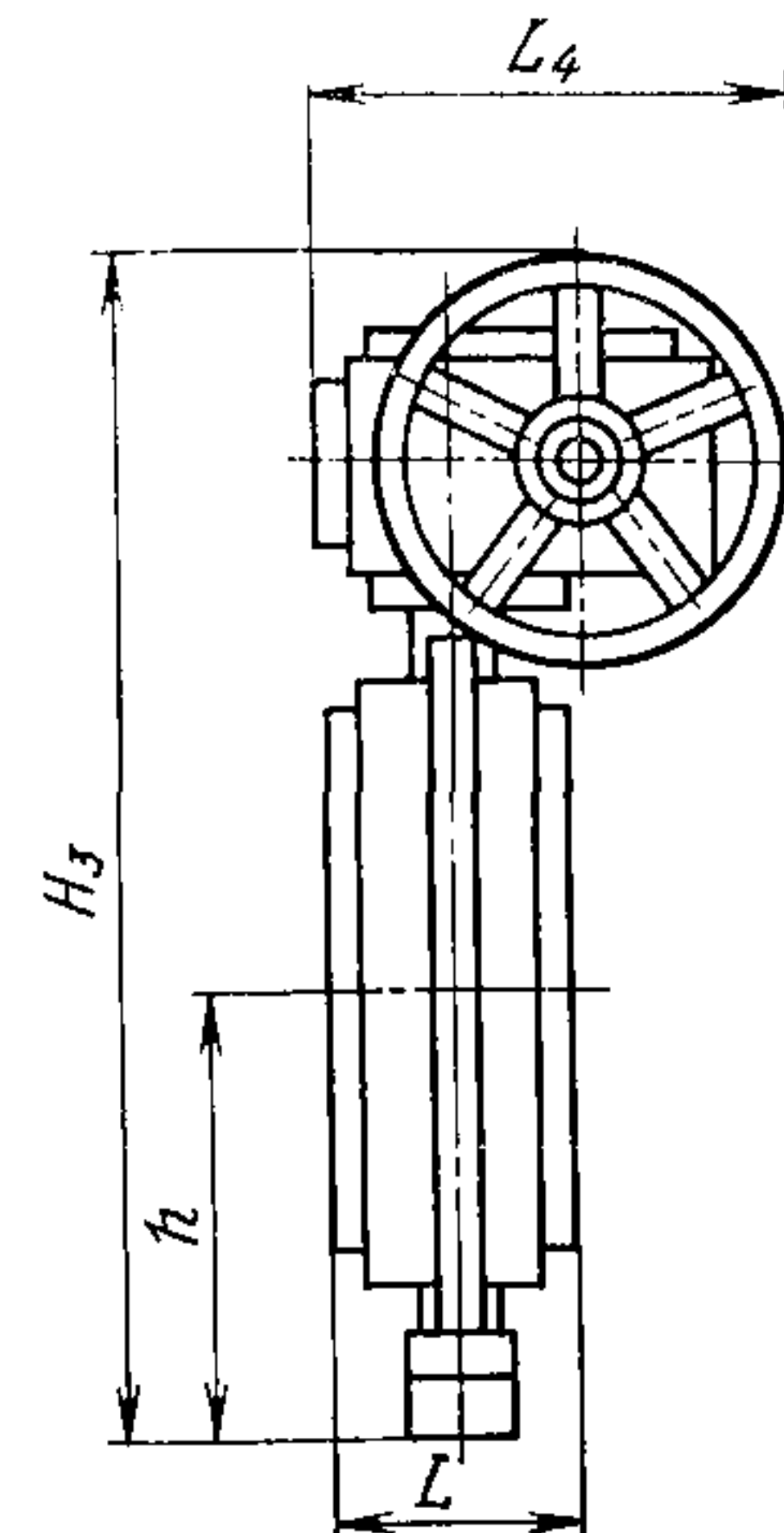
Исполнение с рычажно-винтовым редуктором и электроприводом
