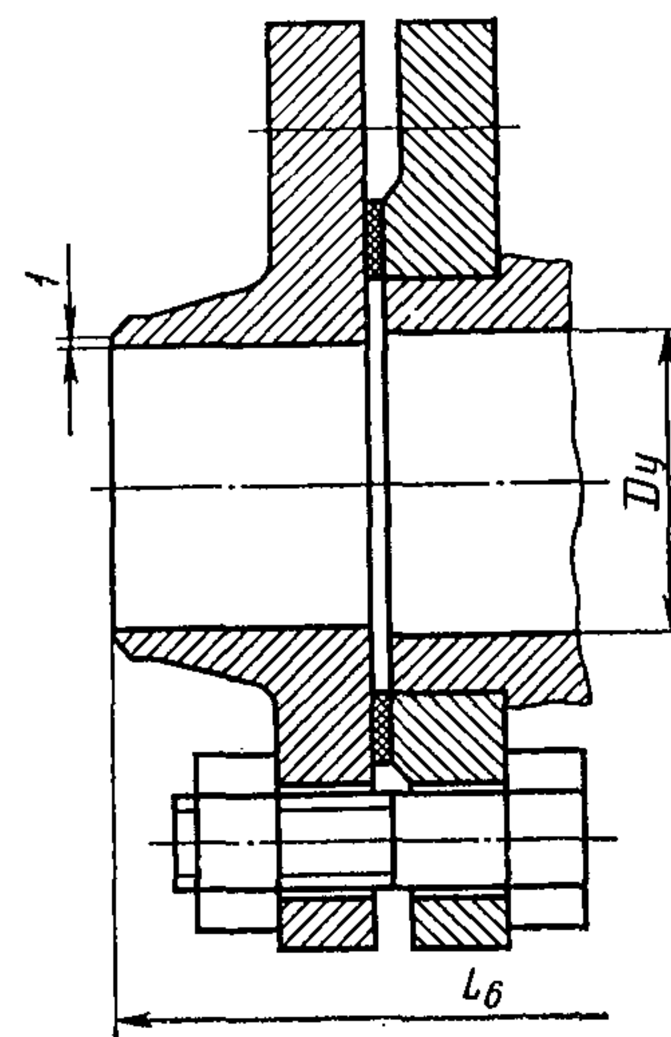
Исполнение с ответными фланцами под приварку
