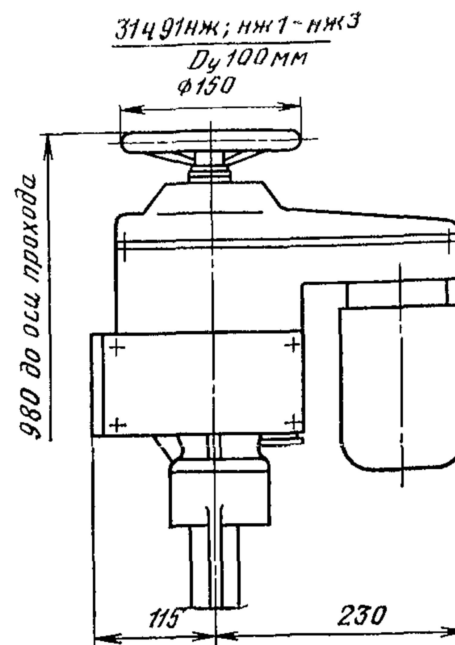
ОСНОВНЫЕ ГАБАРИТНЫЕ И ПРИСОЕДИНИТЕЛЬНЫЕ РАЗМЕРЫ (мм)
