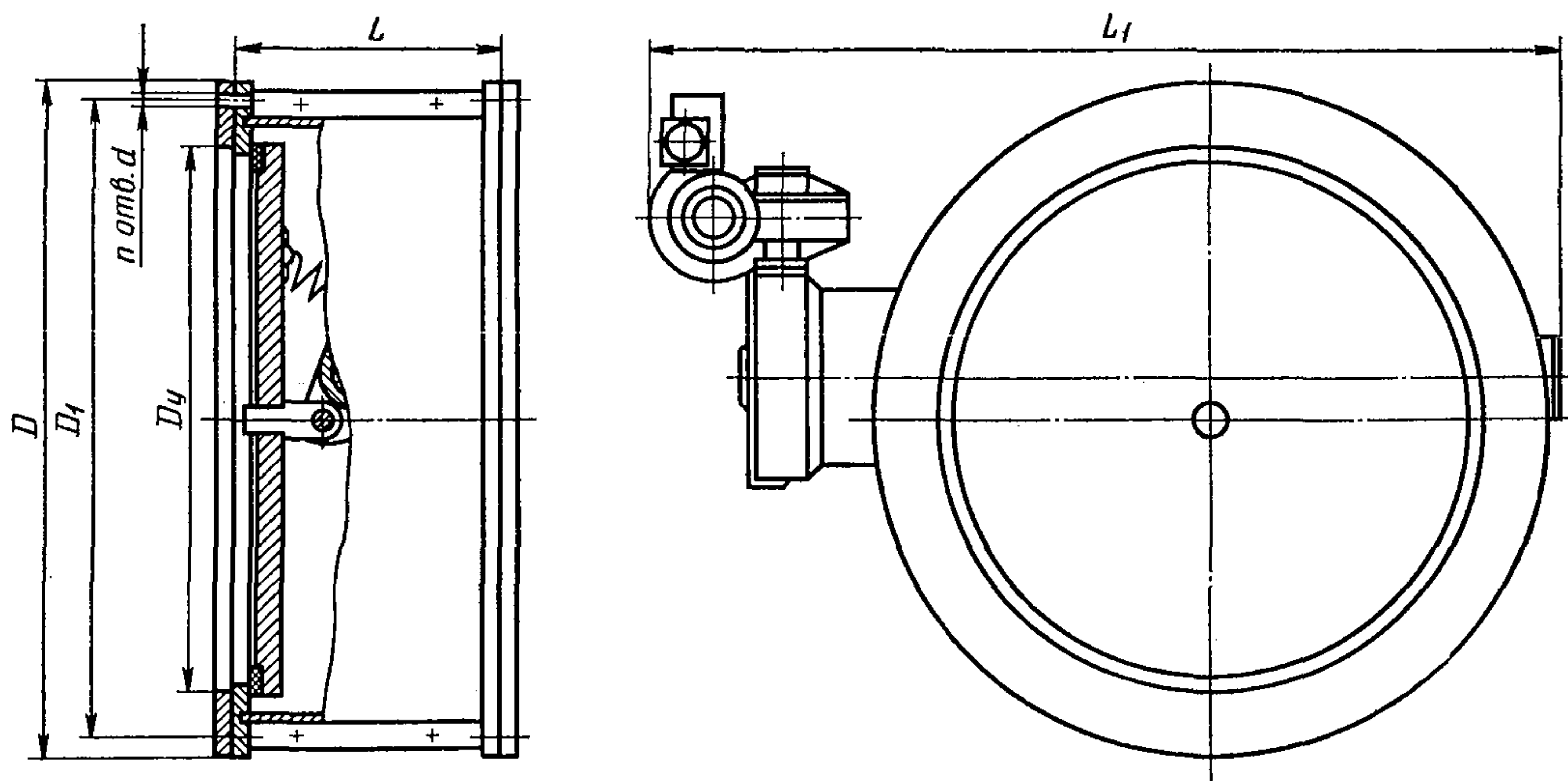
Клапаны D_y 600, 800, 1000 и 1200 мм
