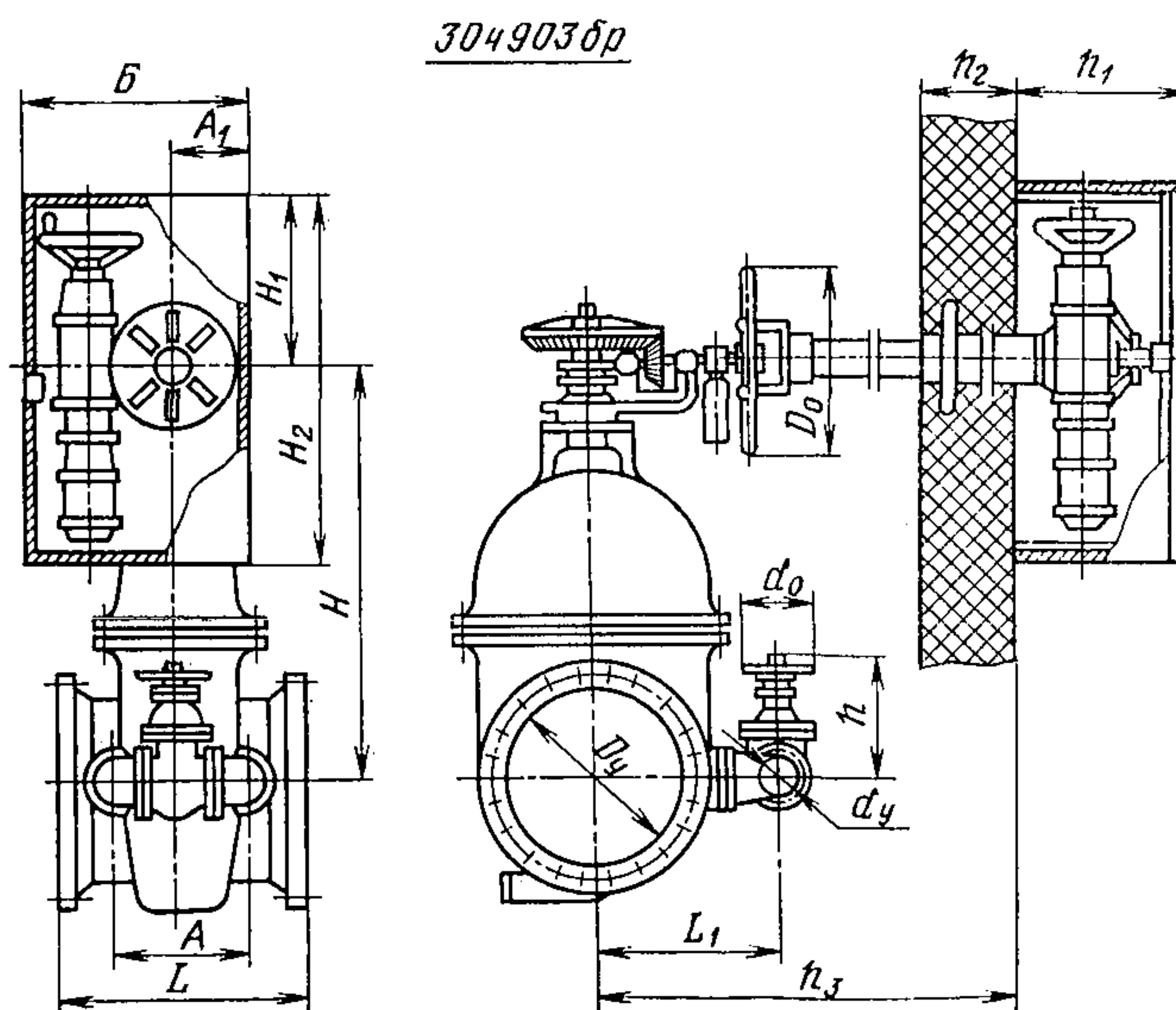
Управление ручное, маховиком через конический редуктор
