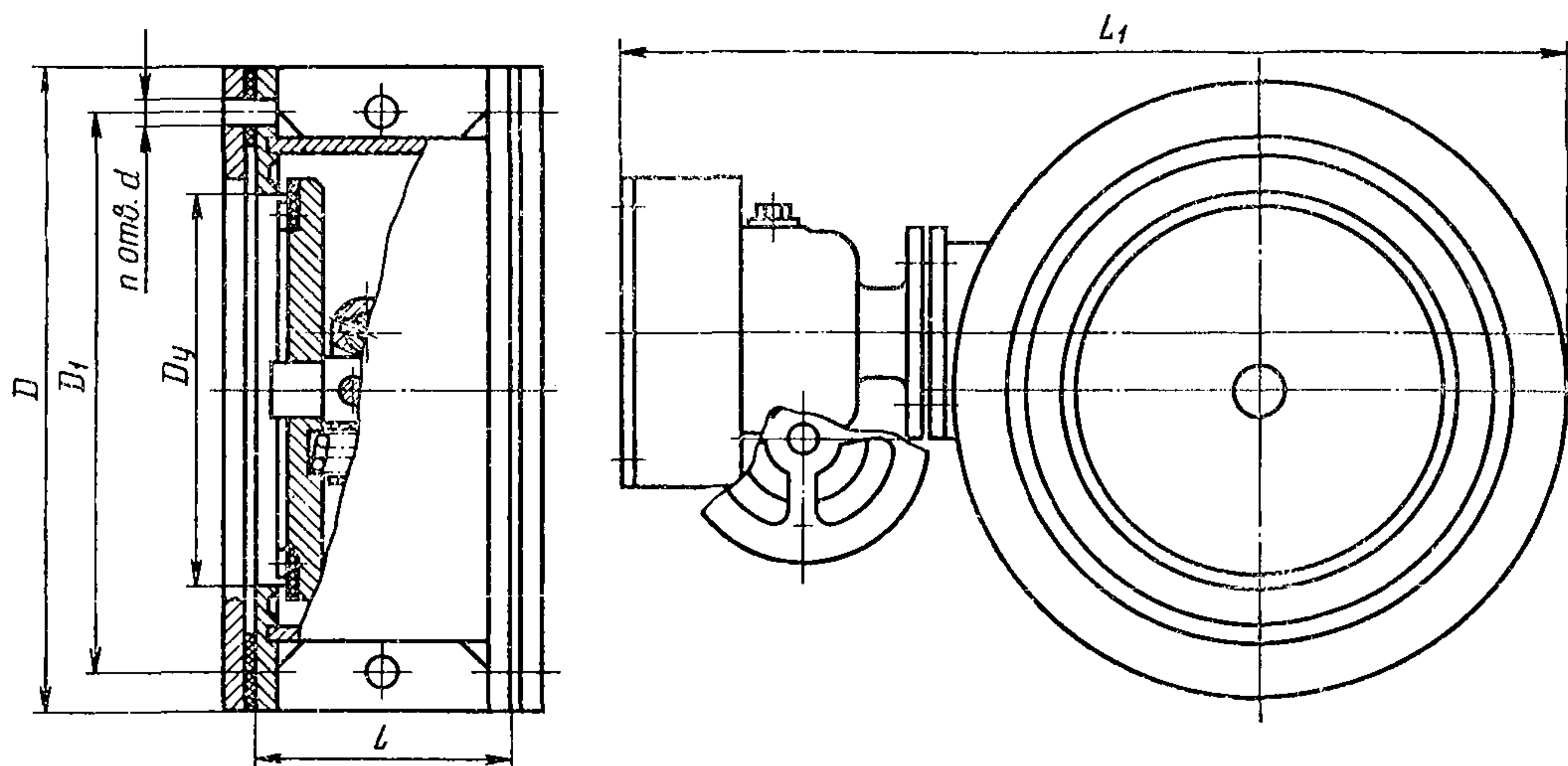
Клапан 19с341нж ( D_y 450 мм)
