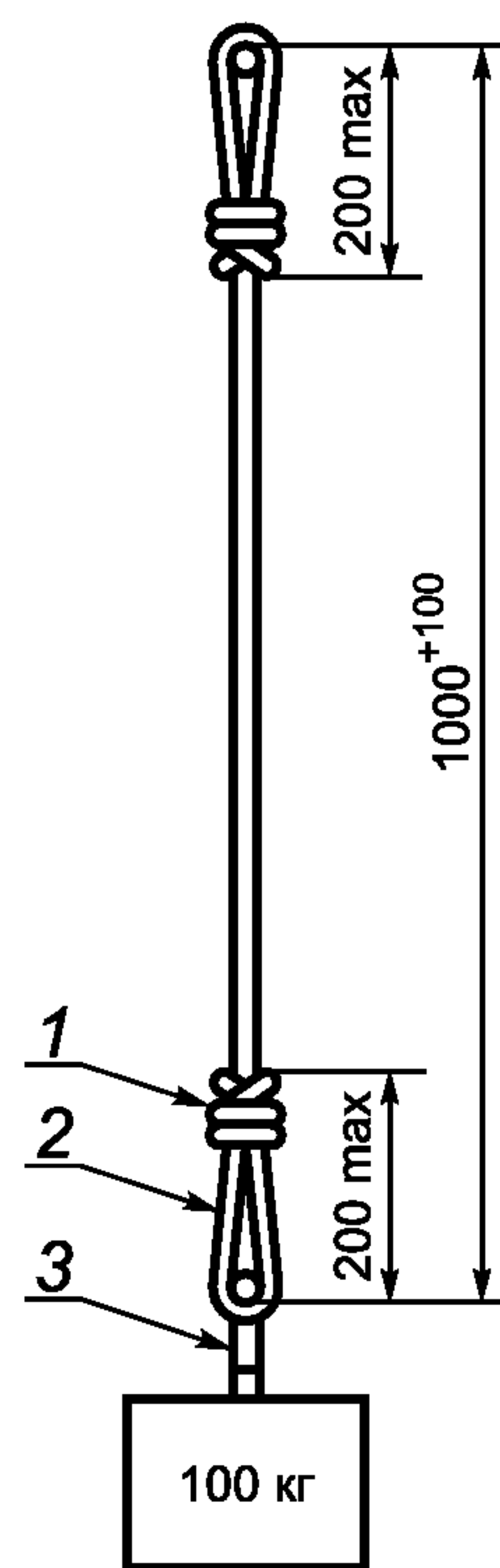
1 — узел; 2 — оконечная петля; 3 — точка присоединения
