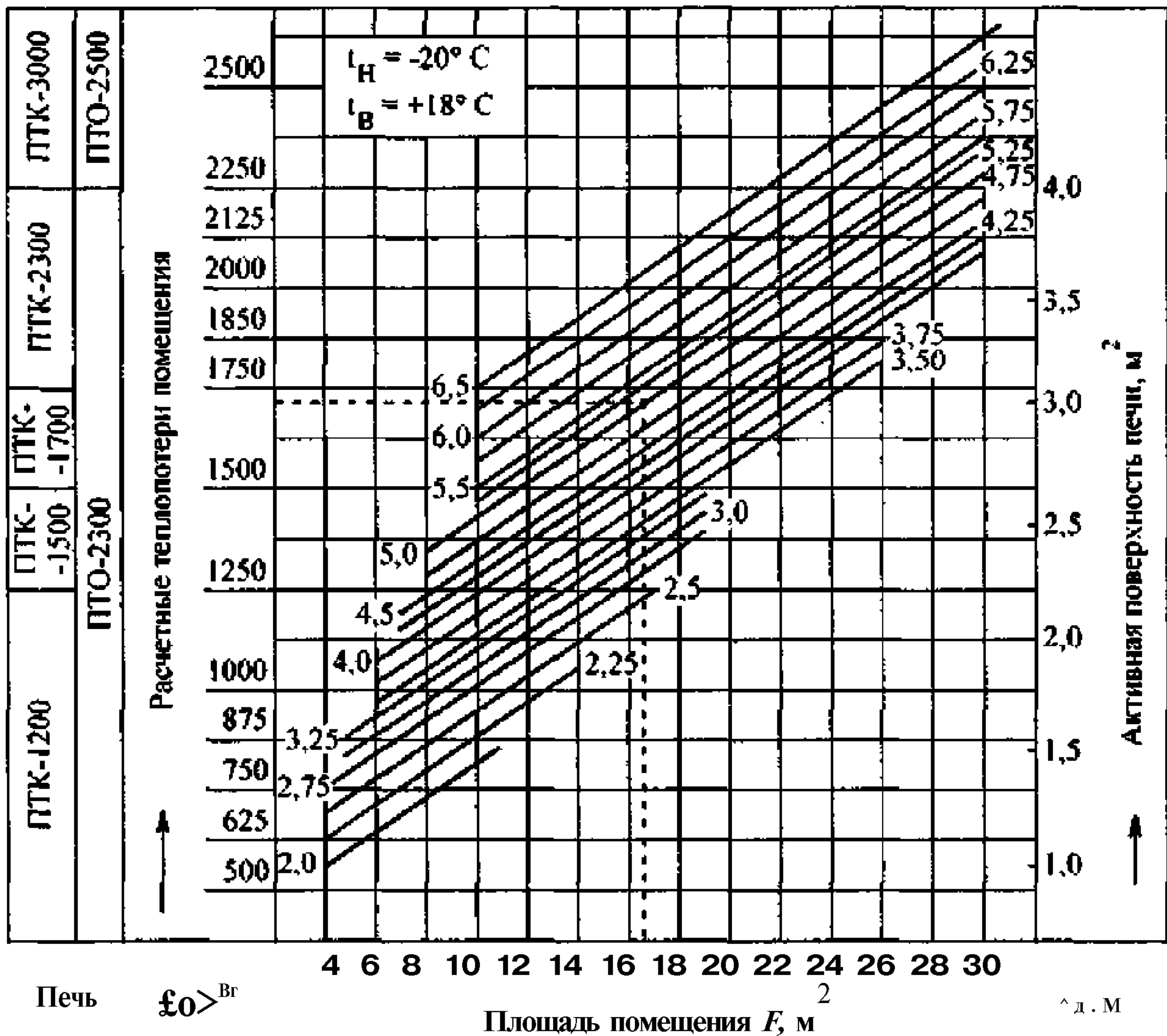
Рис. 3.1. Номограмма для определения теплотерь неугловых комнат.
