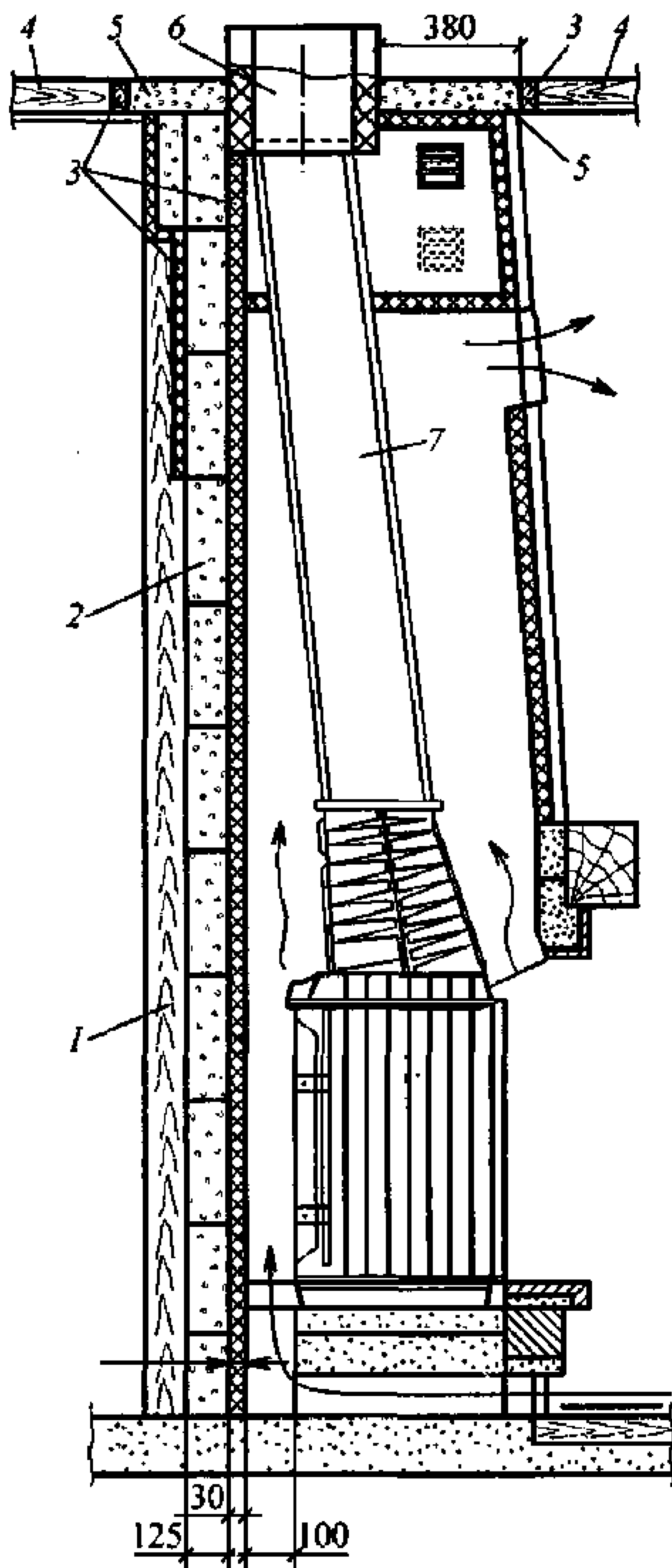
Рис. 4.6. Размещение камина у сгораемых конструкций: 1 - деревянная стена; 2 - кирпич (ячеистый бетон); 3-теплоизоляционный несгораемый материал; 4 - перекрытие из сгораемых материалов; 5 - противопожарная разделка; 6 - дымовая труба; 7 - соединительный патрубок.
