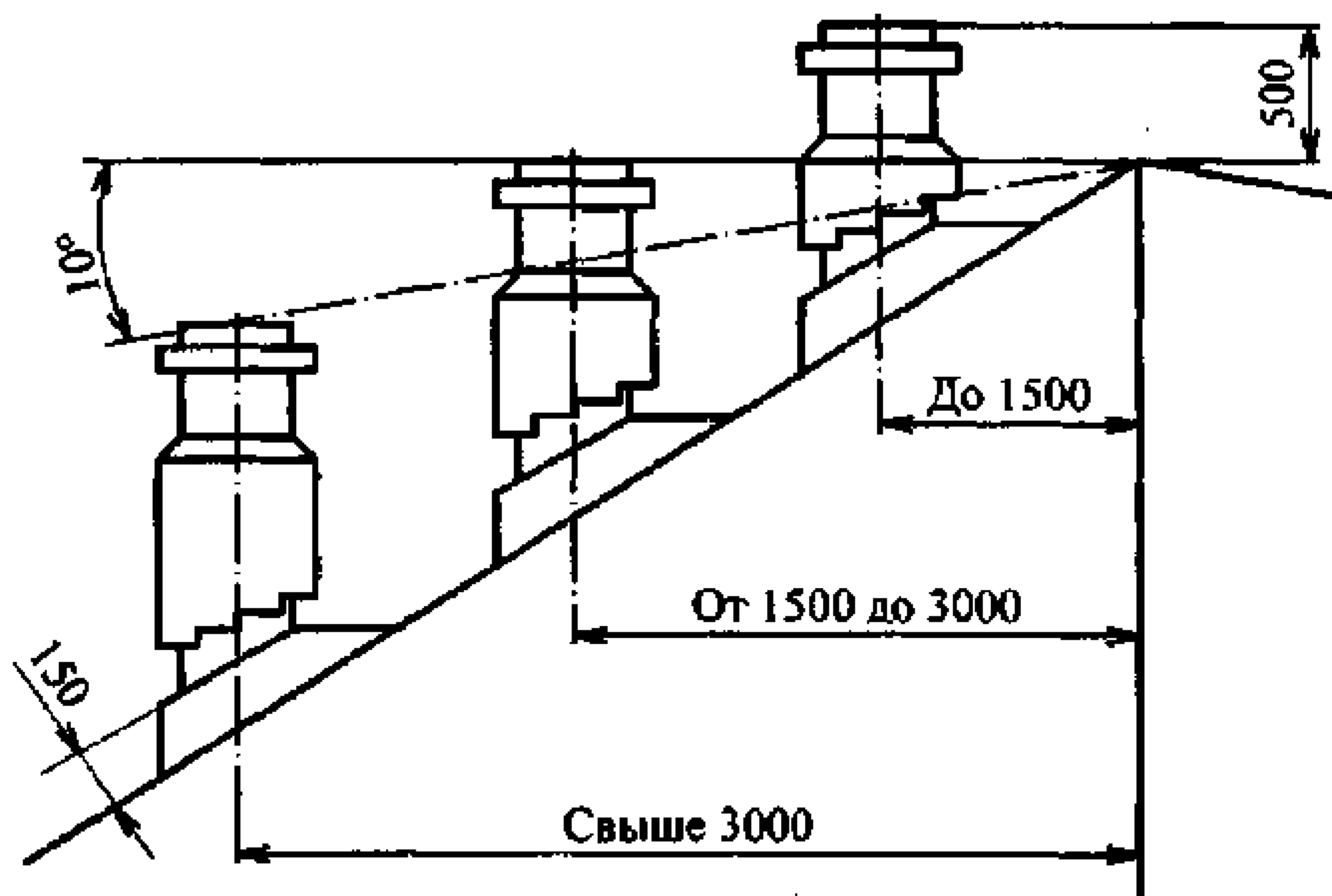
Рис. 3.9. Варианты размещения дымовых каналов над кровлей.
