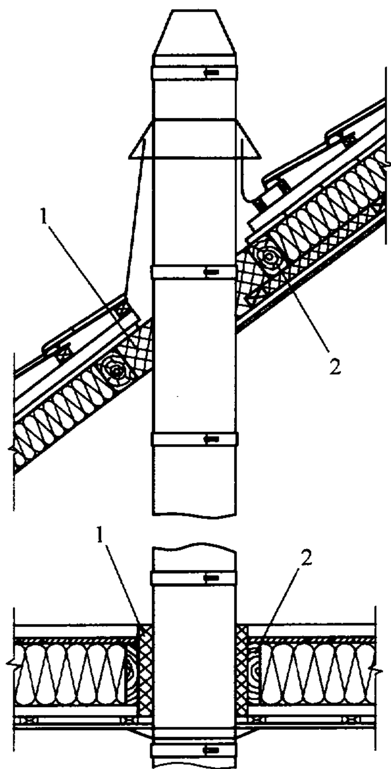
Рис. 6.14. Схема противопожарной разделки: 1 - теплоизоляция; 2 - деревянные конструкции.
