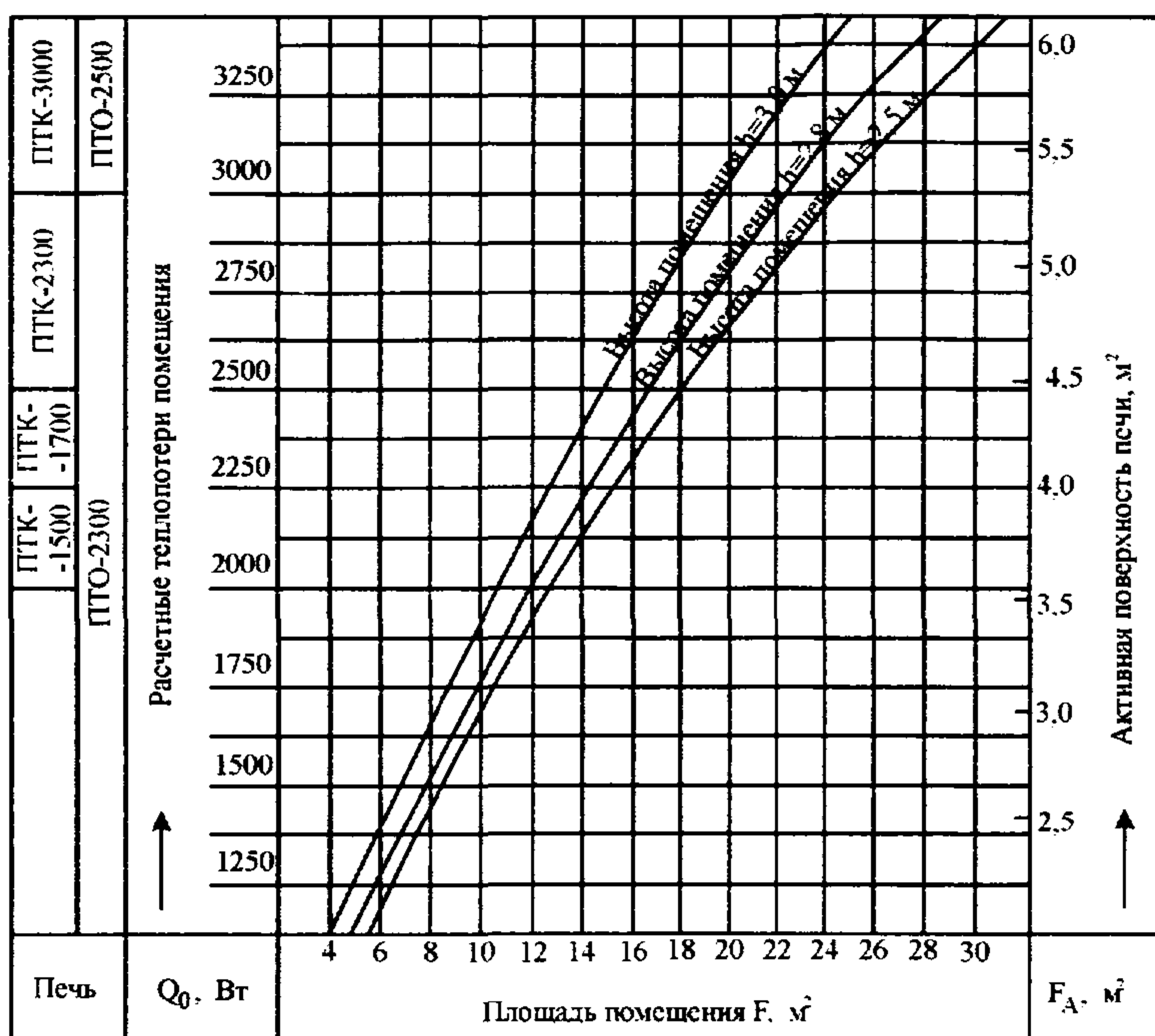
Рис. 3.2. Номограмма для определения тепловых потерь угловых комнат
