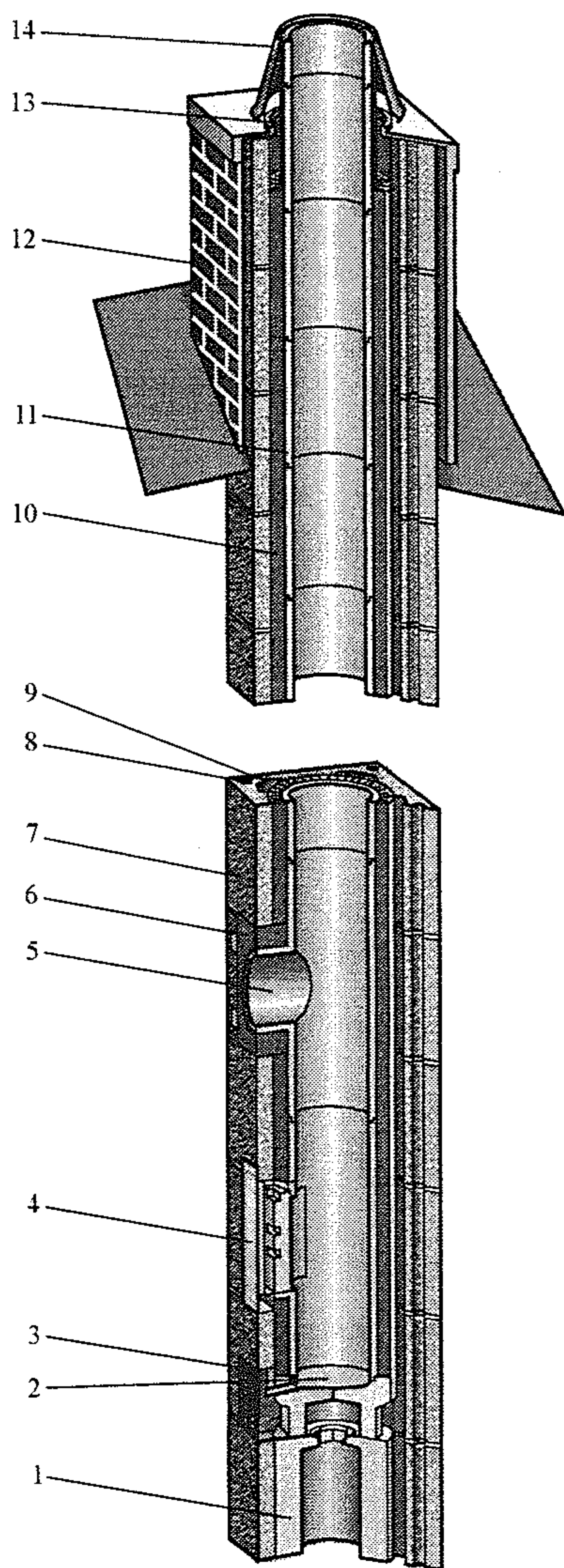
Рис. 6.8. Конструкция керамической дымовой трубы:
