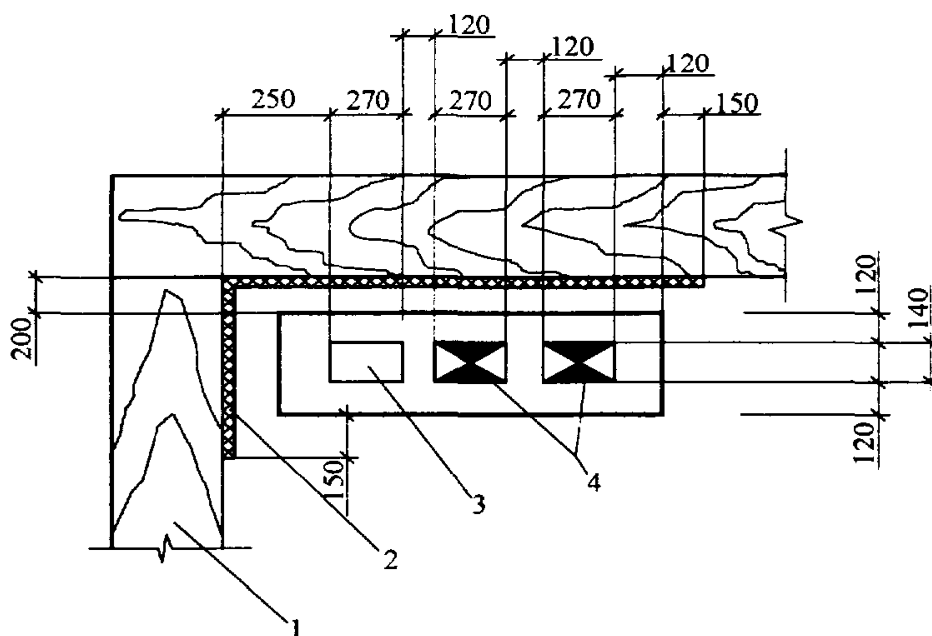
Рис. 6.11. Устройство отступки:
