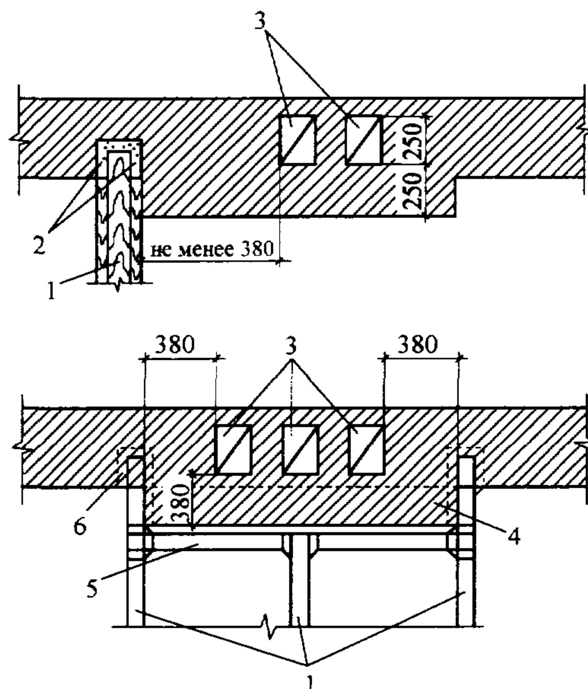
Рис. 6.13. Размещение деревянных балок и ригелей:
