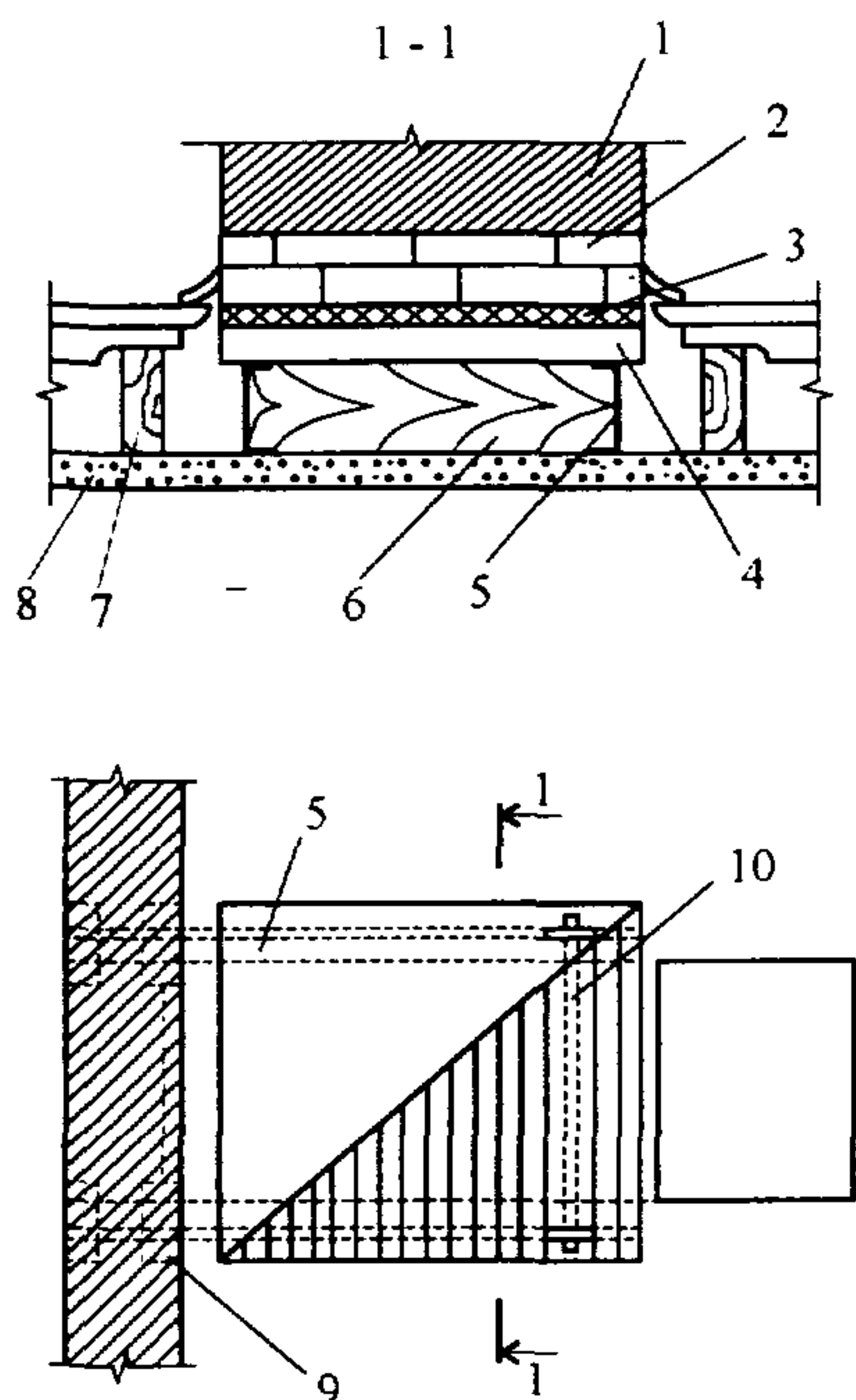
Рис. 3.5. Основание печи на консолях:
