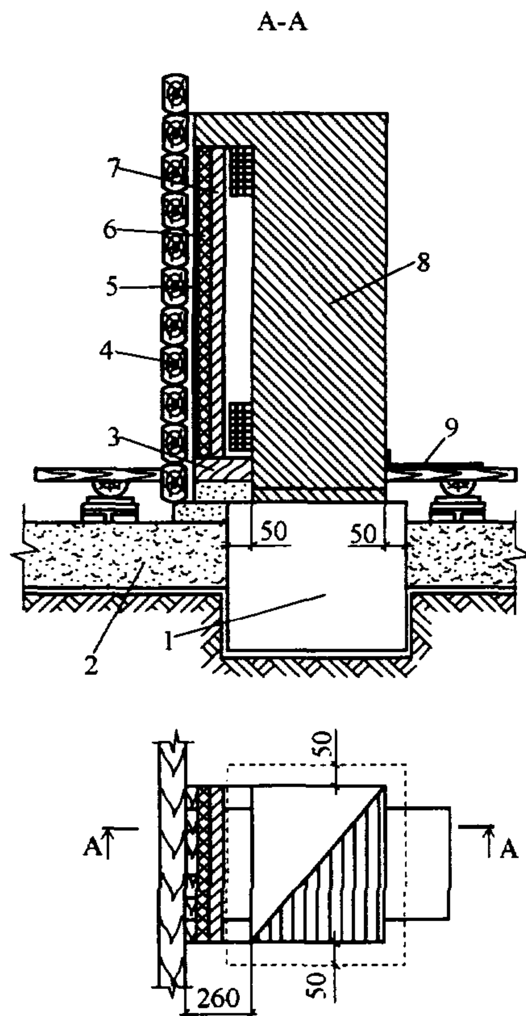
Рис. 3.8. Устройство закрытой отступки: 1 - фундамент печи; 2 - уплотнительный слой; 3 - несгораемый пол; 4 - деревянная стена; 5 - щит из досок; 6 - теплоизоляция (асбест или войлок); 7 - кирпич "на ребро"; 8 - печь; 9 - предтопочный лист.
