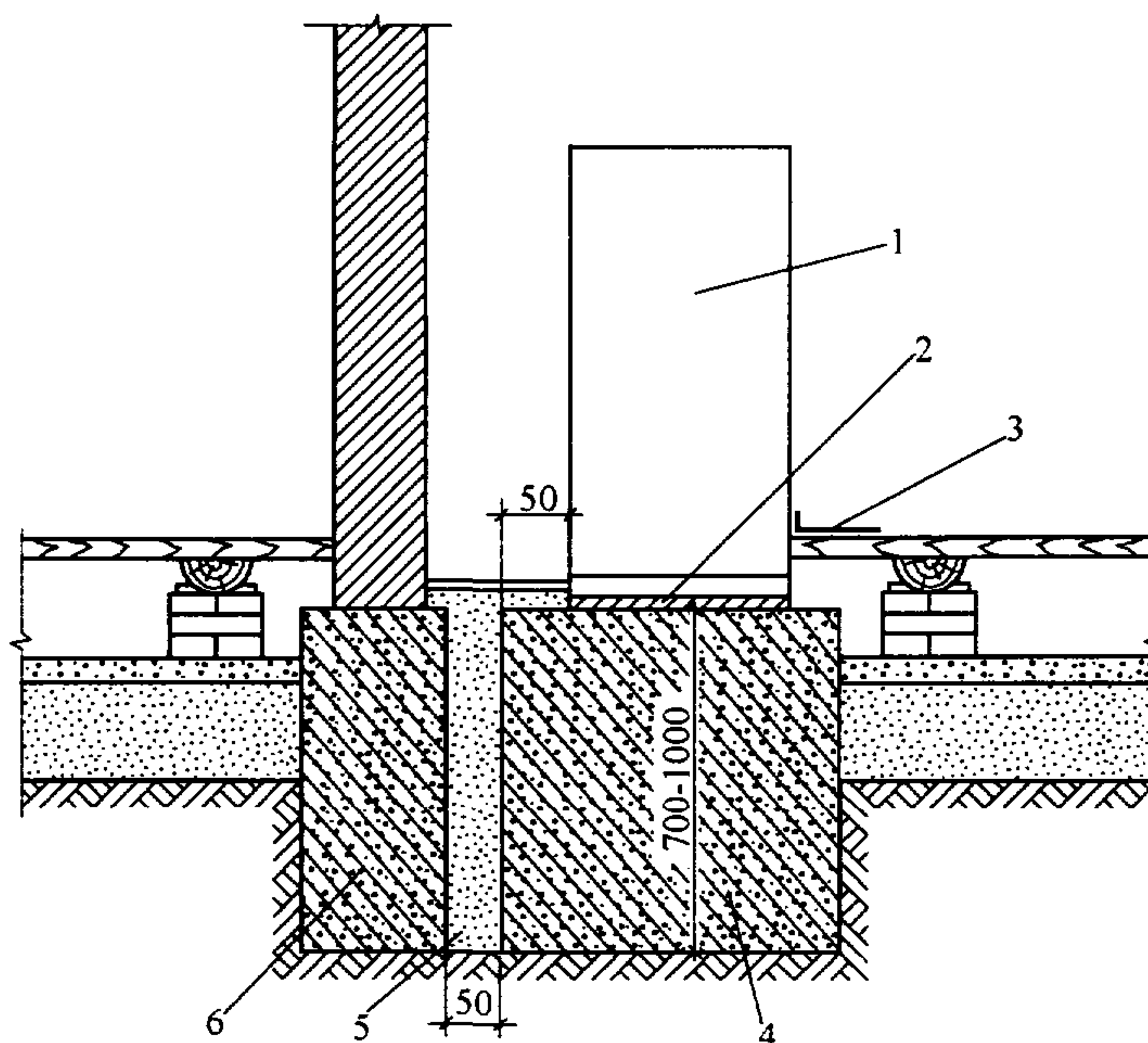
Рис. 3.4. Размещение печи на отдельном фундаменте:
