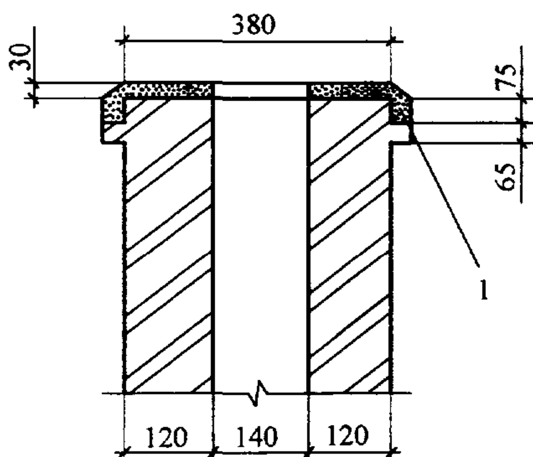
Рис. 6.5. Устройство оголовка:
