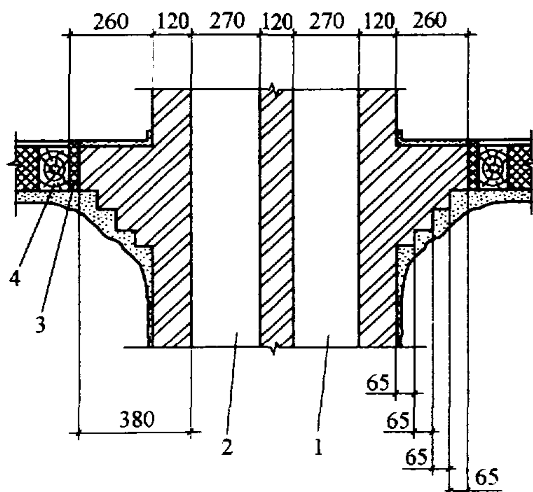
Рис. 6.12. Горизонтальная разделка:
