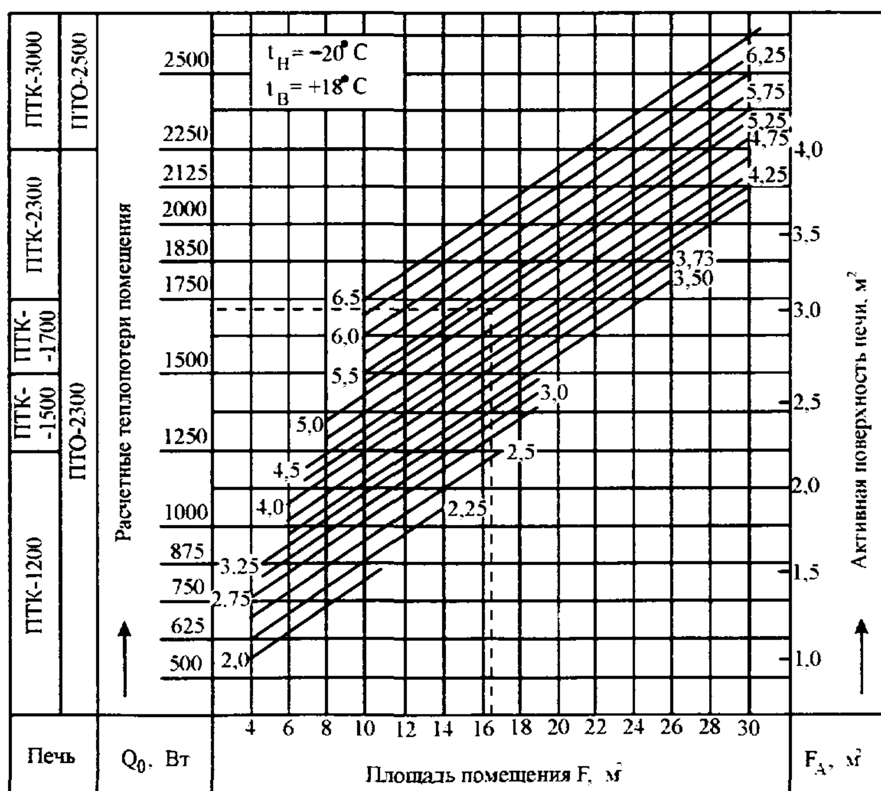
Рис. 3.1. Номограмма для определения теплотерь неугловых комнат
