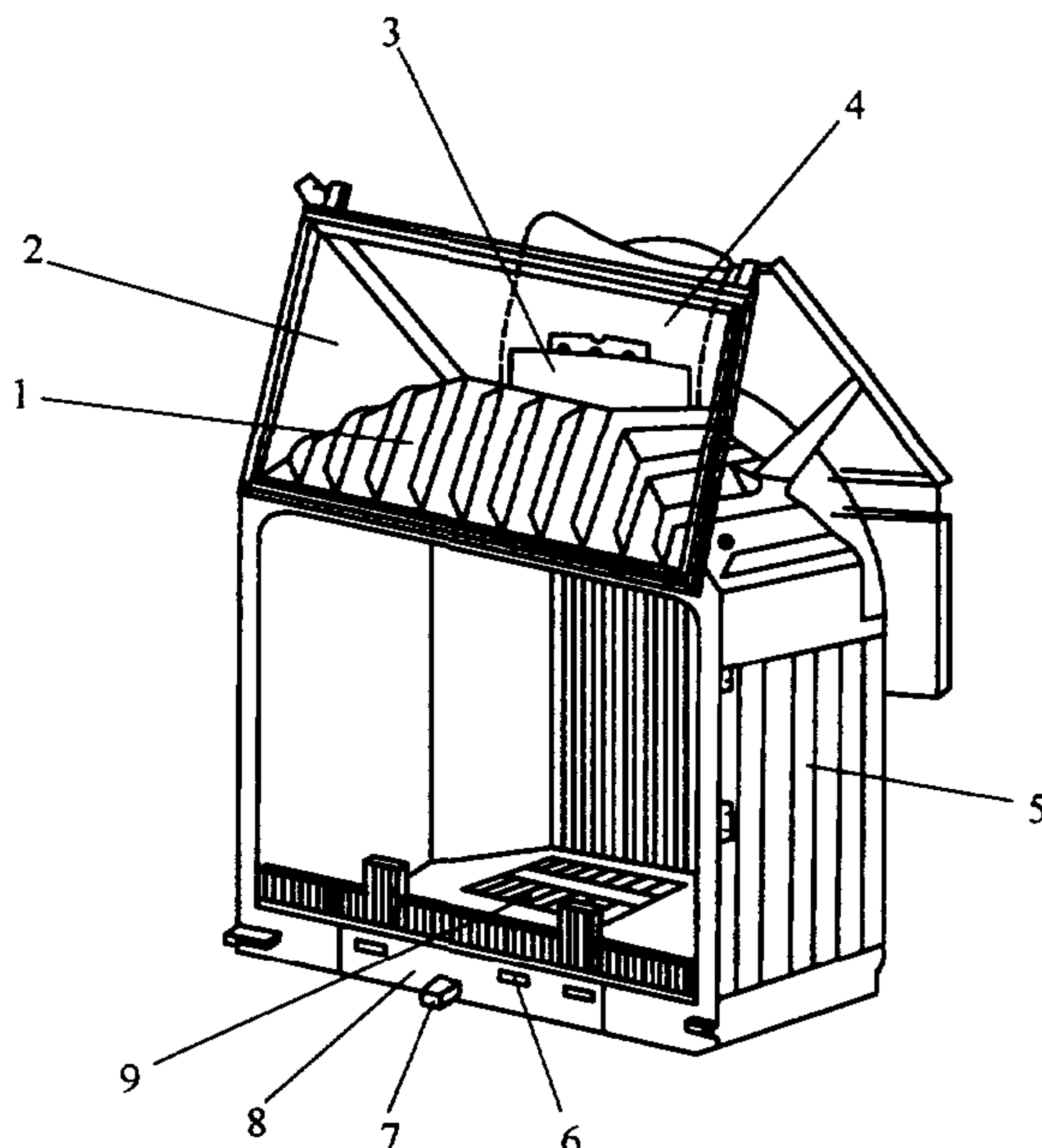
Рис. 5.3. Общий вид топки камина:
