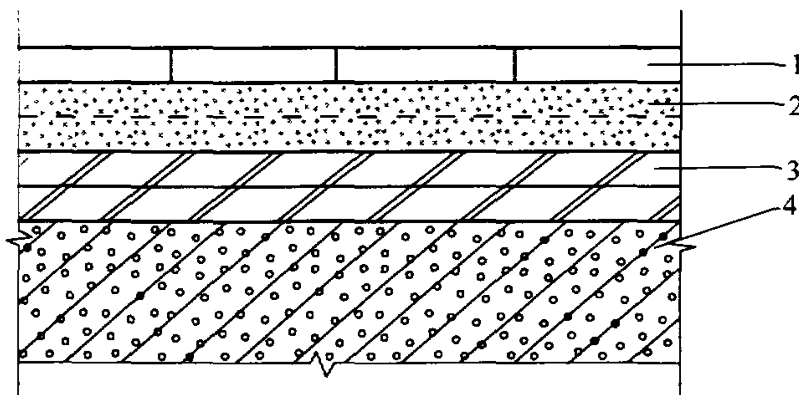
Рис. 5.5. Детали пола:
