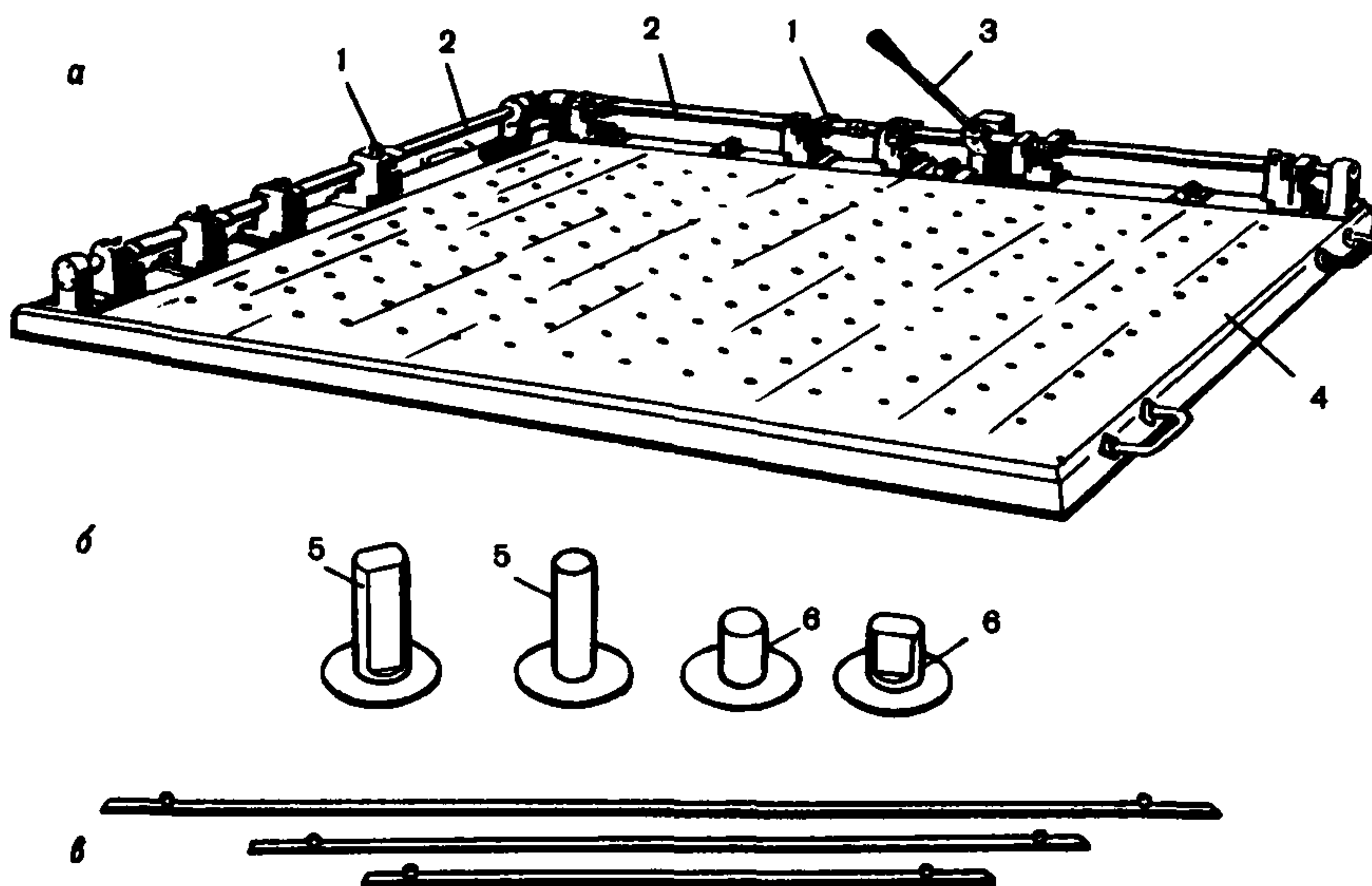
Рис. 22. Универсальное приводное штифтовое устройство (УПШУ-ЦНИИГАиК) а — перфоратор; б — штифты калиброванные; в — приводные линейки со штифтами; 1 — станцевальные головки; 2 — направляющие штанги; 3 — рычаг с ручкой; 4 — рабочий стол; 5 — штифты для монтажных работ; 6 — штифты для копировальных работ
