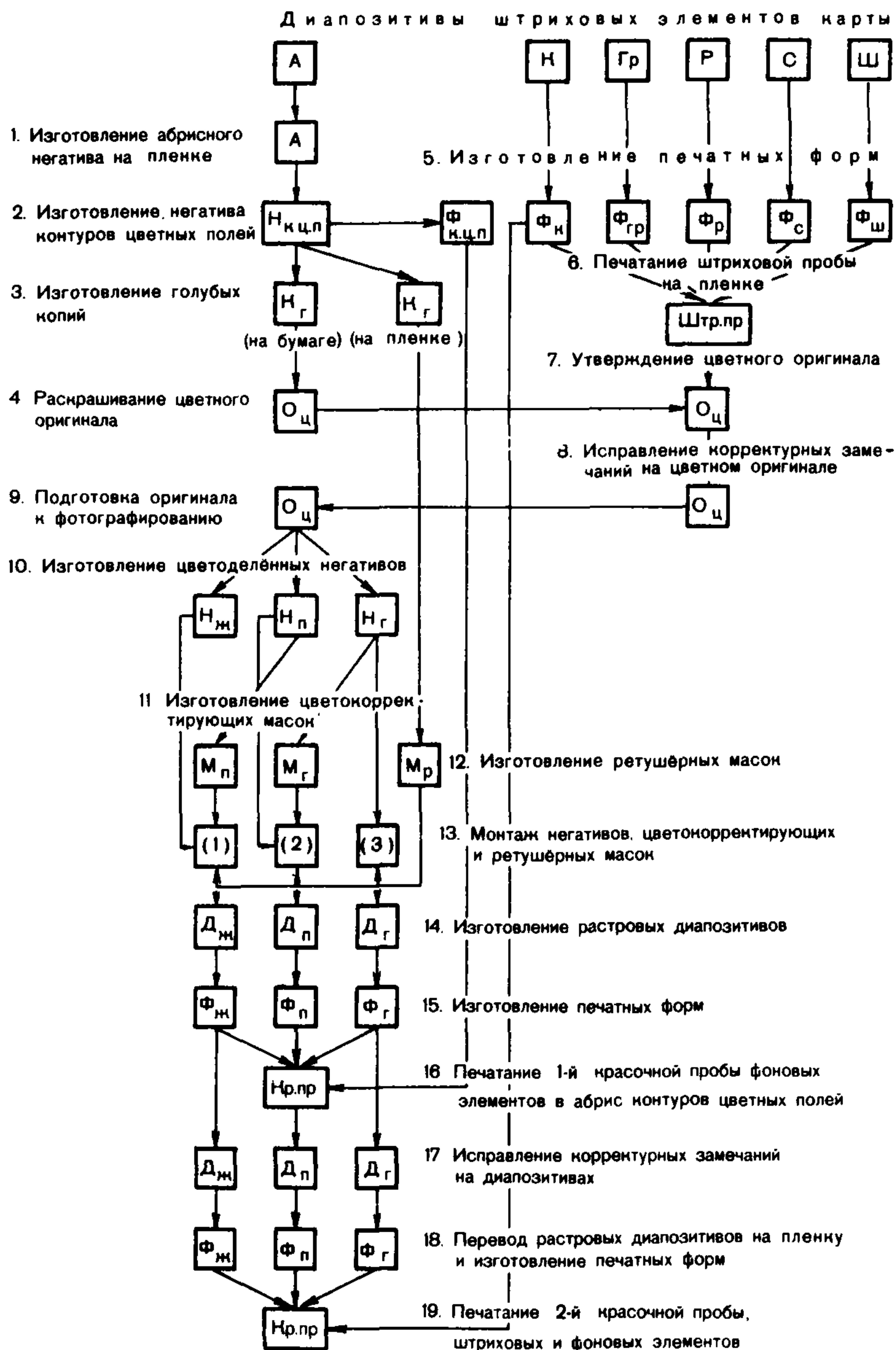
Рис. 14. Схема технологических процессов подготовки и воспроизведения оригиналов ровной фоновой окраски карт с применением фотомеханического цветоделения
