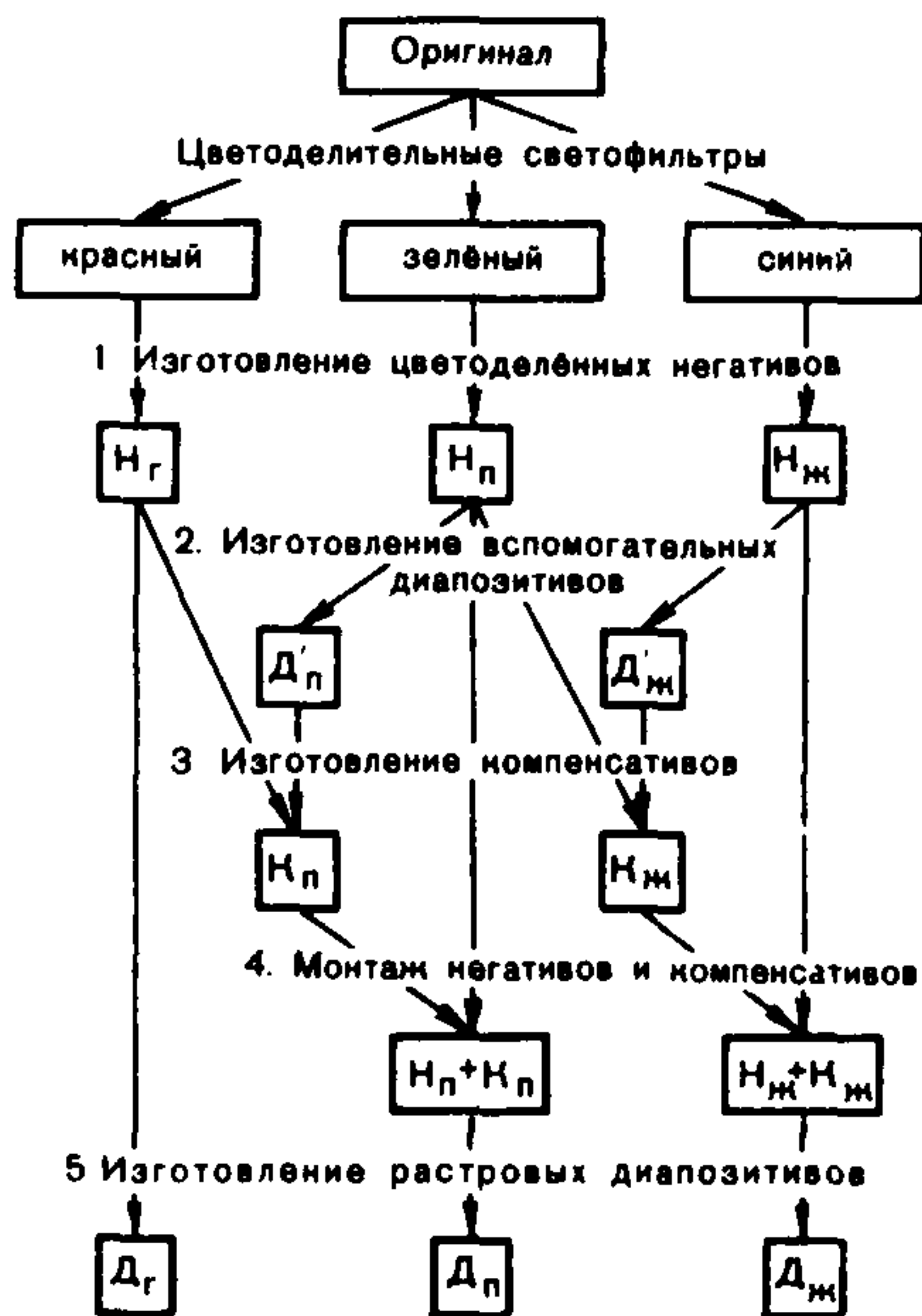
Рис. 11. Схема компенсативного (двух-ступенчатого) маскирования
