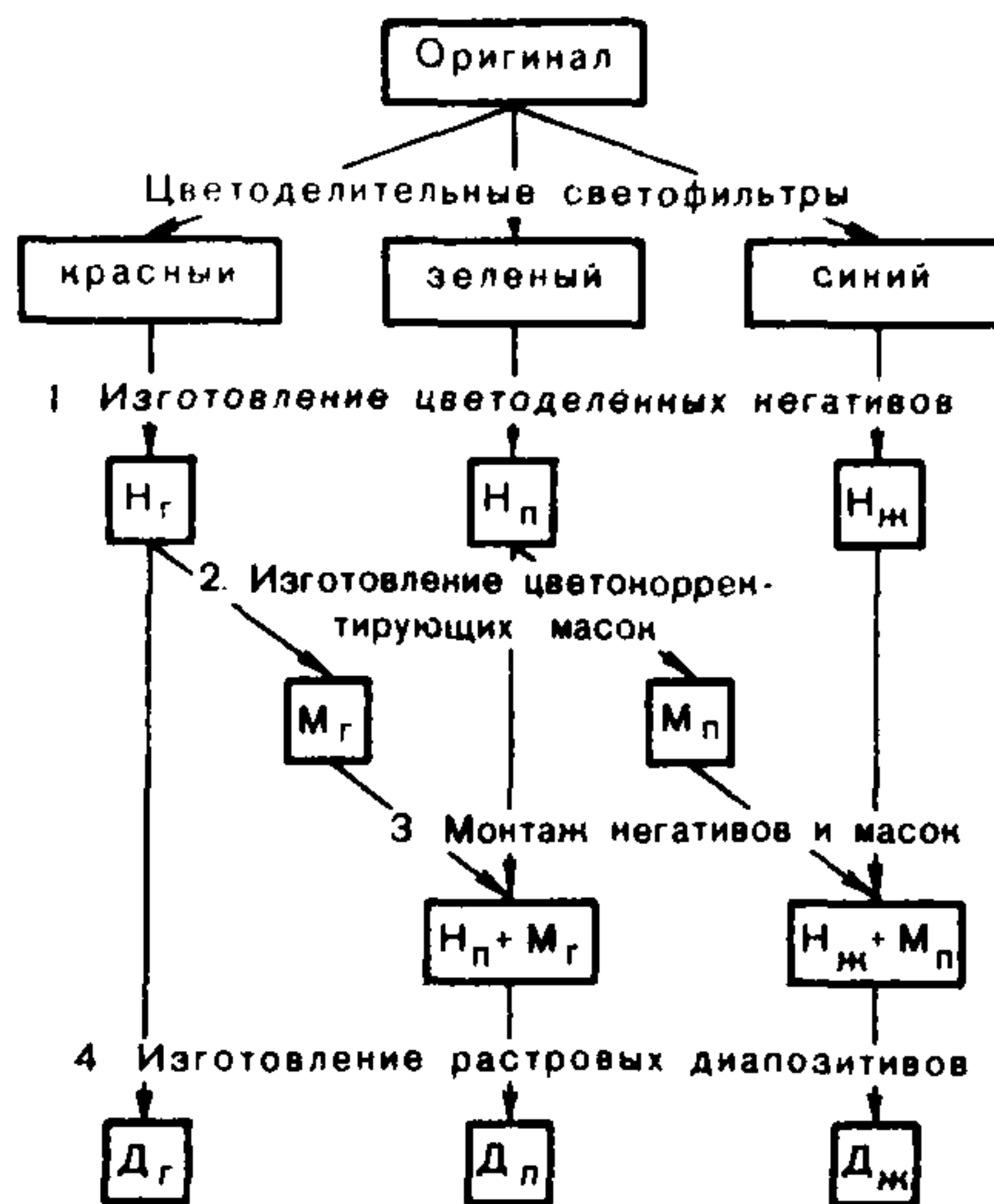
Рис. 10. Схема перекрестного (одно-ступенчатого) маскирования
