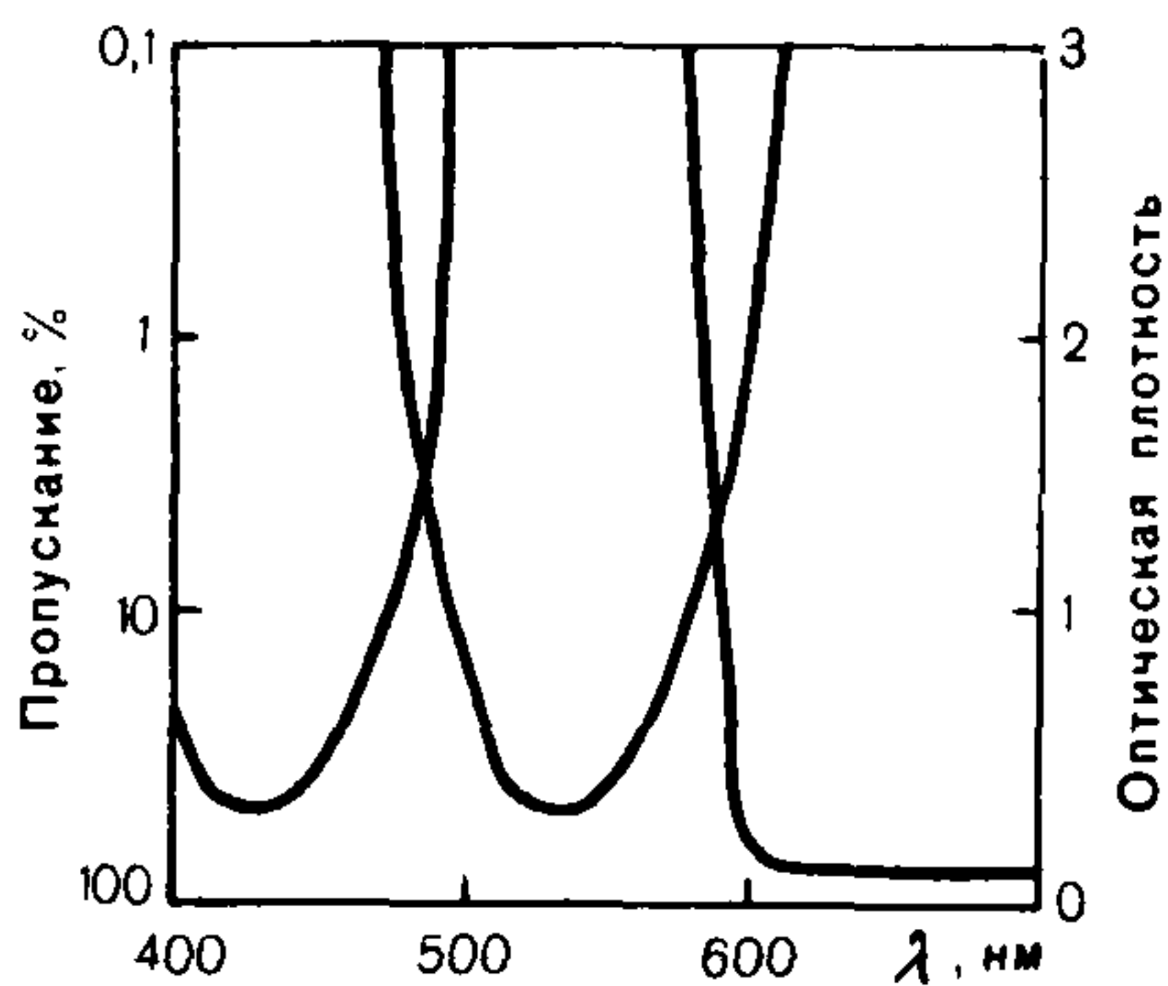
Рис. 9. Кривые спектральной характеристики цветоделительных светофильтров
