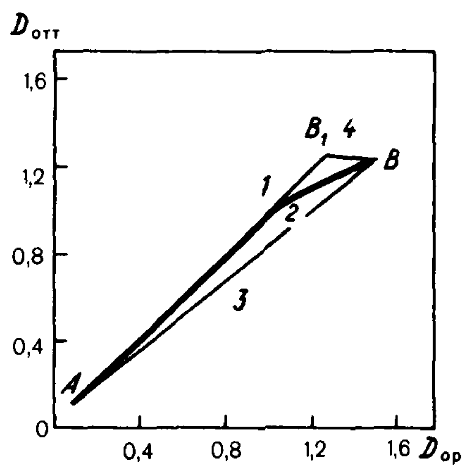
Рис. 7. Схема построения кривой тоновоспроизведения
