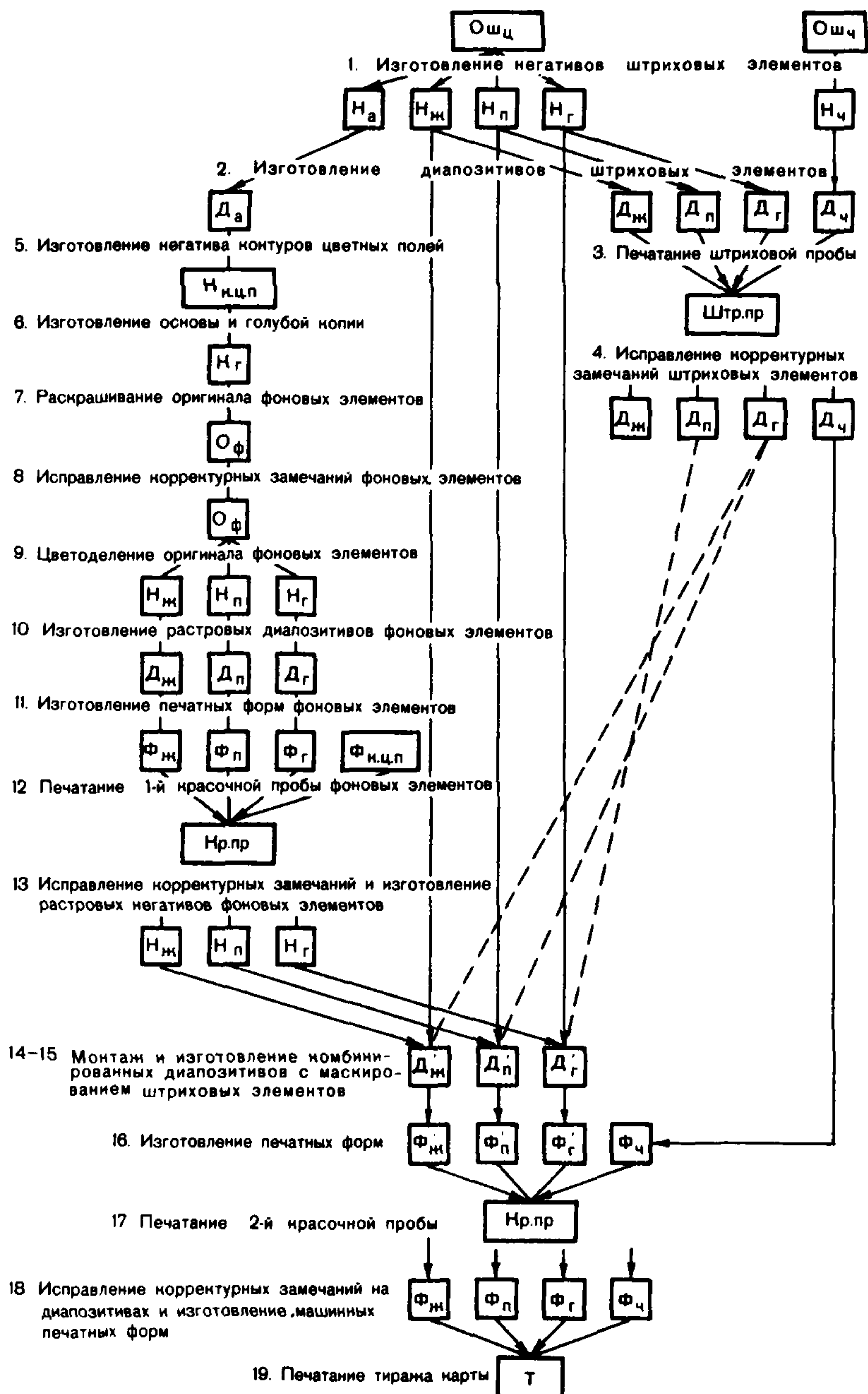
Рис. 17. Схема технологических процессов подготовки и издания карт с изготовлением комбинированных диапозитивов (фон + штрих) на малodeформирующей фототехнической пленке
