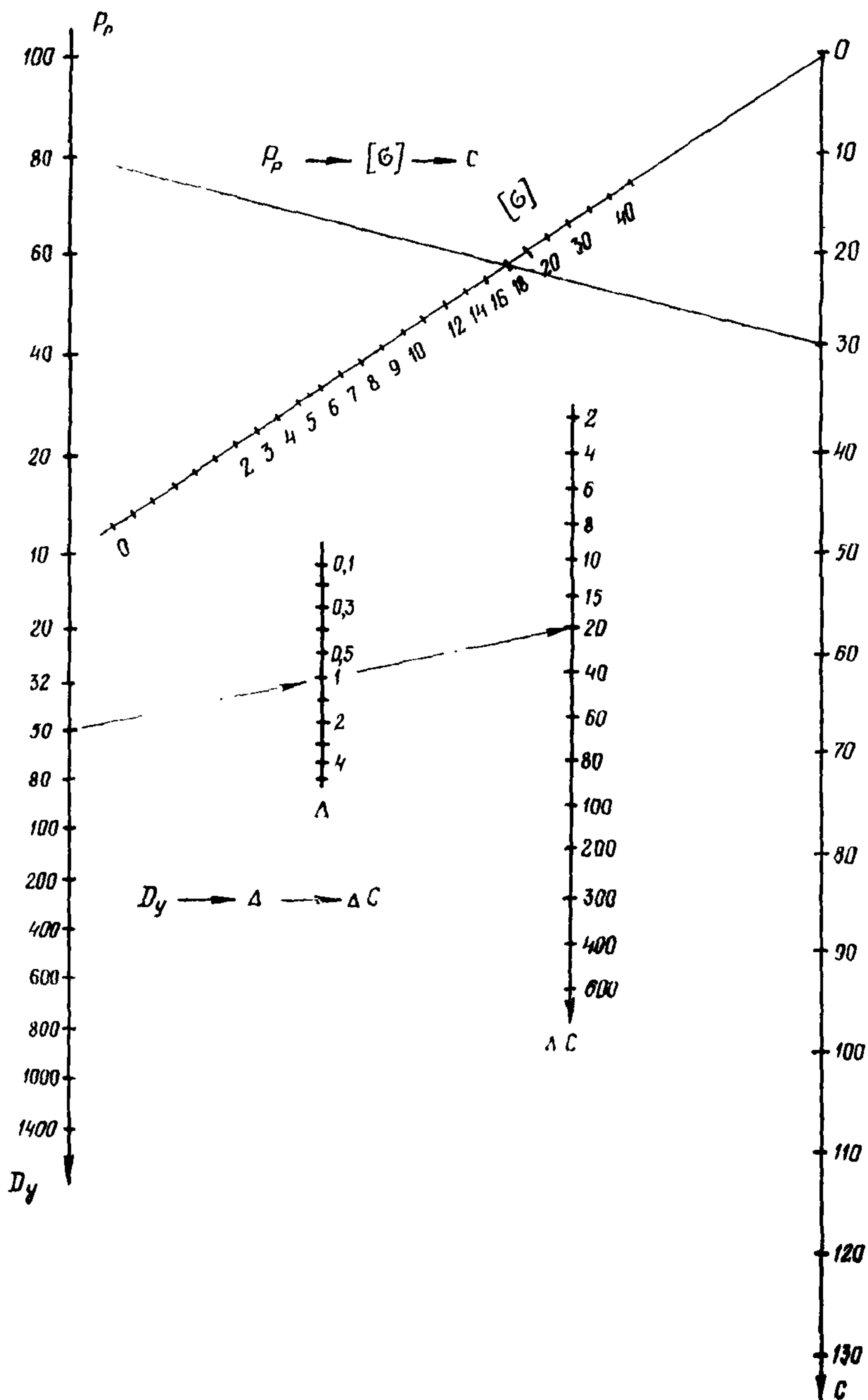
Рис. 1. Номограмма для определения серии труб. Обозначения: [\sigma] — допускаемое напряжение, кгс/мм 2 ; P_p — рабочее давление, кгс/см 2 ; D_y — условный проход, мм; C — серия труб для мало- и неагрессивных сред; \Delta — прибавка на агрессивность среды, мм; \Delta C — поправка к серии труб на агрессивность среды
