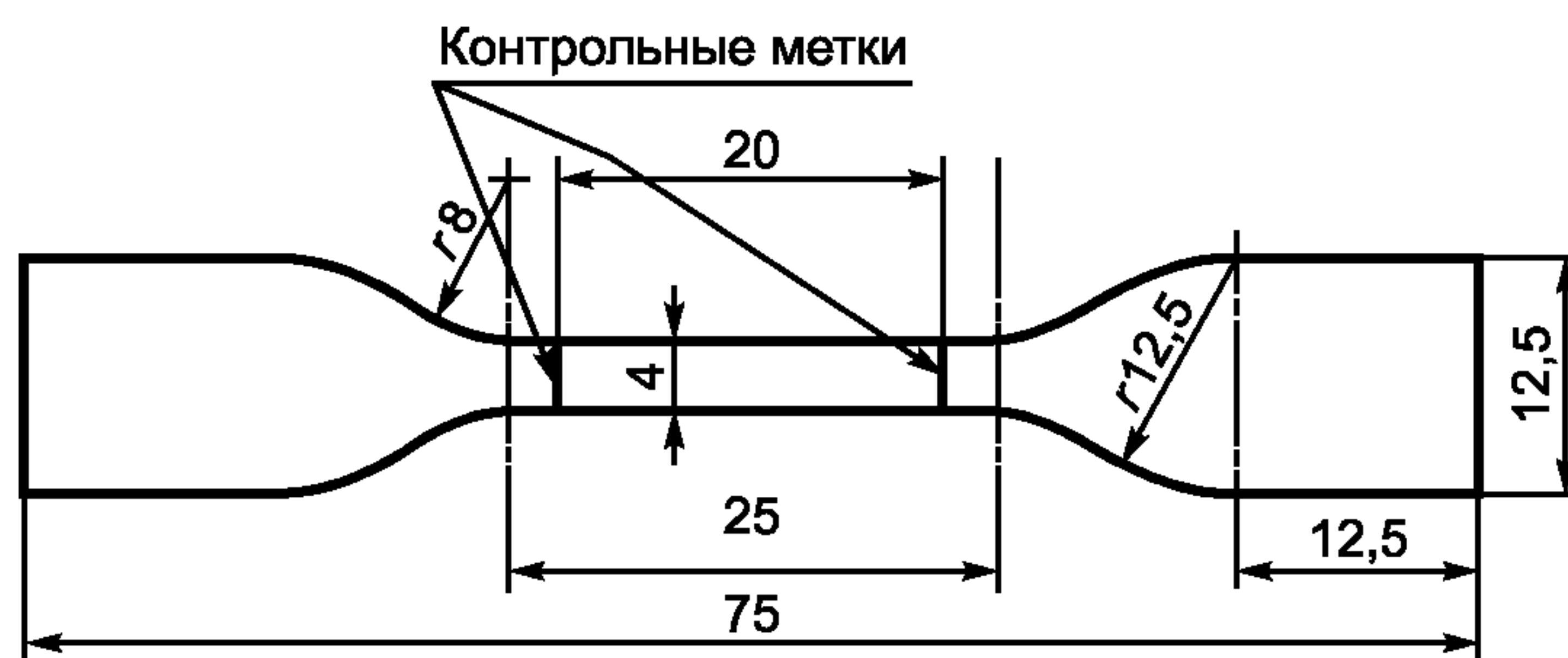
Рисунок 3 — Образец в форме двусторонней лопатки
