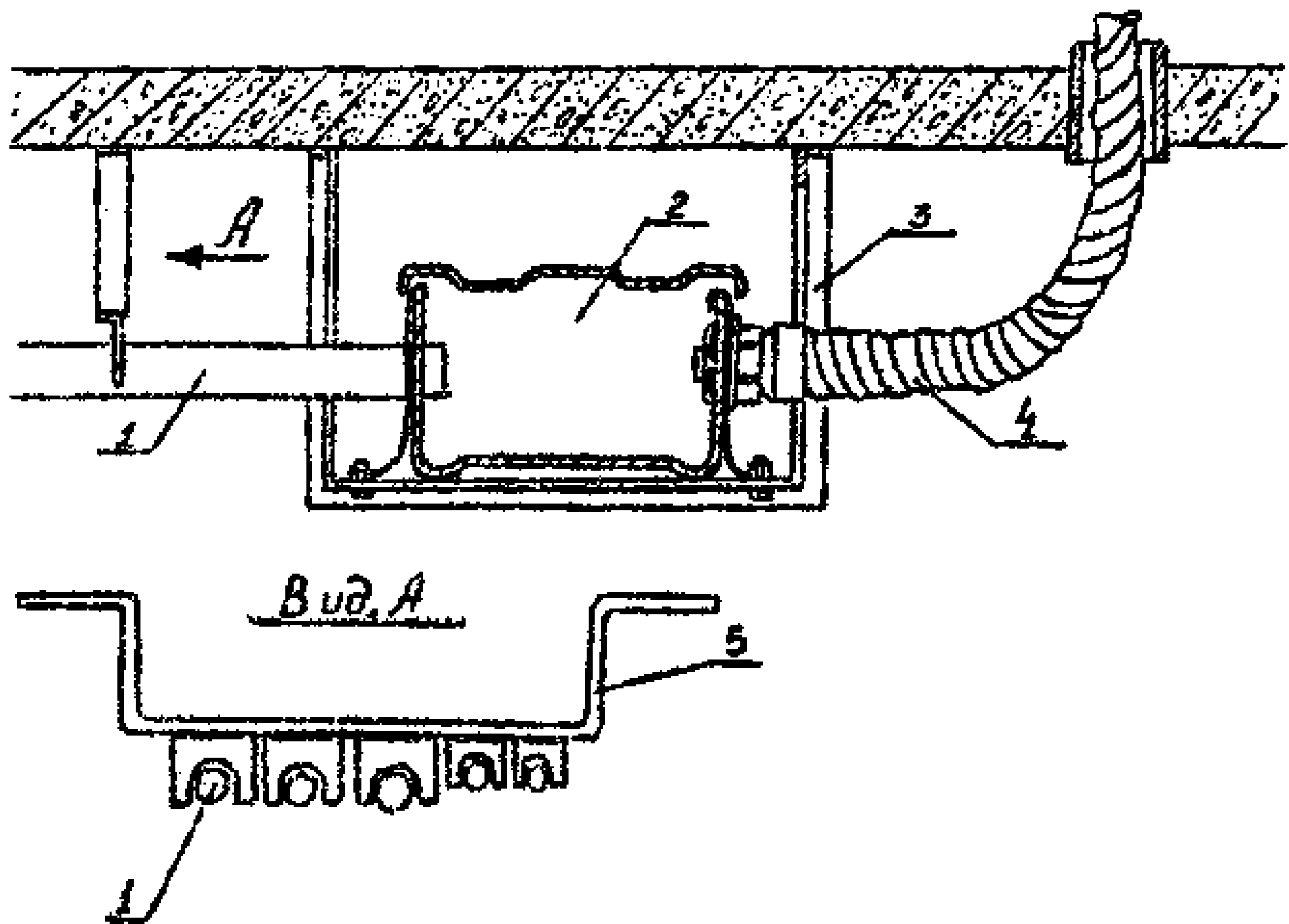
Рис.4. Ввод проводов и кабелей в короб:
