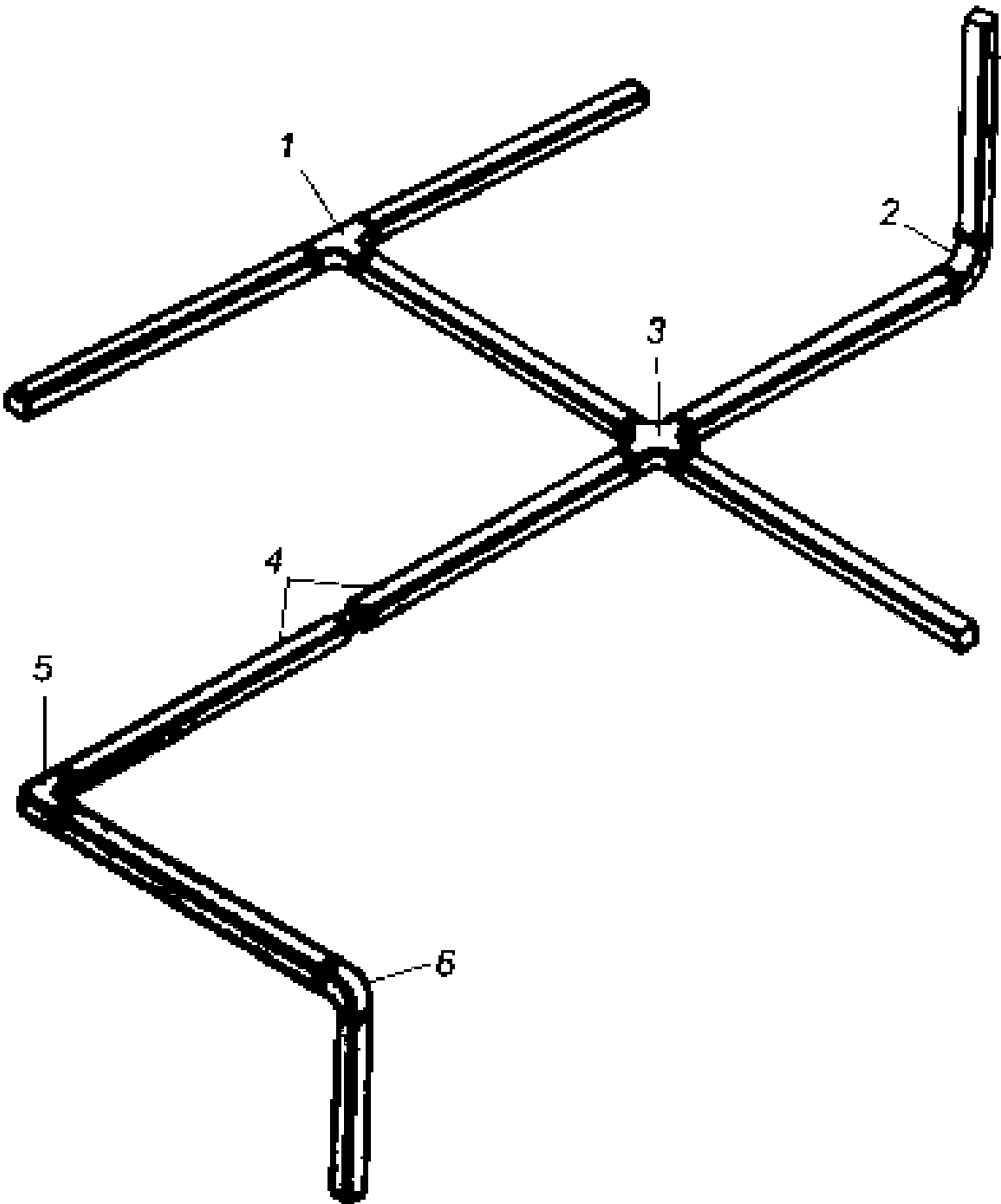
Рис.2. Прокладка трассы из одноканальных металлических коробов:
