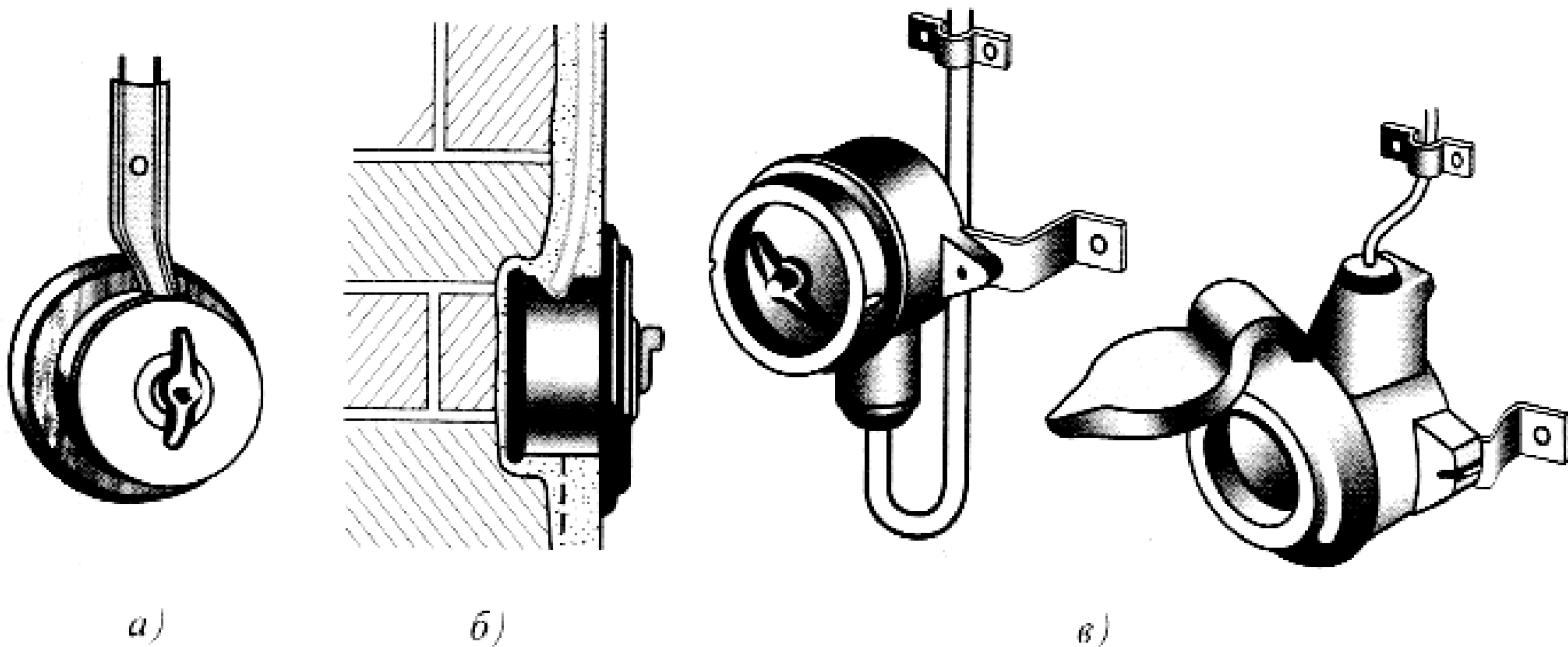
Рис.15. Примеры монтажа установочных приборов:
