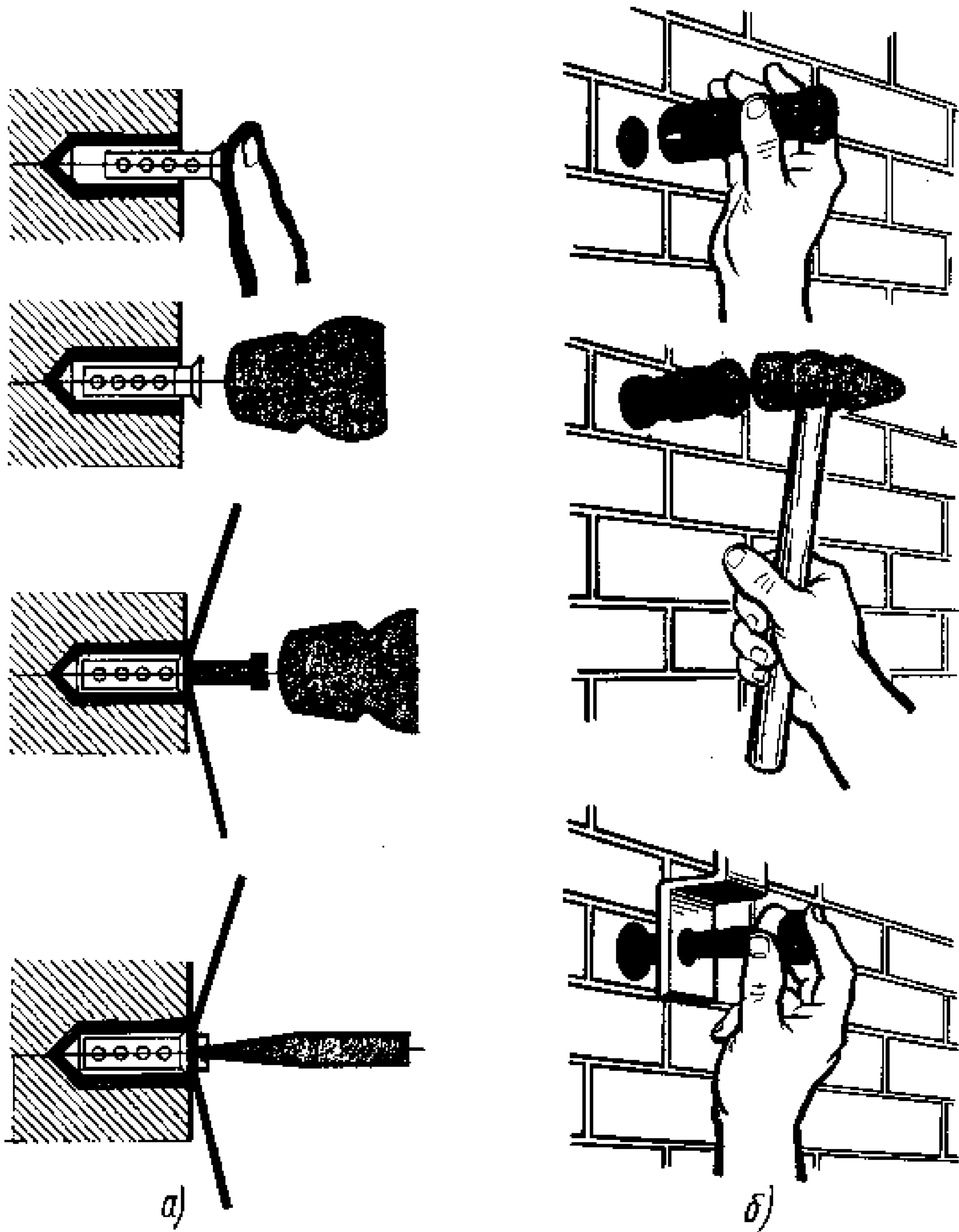
Рис.13. Последовательность операций установки и закрепления распорных дюбелей:
