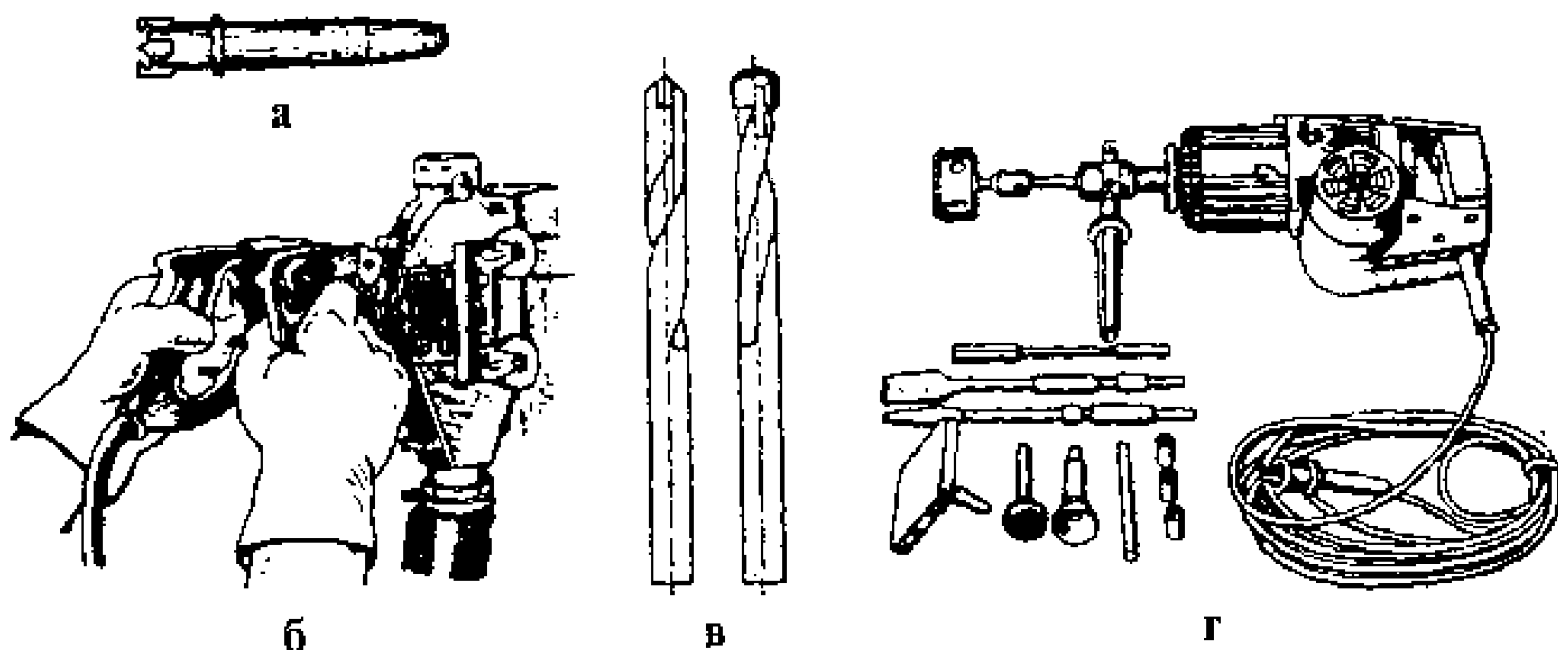
Рис.10. Инструмент, механизмы и приспособления для пробивных работ:
