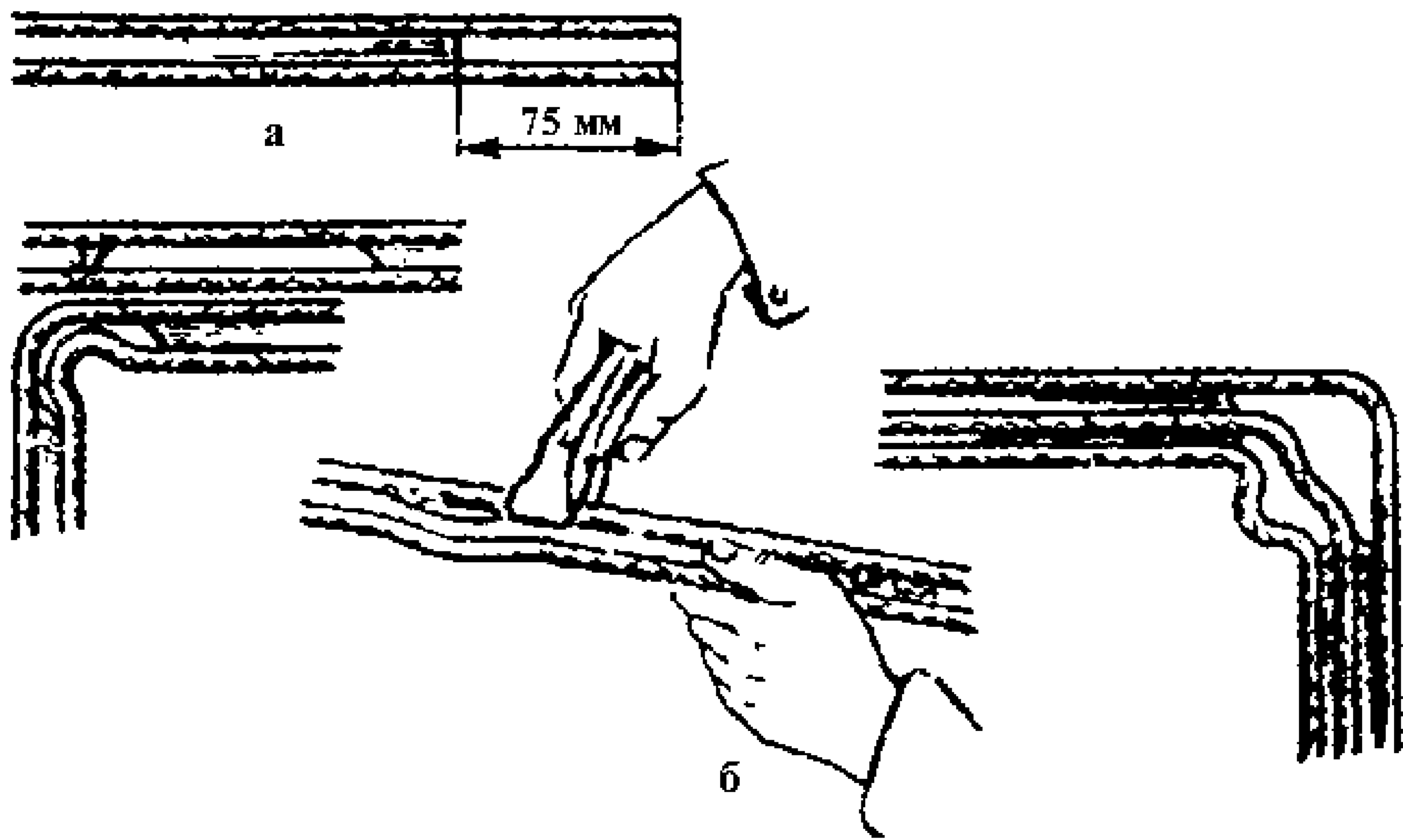
Рис.11. Операции подготовки плоского провода перед монтажом:
