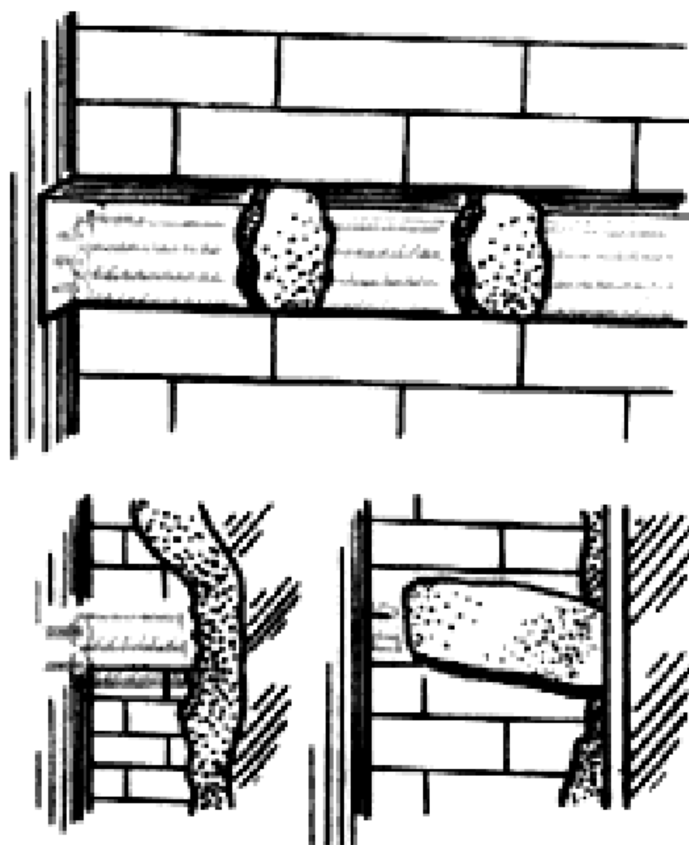
Рис.3. Скрытые электропроводки под несгораемыми основаниями
