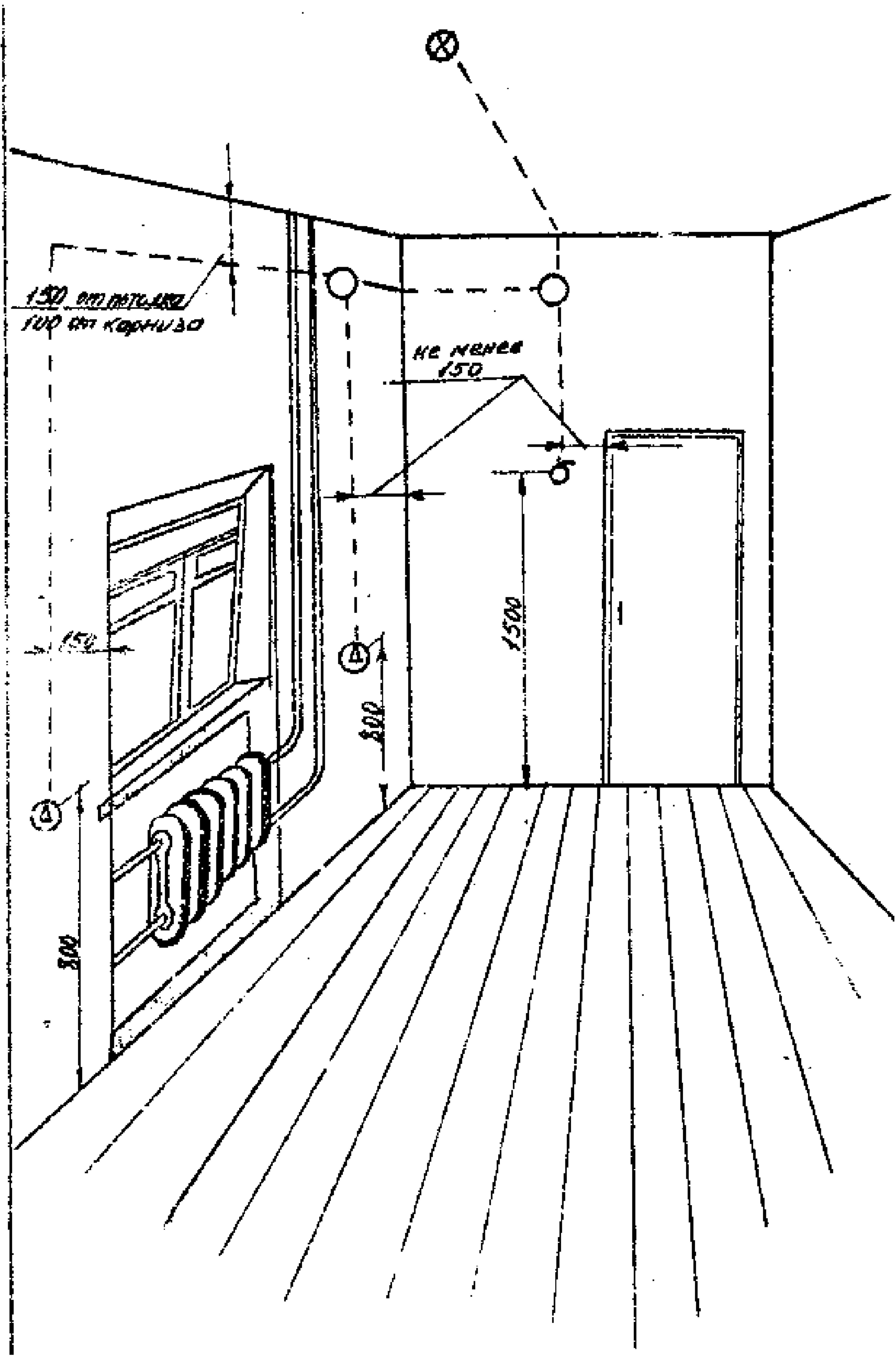
Рис.1. Размещение электроустановочных изделий и групповой сети
