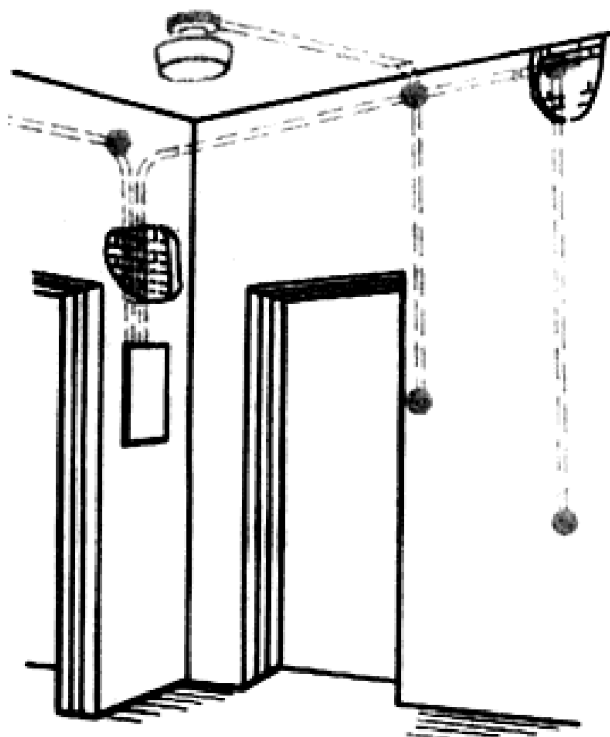
Рис.2. Скрытые электропроводки под слоем мокрой штукатурки
