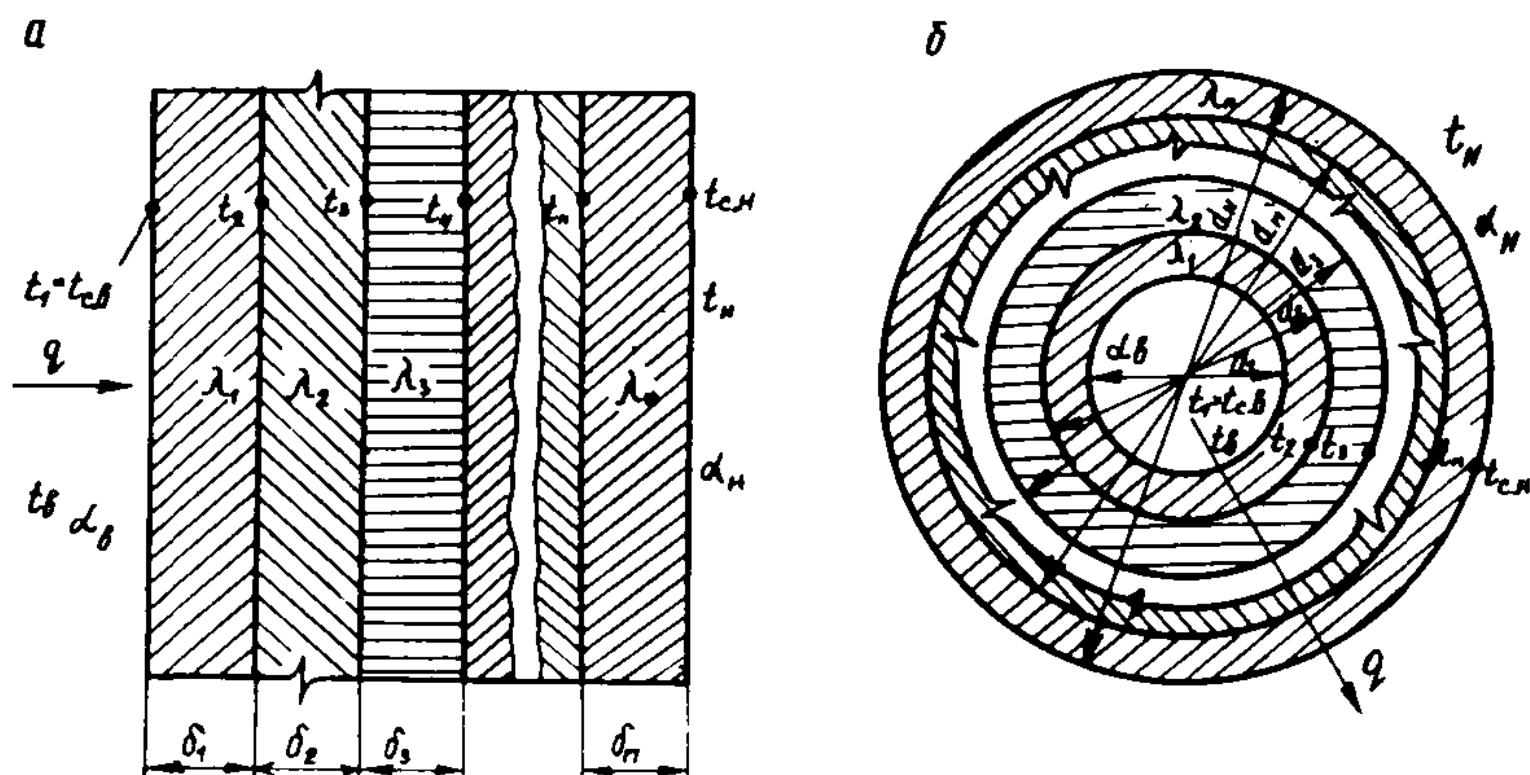
Рис. 1. Расчетная схема многослойной стенки: а-плоской; б-цилиндрической
