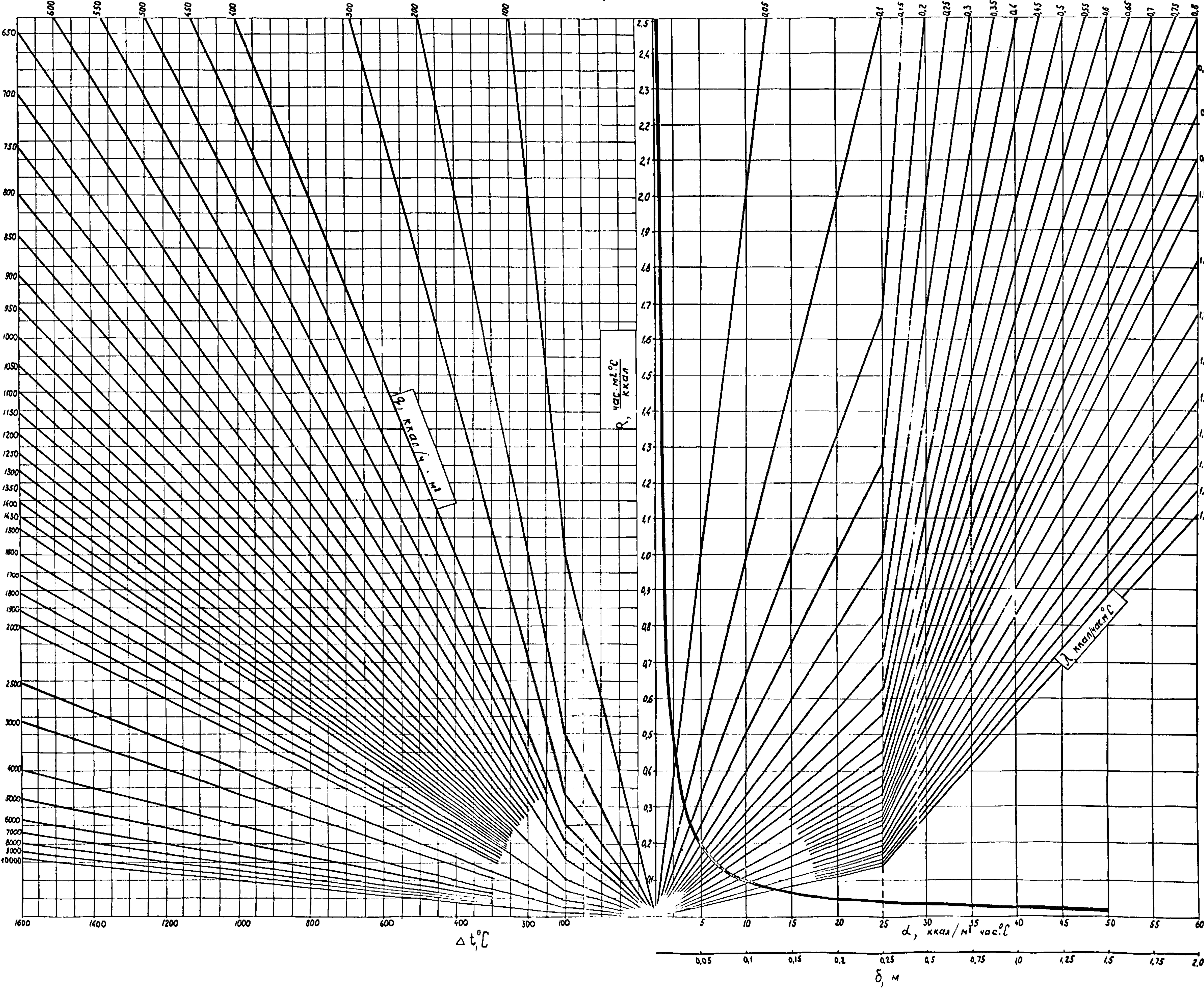
График для расчёта плоской стенки
