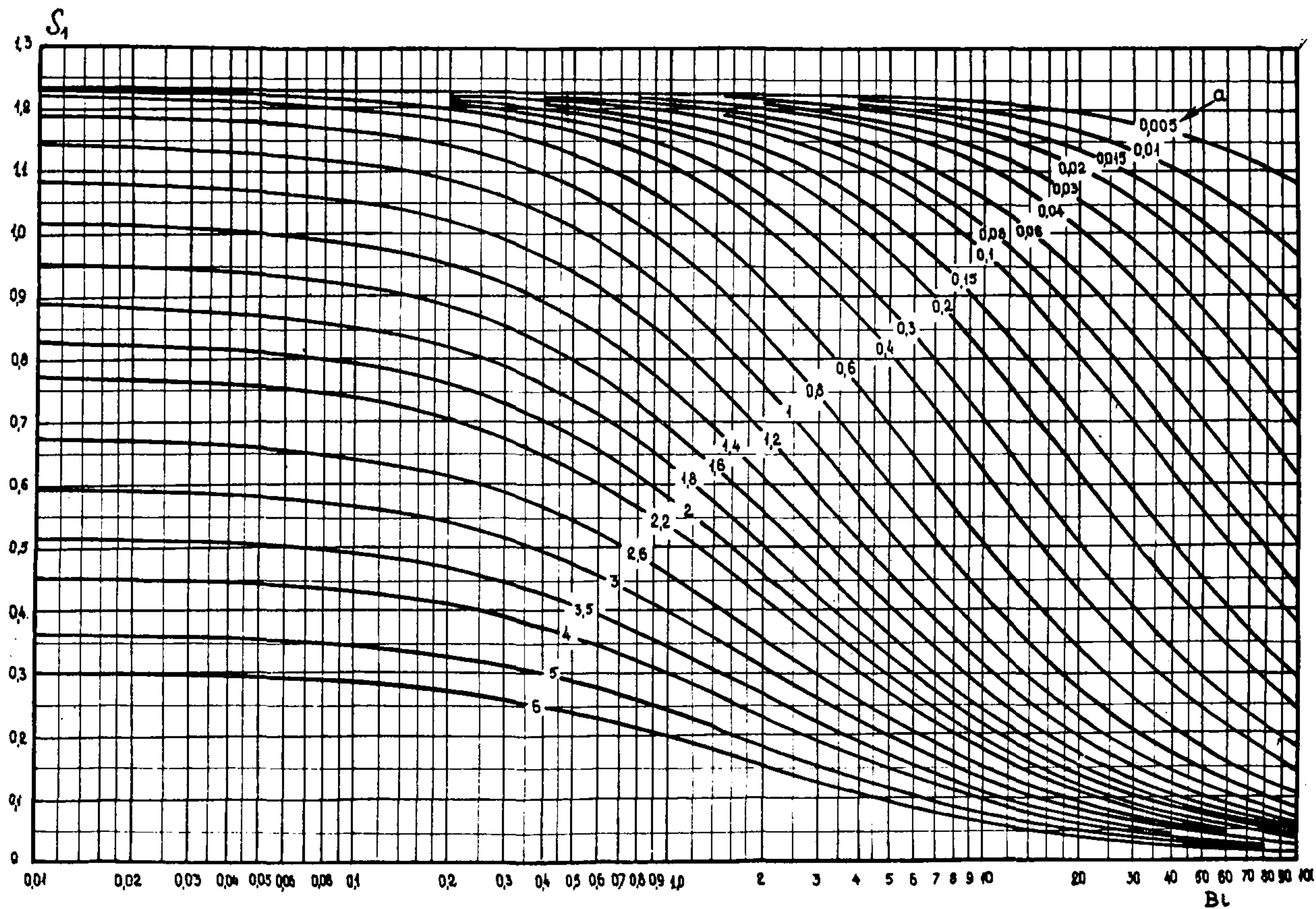
График для определения величин \Sigma_1, \Sigma_2
