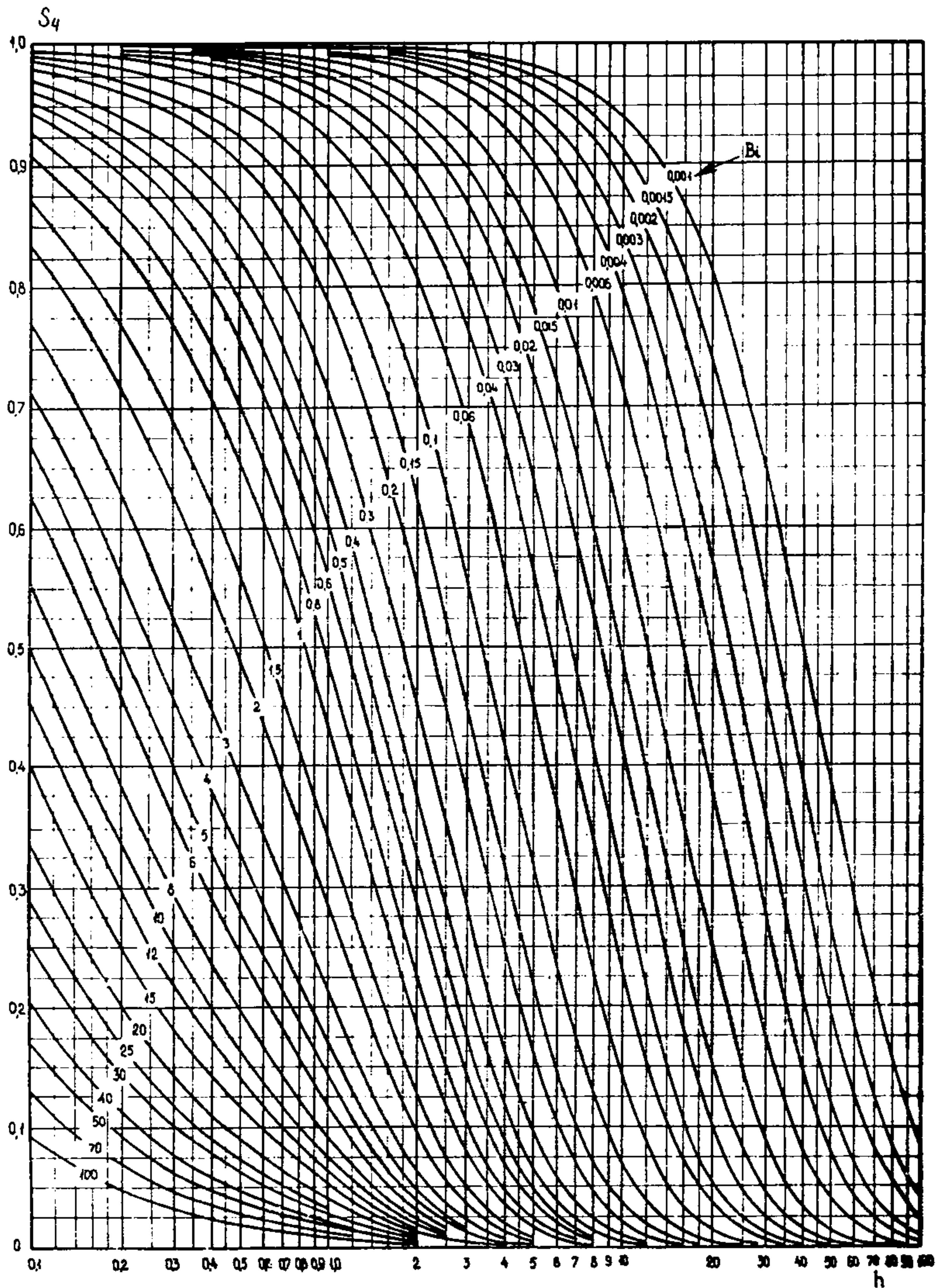
График для определения величины S_4
