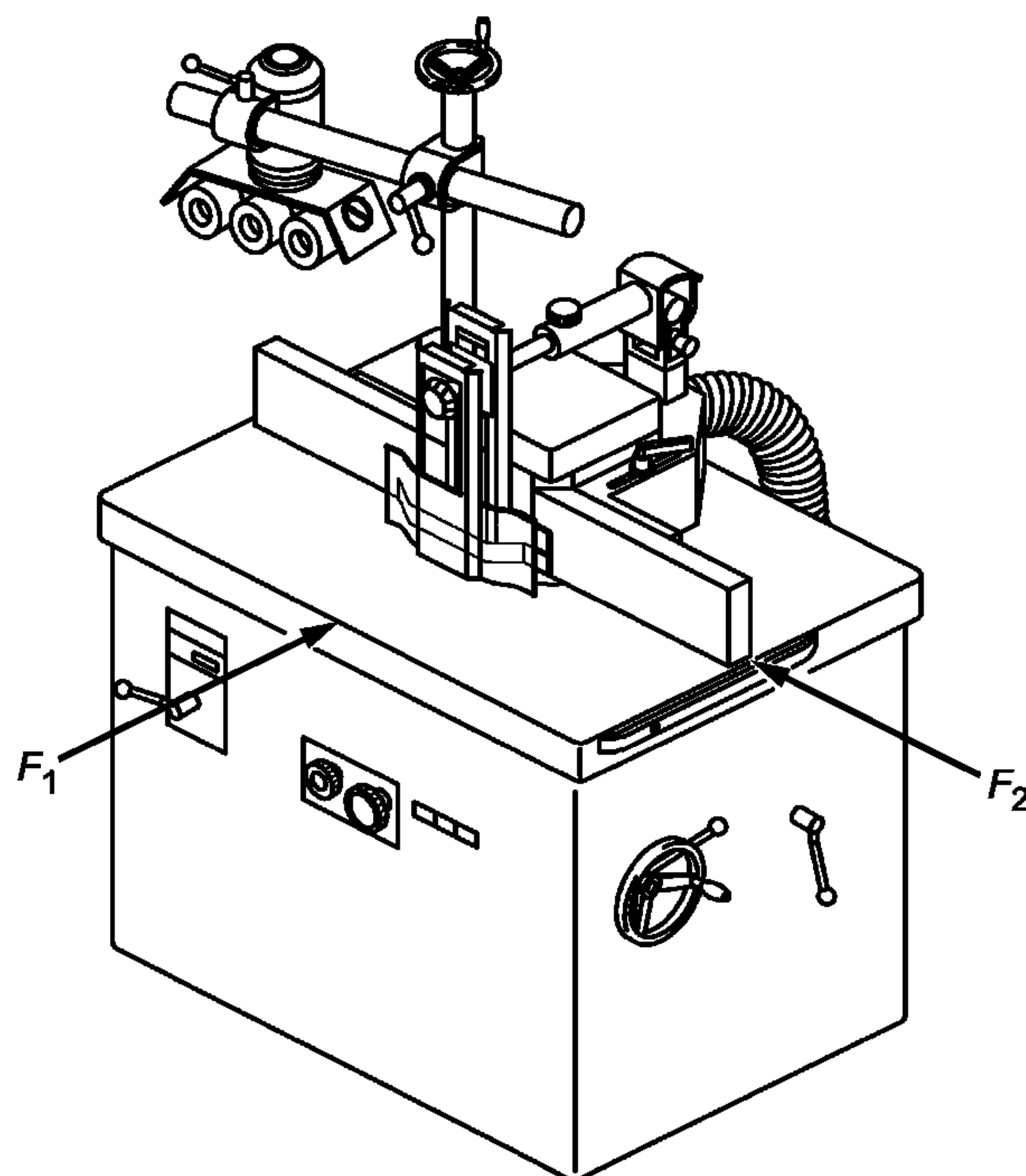
Рисунок С.1 — Испытание на устойчивость передвижных станков
