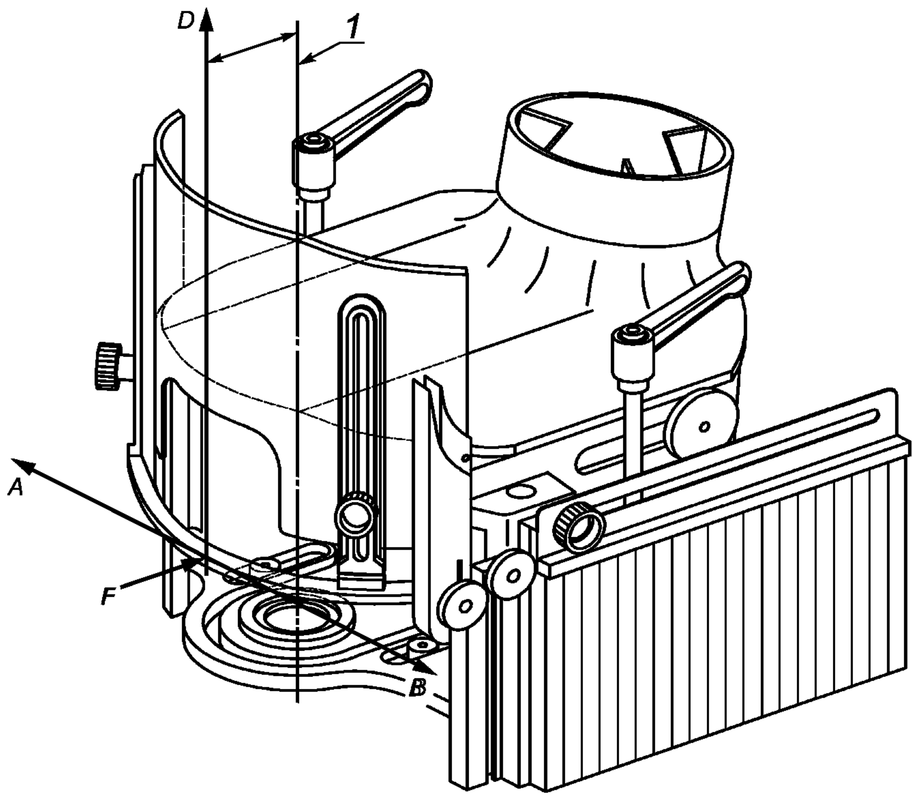
1 — ось шпинделя
