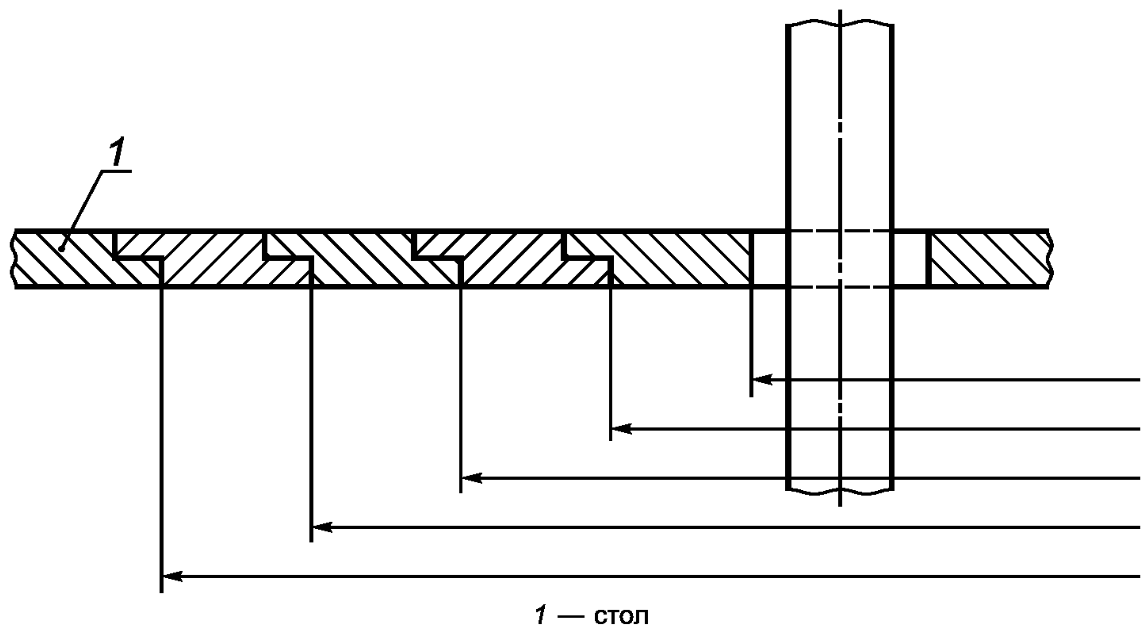
Рисунок 15 — Кольца стола
