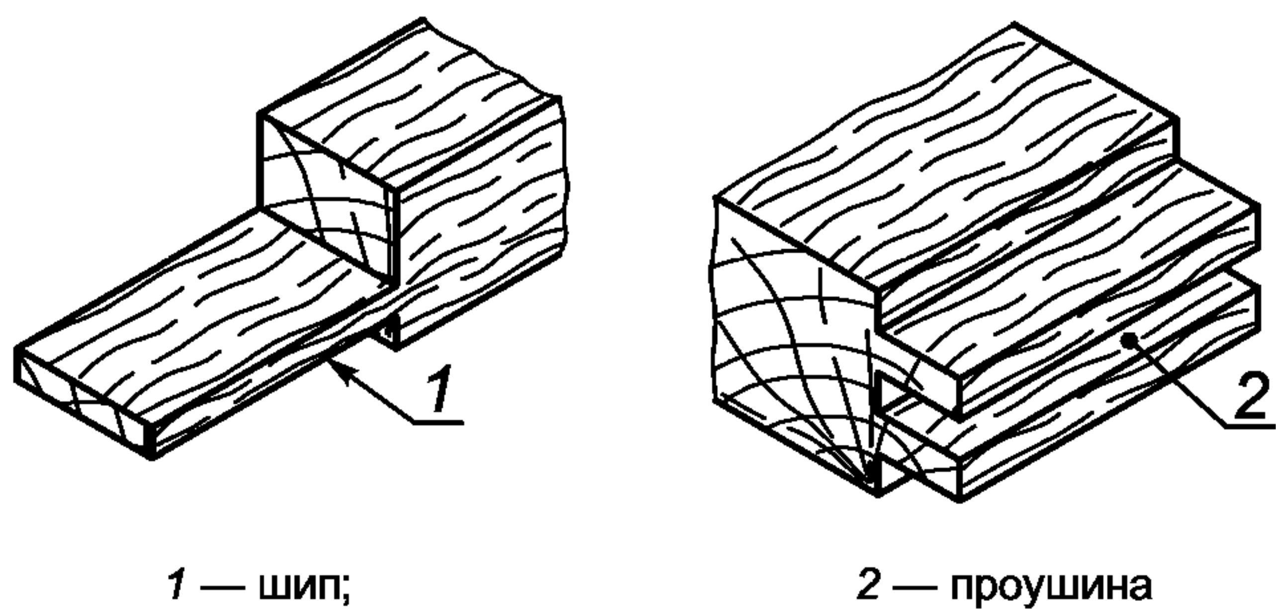
Рисунок 3 — Пример обработанной заготовки с шипом/проушиной
