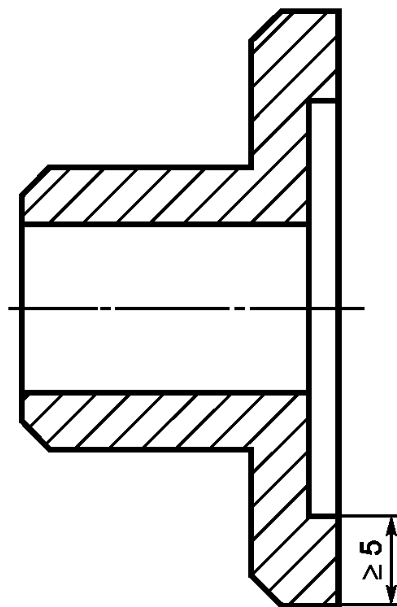
Рисунок 10 — Фланец для крепления дисковой пилы
