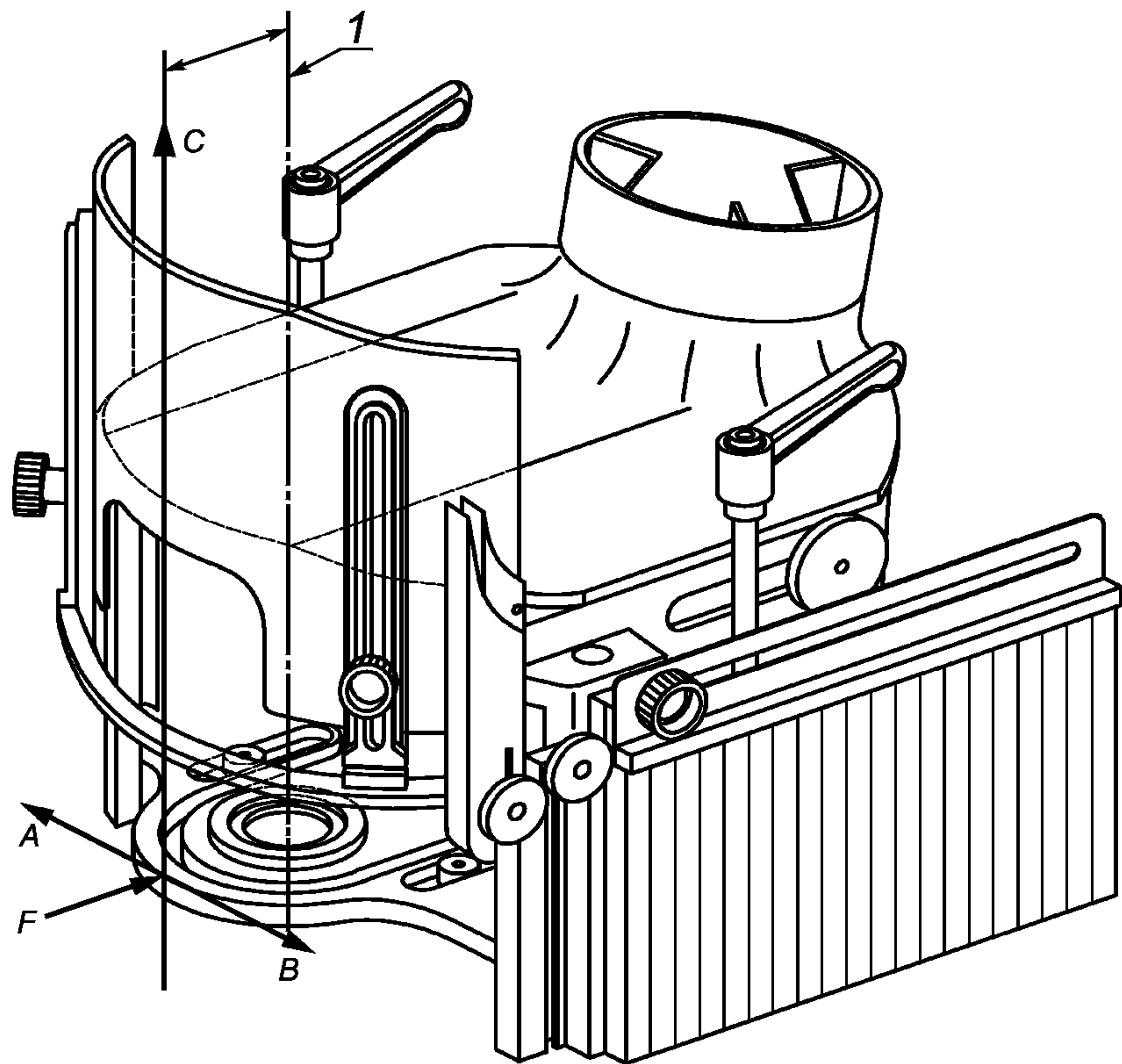
1 — ось шпинделя
