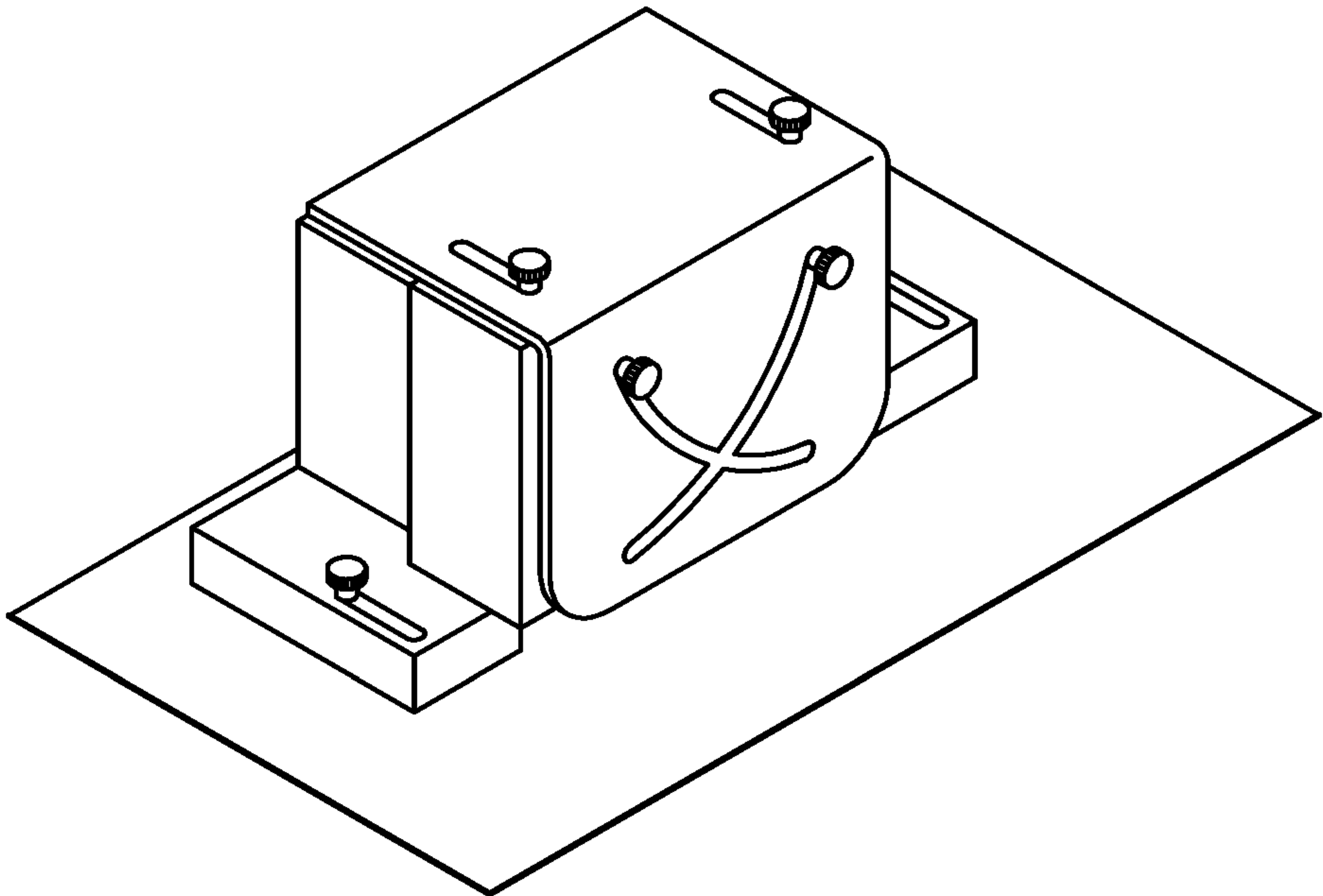
Рисунок 6d) — Пример перемещаемого саморегулируемого защитного ограждения на фрезерном станке, оборудованном для нарезания шипов Рисунок 6 — Фрезерный одношпиндельный станок с вертикальным нижним расположением шпинделя
