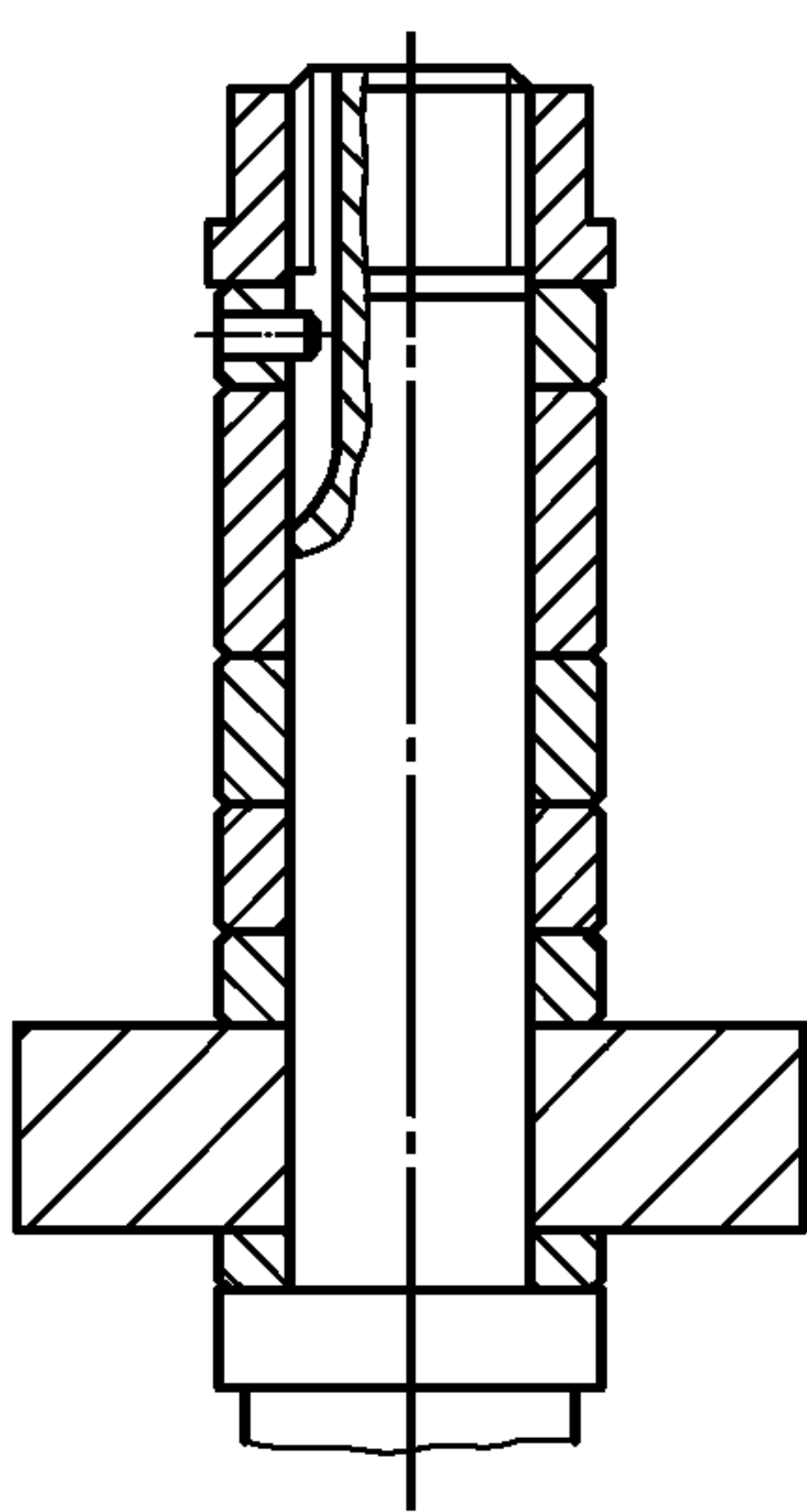
Рисунок 9а) — Пример применения фиксирующего штифта в шпиндельном кольце
