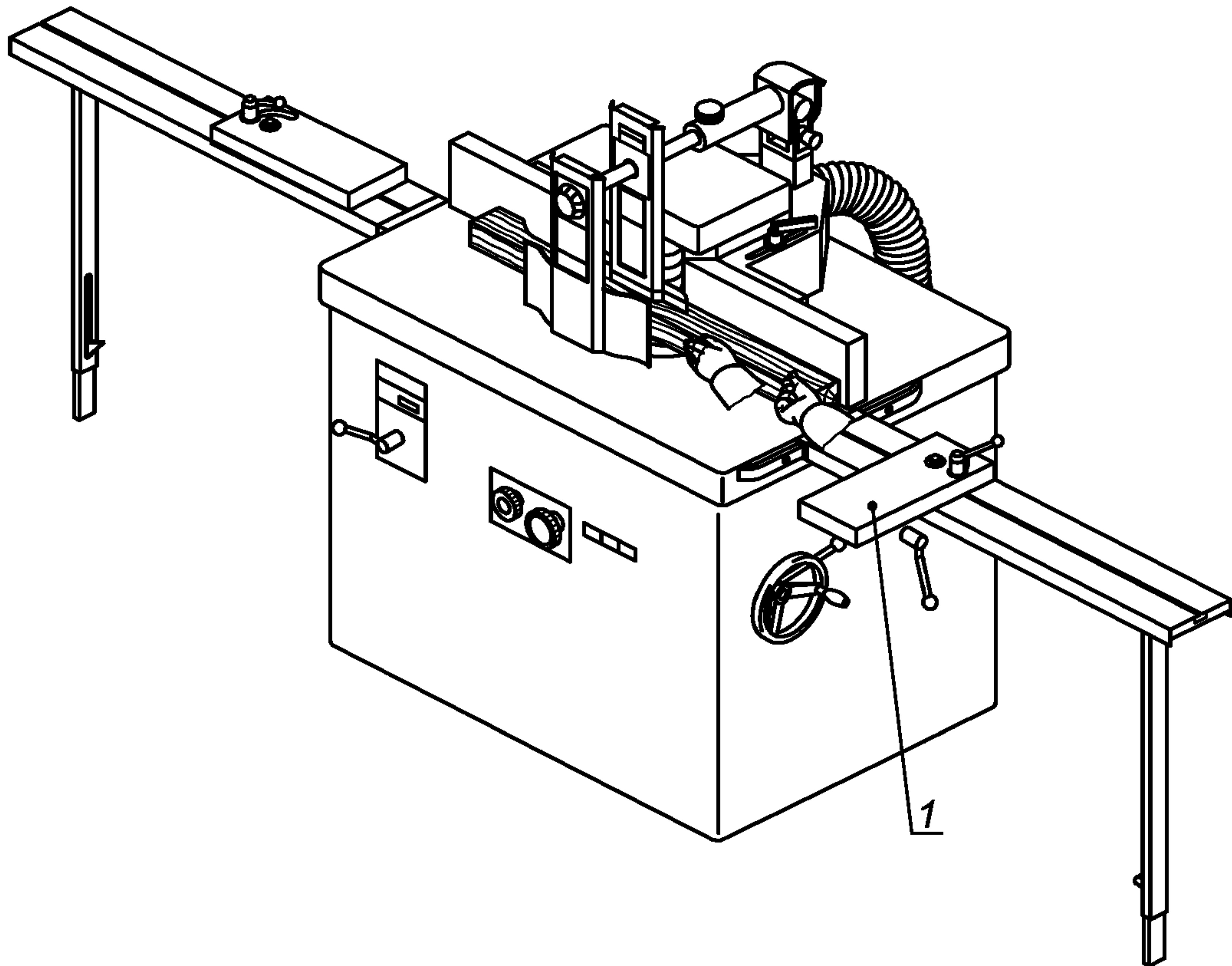
Рисунок 4 — Пример ограниченной прямолинейной обработки
