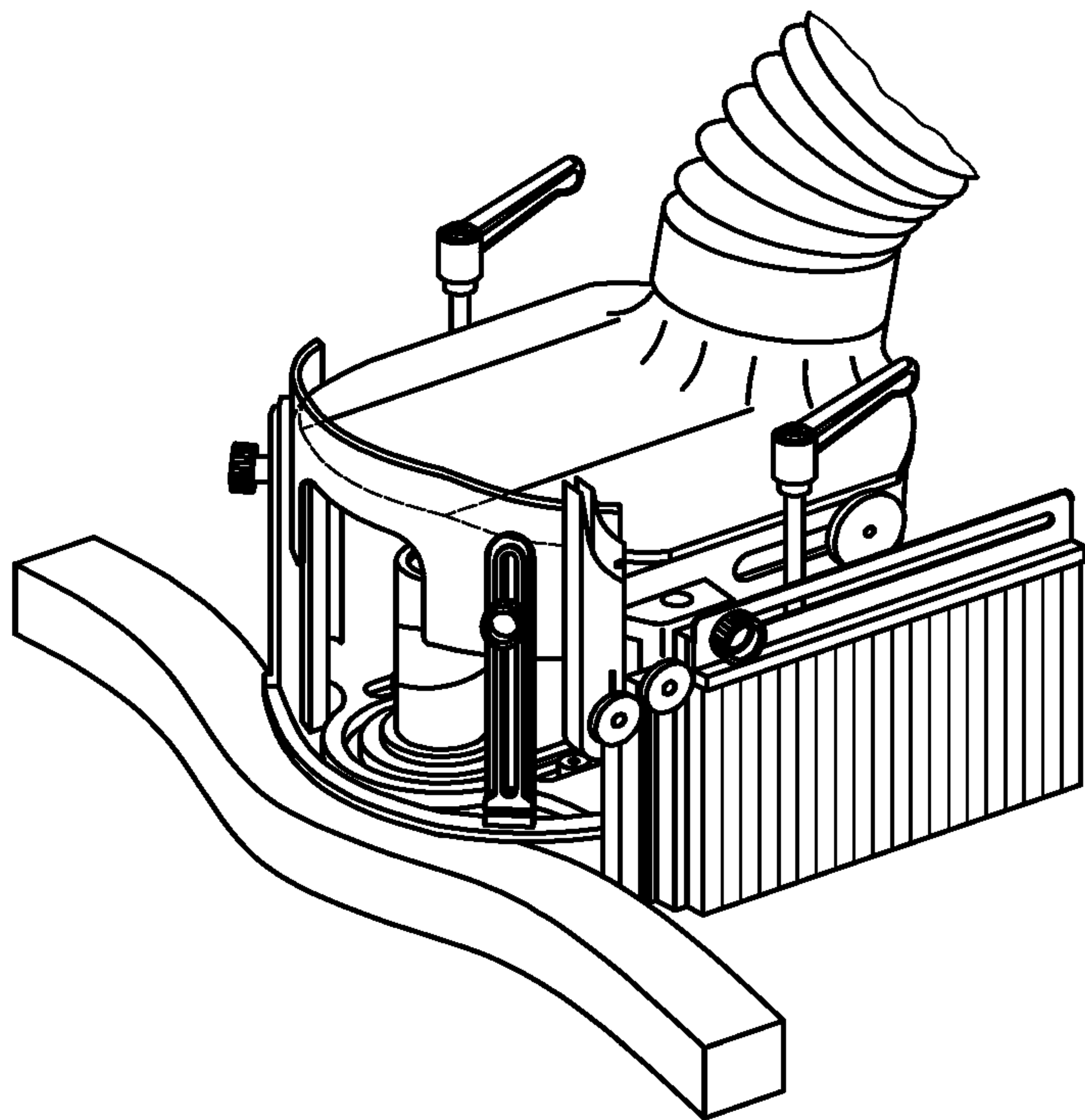
Рисунок 2 — Пример криволинейного фрезерования
