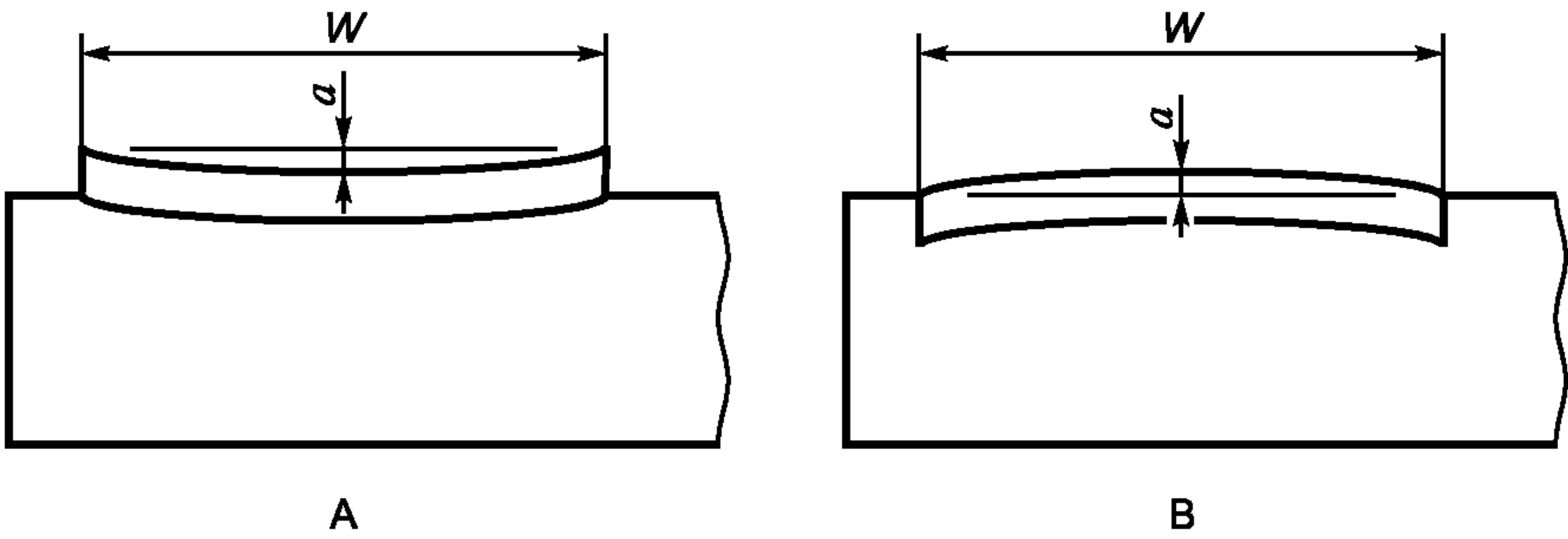
Рисунок 3 — Профиль поверхности
