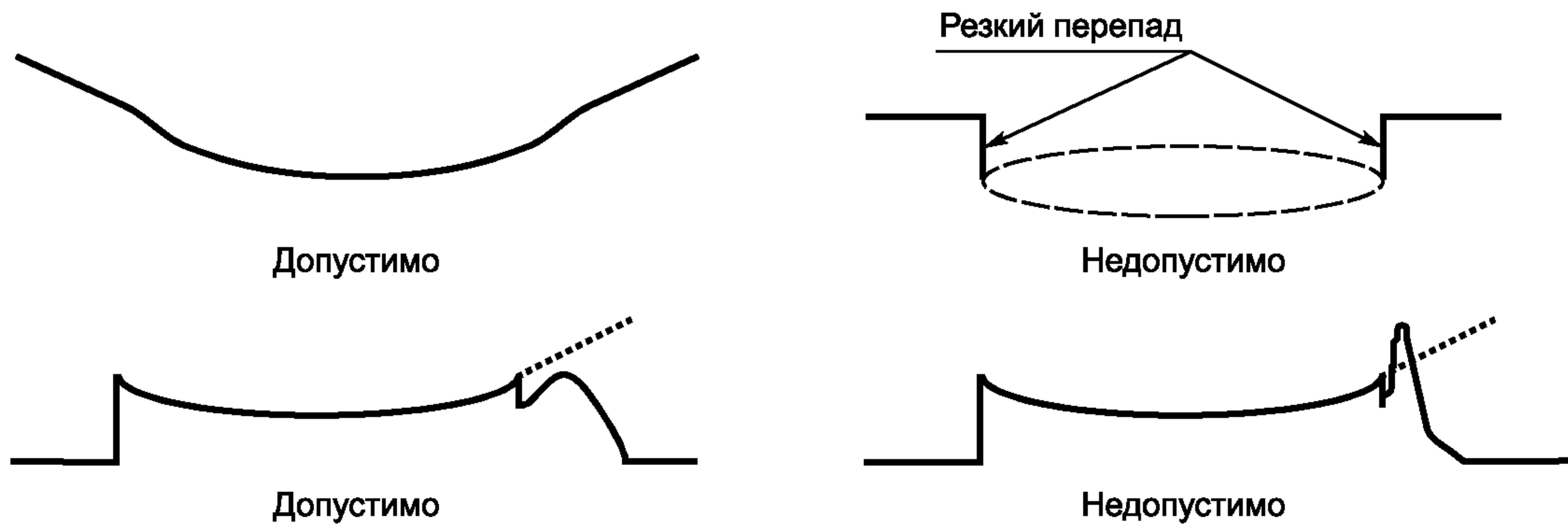
Рисунок 4 — Примеры профилей поверхности
