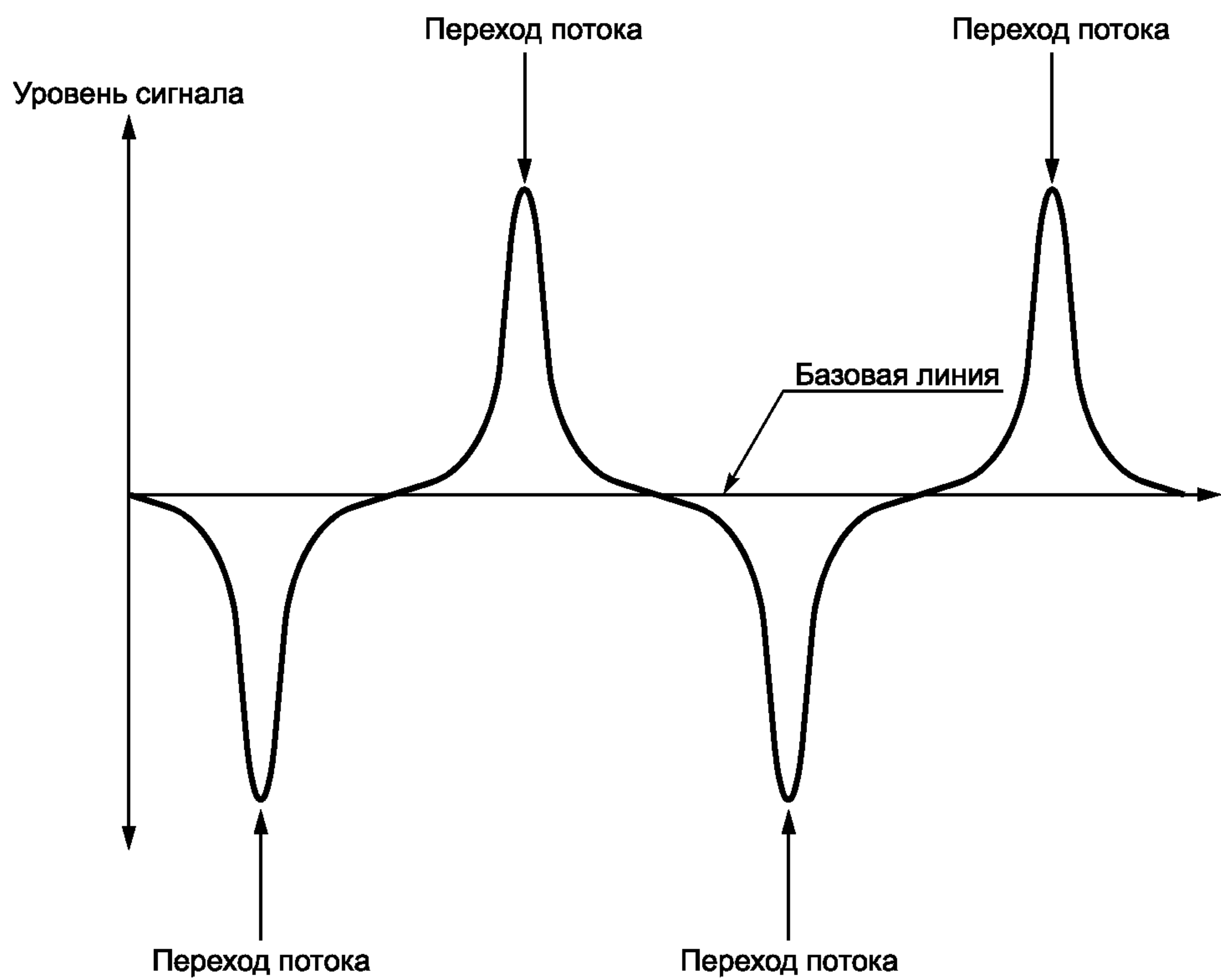
Рисунок 7 — Пример формы сигнала
