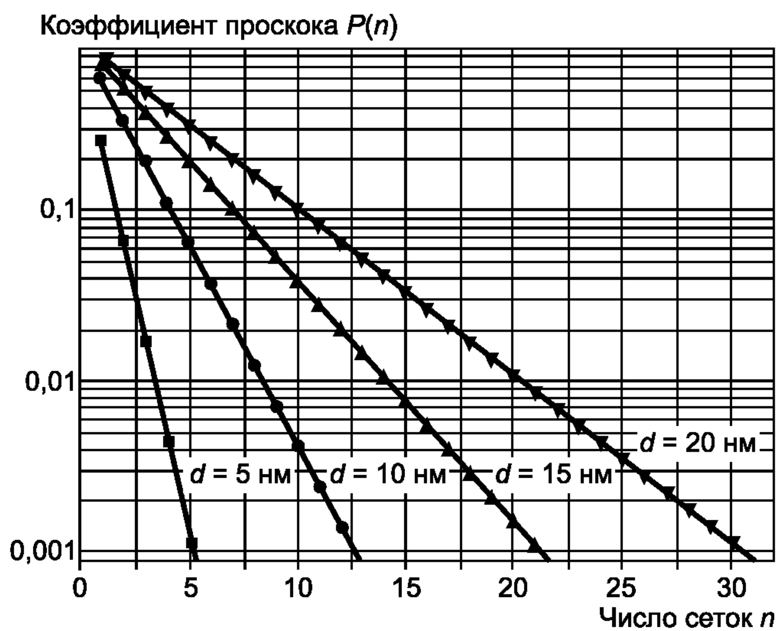
Рисунок А.1 — Теоретическая зависимость коэффициента проскока аэрозольных частиц размерами от 5 до 20 нм от числа сеток при скорости потока аэрозоля 1 дм³/мин
