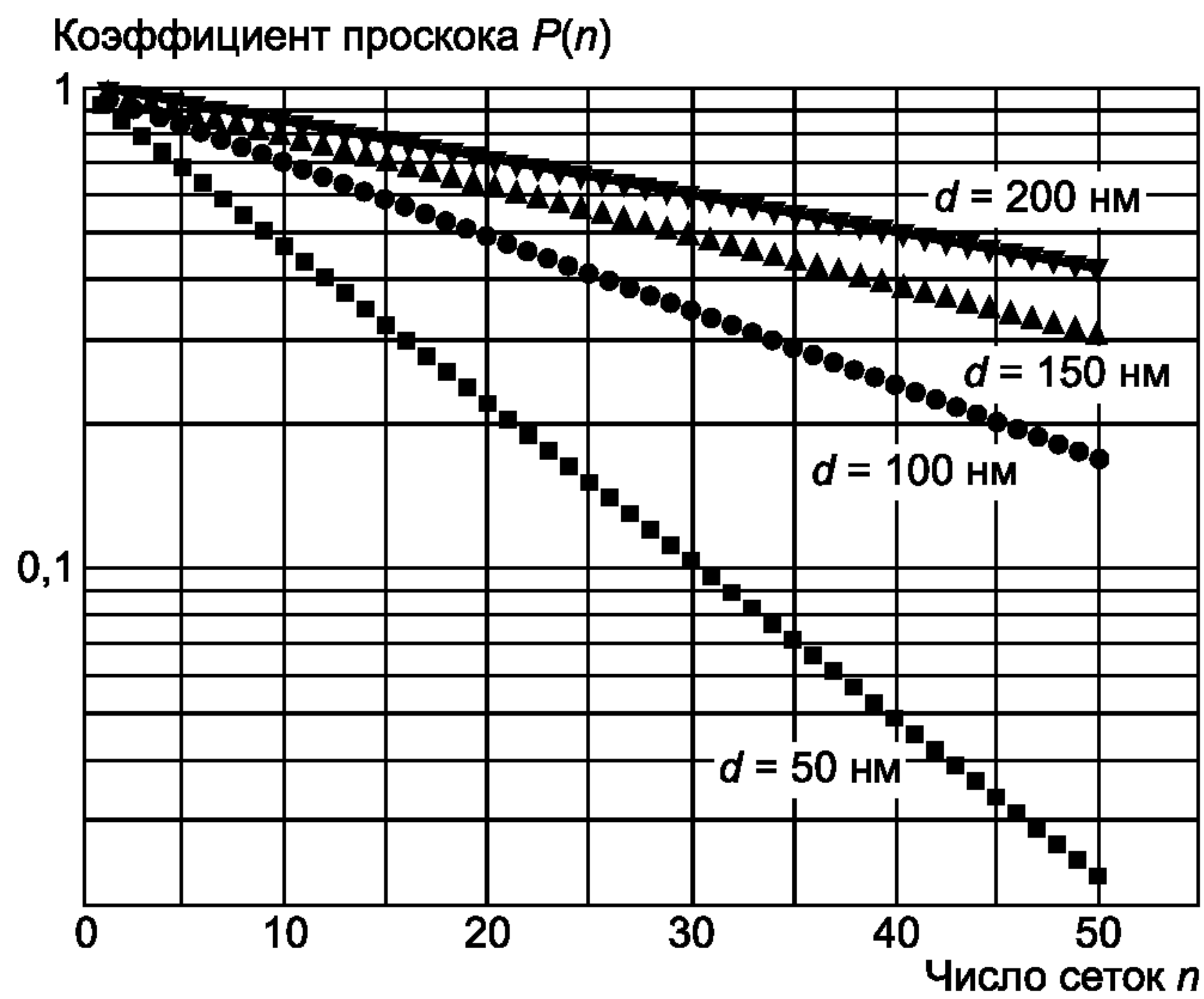
Рисунок А.2 — Теоретическая зависимость коэффициента проскока частиц размерами от 50 до 200 нм от числа сеток при скорости потока аэрозоля 1 дм³/мин
