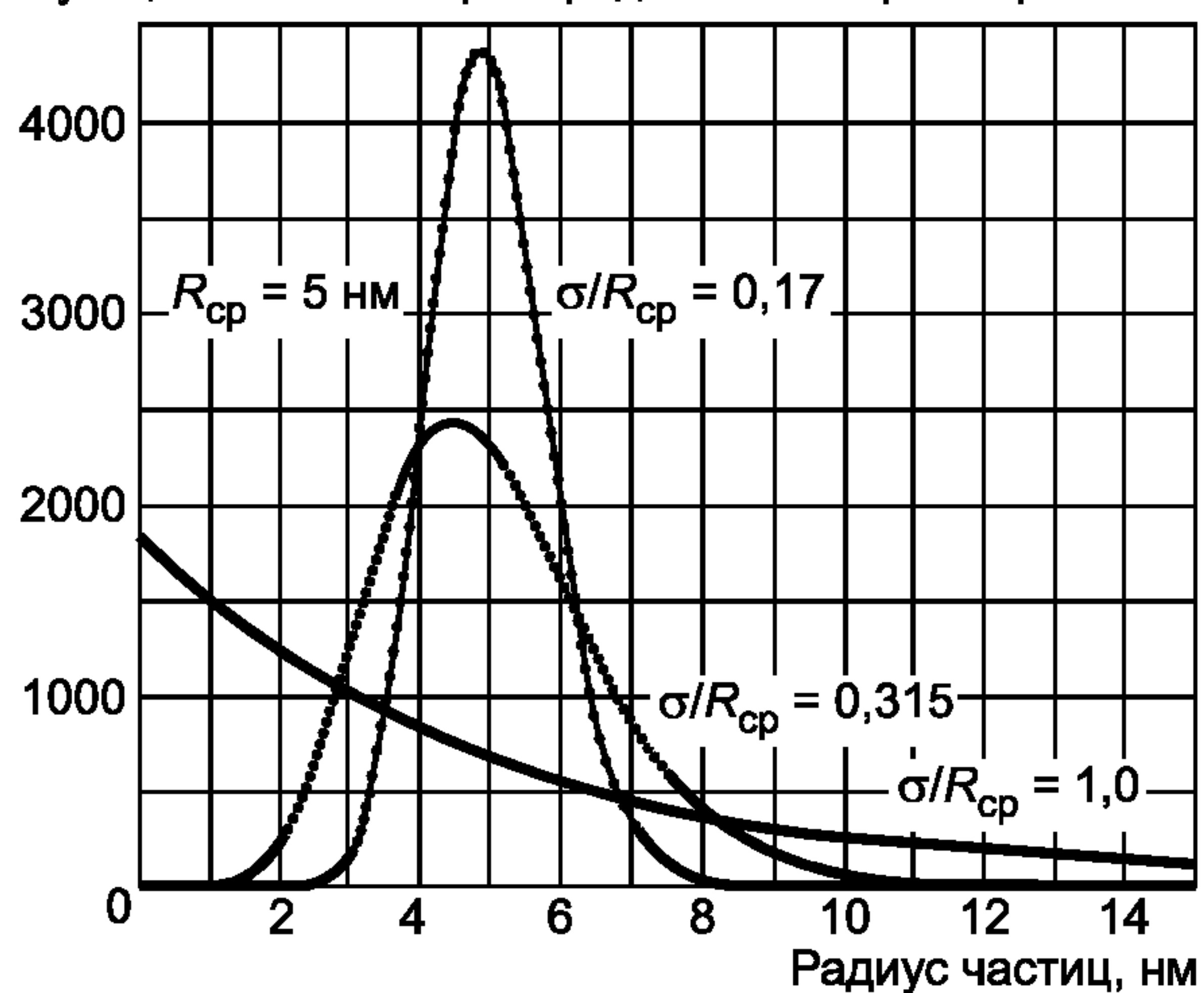
Функция плотности распределения по размерам
