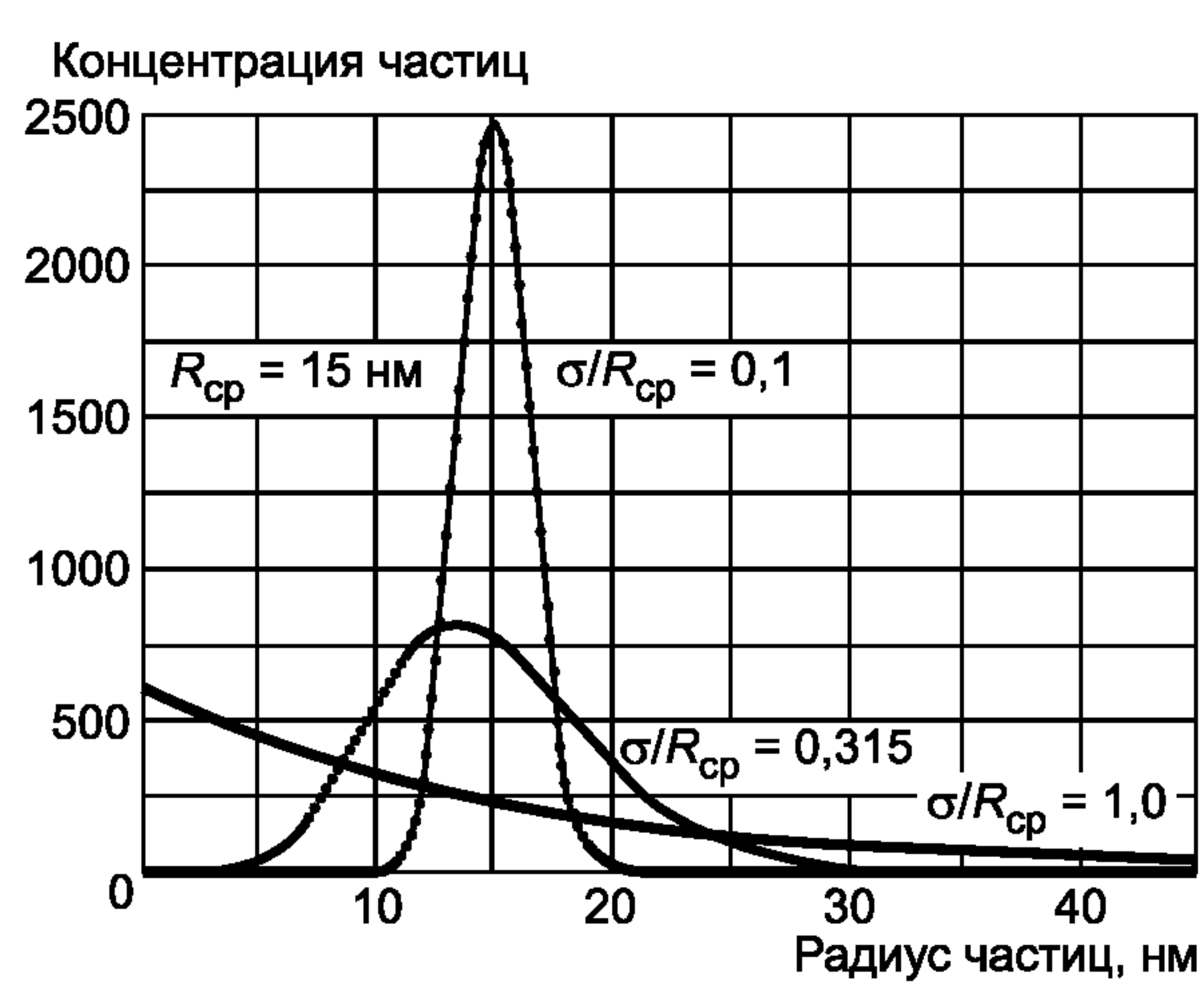
а) Функция f(d)
