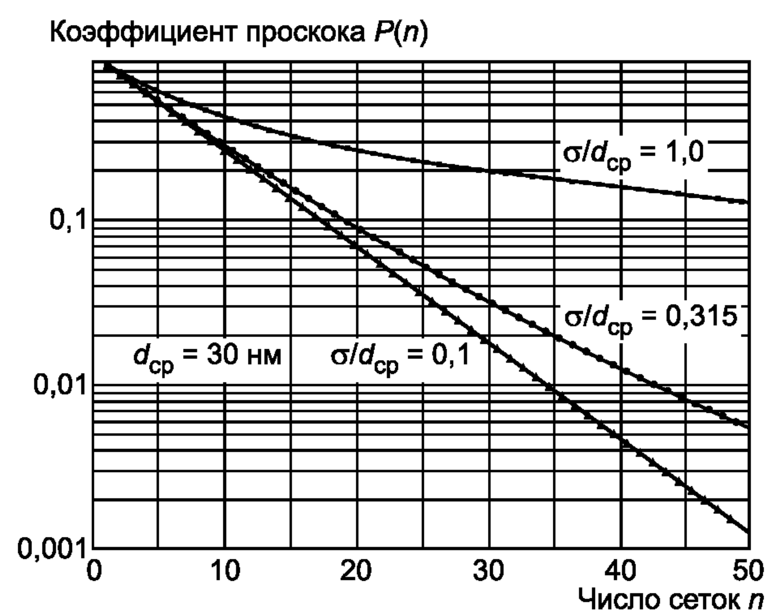
б) Функция P(n)
