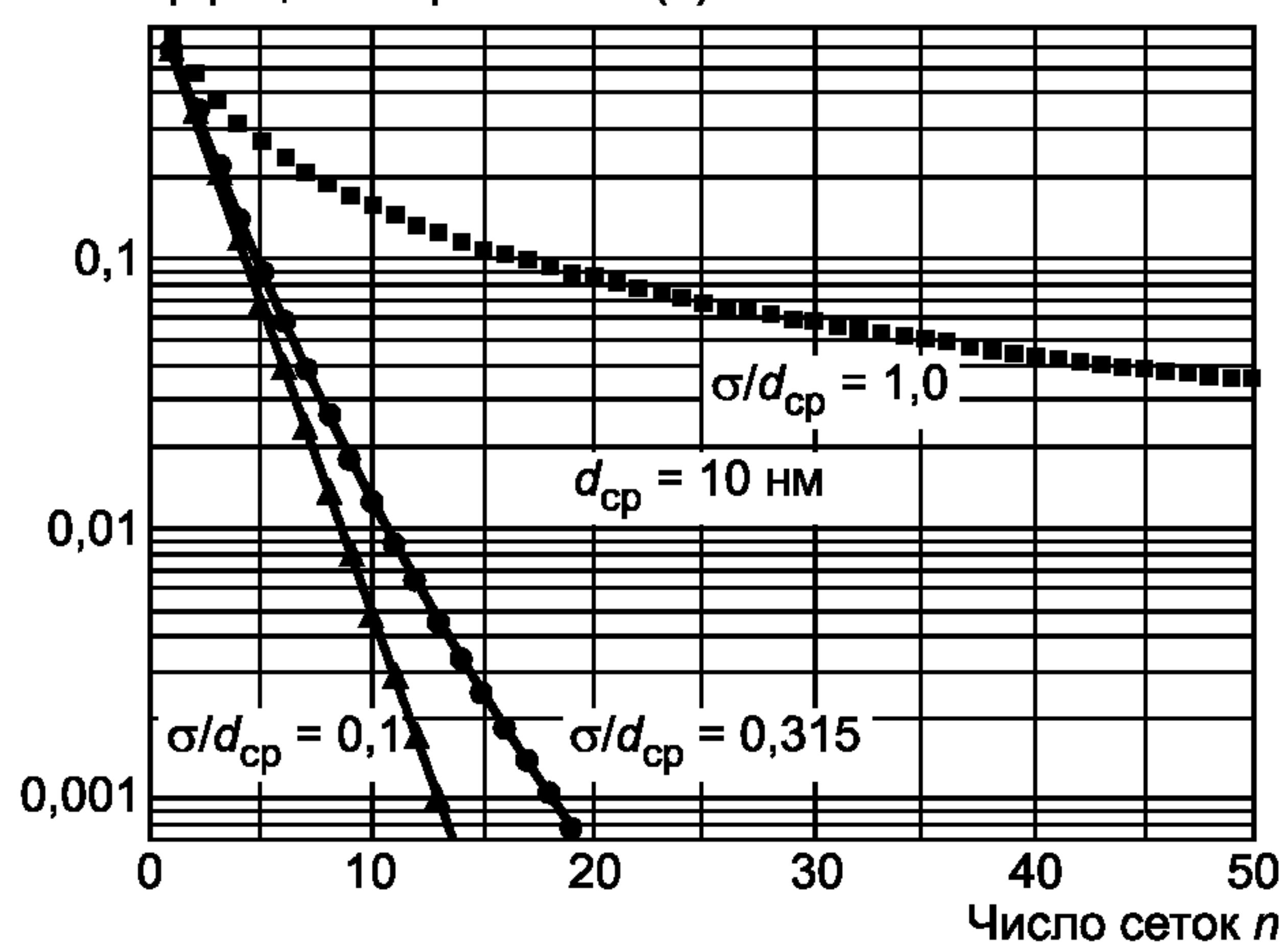
Коэффициент проскока P(n)
