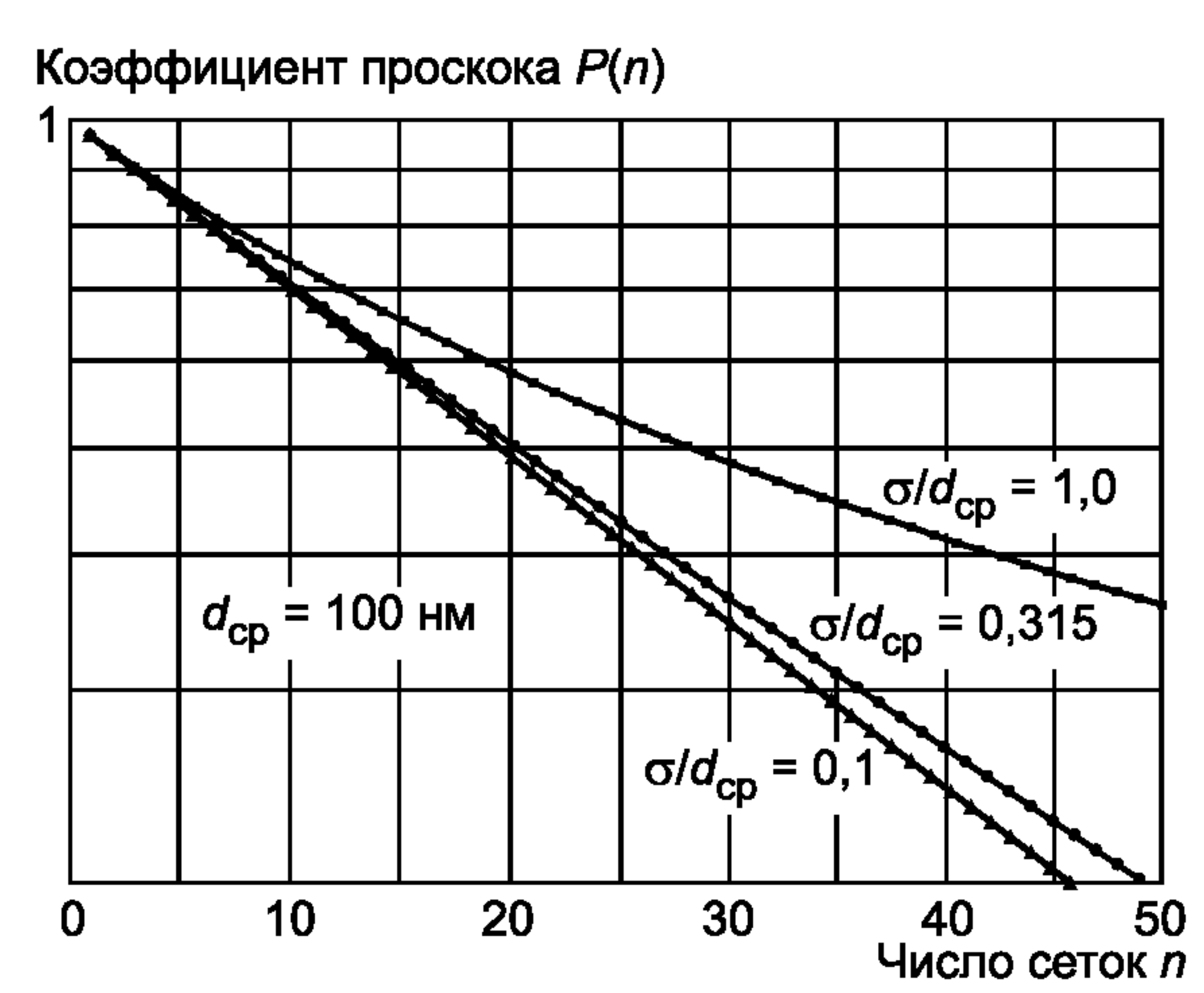
б) Функция P(n)
