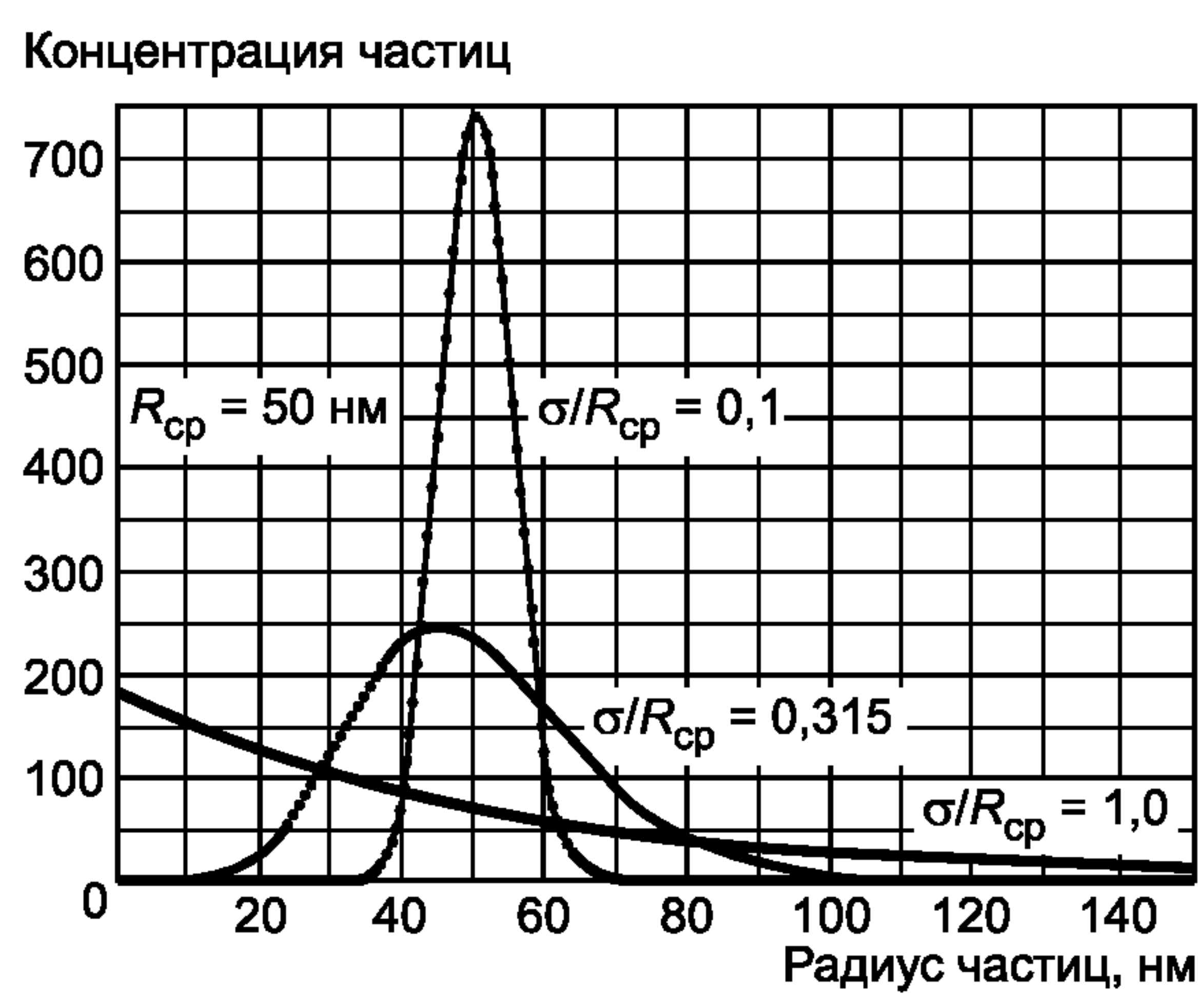
а) Функция f(d)
