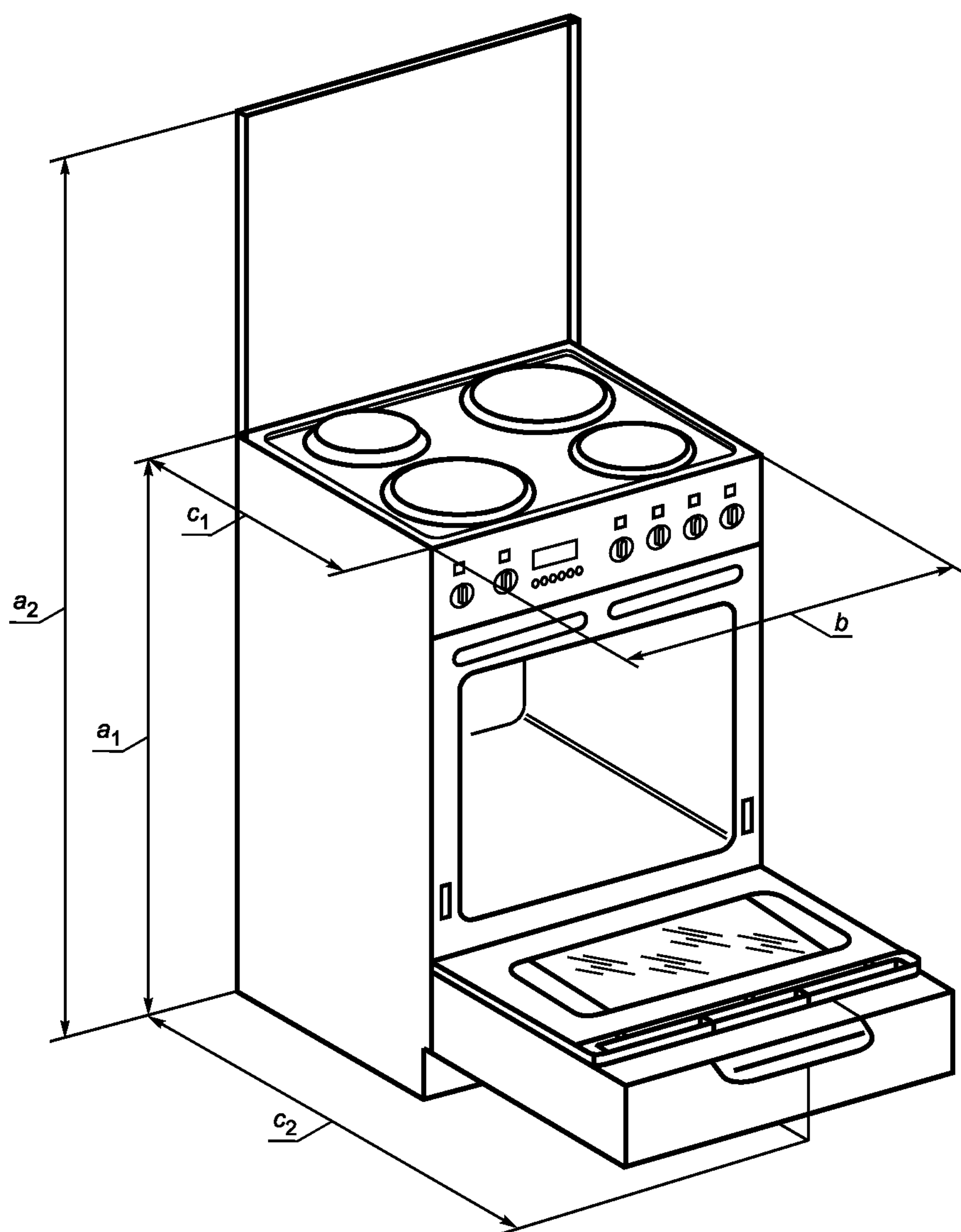
Рисунок 1 — Размеры приборов
