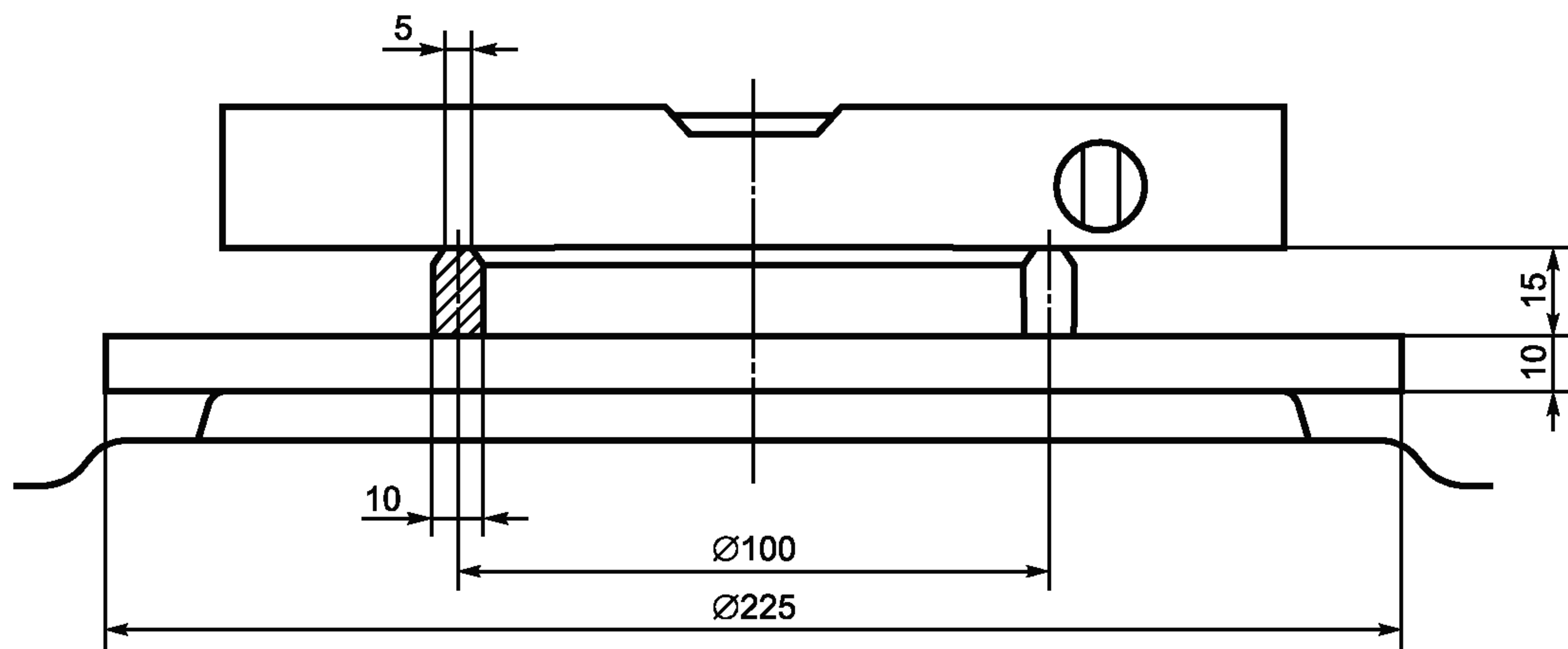
Рисунок 5 — Устройство для проверки уровня конфорок и противней
