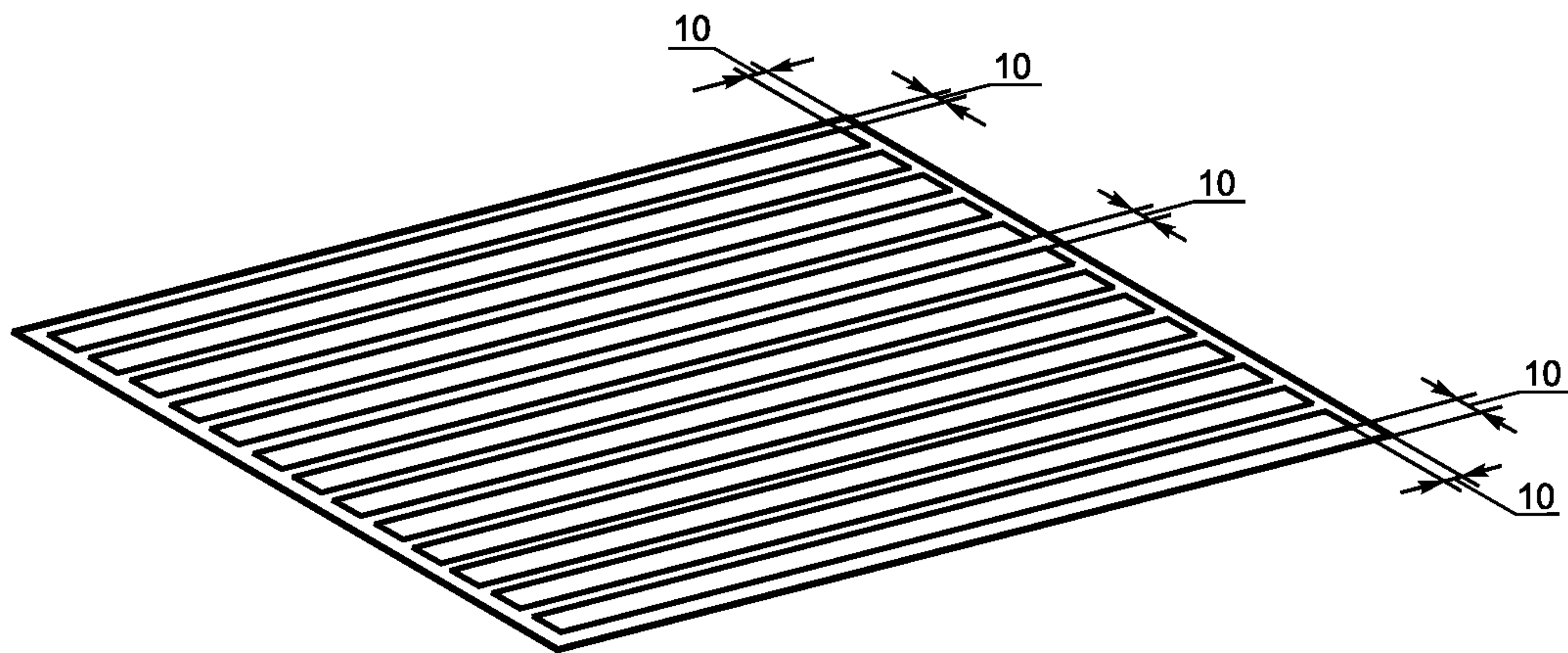
Рисунок 10 — Расположение полосок для выпечки на противне для выпекания
