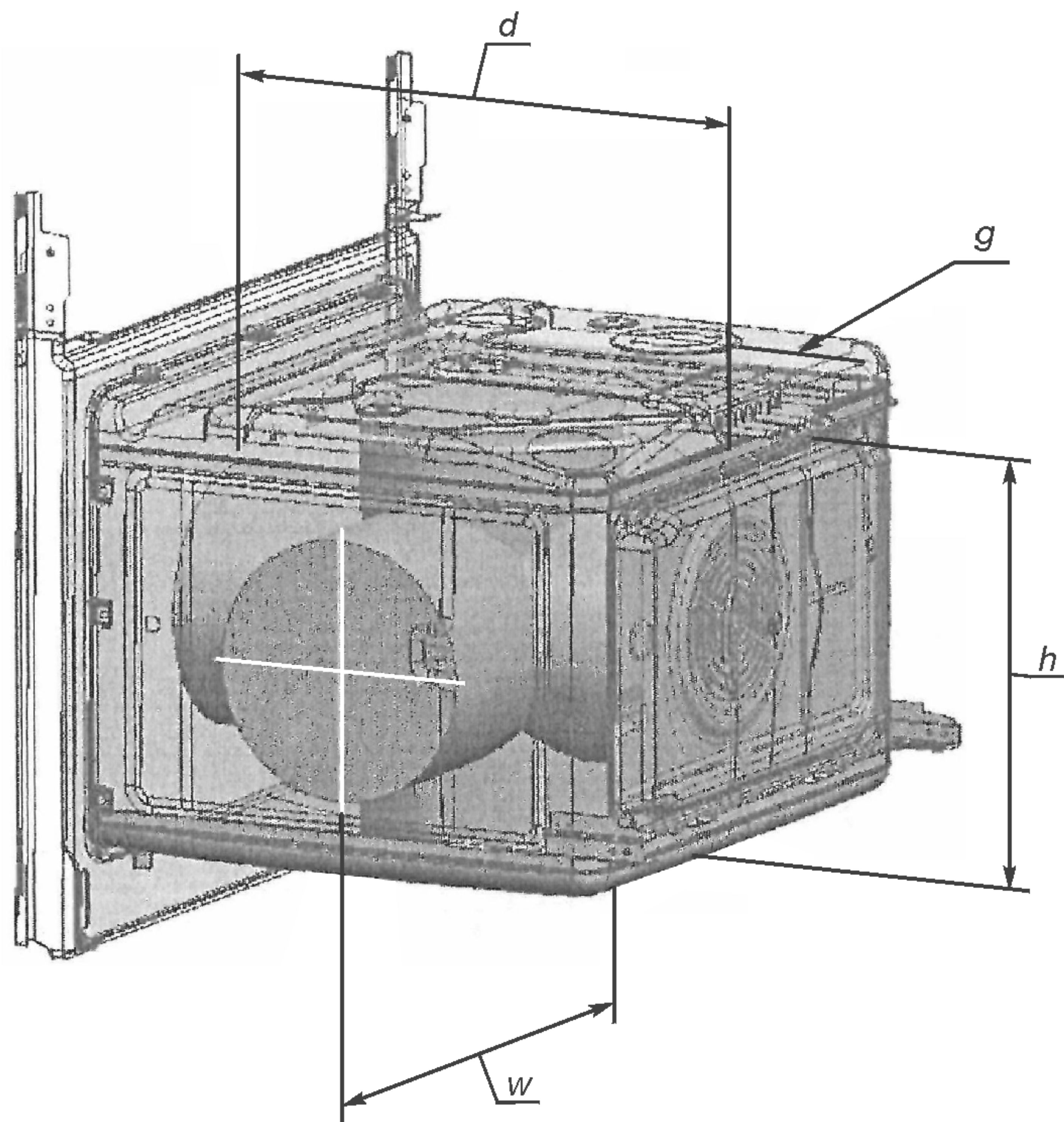
d — полезная глубина; g — нагревательный элемент; h — полезная высота; w — полезная ширина Рисунок 4а — Порядок проведения измерения
