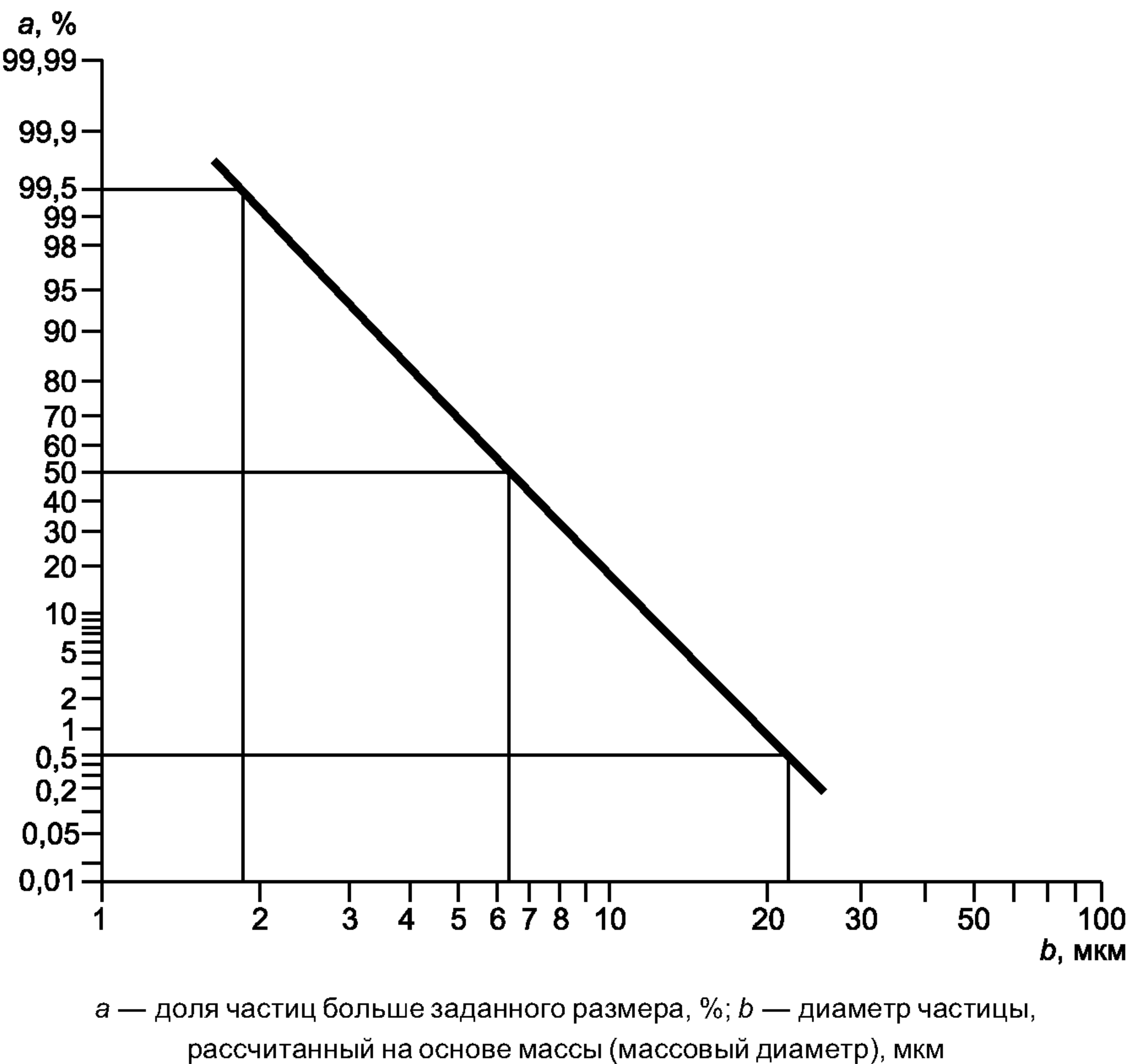
Рисунок 10 — Распределение частиц доломитовой пыли по размерам
