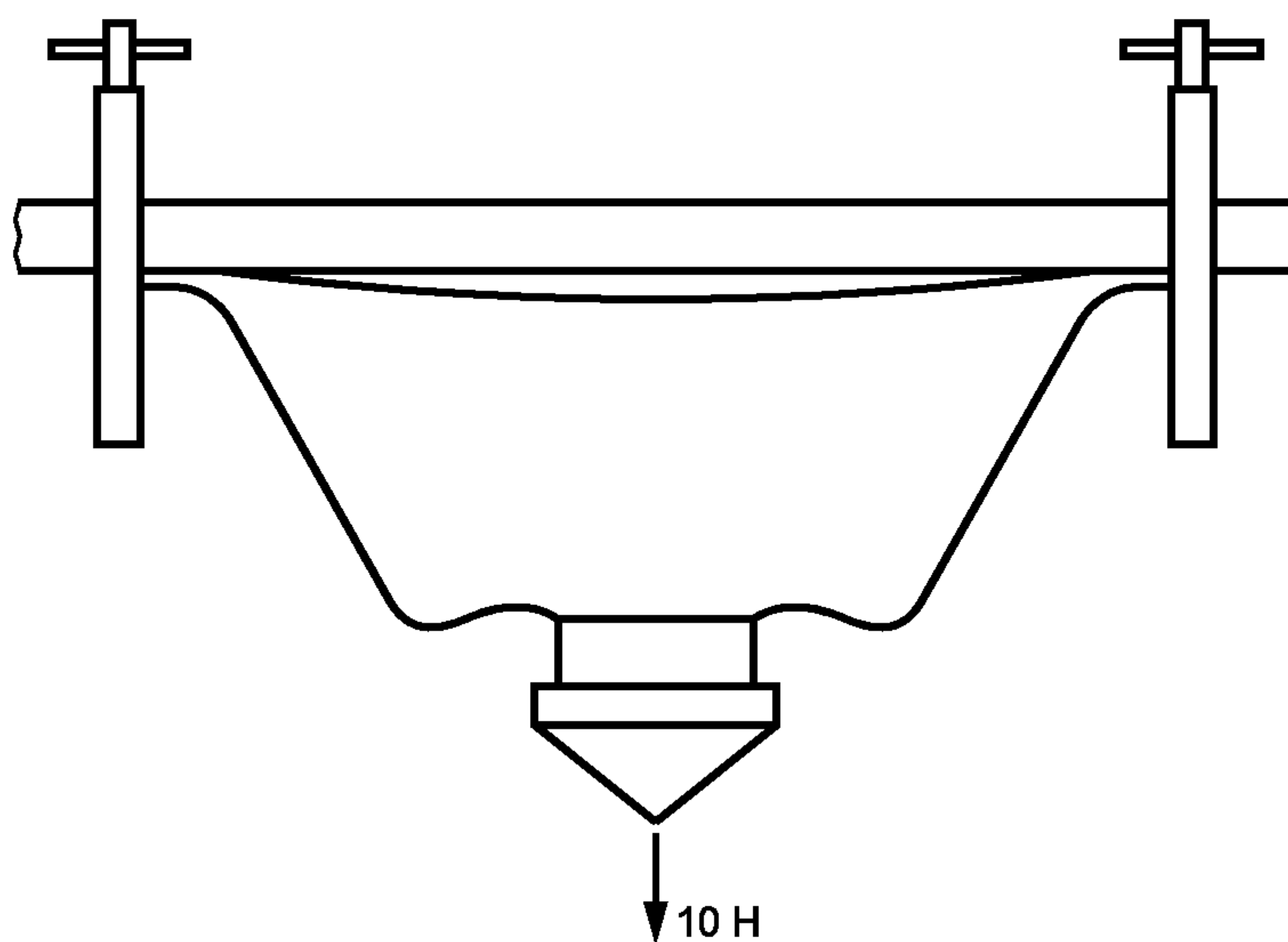
Рисунок 8 — Зажимное устройство для фильтрующей полумаски
