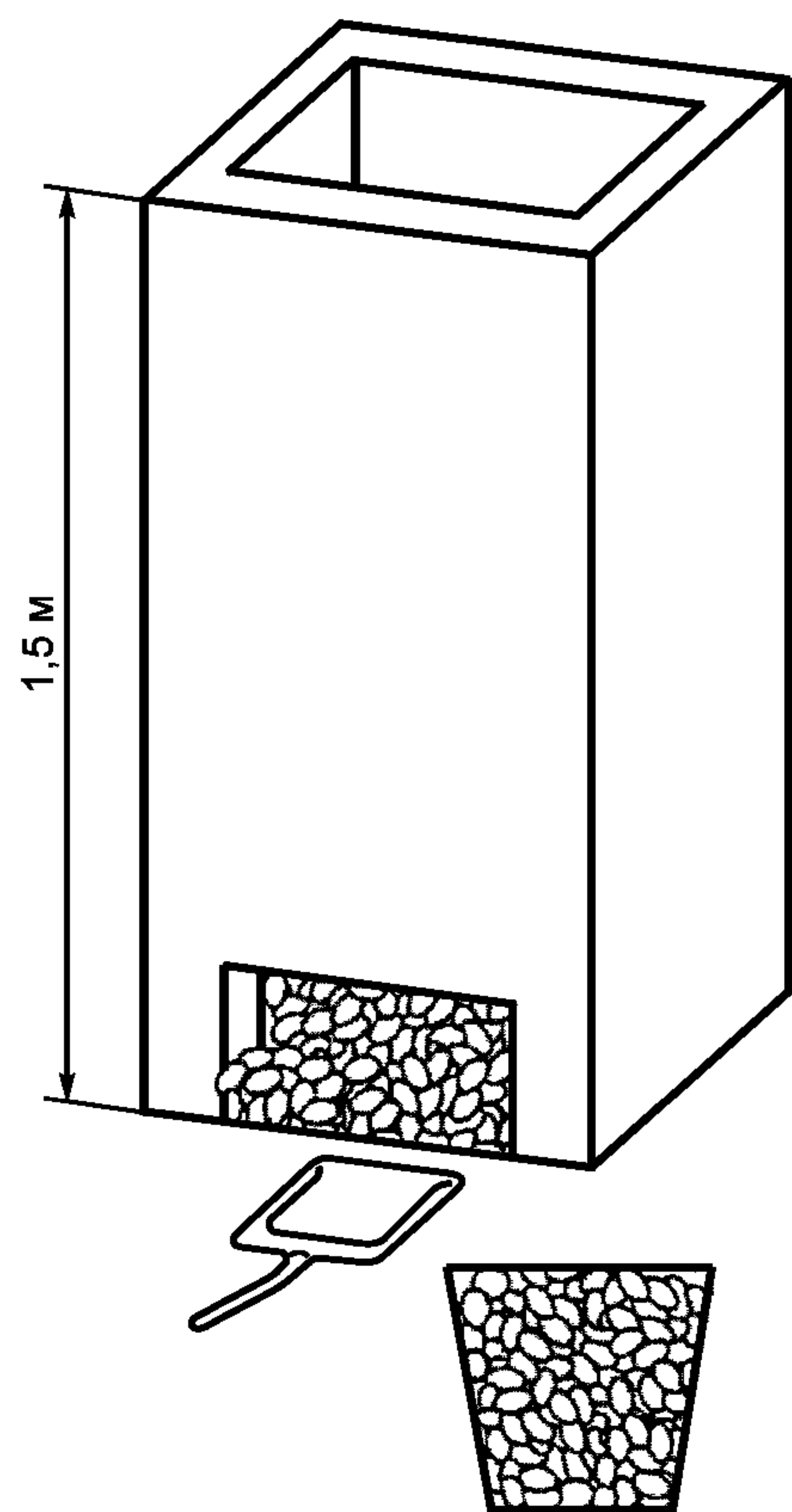
Рисунок 1 — Корзина и контейнер с резиновой стружкой
